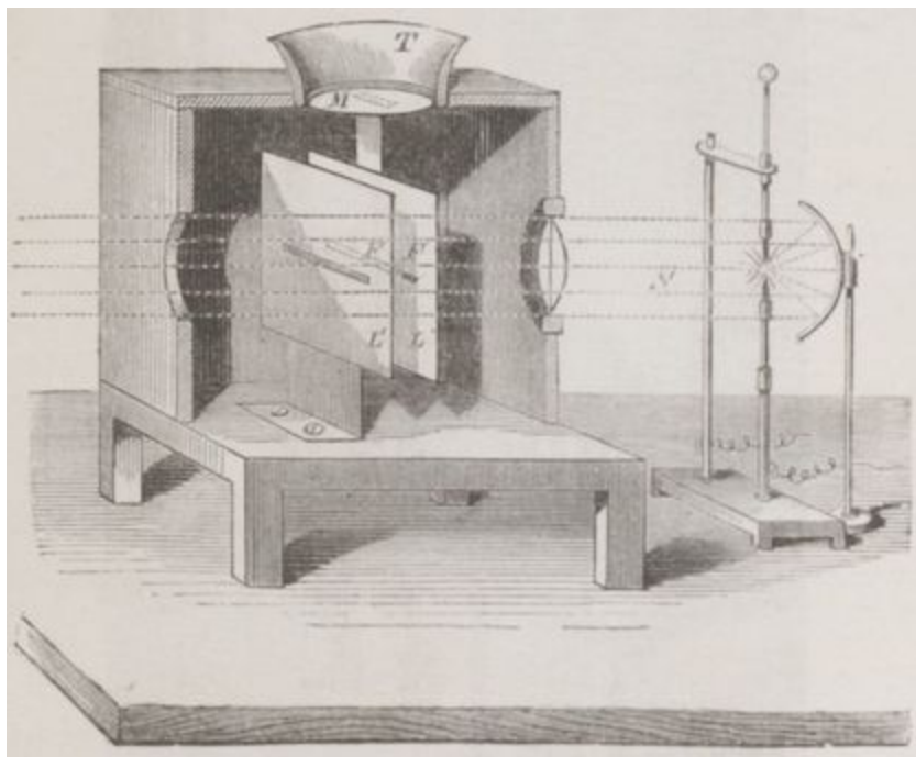
Le photophone (appareil expéditeur).
