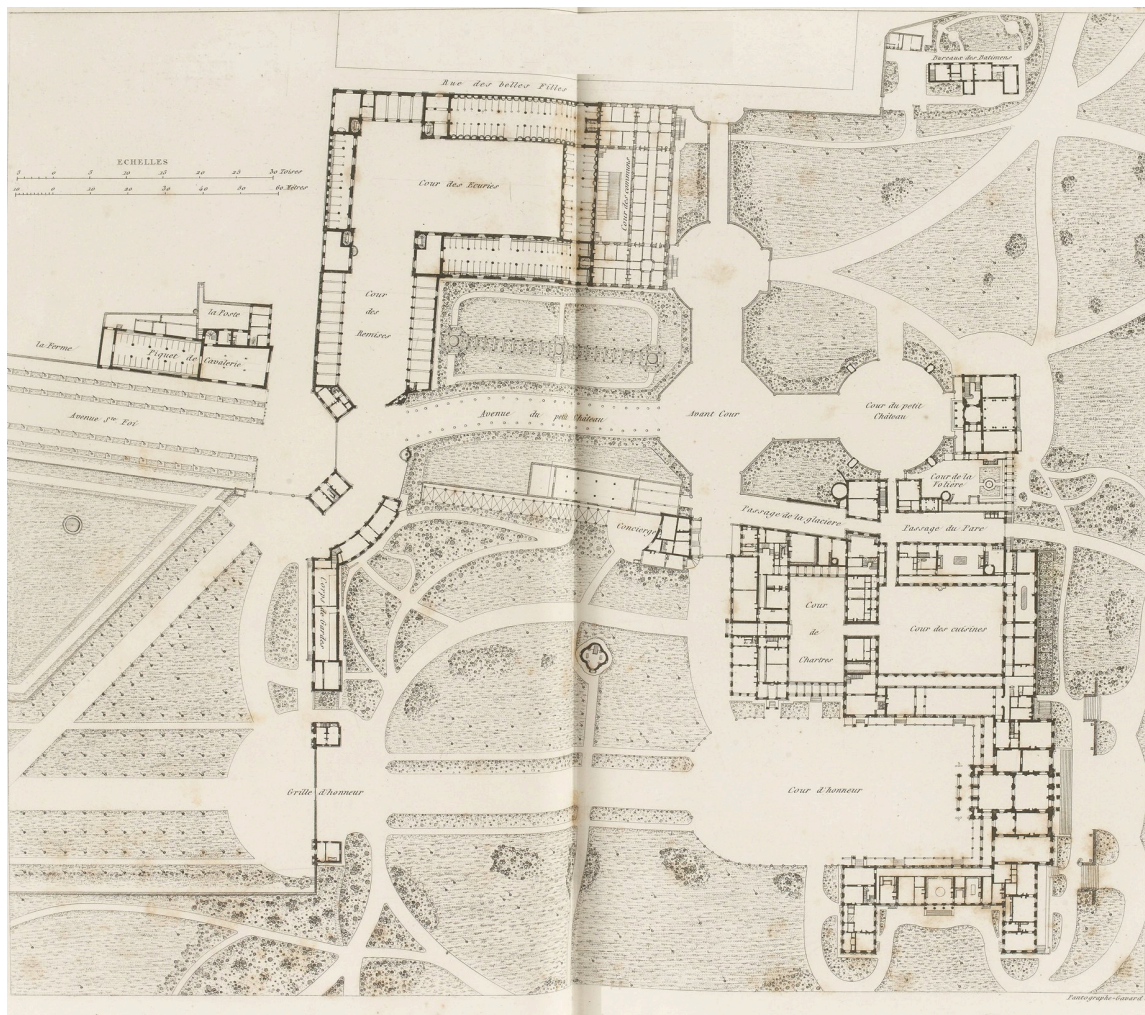
CHATEAU DE NEUILLY Plan général du Château et d'une partie des dépendances Rez-de-chaussée
