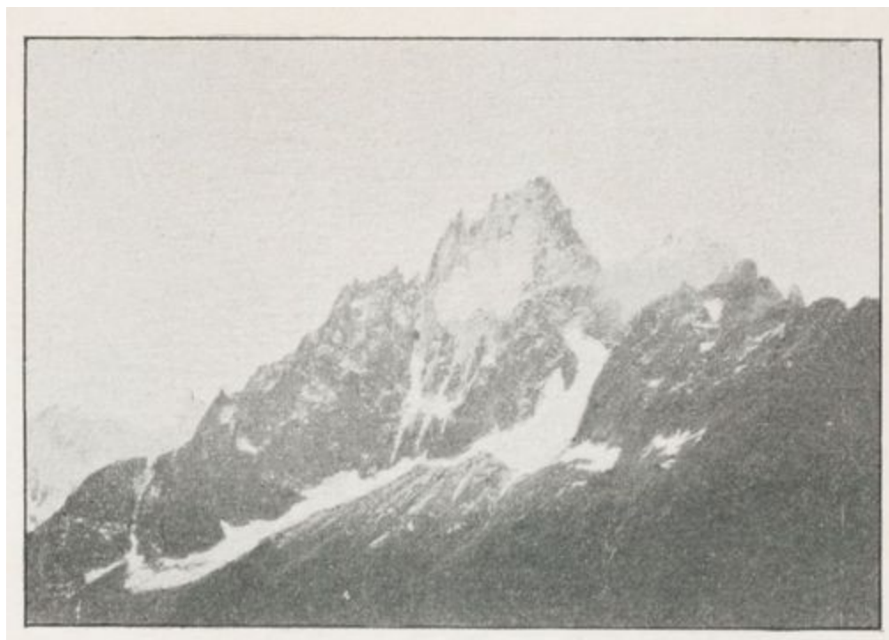
AIGUILLE DU CHARMOZ, VUE PRISE DE MONTANVERT
