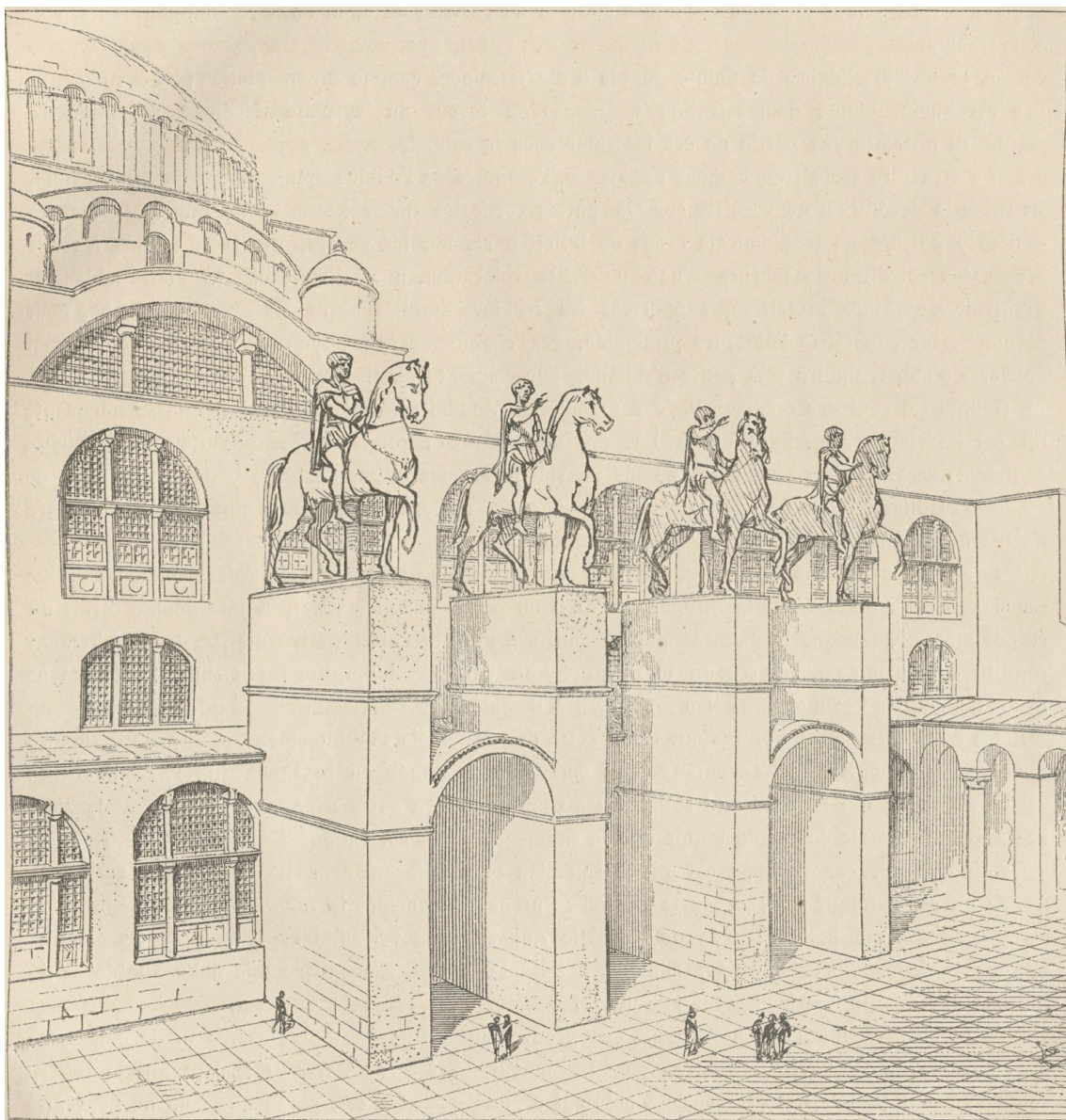
FIG. 17. – ENTRÉE PRINCIPALE DE SAINTE-SOPHIE DE CONSTANTINOPLE. EXONARTHEX.
