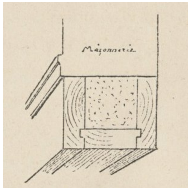
Fig. 13. – Pompei. Plates-bandes et poitraux.
