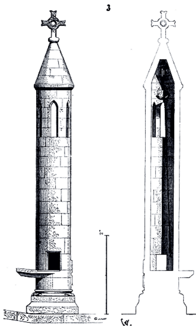
La fig. 3 présente l'élévation et la coupe de ce monument, bien conservé encore aujourd'hui. La lanterne est à claire-voie, de manière à laisser voir la lumière de tous les points de l'horizon.
