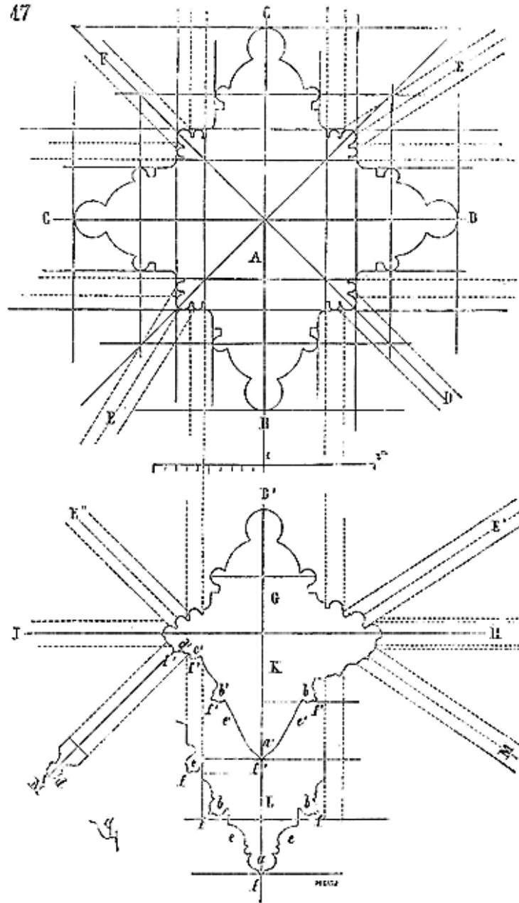
La figure 17 présente en A une des quatre piles du transept. Cette pile porte deux arcs-doubleaux B des grandes voûtes, deux archivoltes C de bas côtés, la branche d'arc ogive D de la voûte de la croisée, deux branches d'arcs ogives E
