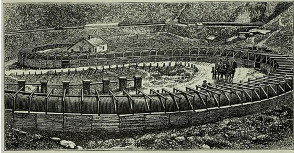
Parties couvertes du chemin de Fell (versant italien).
