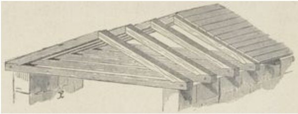
TOITURE AVEC CHEVRONS TENANT LIEU DE FORCES.
