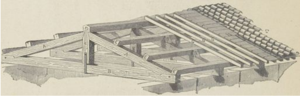
TOITURE AVEC CHEVRONS TENANT LIEU DE FORCES.
