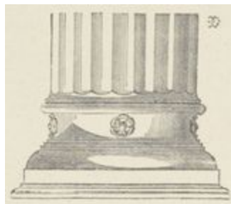
COLONNE DORIQUE DE VIGNOLE
