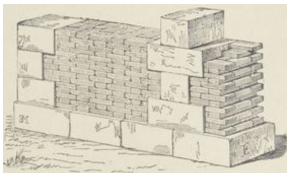
CHAINES DE PIERRES,
