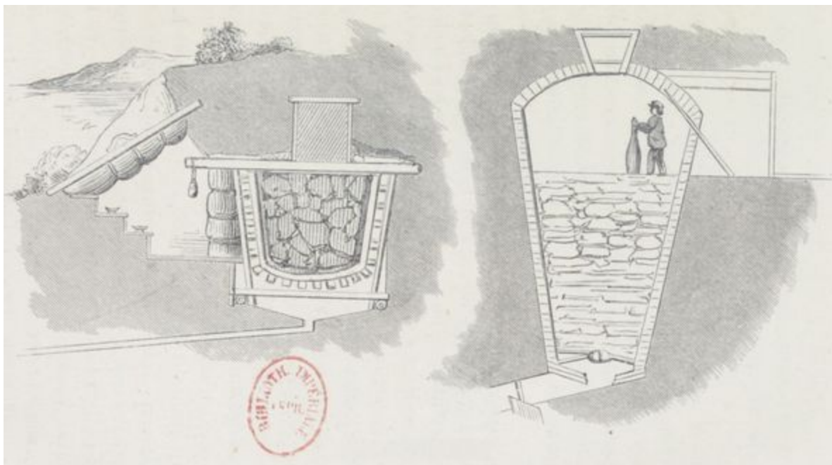
Glacières artificielles.
