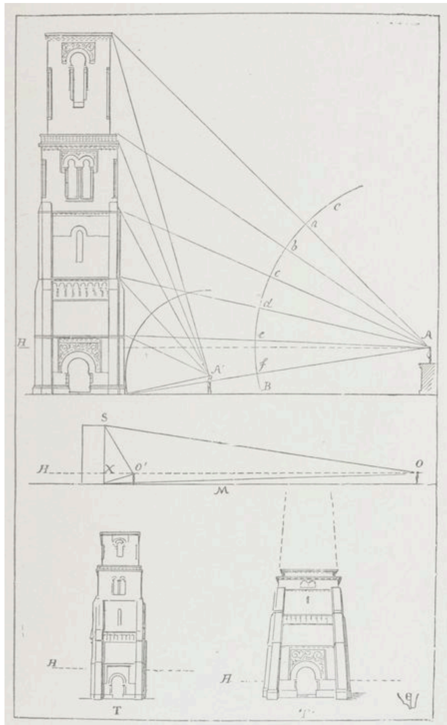
Fig. 42. — Déformations perspectives.
