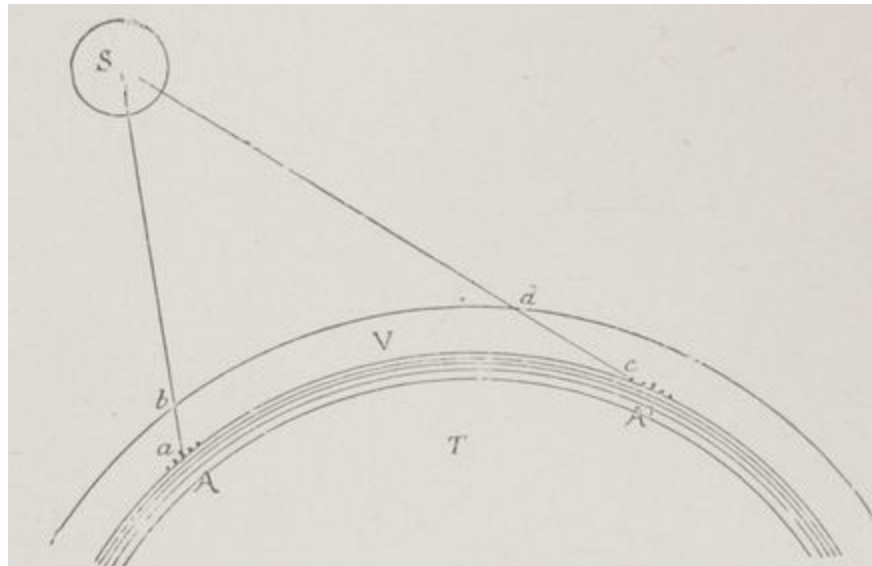
Fig. 22. — Pourquoi la lumière du soleil est colorée en rouge ou en jaune, le soir.
