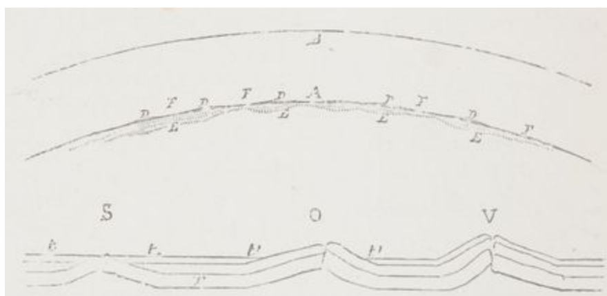
Fig. 101. — Refroidissement de la croûte terrestre et terrains sédimentaires.
