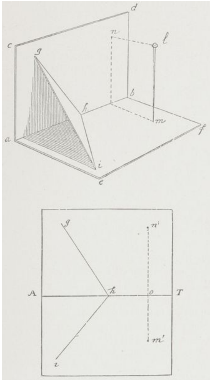
Fig. 37. — Géométrie perspective. (Premier exemple.)
