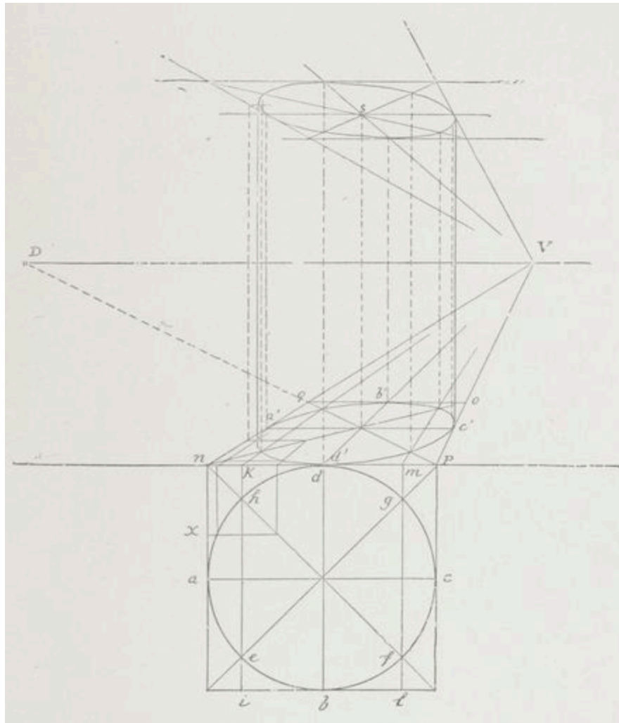
Fig. 39. — Perspective. (Neuvième exemple.)
