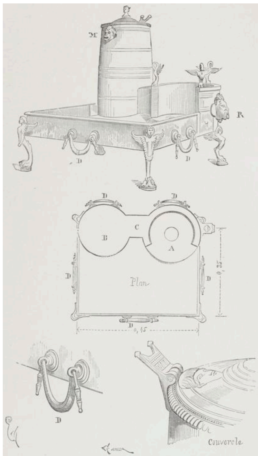
Fig. 85 — Cuisine portative, musée de Naples.
