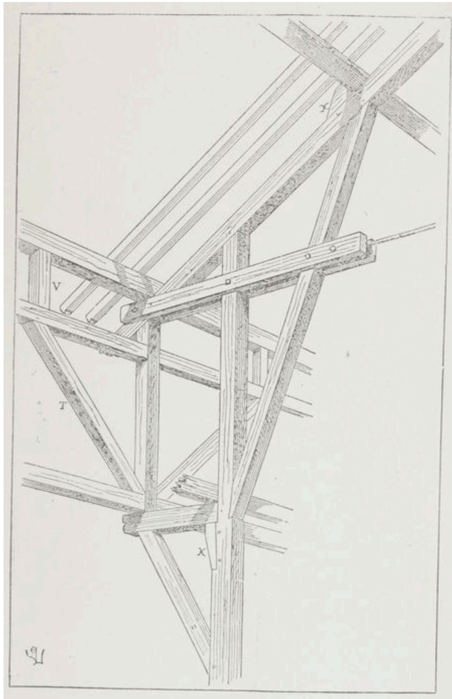
Fig. 69. Détail de charpente.
