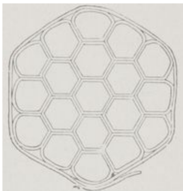
Fig. 11. — Réunion d'hexagones.
