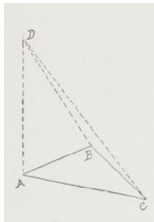
Fig. 18. — Tétraèdre irrégulier.
