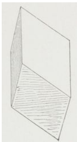
Fig. 19. — Rhomboèdre.
