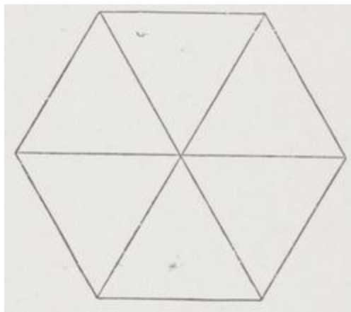
Fig. 13. — Hexagone régulier.
