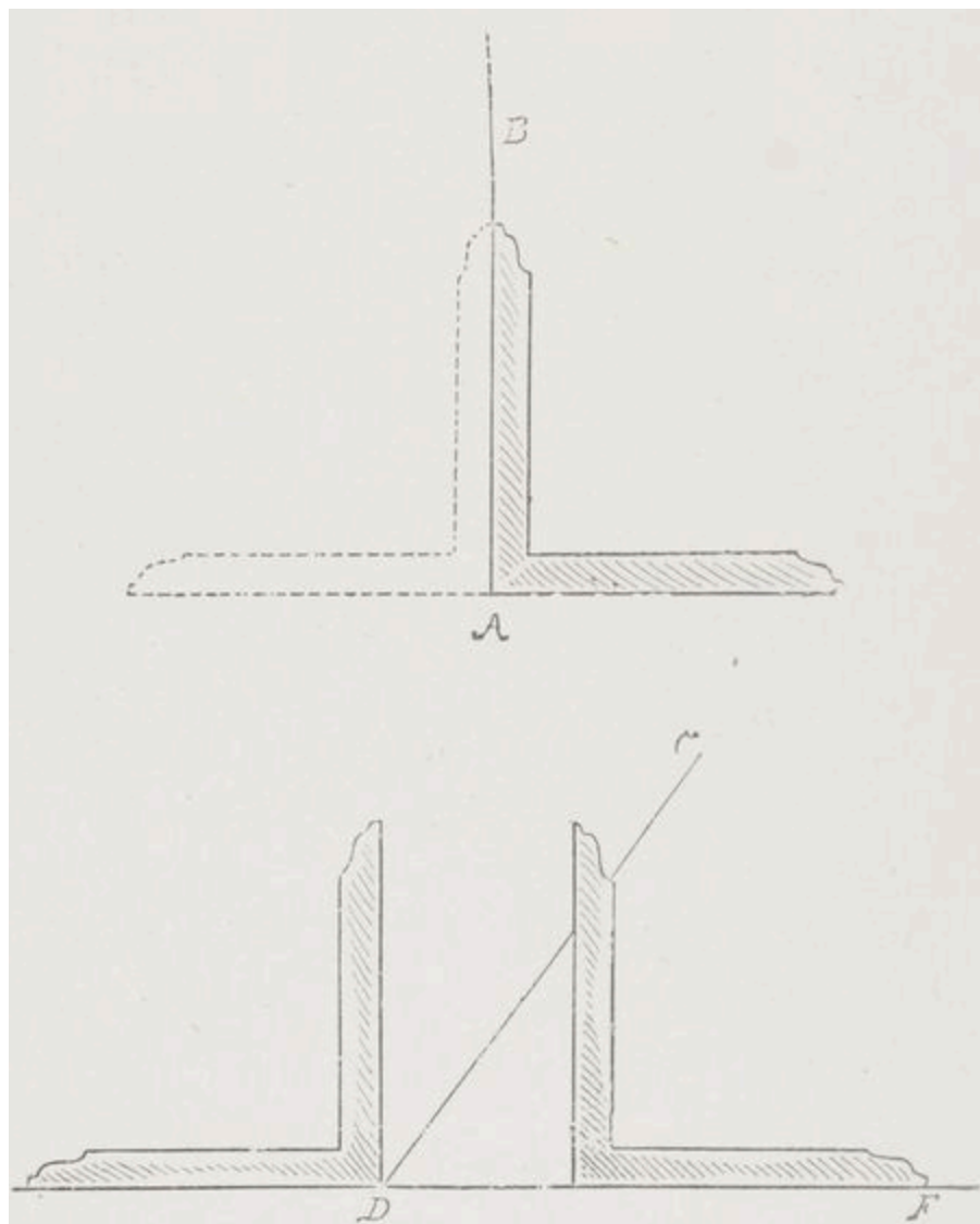
Fig. 3. - Angles droits, angles aigus, angles obtus.
