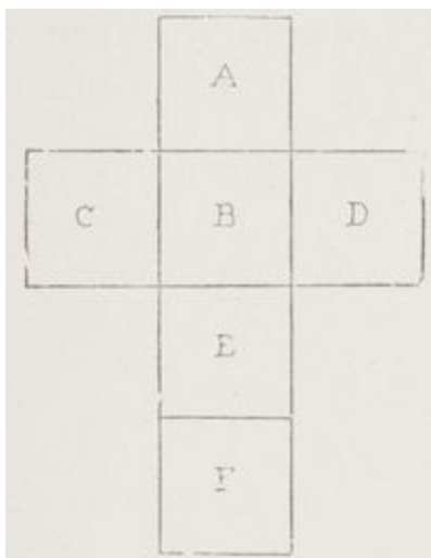
Fig. 14. — Développement du cube.
