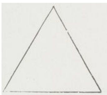
Fig. 12. — Triangle équilatéral.
