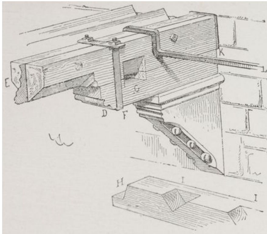
33. — ENCHEVÊTURES DE PLANCHERS (p. 113).
