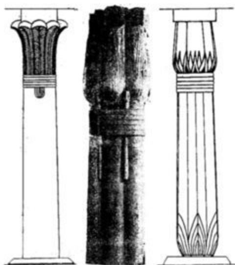
Fig. 107 et 108. Colonnes palmiforme et papyriforme (d'apr. BORCHARDT. Sahuré, p. 44; Ne-user-Ré, p. 64).
