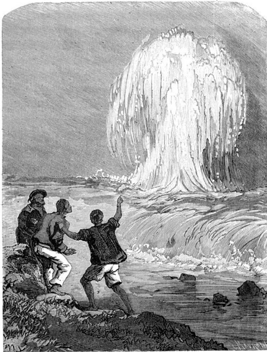
Fig. 77. — Éruption vaseuse.
