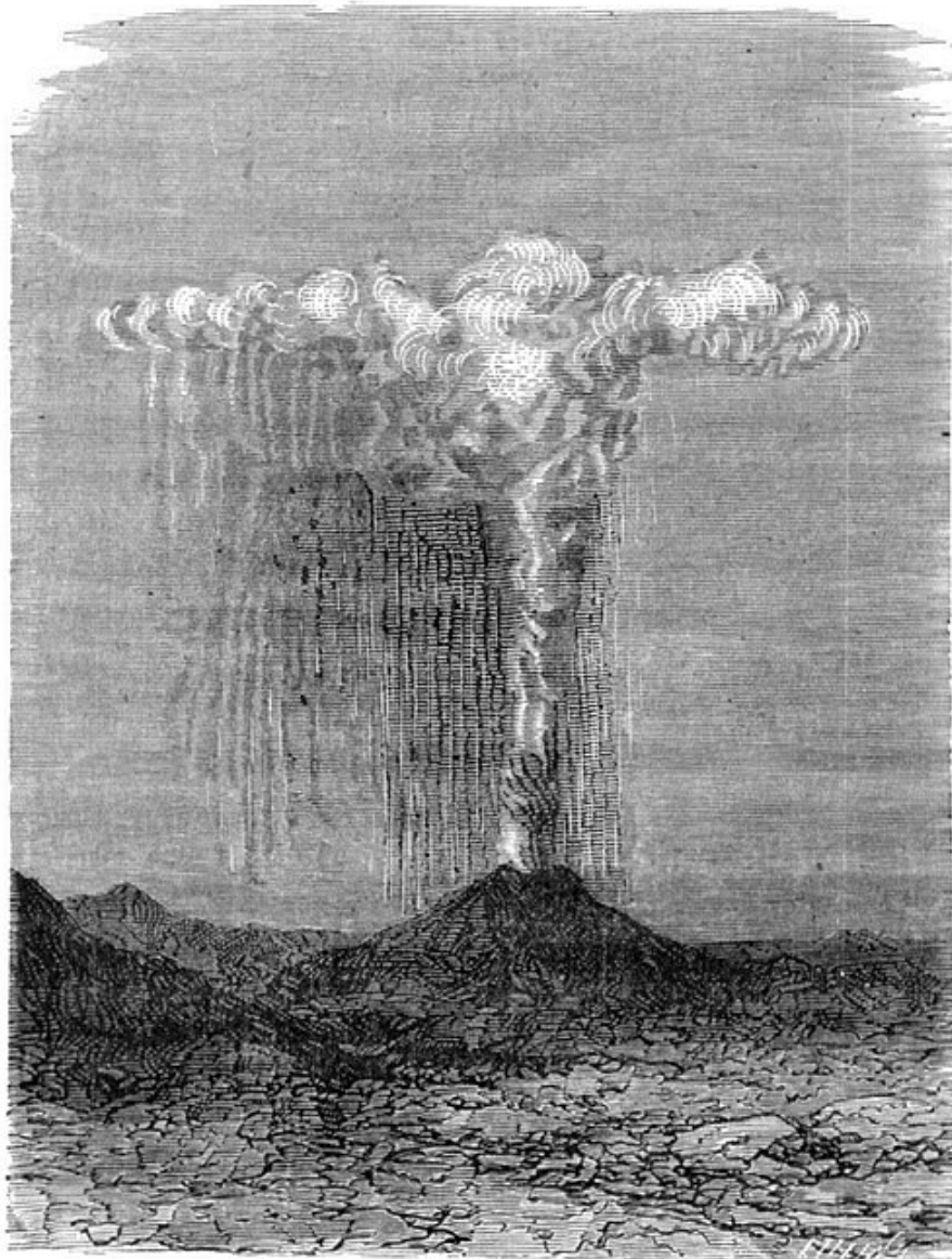
Fig. 78. — Éruption vaseuse.
