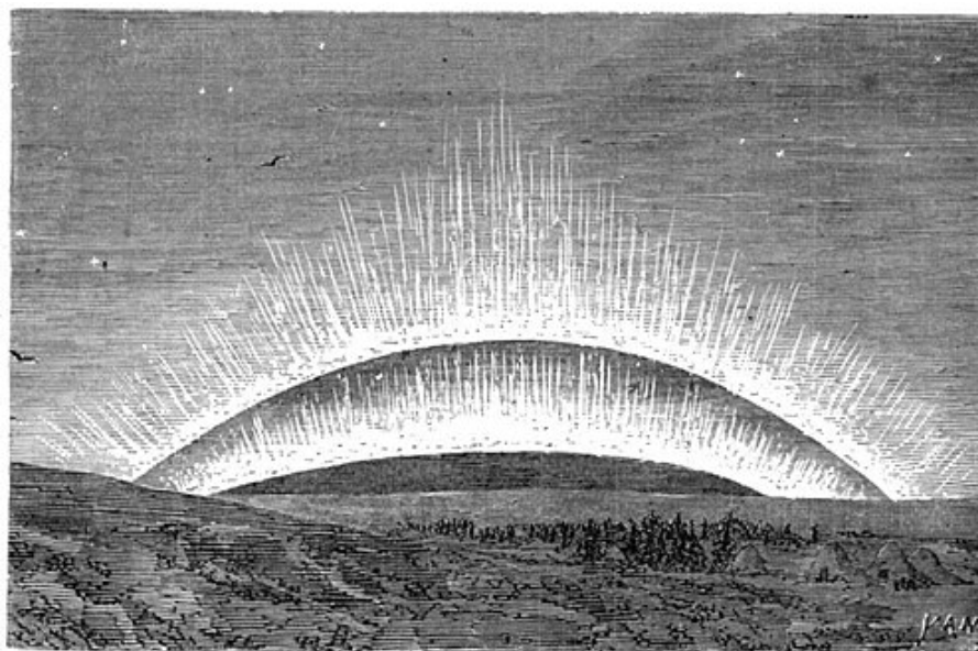
Fig. 72. — Arcs réguliers d'aurore boréale.
