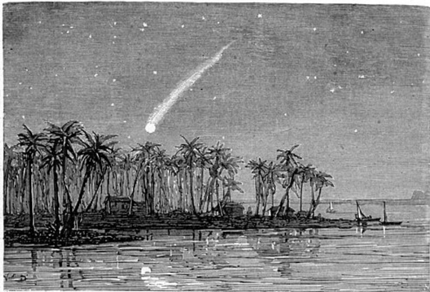
Fig. 87. — Étoile filante.
