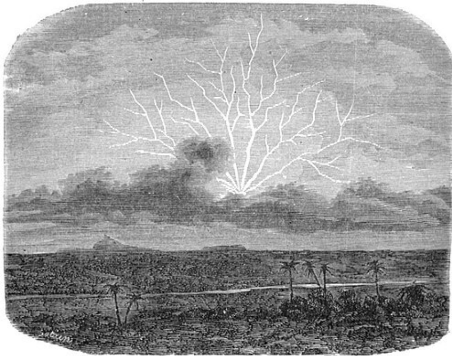
Fig. 66. — Éclair divisé et radié.
