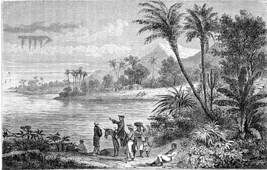
Fig. 60 — Mirage à l'île de France (vaisseau à quatre mâts).
