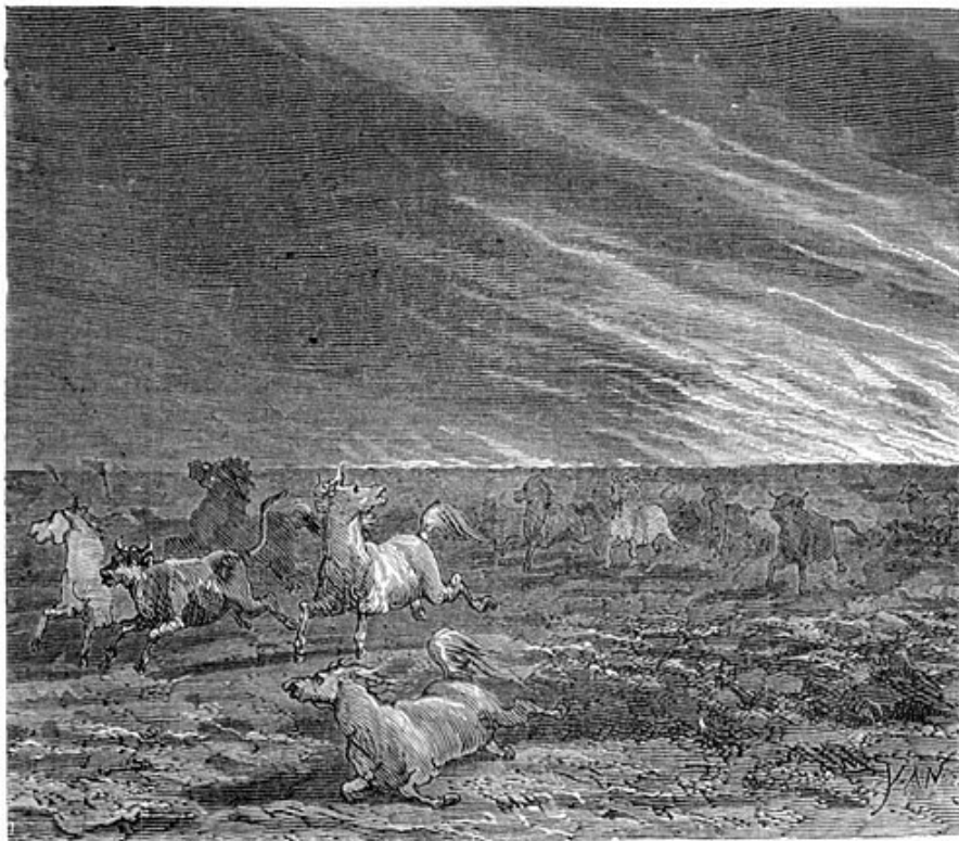
Fig. 12. — Incendie dans les campos.
