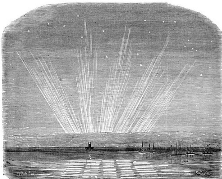
Fig 73. — Aurore boréale du 31 octobre 1853.
