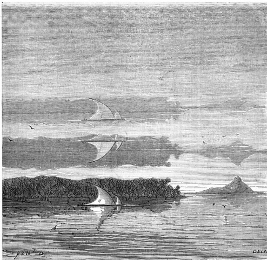
Fig. 61. — Mirage.
