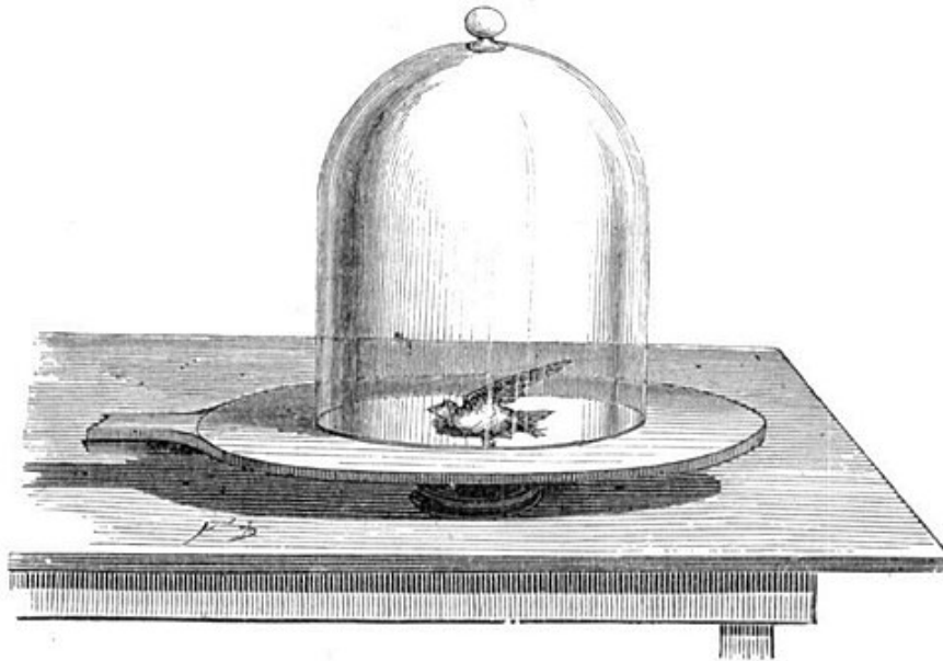
Fig. 28. — Oiseau sous la cloche de la machine pneumatique.
