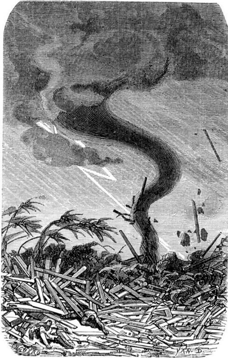
Fig. 50. — Trombe sur terre.
