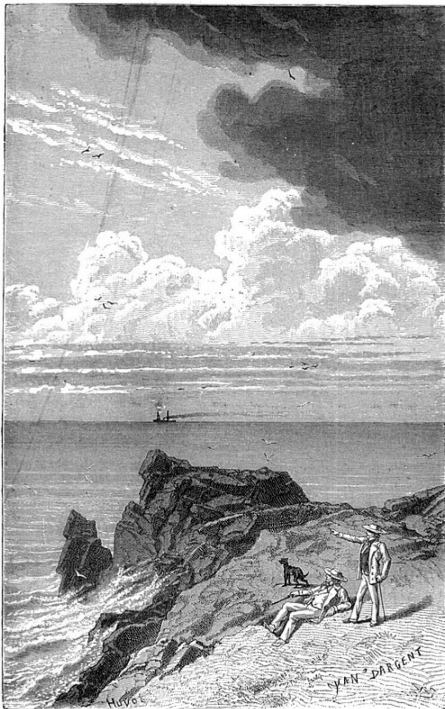
Fig. 37. — Diverses espèces de nuages. stratus, cumulus, cirrus, nimbus.
