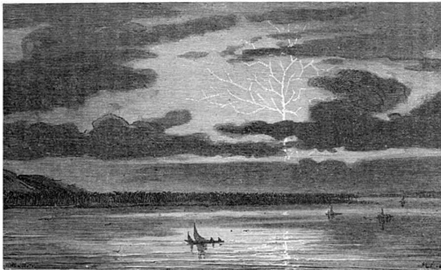
Fig. 65. — Éclairs arborescents.
