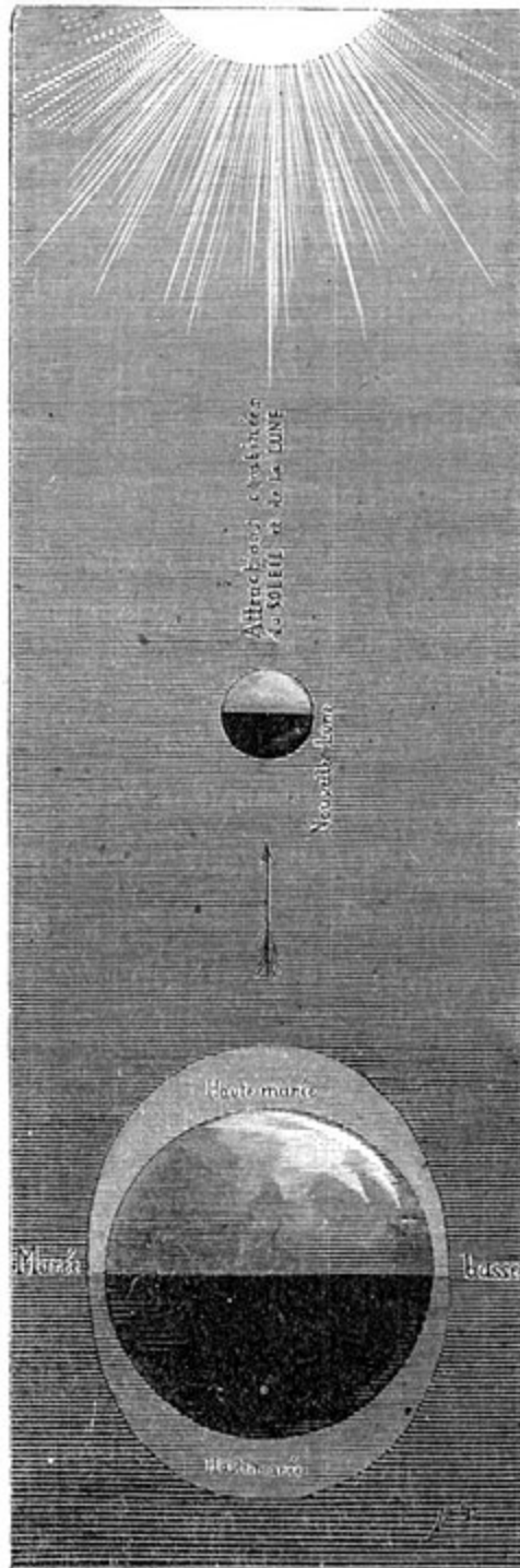
Fig. 44. - Phénomène des marées.
