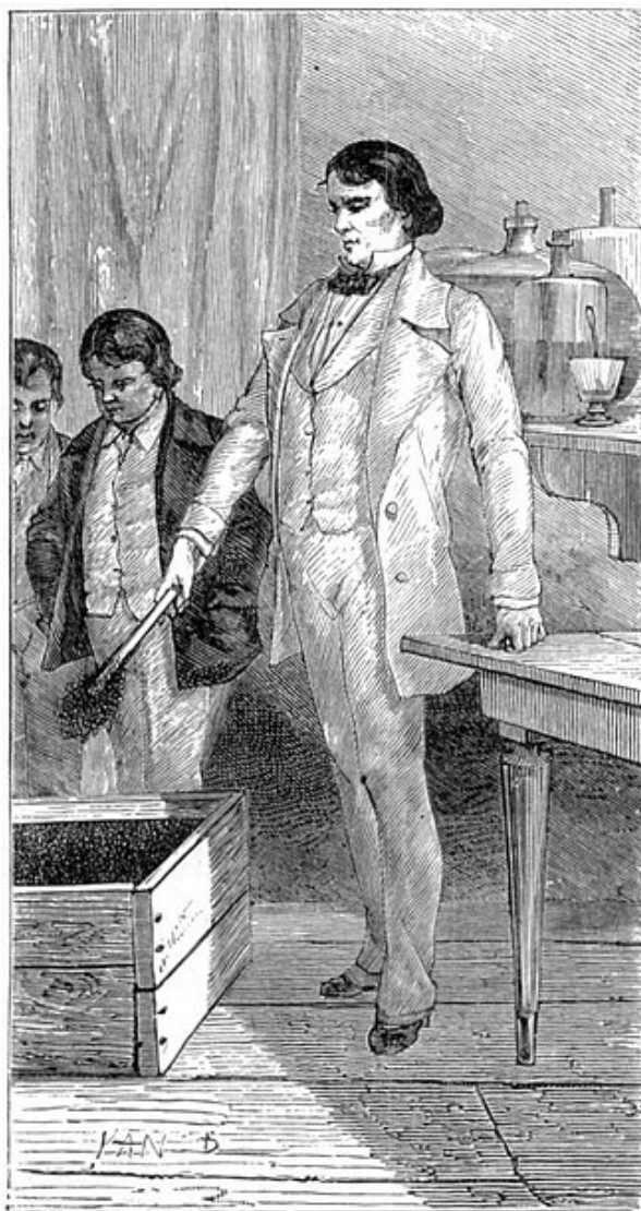
Fig. 22. — Limaille de fer portée par un aimant.
