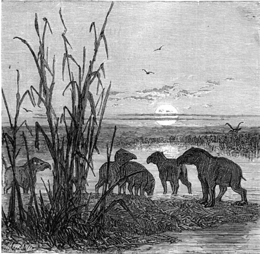
Fig. 36. — Brouillard d'horizon tranchant sur le soleil.
