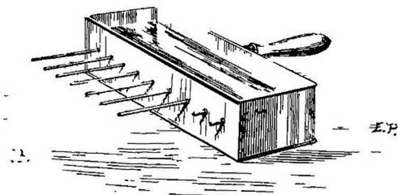
Fig. 9. — Appareil d'Ingenhousz pour comparer la conductibilité des différents métaux [2].
