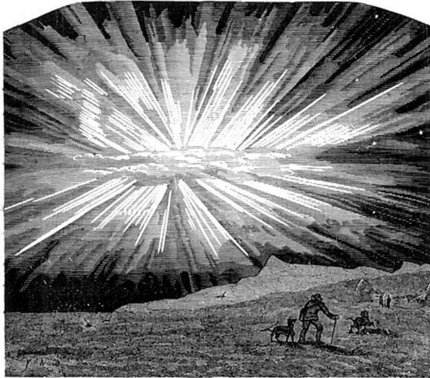
Fig. 71. — Couronne boréale.
