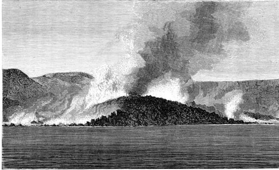
Fig. 84. — Volcans de Santorin.
