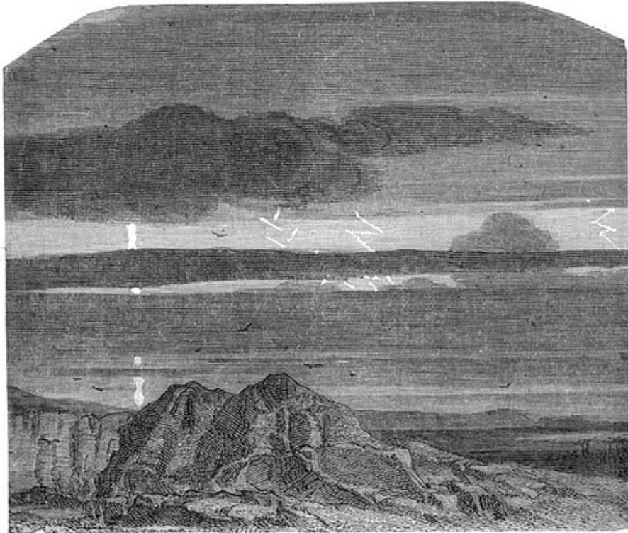
Fig. 67. — Diverses sortes d'éclairs simples.
