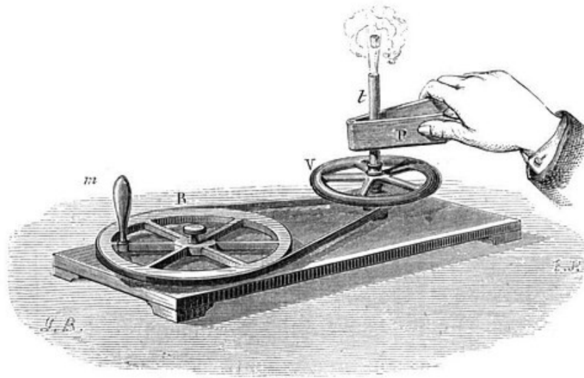
Fig. 7. — Appareil de M. Tyndall pour montrer la chaleur créée par le travail détruit [1] .
