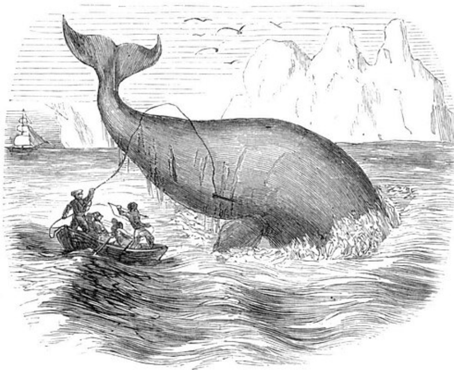
Fig. 46. — Baleine franche.
