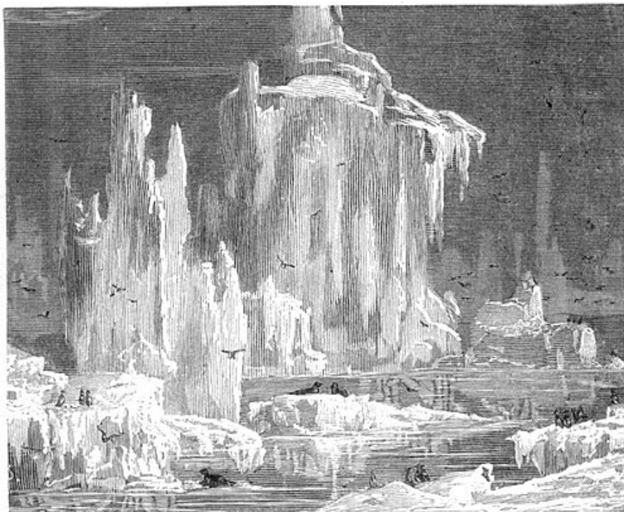
Fig. 48. — Montagnes de glace des pôles.
