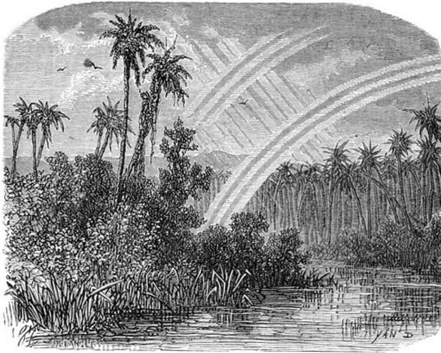
Fig 59. — Arc-en-ciel.
