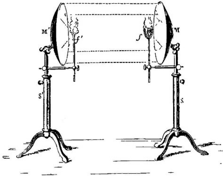
Fig. 8. — Miroirs démontrant les lois de la réflexion des rayons calorifiques [1] .
