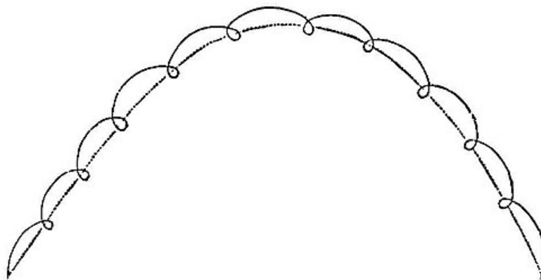
Fig. 53. — Mouvement du cyclone sur sa parabole.
