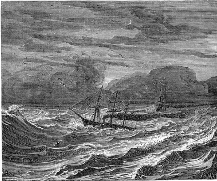
Fig. 53. — Ouragan.
