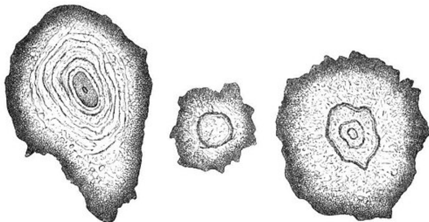
Fig. 40. — Coupe de différents grêlons.
