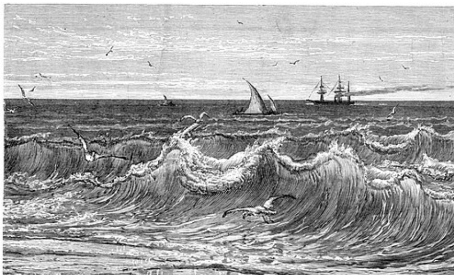
Fig. 57. — Vagues se brisant au rivage.
