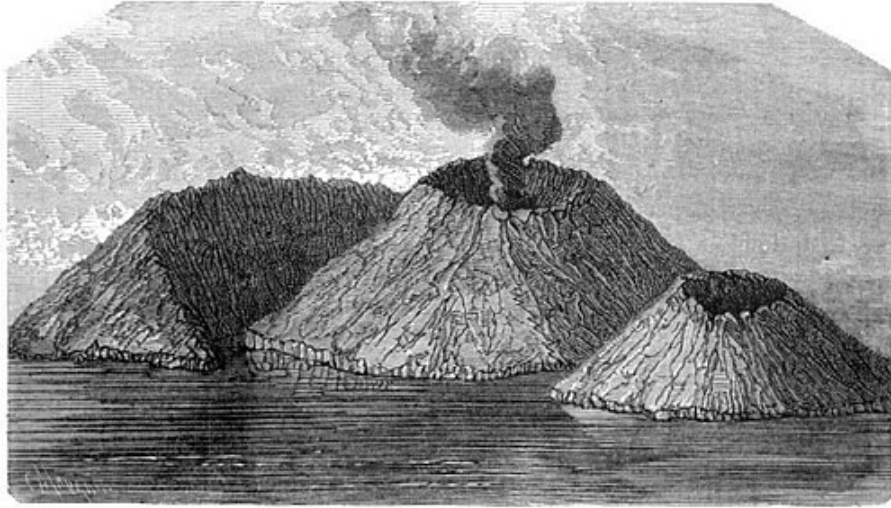
Fig. 76. — Volcano et volcanello.
