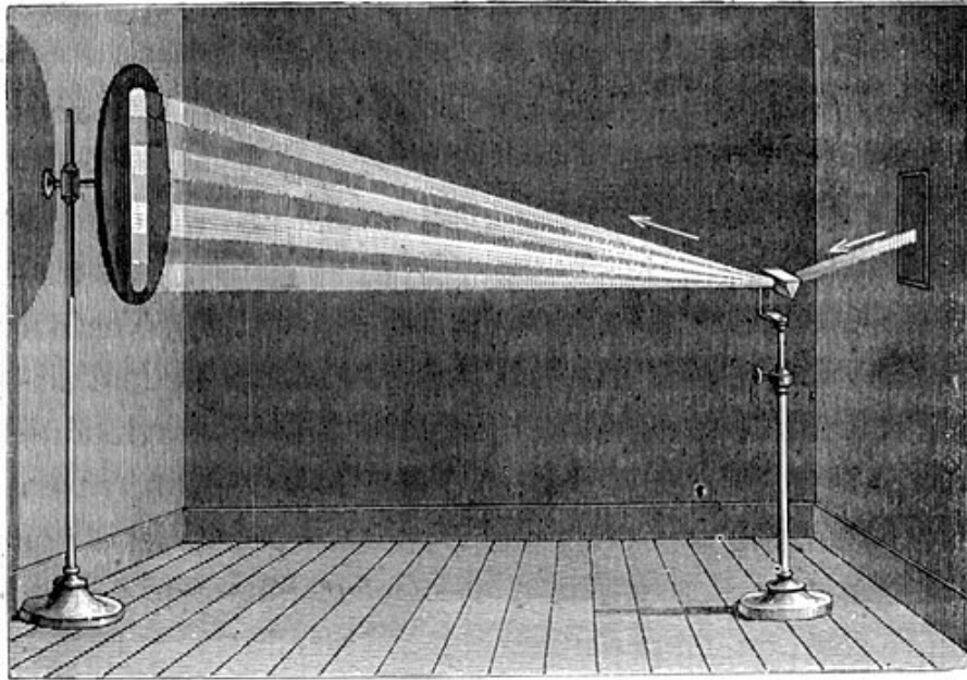
Fig. 13. — Spectre solaire.
