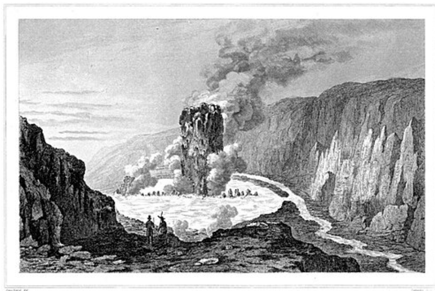
Cratère du Krabla.
