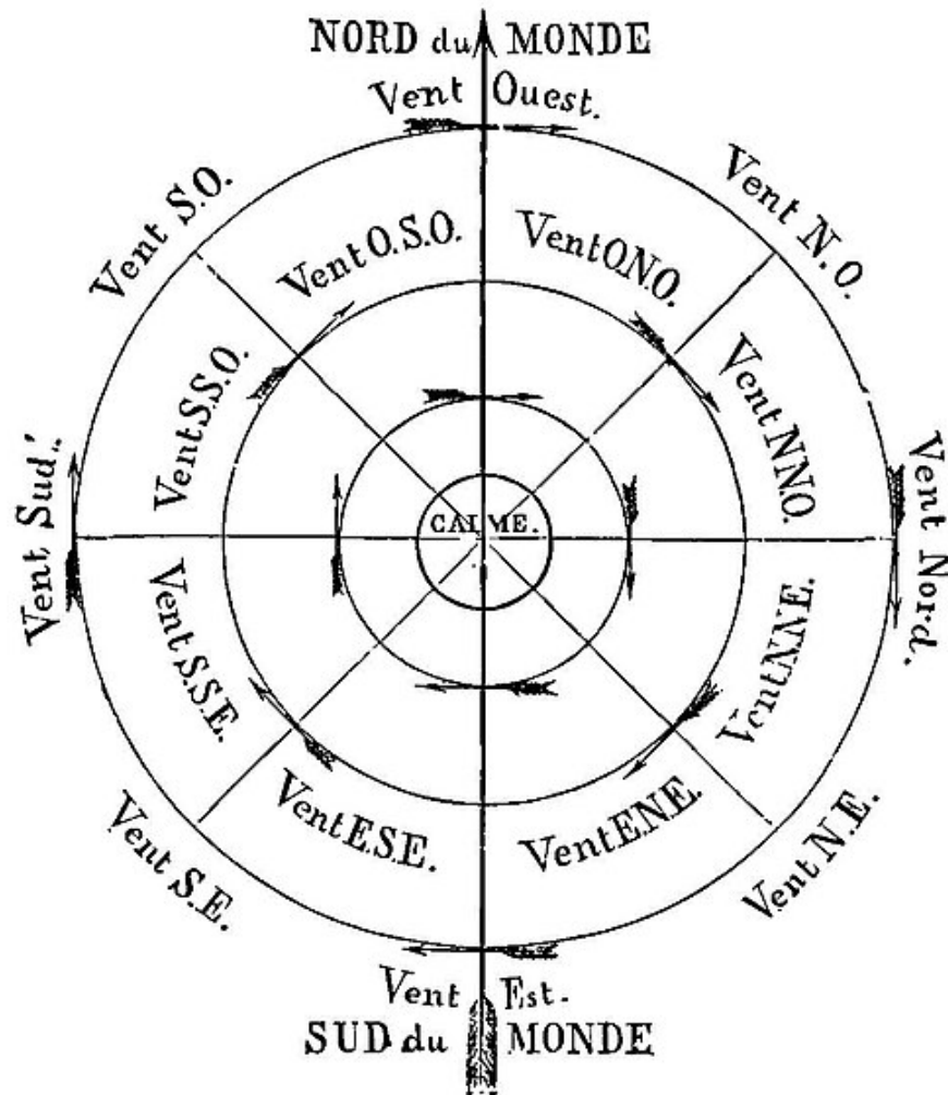
Fig. 54. — Mouvement circulaire du cyclone.
