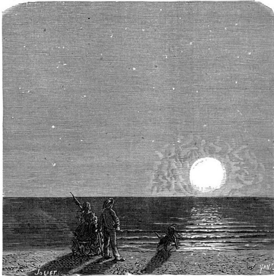
Fig. 62. — Phénomènes de réfraction.
