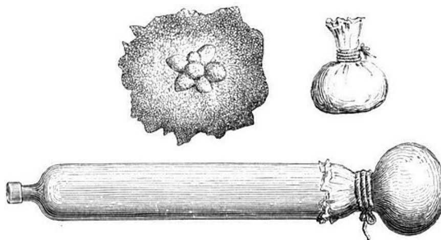
Fig. 41. — Formation des grêlons ; appareil de M. Sanna-Solaro.
