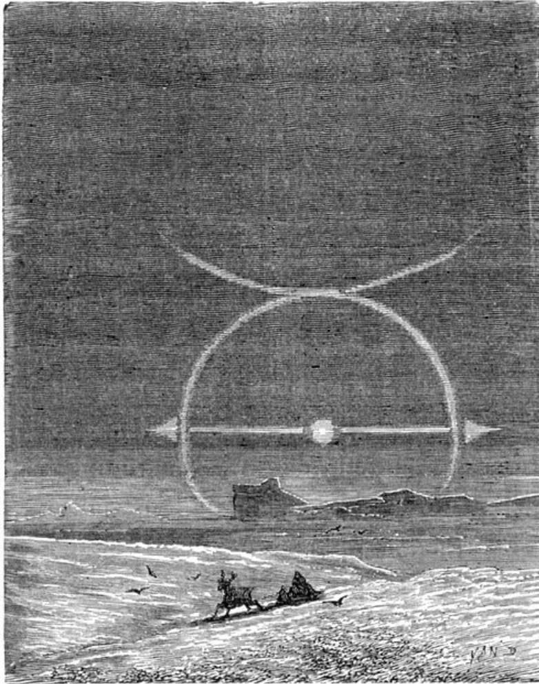
Fig. 63. — Parasélène.
