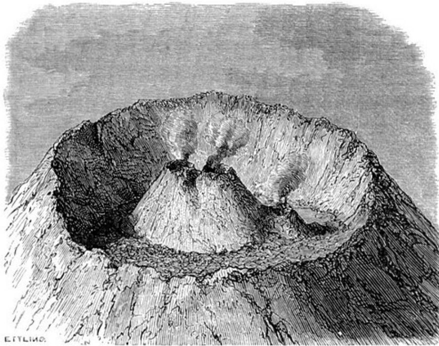
Fig 82. — Cratères du Vésuve.
