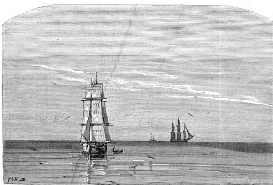
Fig. 43. — Mer calme.
