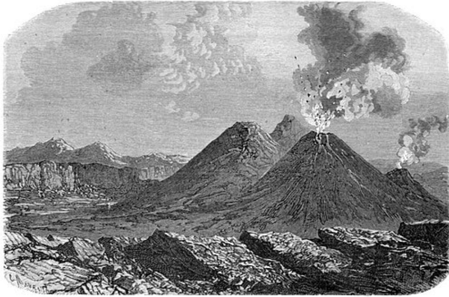
Fig. 5. — Volcan de la Réunion.
