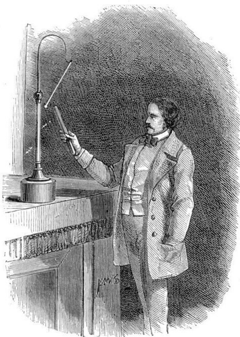
Fig. 17. — Pendule électrique. — Répulsion électrique.
