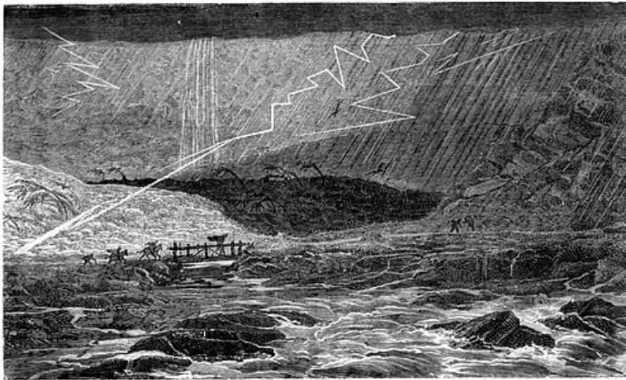
Fig. 56. — Orages au pied des montagnes.
