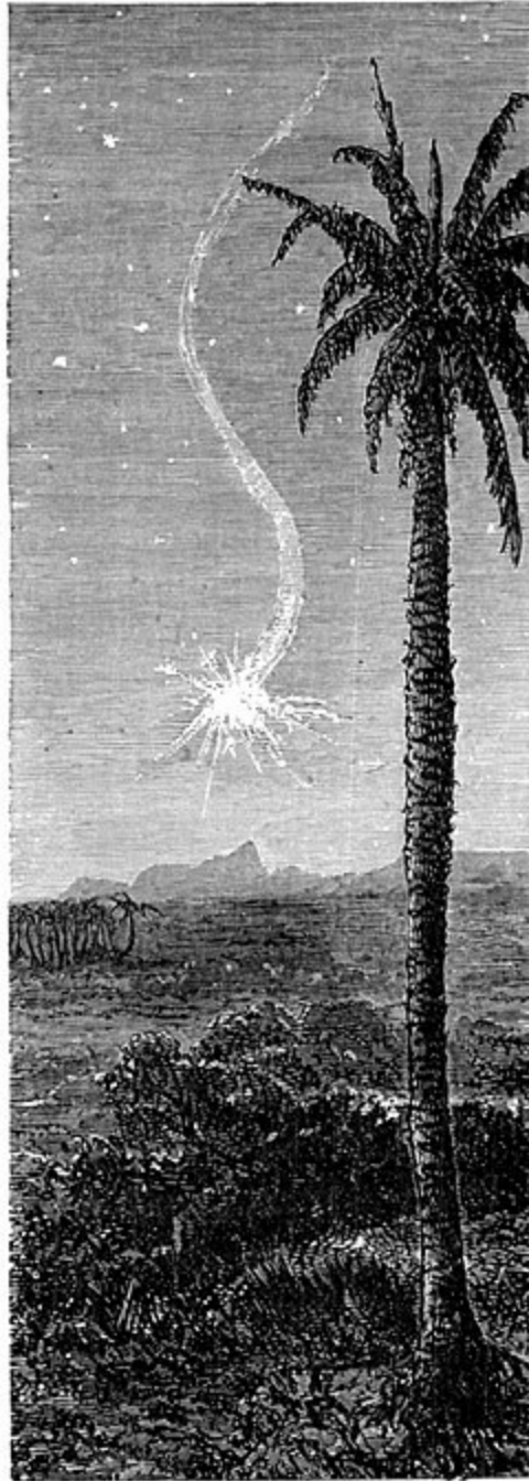
Fig. 88. — Étoile filante.
