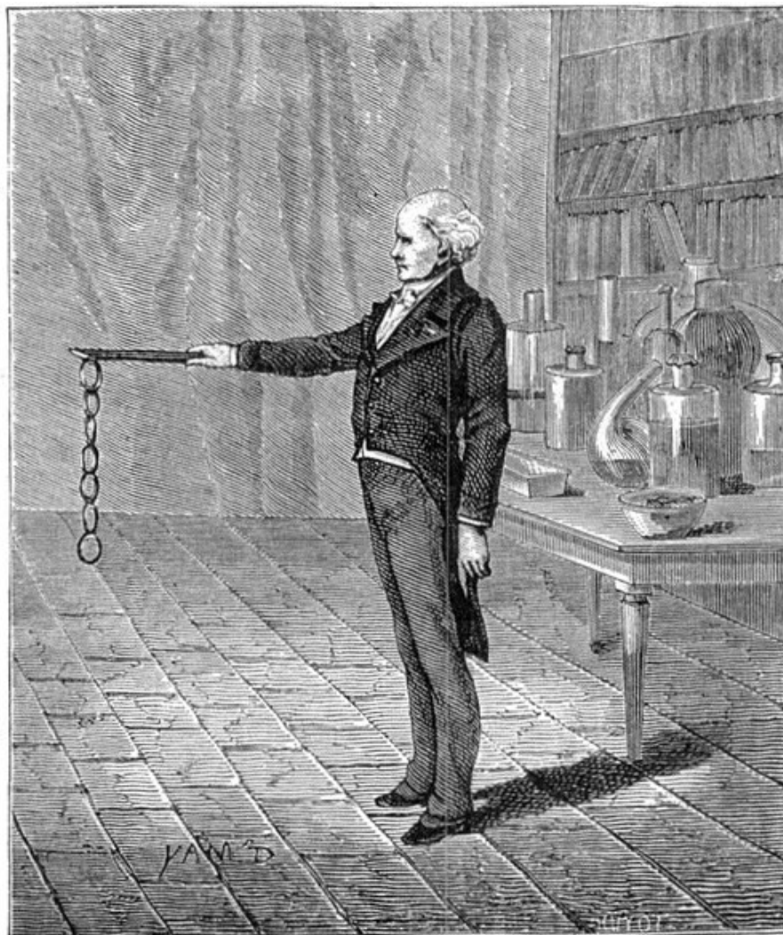
Fig. 20. — Aimantation par influence.
