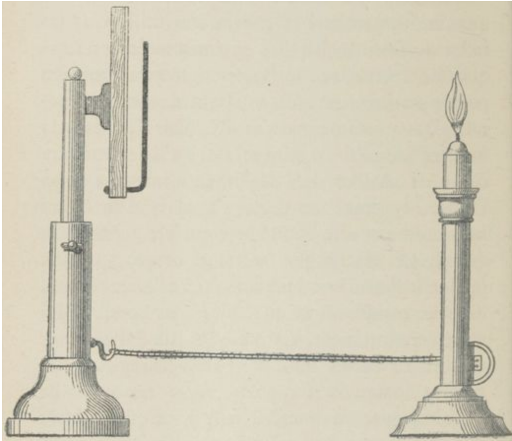
Fig. 32. — Photomètre de Bertin-Sans.
