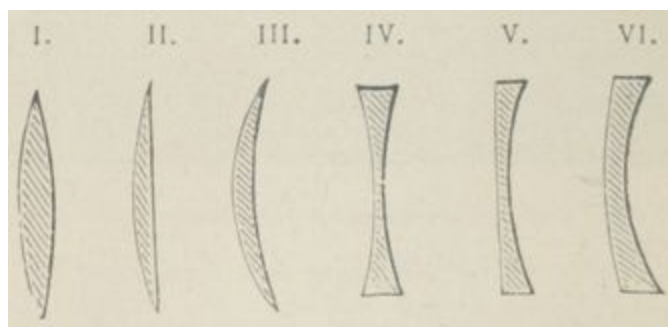
Fig. 18. — Formes diverses de lentilles 18 .
