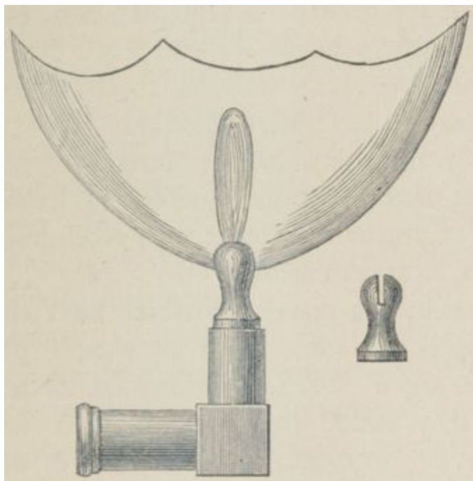
Fig. 28. — Bec de gaz dit à papillon.
