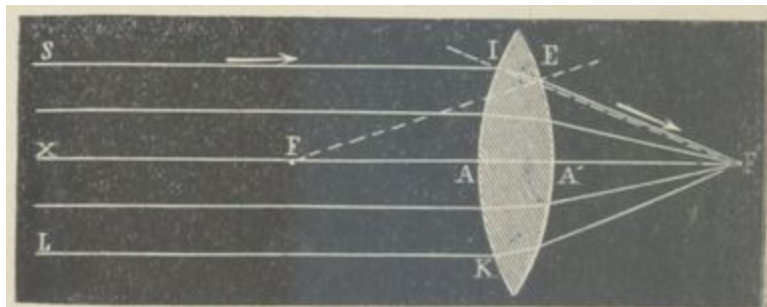
Fig. 16. — Foyer principal d'une lentille biconvexe 16 .
