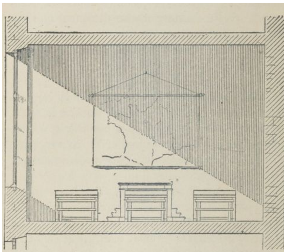
Fig. 30. — Éclairage unilatéral : la baie d'éclairage doit être assez grande pour assurer à toutes les places indistinctement la même quantité de lumière.
