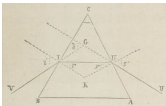
Fig. 17. — Réfraction dans un prisme 17 .
