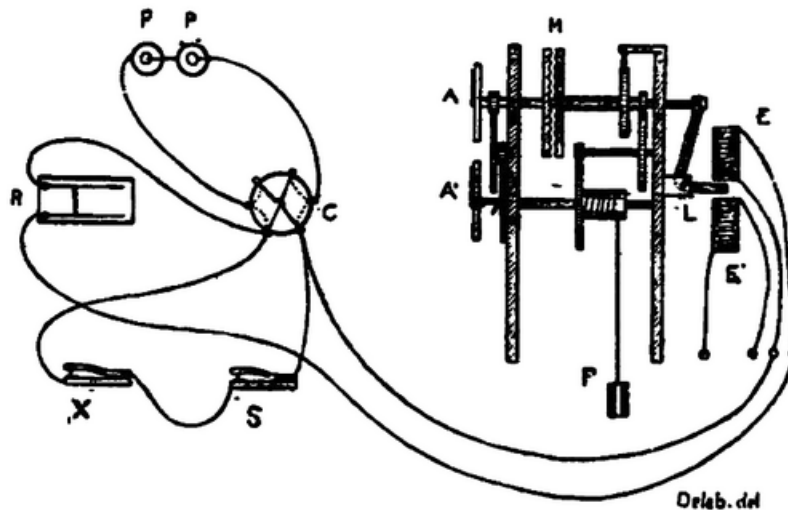
Fig. 9. — Chronoscope de Hipp. AA', les deux cadrans ; — EE', les deux aimants ; — L, le levier ; — M, l'engrenage ; — C, commutateur ; — R, rhéostat ; — PP, piles ; — SX, contacts.
