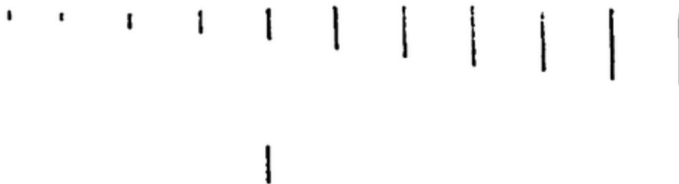
Fig. 8. — Série de lignes employées pour l'étude de la mémoire par la méthode de reconnaissance . Au-dessous de la série, se trouve la ligne modèle à retenir.
