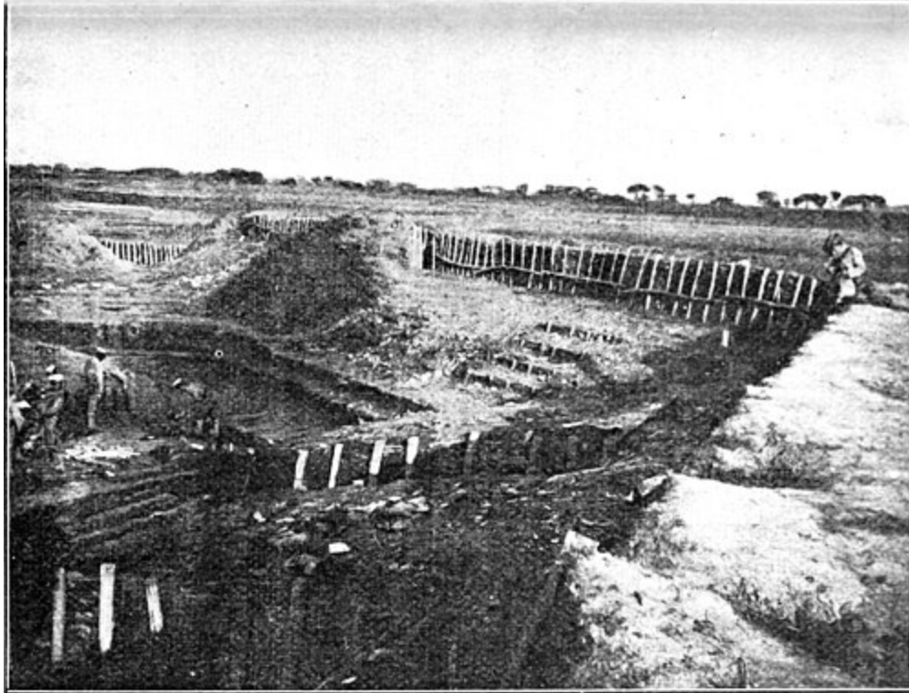
Redoute de Liaoyang ; parapets et revêtements.
