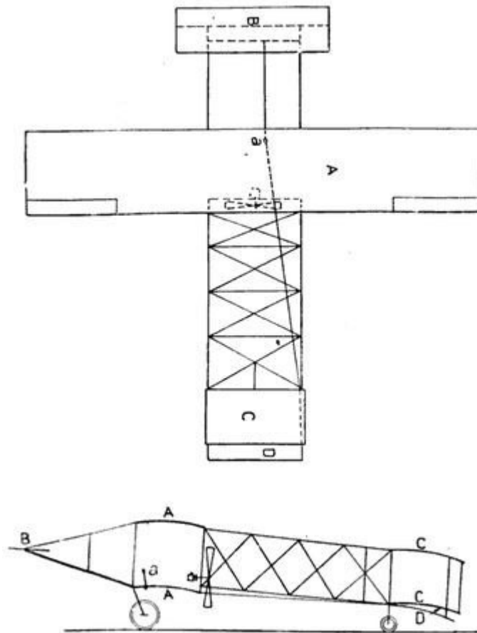
FIG. 142 et 143.—Biplan GOUPLY ET VOISIN.
