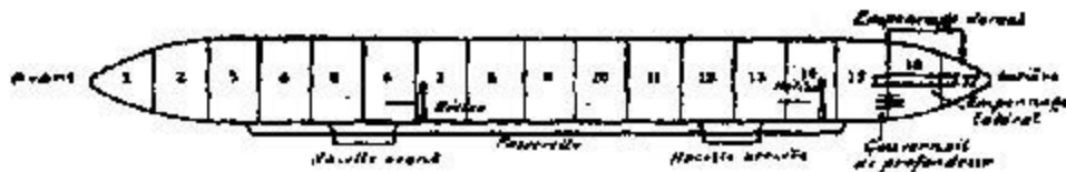
FIG. 11.—Coupe longitudinale montrant le cloisonnement du Zeppelin .
