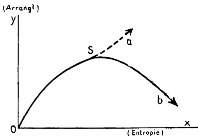
FIG. 2. — Courbe d'évolution de l'Énergie en fonction des deux courants cosmiques fondamentaux de complexité-conscience et d' entropie .
