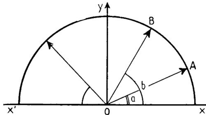
FIG. 3. — Expression symbolique de l'« onde de cérébration ».
