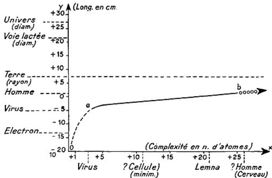
FIG. 1 « — Courbe suggérant une distribution naturelle des corpuscules (eu-corpuscules) organisés, en fonction de leurs dimensions linéaires et de leur complexité, celle-ci étant
