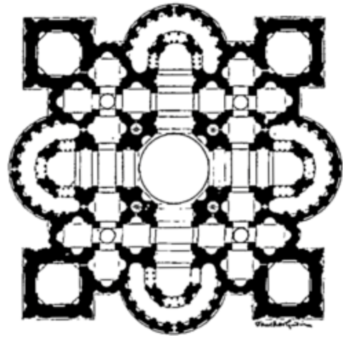
Fig. 10. — Saint-Pierre. (Plan de Peruzzi.)
