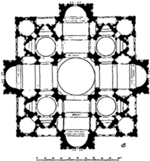
Fig. 6. — Saint-Pierre. (Plan de Bramante.)
