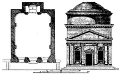
Fig. 17. — Église Saint-André, à Rome.
