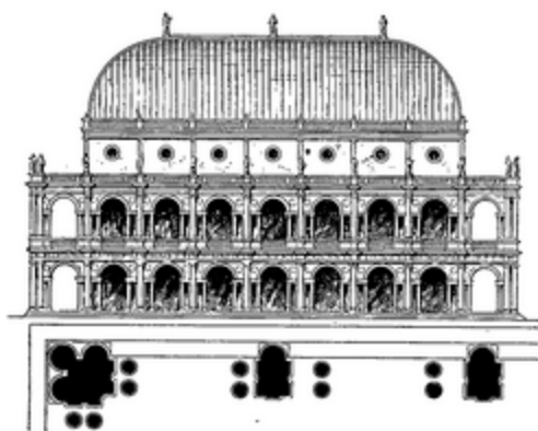
Fig. 19. — Basilique de Vicence.
