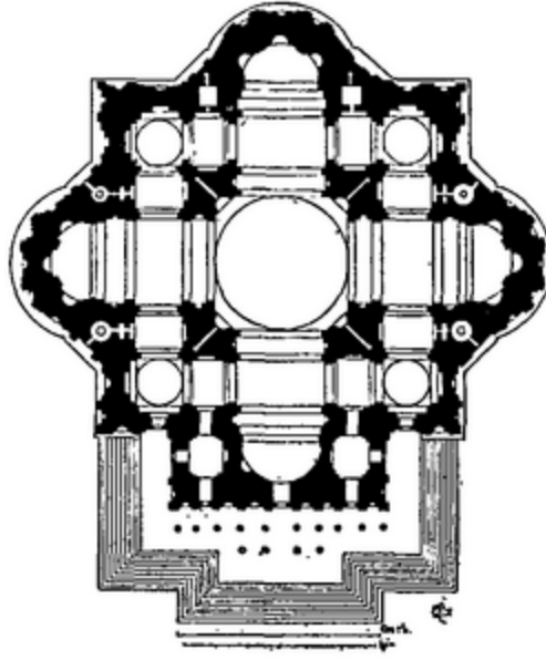
Fig. 13. — Saint-Pierre. (Plan de Michel-Ange.)
