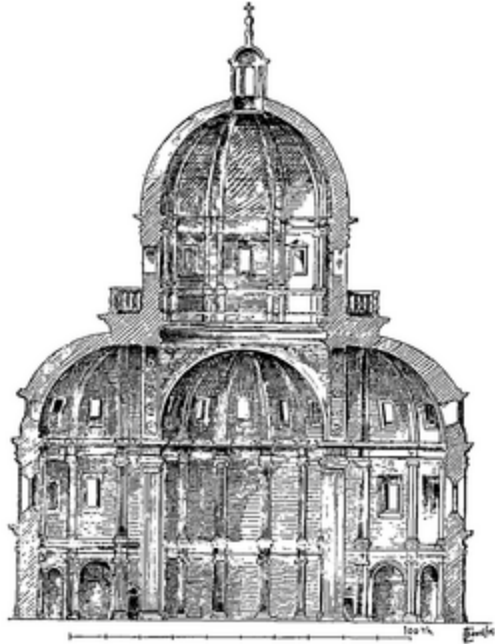
Fig. 2. — Consolazione de Todi (Burckhardt). (Coupe.)
