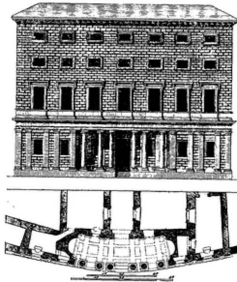
Fig. 11. — Palais Massimi, à Rome.
