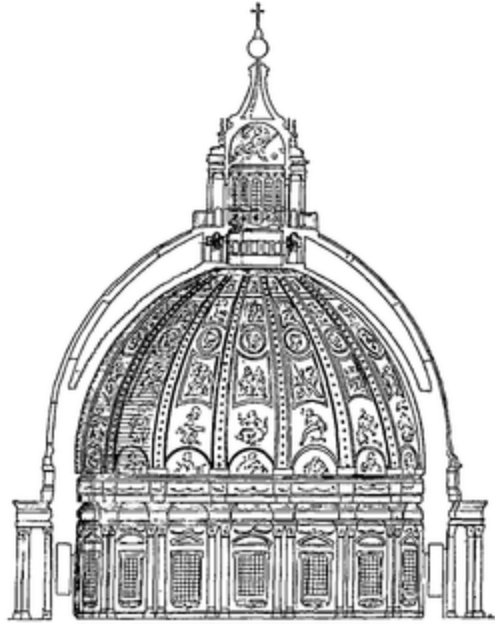
Fig. 25. — Coupole de Saint-Pierre.
