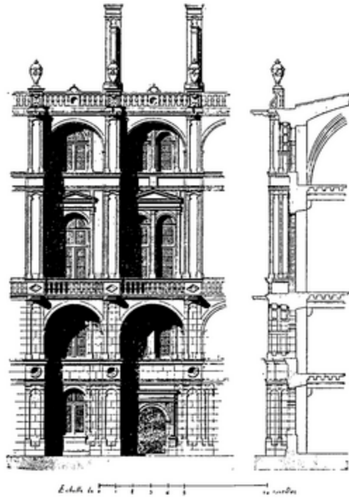
Fig. 55. — Détails de Saint-Germain-en-Laye (Sauvageot).
