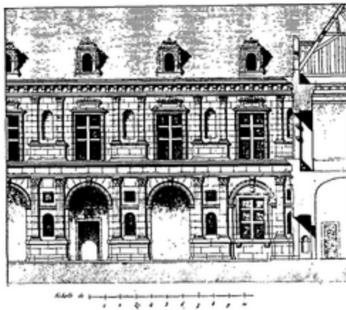
Fig. 61. — Ancy-le-Franc (S Sauvageot).
