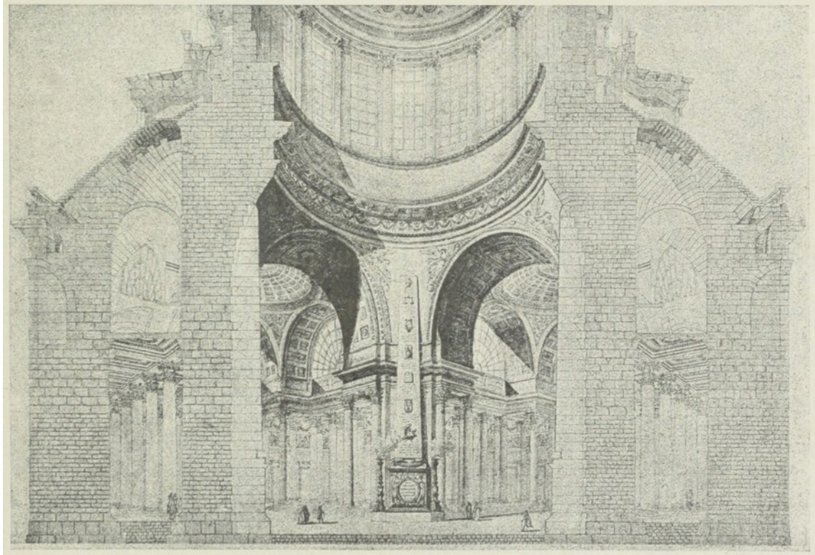
FIG. 4. – Vue intérieure du Panthéon. Étude pour la construction du dôme, par Brongniart.
