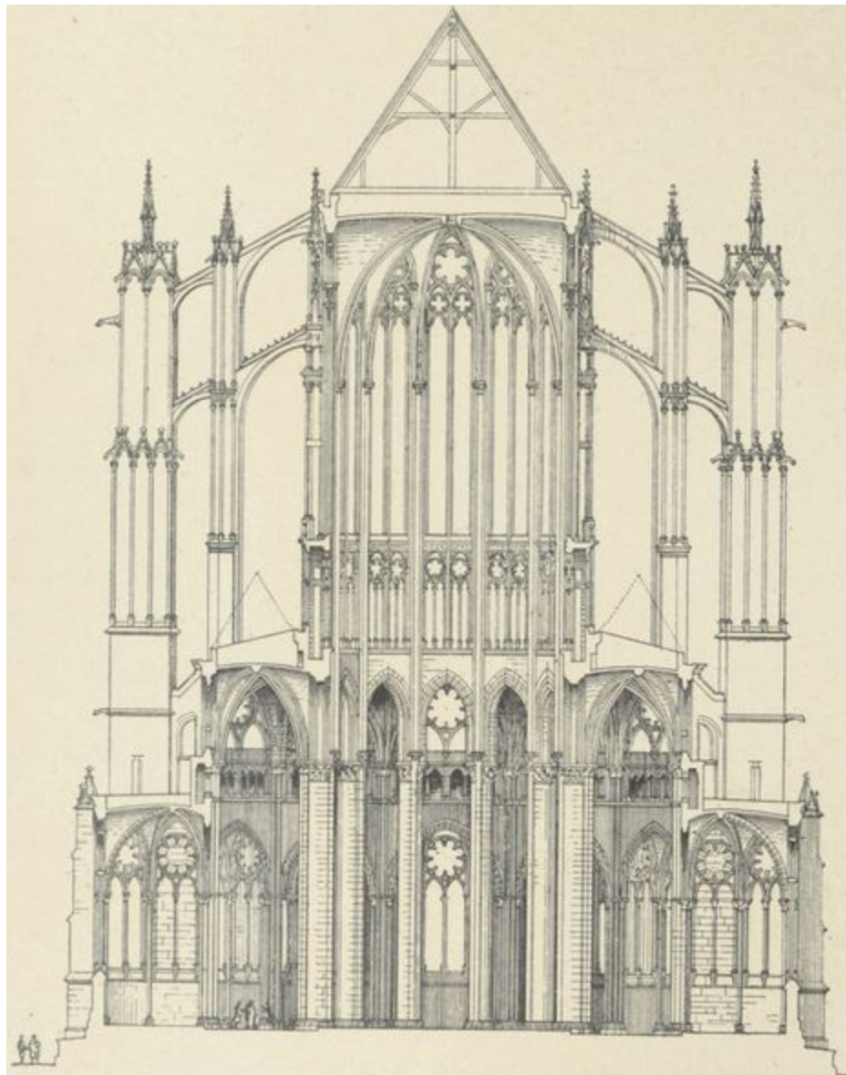
Fig. 42. — Cathédrale de Beauvais. (Coupe transversale).
