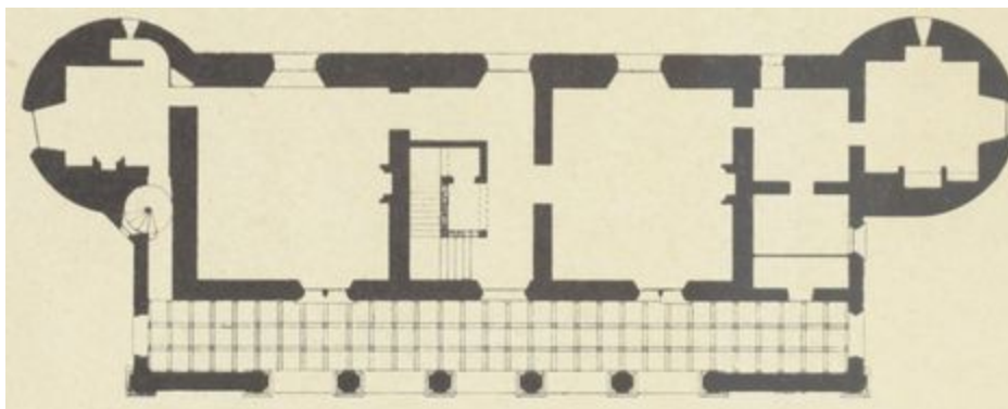
Fig. 62. — Château de Dampierre (Charente-Inférieure). (Plan du Rez-de-Chaussée).
