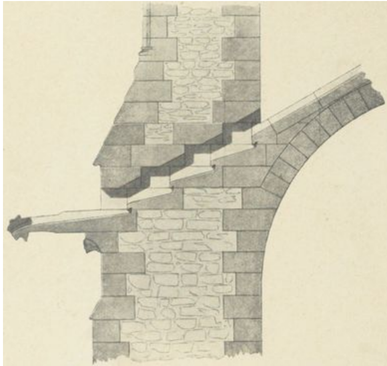
Fig. 44. — Coupe sur un contrefort au droit d'une gargouille.
