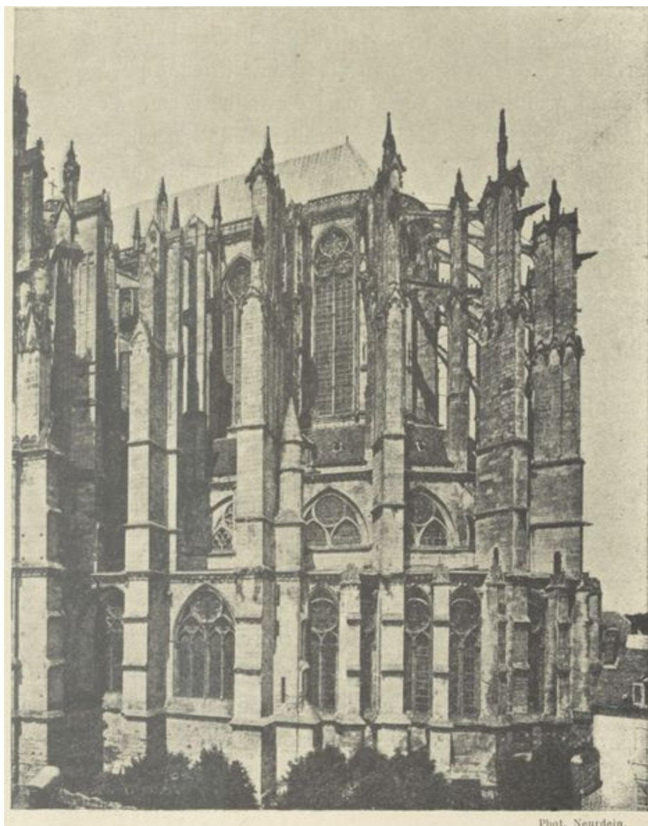
Fig. 43. — Cathédrale de Beauvais. (Extérieur).
