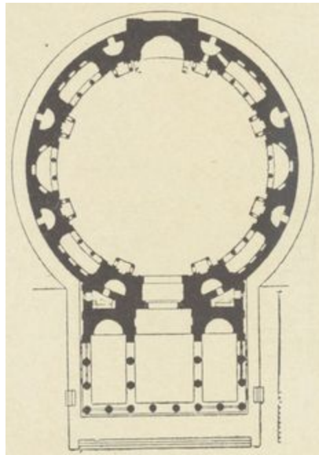
Fig. 10. — Plan du Panthéon de Rome.
