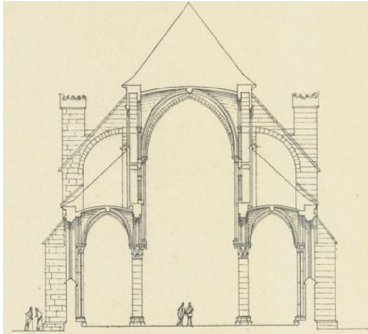
Fig. 38. — Notre-Dame de Dijon. (Coupe).
