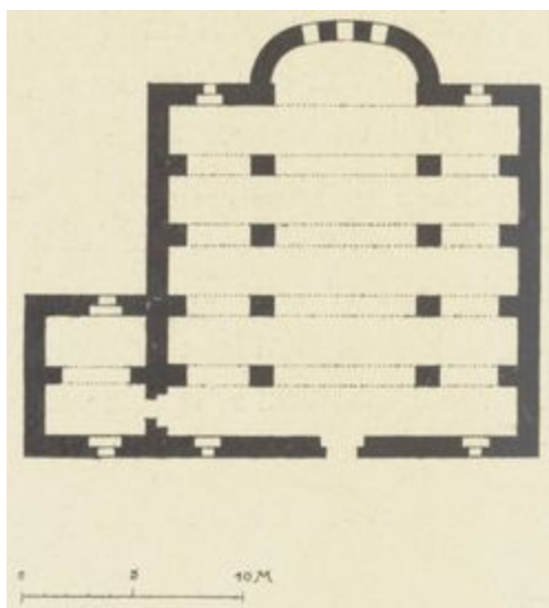
Fig. 19. — Plan de l'Eglise de Tarkha. (Syrie centrale).
