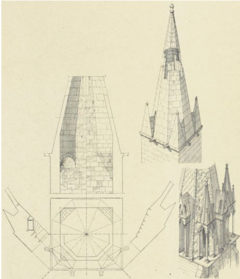
Fig. 30 et 31. — Clochers et flèches.
