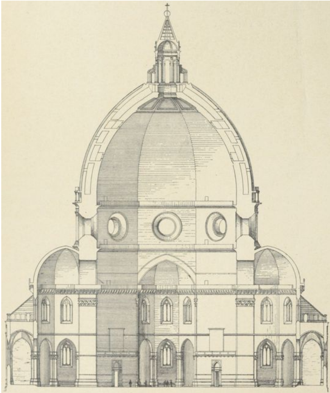
Fig. 54. — Dôme de Sainte-Marie des Fleurs. (Coupe).
