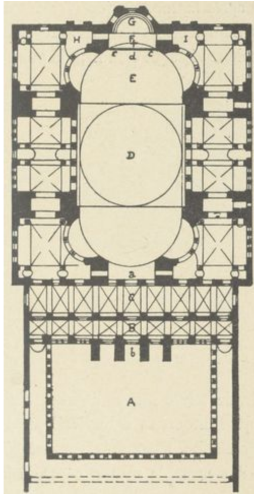
Fig. 15. — Plan de Sainte-Sophie de Constantinople.
