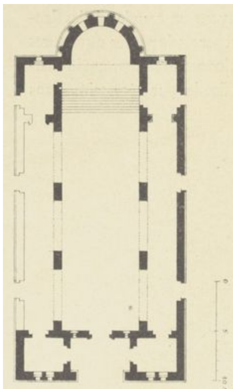
Fig. 21. — Plan de l'Église de Qalb-Louzeh (Syrie centrale).
