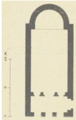
Fig. 23. — Plan de l'Église de Babouda. (Syrie centrale).
