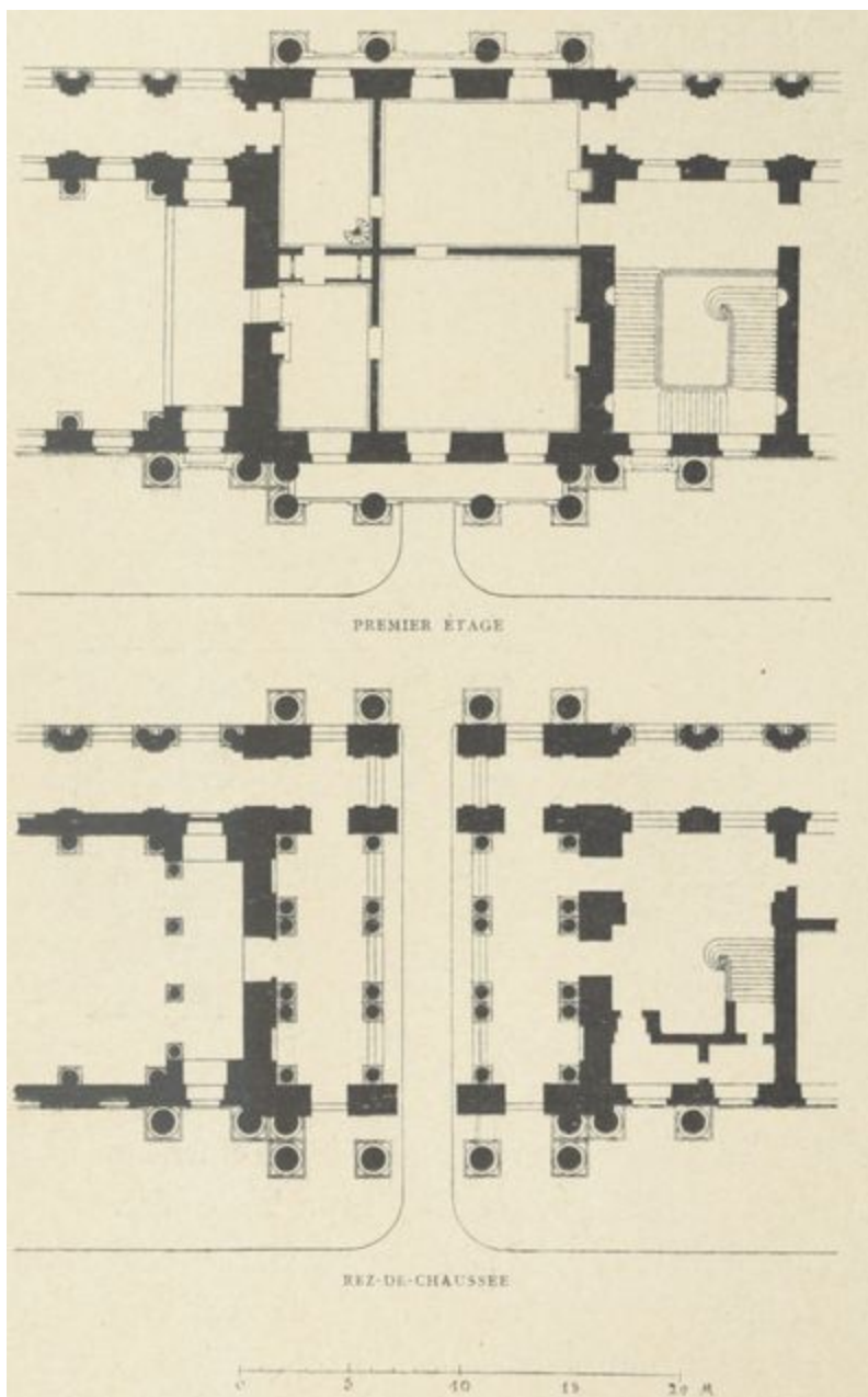
Fig. 75 — Ecole militaire. Plans de la partie centrale,.
