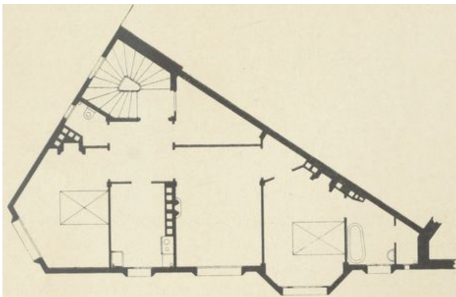
Fig. 88. — Maison rue Belliard. (M. Deneux architecte. Plan).
