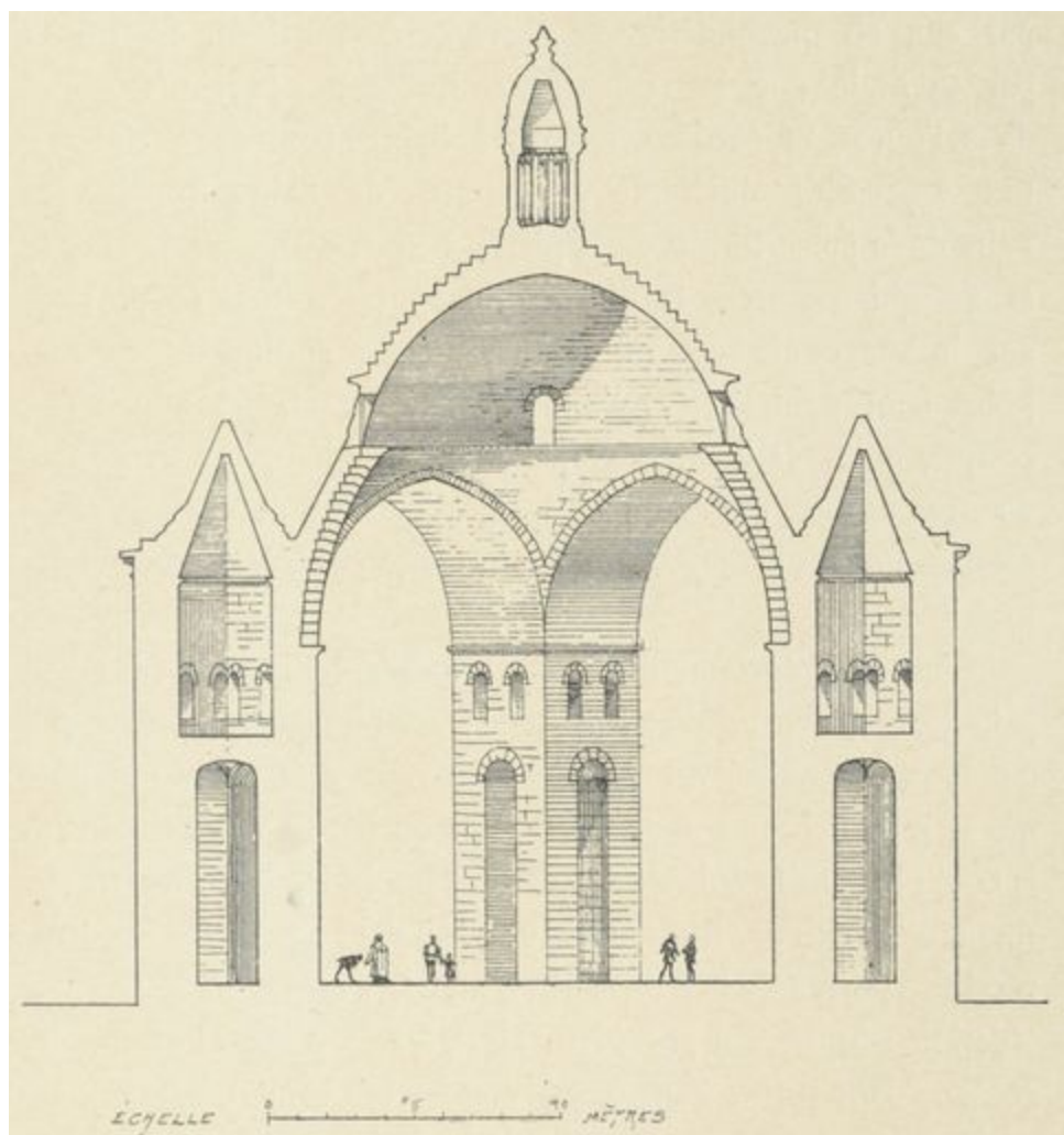
Fig. 26. — Coupe de Saint-Front de Périgueux.
