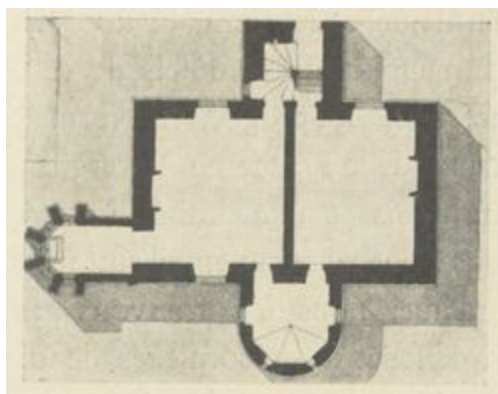
Fig. 50. — Plan du Château du Moulin (Loir-et-Cher).
