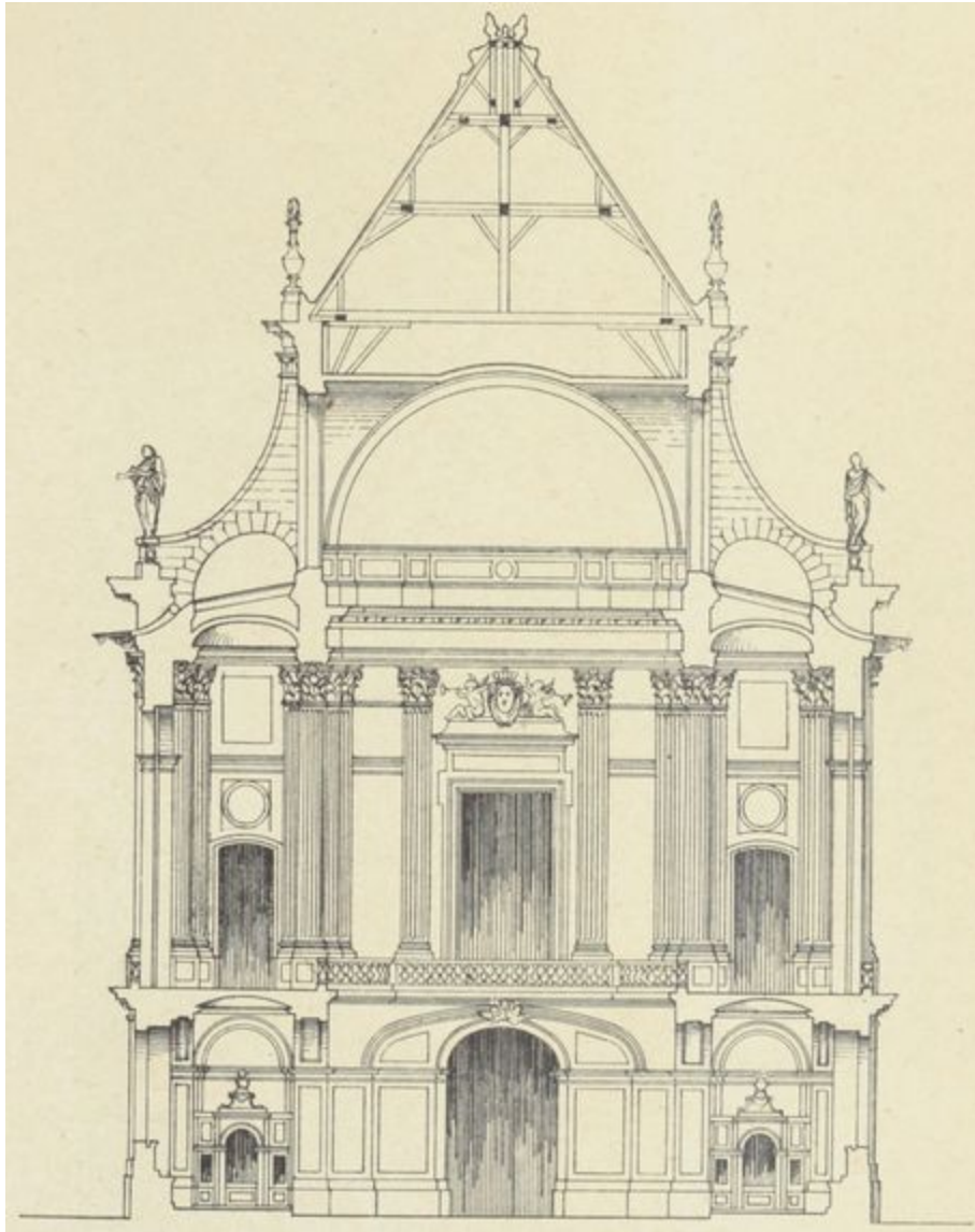
Fig. 73. — Chapelle du château de Versailles. (Coupe transversale).
