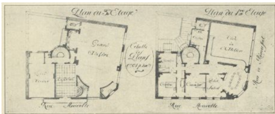
Fig. 87. — Maison à Auteuil. (Plan).
