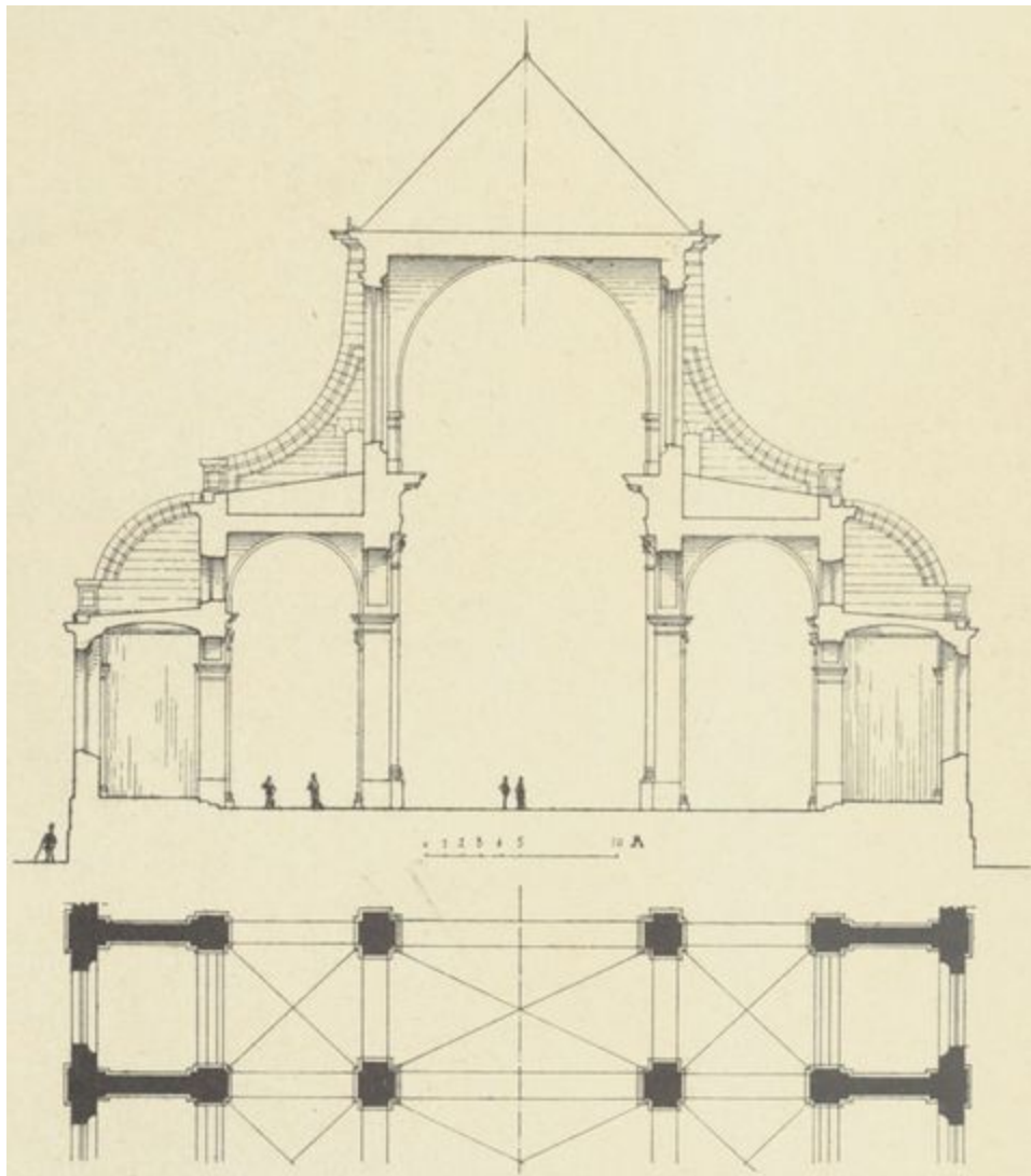
Fig. 74. — Eglise Saint-Sulpice à Paris. (Plan et coupe transversale).
