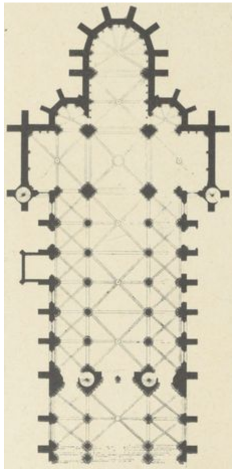
Fig. 37. — Eglise Notre-Dame de Dijon. Plan.
