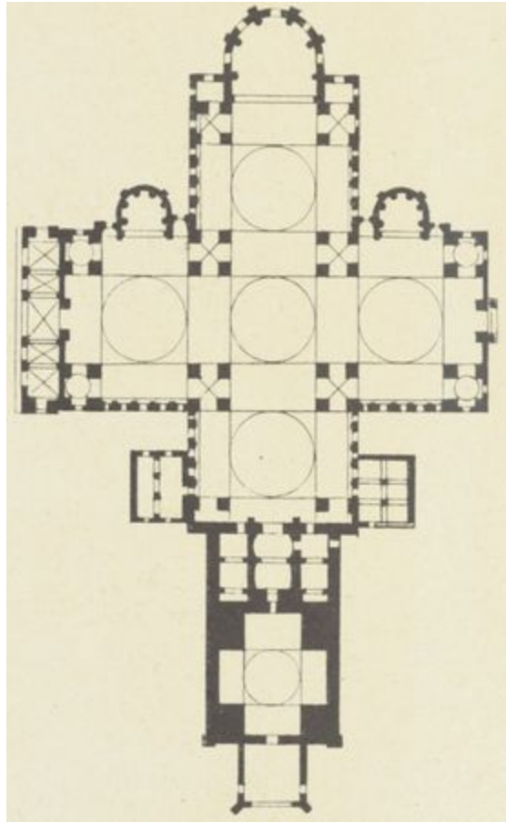
Fig. 25. — Plan de Saint-Front de Périgueux.
