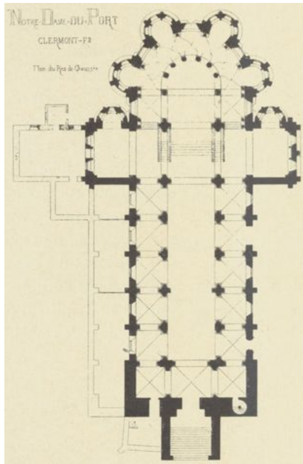
Fig. 27. — Plan de Notre-Dame-du-Port à Clermont-Ferrand.
