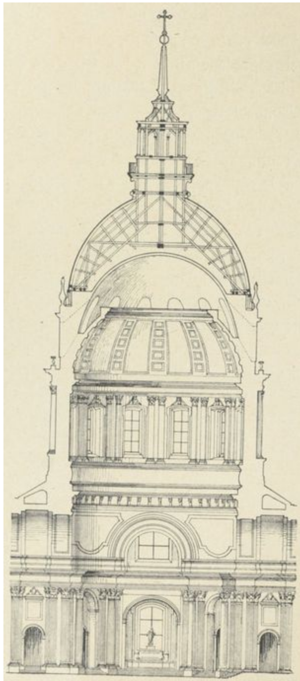
Fig. 69. — Dôme des Invalides. (Coupe).
