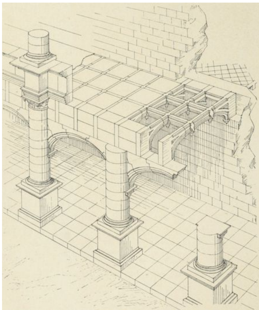
Fig. 64. — Château de Dampierre. (Structure de la galerie).
