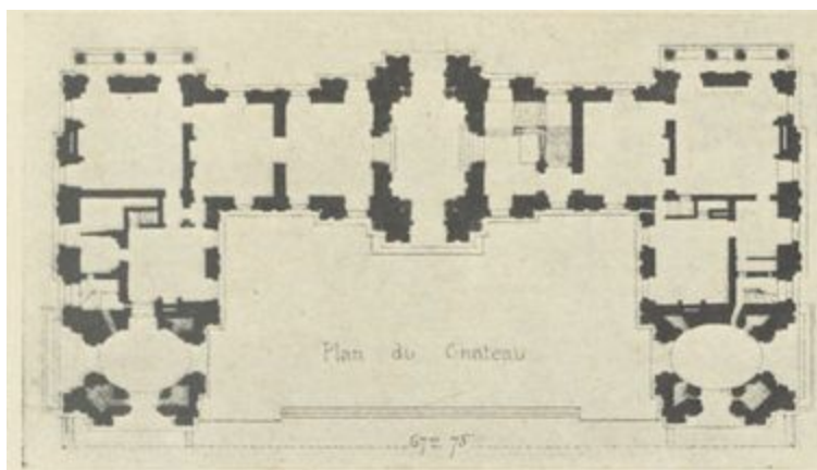
Fig. 67. — Château de Maisons-sur-Seine. (Plan).
