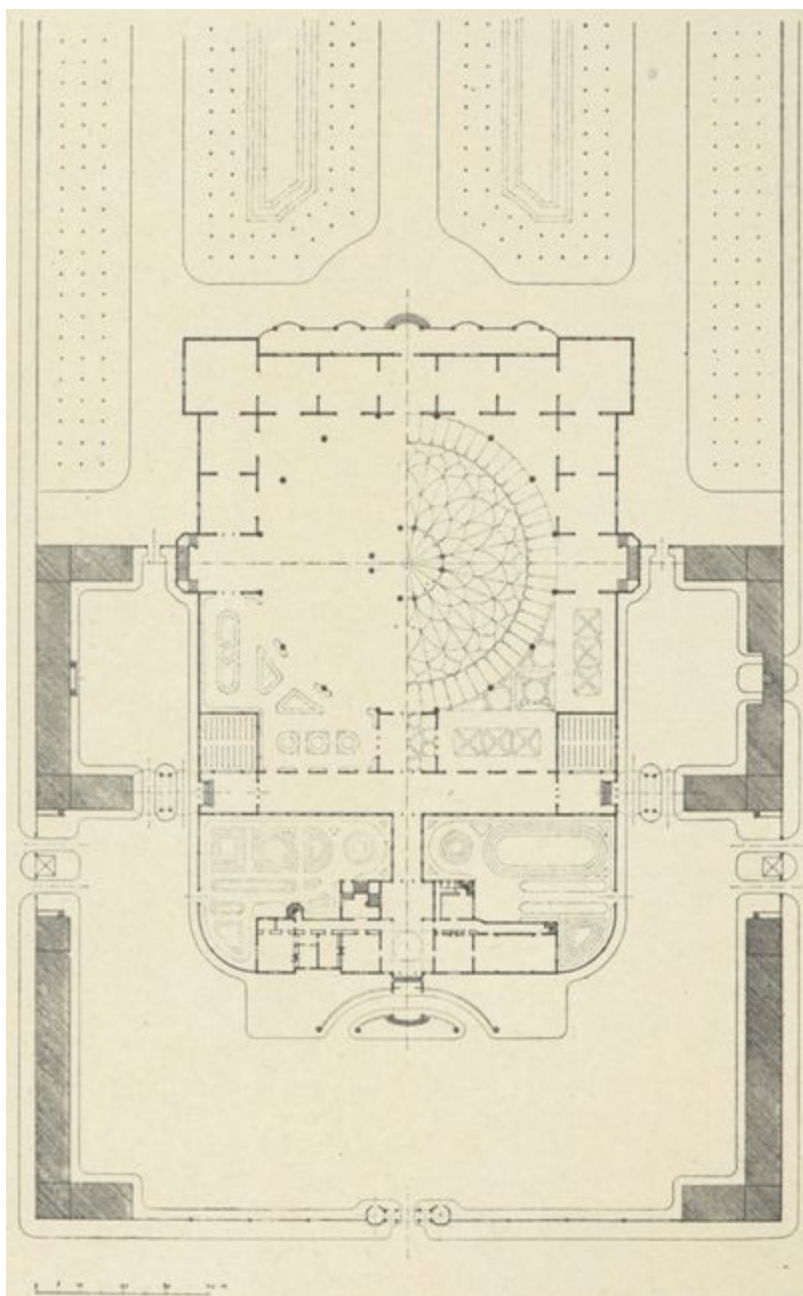
Fig. 96. — Projet-esquisse de Présidence de la République. (Plan).
