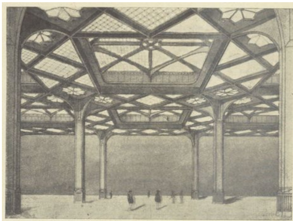
Fig. 93. — Intérieur indiquant la solution par croisements.
