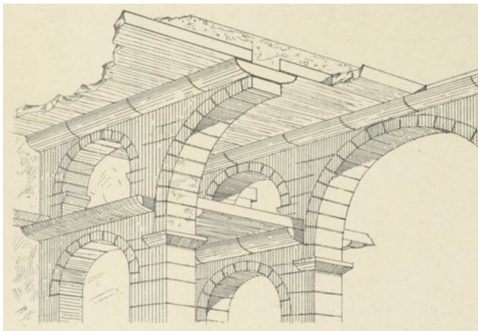
Fig. 20. — Eglise de Tafkha. (Perspective intérieure).
