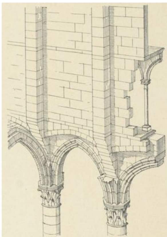
Fig. 39. — Notre-Dame de Dijon.
