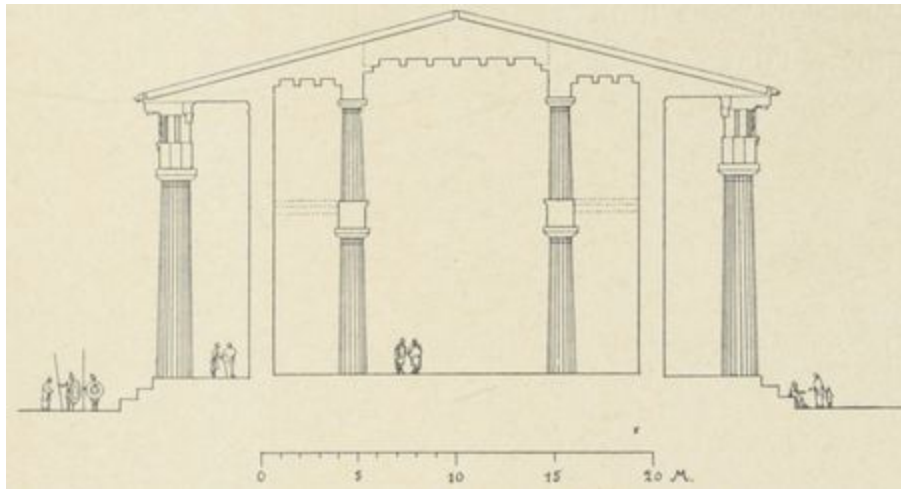
Fig. 6. — Coupe sur le Parthénon.
