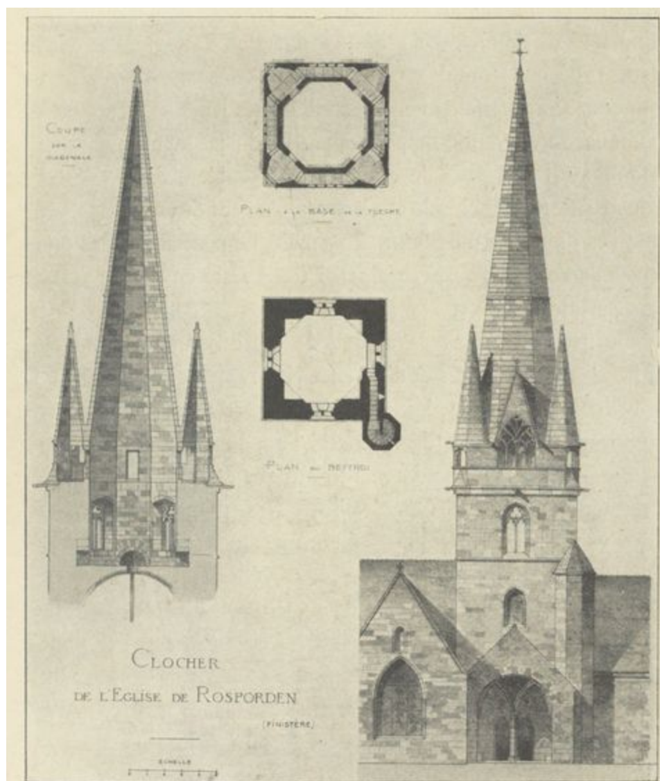
Fig. 46. — Eglise de Rosporden, Finistère. (Clocher).
