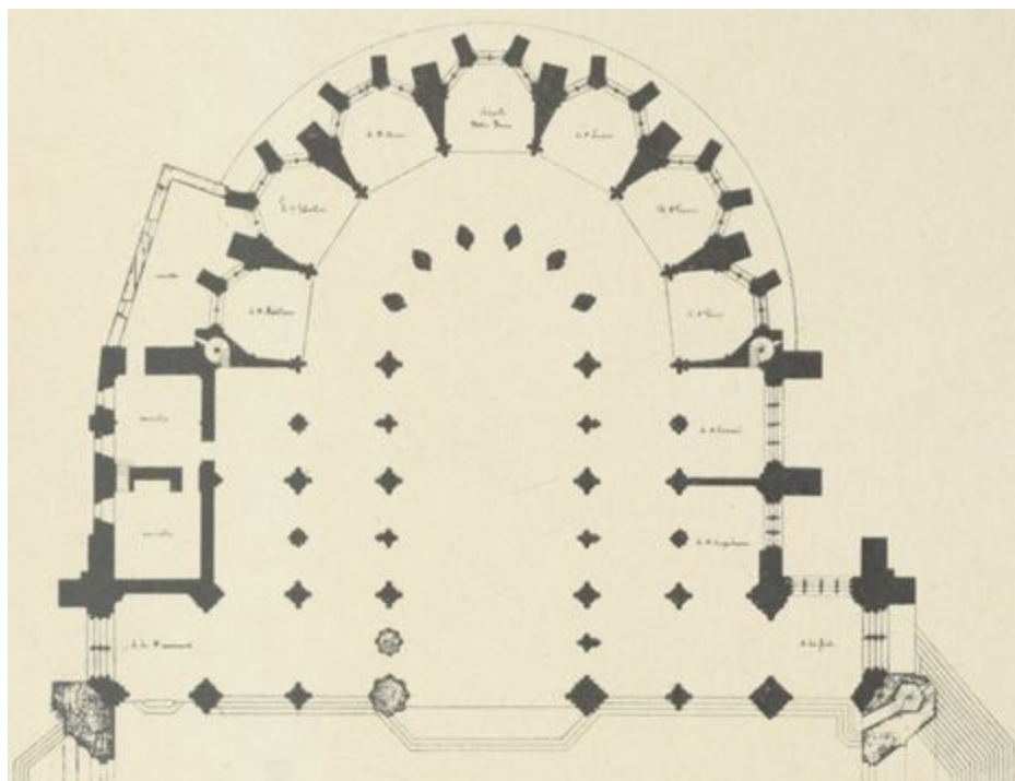
Fig. 41. — Cathédrale de Beauvais. (Plan du chœur).
