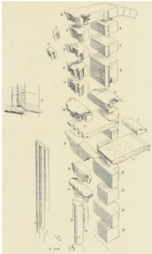
Fig. 40. — Notre-Dame de Dijon.
