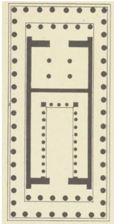
Fig. 5. — Plan du Parthénon.
