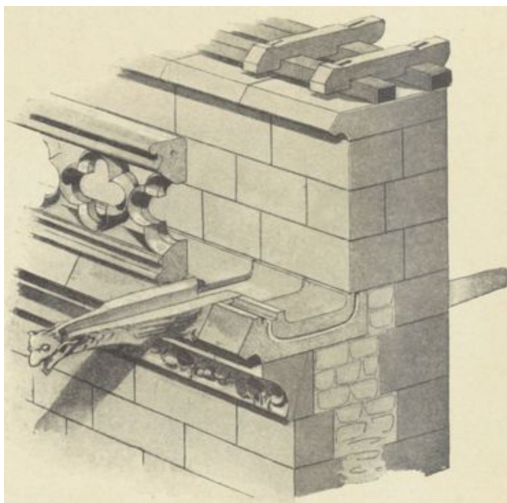
Fig. 45. — Gargouille vue de l'extérieur.
