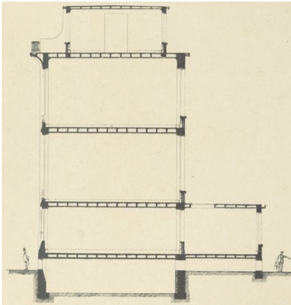
Fig. 84. — Bureau téléphonique. (Coupe).
