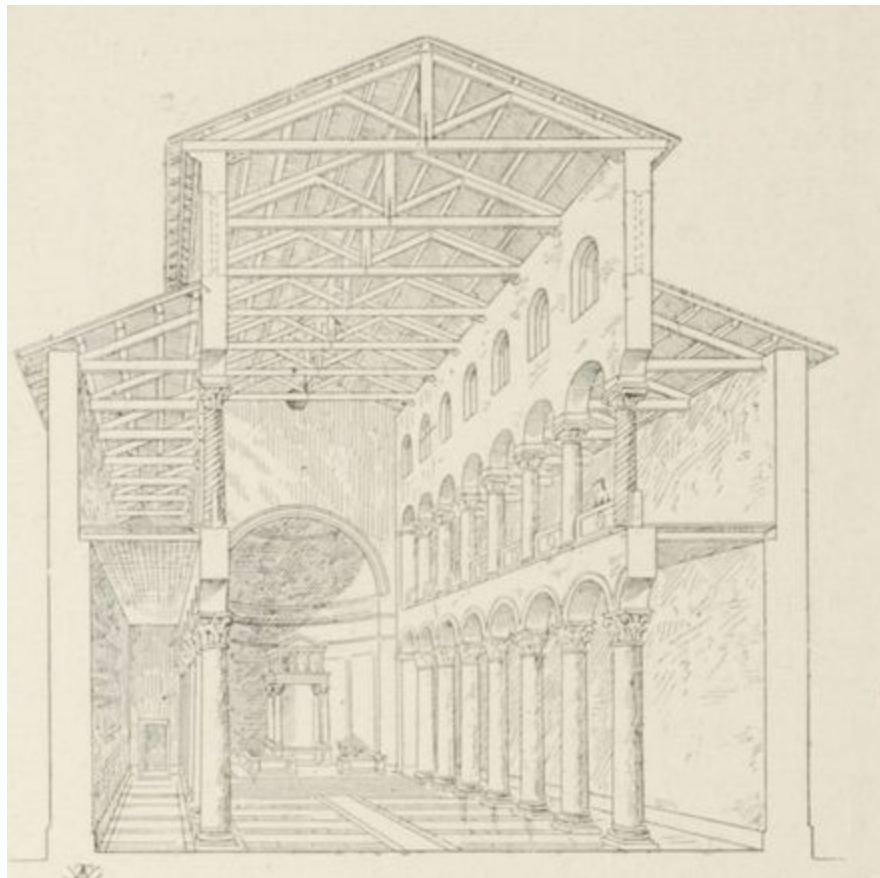
FIG. 57. — BASILIQUE DE SAINTE-AGNÈS-HORS-LES-MURS. (Vue perspective intérieure.)
