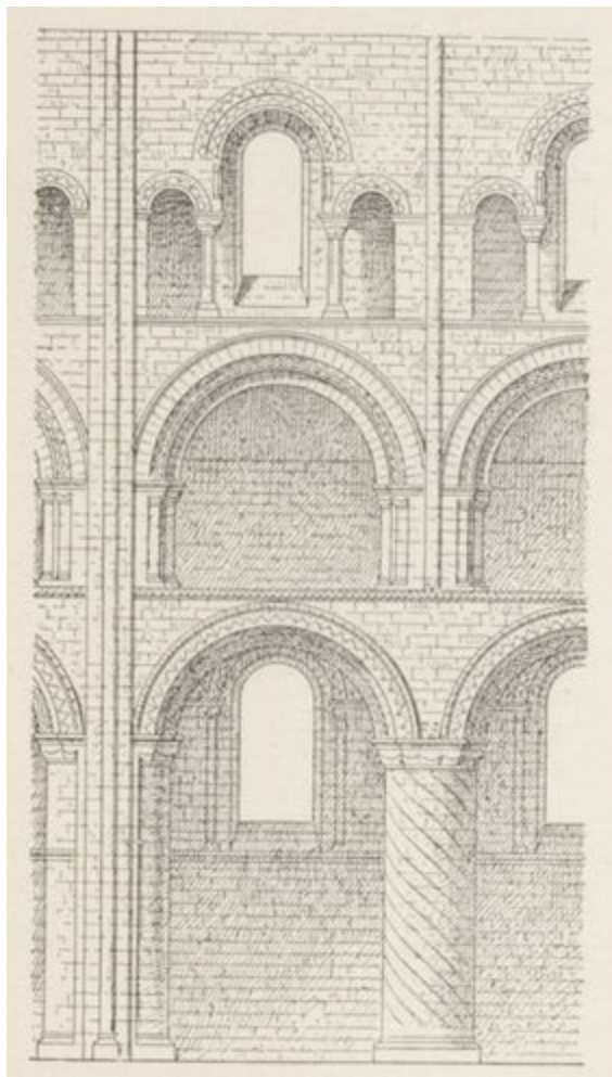
FIG. 114 . — ÉGLISE DE WALTHAM-ABBEY (ANGLETERRE). (Coupe longitudinale, fragment.)
