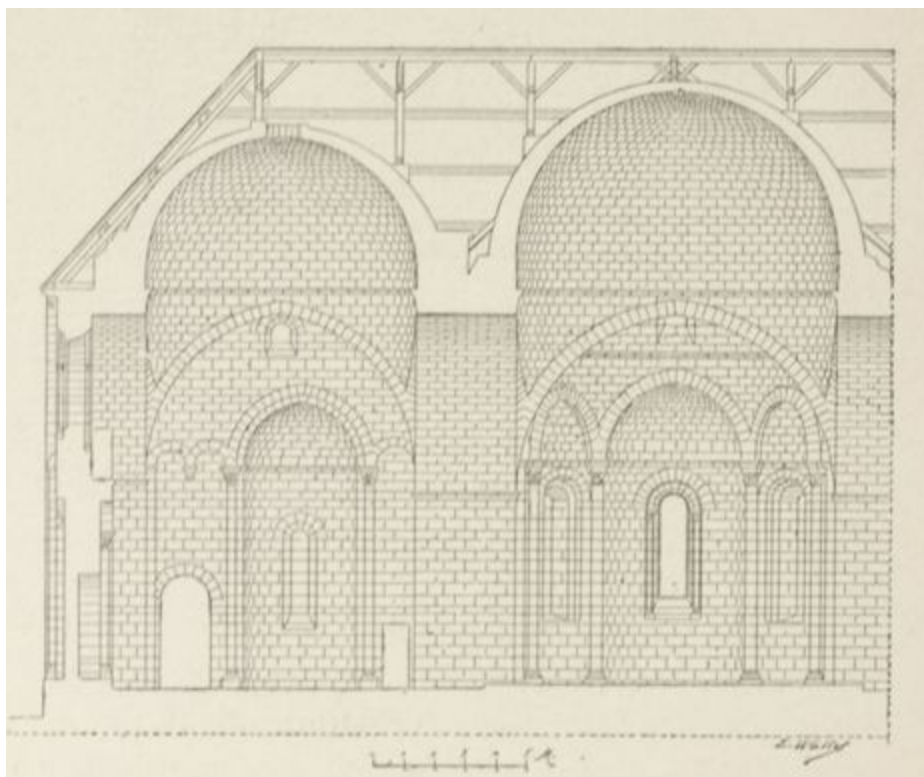
FIG. 174. — ÉGLISE DE SOLIGNAC. (Coupe sur le transept, fragment.)
