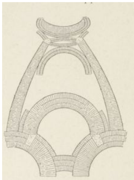
FIG. 13. — COUPOLE DU PANTHÉON DE ROME (Détails de construction de la voûte.)
