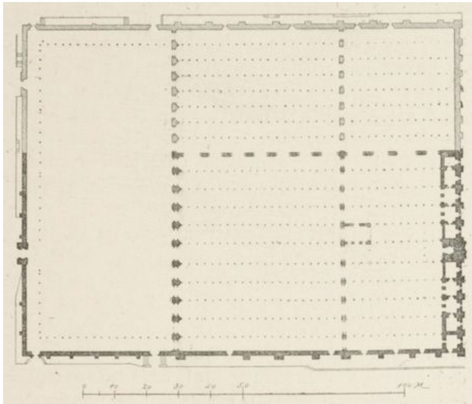
FIG. 61. — MOSQUÉE DE CORDOUE (ESPAGNE). (Plan.)
