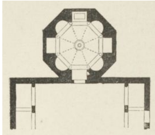
FIG. 27. BAPTISTÈRE DE NOVARE. (Plan.)
