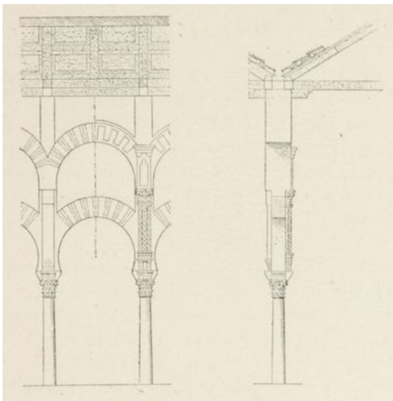
FIG. 62. — MOSQUÉE DE CORDOUE (ESPAGNE). (Coupes longitudinale et transversale des nefs.)
