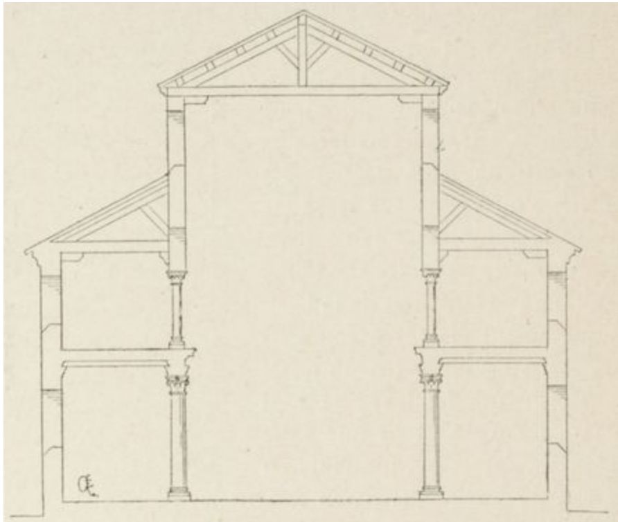
FIG. 3. — BASILIQUE CIVILE. (Coupe transversale.)
