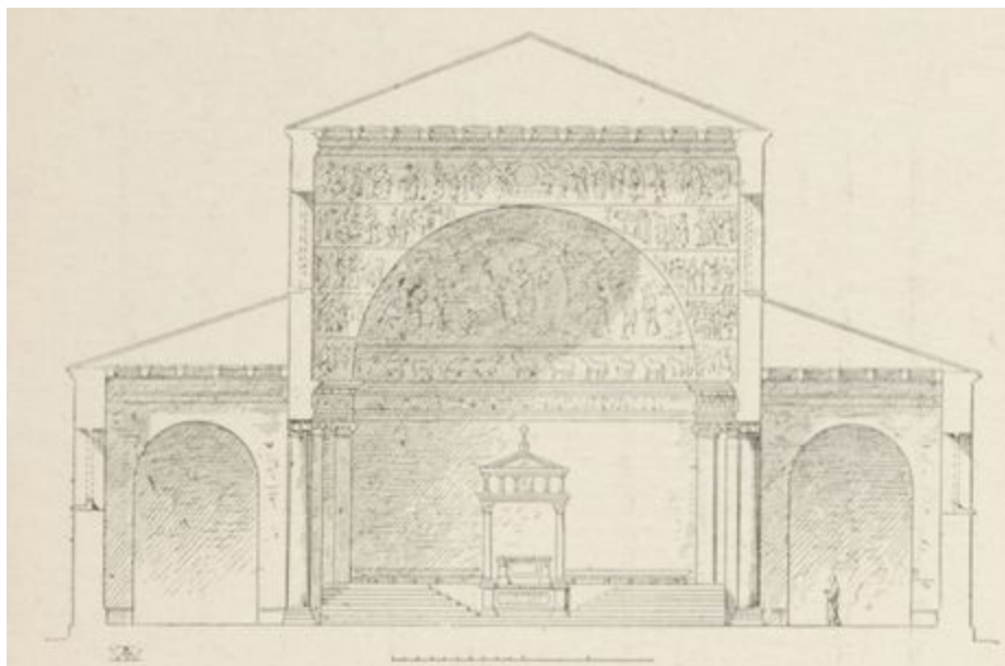
FIG. 21. — BASILIQUE DE SAINTE-MARIE-MAJEURE, A ROME. (Coupe transversale.)
