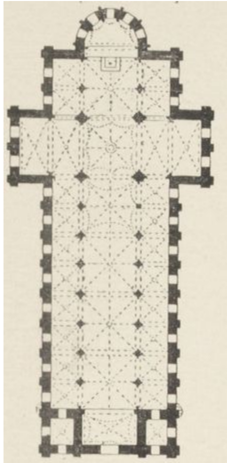
FIG. 189. — ÉGLISE DE LA TRINITÉ, A CAEN (FRANCE). (Plan.)
