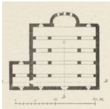
FIG. 28. BASILIQUE DE TAFKHA (SYRIE CENTRALE). (Plan.)
