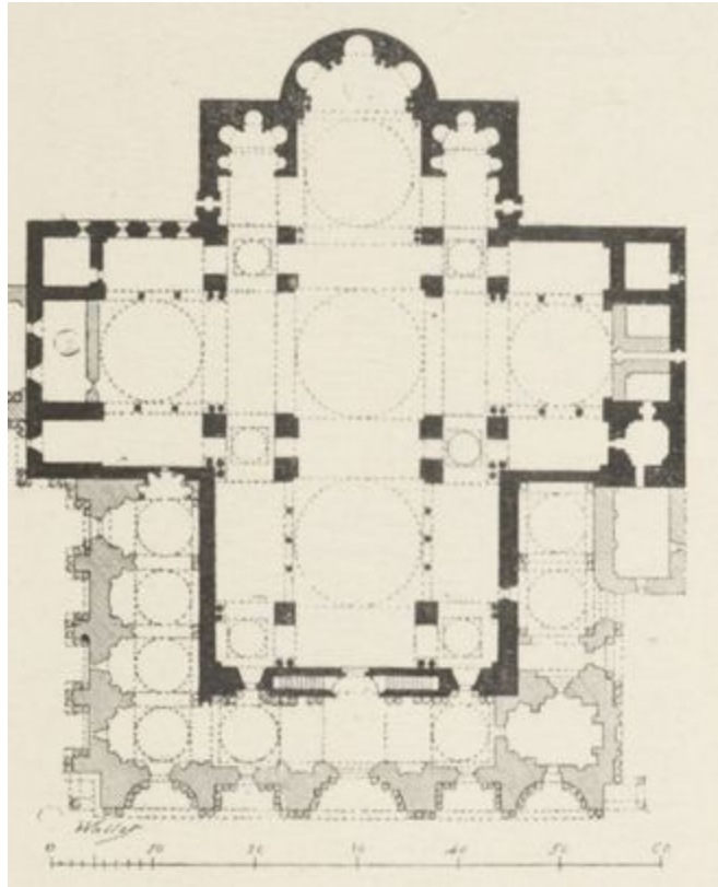
FIG 153. — ÉGLISE DE SAINT-MARC, A VENISE (Plan.)
