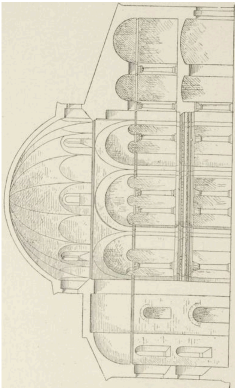
FIG. 63 — ÉGLISE DES SS. SERGE ET BACCHUS, A CONSTANTINOPLE. (Coupe longitudinale, de l'abside au narthex.)
