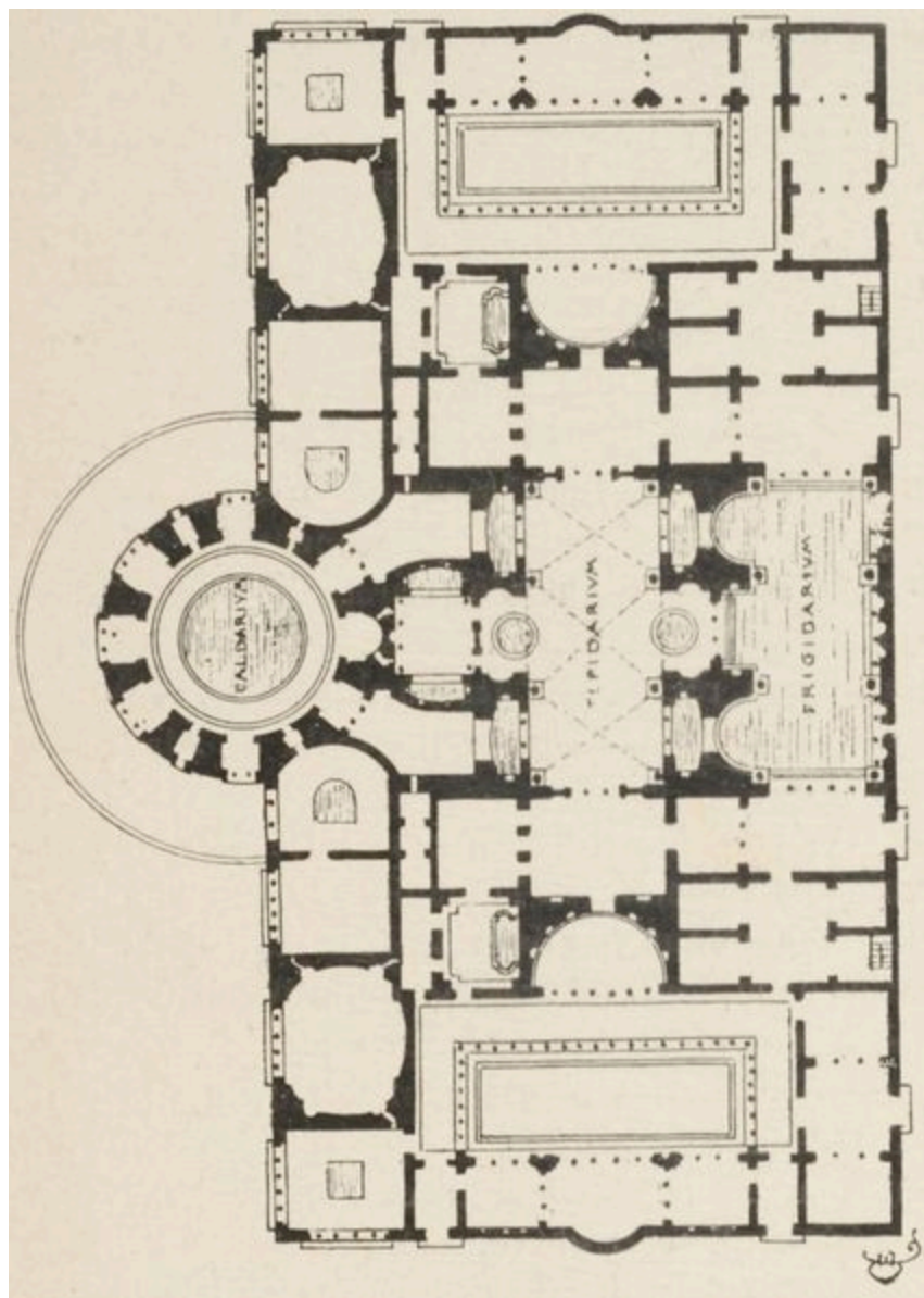
FIG. 8. — THERMES D'ANTONIN CARACALLA. A ROME. (Plan.)
