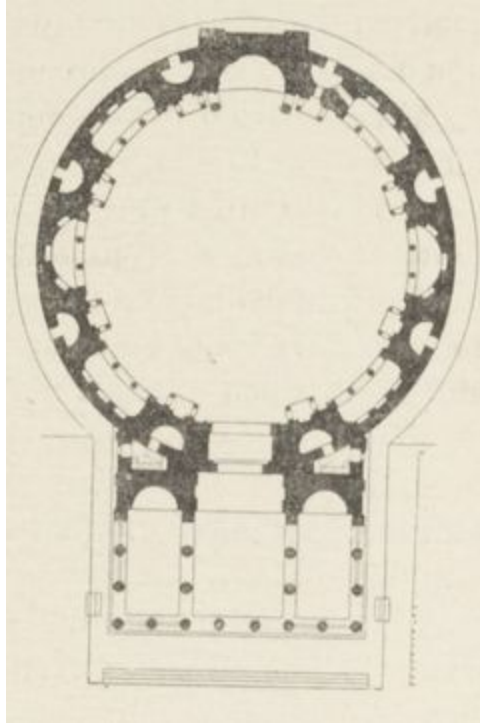
FIG. II. LE PANTHÉON DE ROME. (Plan.)
