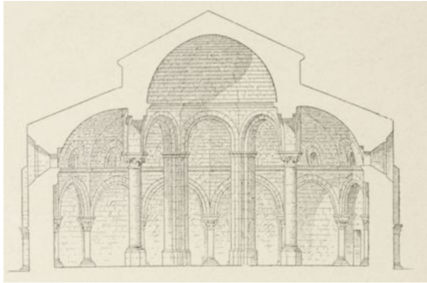
FIG. 125. — ÉGLISE DE RIEUX-MÉRINVILLE (FRANCE). (Coupe.)
