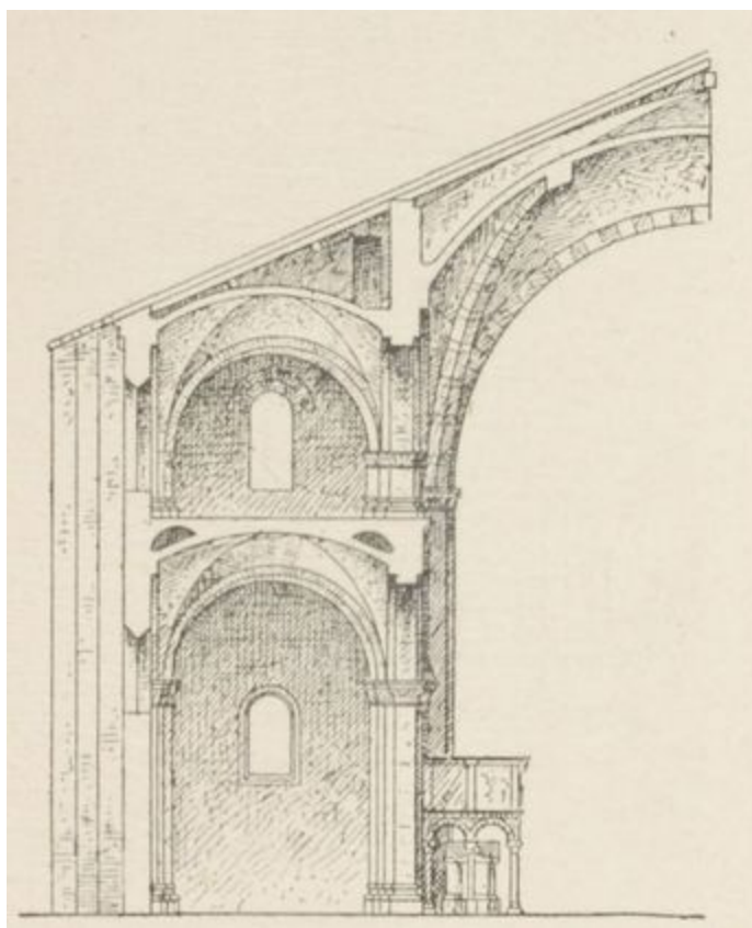
FIG. 187. ÉGLISE DE SAINT-AMBROISE, A MILAN (ITALIE). (Coupe transversale.)
