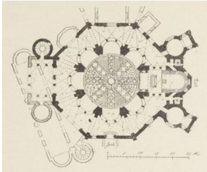
FIG. 65. — ÉGLISE DE SAINT-VITAL, A RAVENNE. (Plan.)
