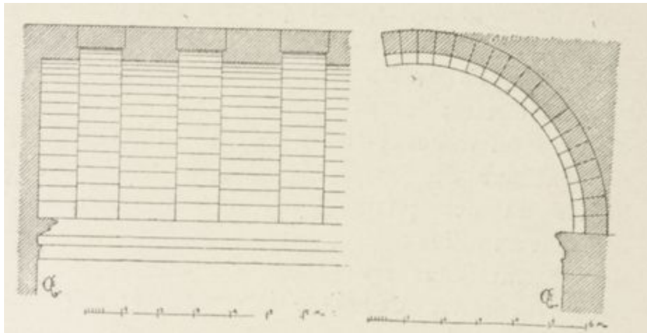
FIG 129 ET 130. — NYMPHÉE DE NIMES. (Coupes de la voûte en berceau.)
