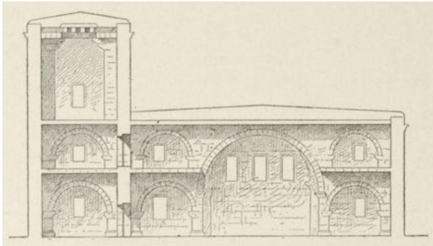
FIG. 29. — BASILIQUE DE TAFKHA (SYRIE CENTRALE). (Coupe transversale sur A-B du plan.)
