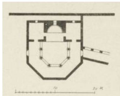
FIG. 31. — BAPTISTÈRE DE MOUDJELEIA (SYRIE CENTRALE). (Plan.)
