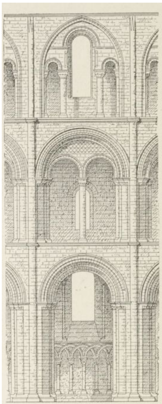
FIG. 117. — ÉGLISE DE PETERBOROUGH (ANGLETERRE). (Coupe longitudinale, fragment.)
