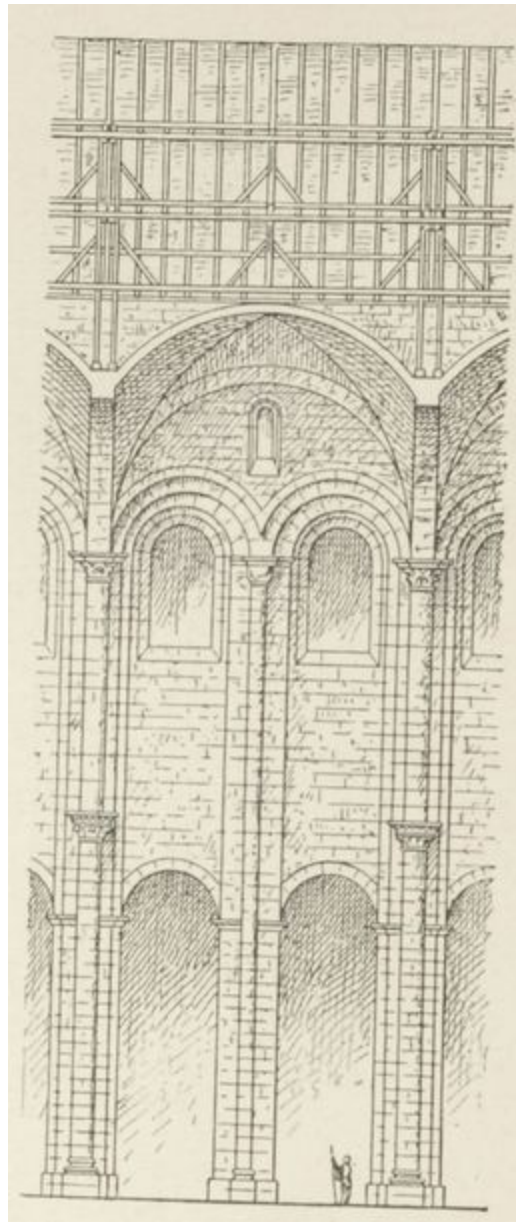
FIG. 185. ÉGLISE DE SPIRE (ALLEMAGNE). (Coupe longitudinale.)
