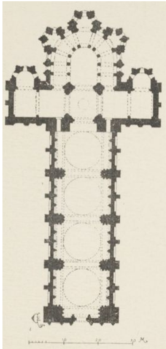
FIG. 175. ÉGLISE DE FONTEVRAULT. (Plan.)
