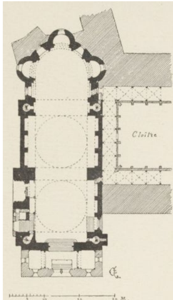
FIG. 161. — ÉGLISE DE CAHORS. (Plan.)
