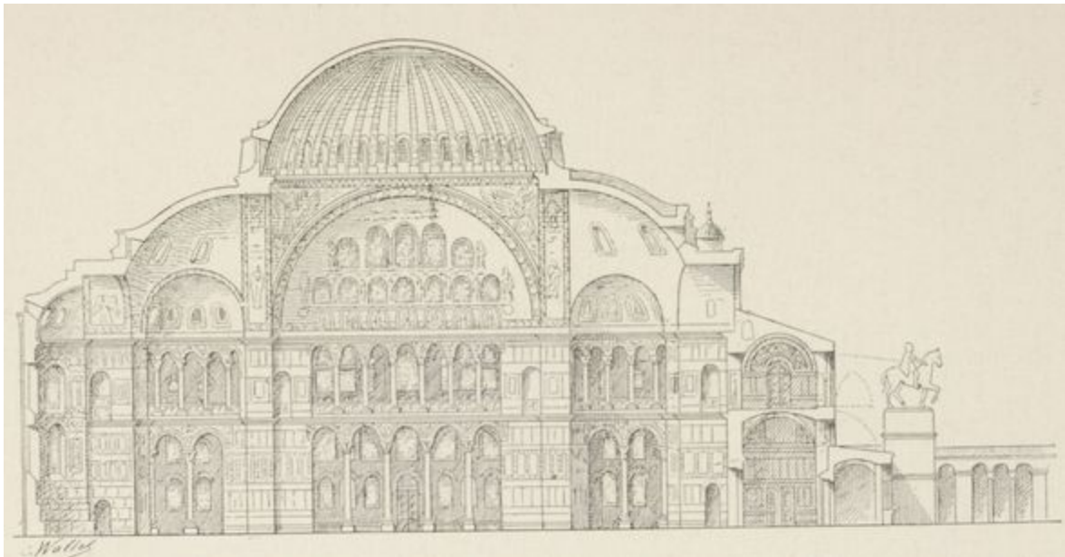
FIG 69. — ÉGLISE DE SAINTE-SOPHIE, A CONSTANTINOPLE. (Coupe longitudinale, de l'abside à l'atrium.)
