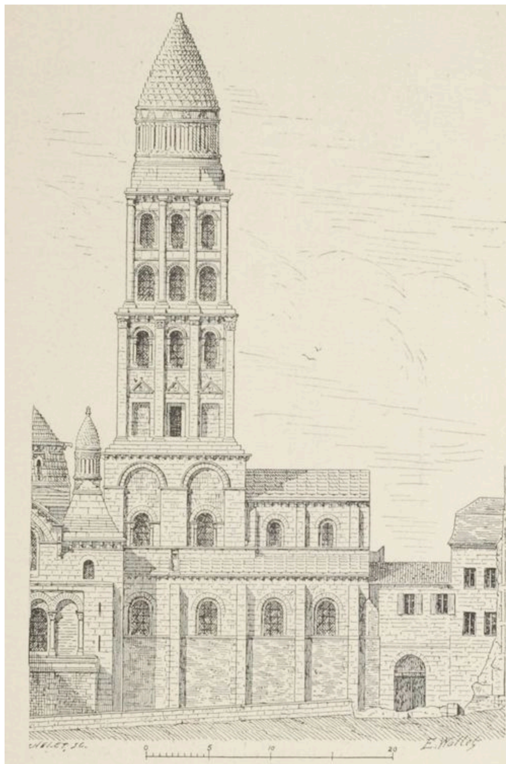
FIG. 54. — ÉGLISE LATINE ET CLOCHER DE SAINT-FRONT. (Façade nord montrant 2 travées de la nef latine.)
