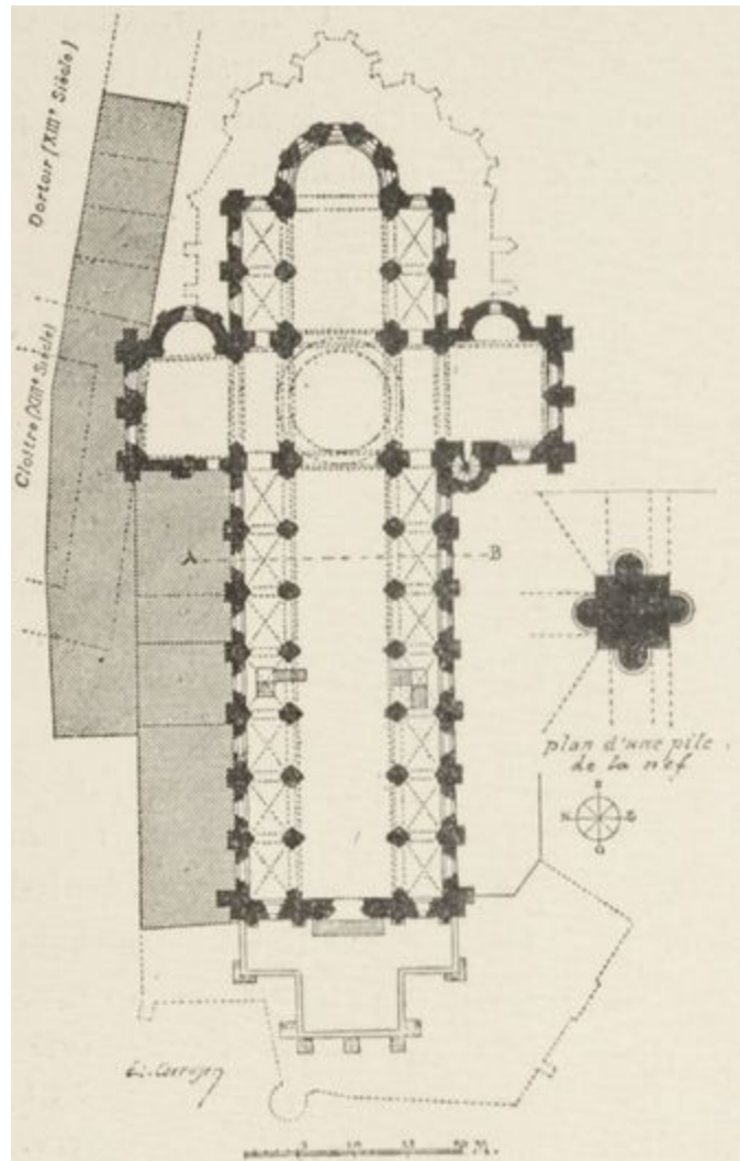
FIG. 9, 109. — ÉGLISE ABBATIALE DU MONT SAINT-MICHEL (FRANCE). (Plan.)
