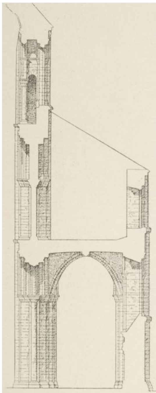
FIG. 116. — ÉGLISE DE PETERBOROUGH (ANGLETERRE). (Coupe transversale.)
