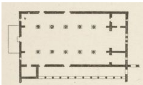
FIG. 34. — ÉGLISE DE BEHIO (SYRIE CENTRALE). (Plan.)
