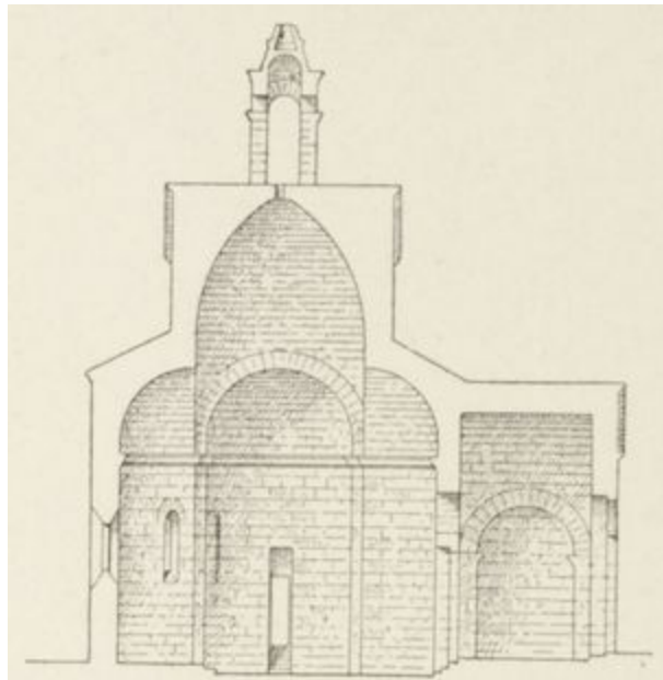
FIG. 99. CHAPELLE SAINTE-CROIX DE MONTMAJOUR (PRÈS D'ARLES). (Coupe longitudinale.)
