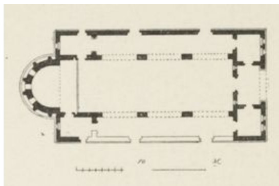
FIG.43. ÉGLISE DE QALB-LOUZEH (SYRIE CENTRALE). (Plan.)
