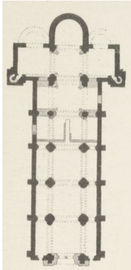
FIG. 144. ÉGLISE DE SAINT-TROPHIME A ARLES. (Plan.)
