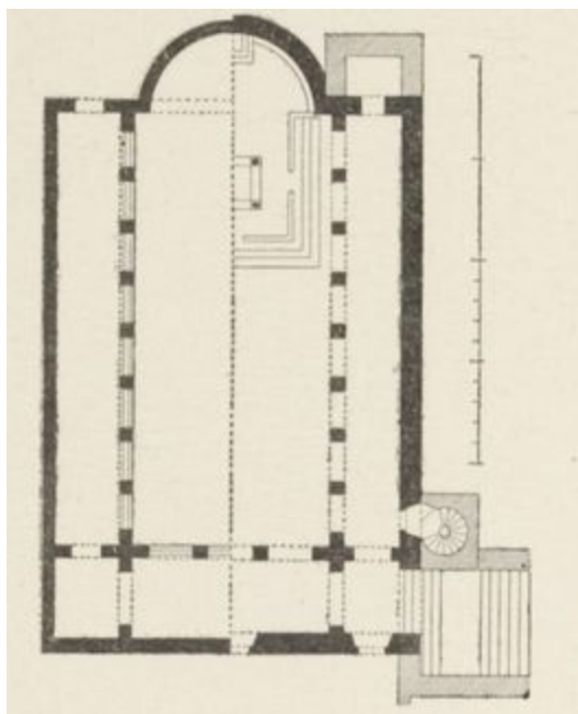
FIG. 56. — BASILIQUE DE SAINTE-AGNÈS-HORS-LES-MURS, A ROME. (Plan.)
