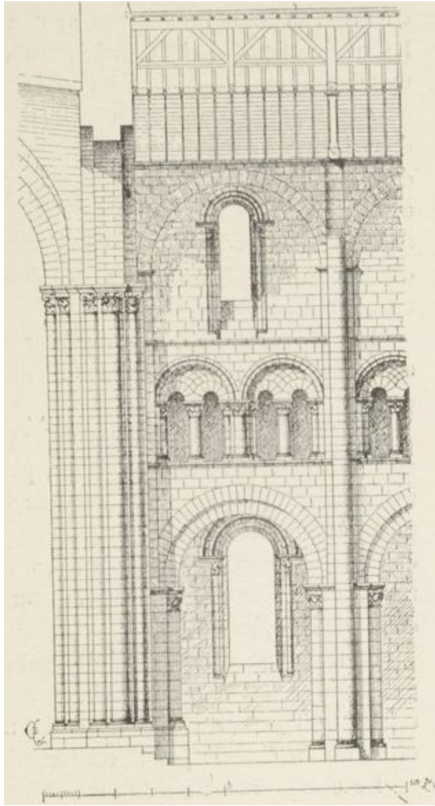
FIG. 111. ÉGLISE ABBATIALE DU MONT SAINT-MICHEL (FRANCE). (Coupe longitudinale, fragment.)
