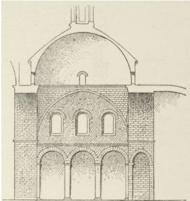
FIG. 162. — ÉGLISE DE CAHORS. (Coupe longitudinale, fragment.)
