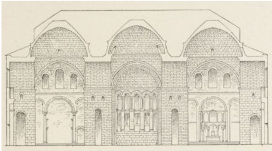
FIG. 158. — ÉGLISE DE SAINT-FRONT, A PÉRIGUEUX. (Coupe transversale du nord au sud.)
