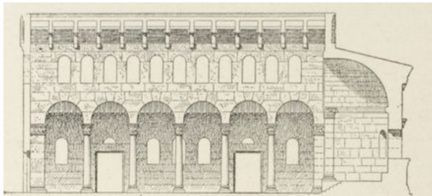
FIG. 41. — ÉGLISE DE BAQOUZA (SYRIE CENTRALE). (Coupe longitudinale.)
