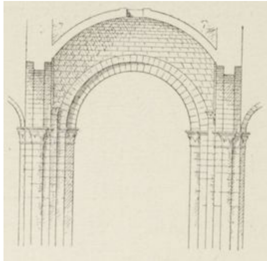
FIG. 176. — ÉGLISE DE FONTEVRAULT. (Coupe de la voûte de la croisée du transsept.)
