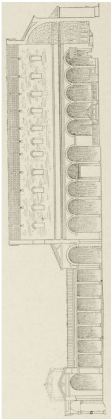
FIG. 59. — BASILIQUE DE SAINT-CLÉMENT, A ROME. (Coupe longitudinale.)
