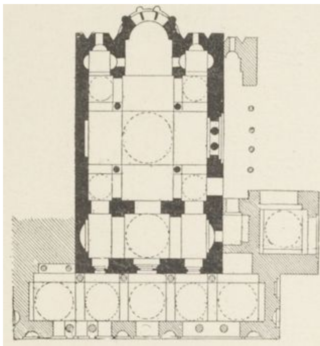
FIG. 72. — ÉGLISE DE THÉOTOCOS, A CONSTANTINOPLE. (Plan.)
