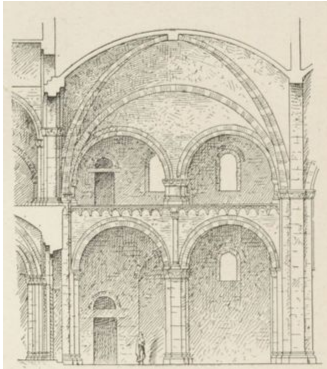
FIG. 188. ÉGLISE DE SAINT-AMBROISE, A MILAN (ITALIE). (Coupe longitudinale.)
