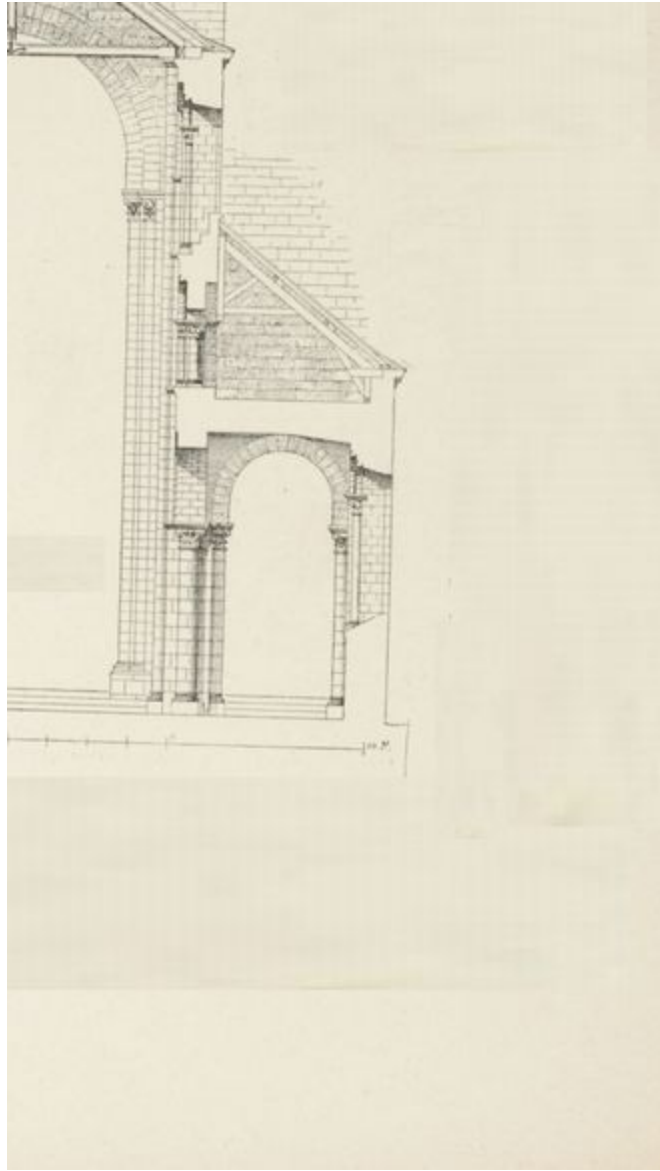
FIG. 110. ÉGLISE ABBATIALE DU MONT SAINT-MICHEL (FRANCE). (Coupe transversale de la nef.)
