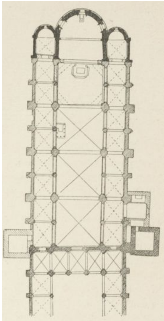
FIG. 186. ÉGLISE DE SAINT-AMBROISE A MILAN (ITALIE. (Plan.)
