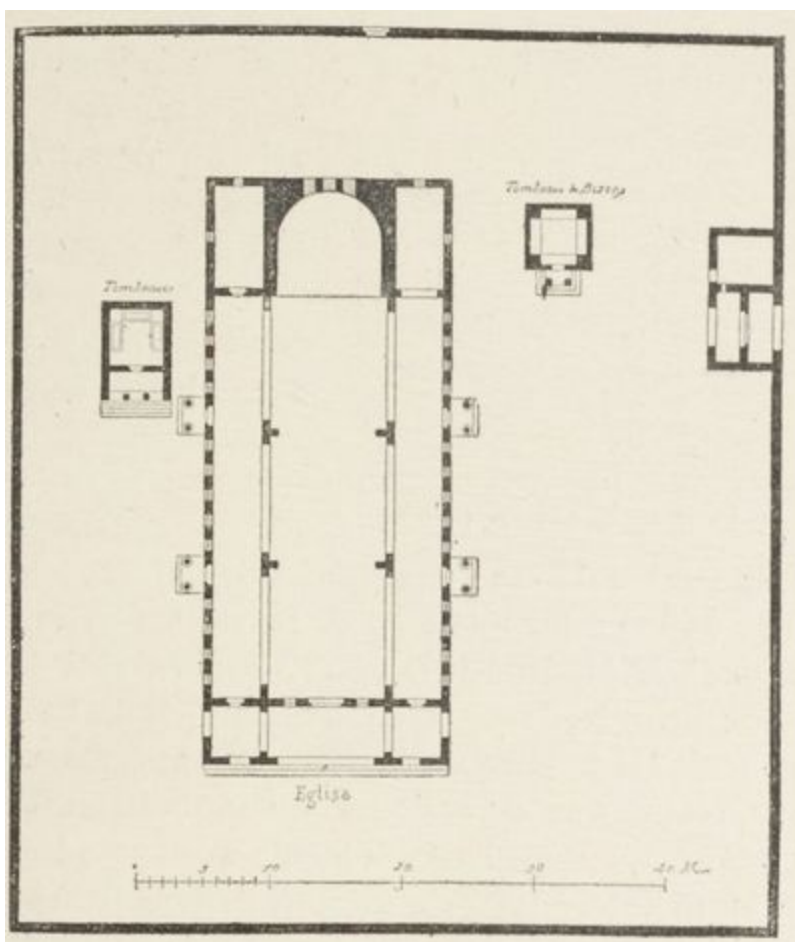
FIG. 48. — ÉGLISE DE ROUEIHA. (SYRIE CENTRALE). (Plan.)
