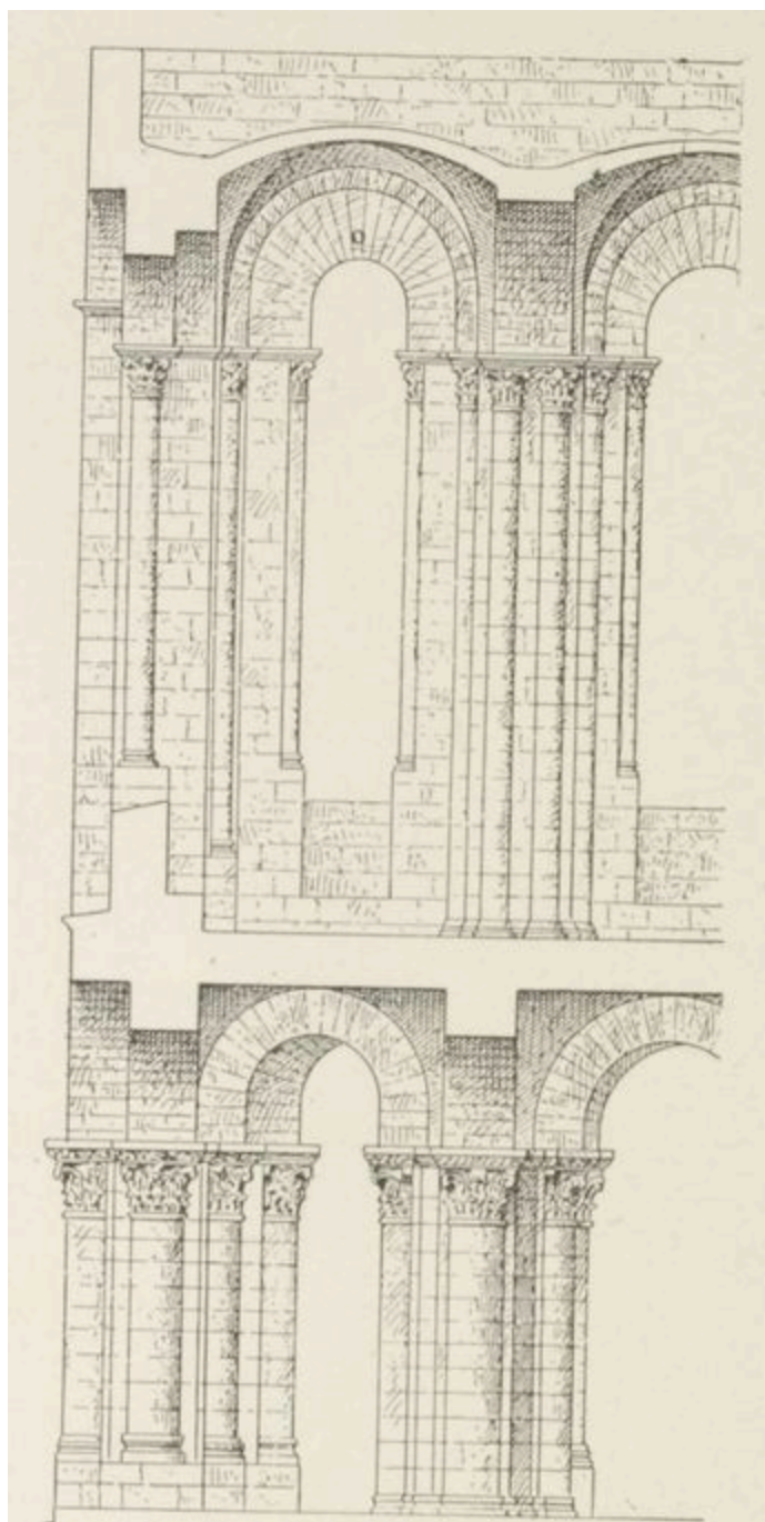
FIG. 136. — NARTHEX DE L'ÉGLISE DE SAINT-BENOIT-SUR-LOIRE. (Coupe.)
