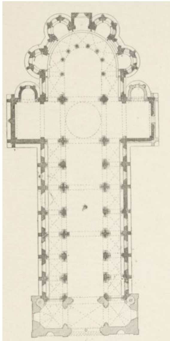
FIG. 137. ÉGLISE DE SAINT-PAUL, A ISSOIRE. (Plan.
