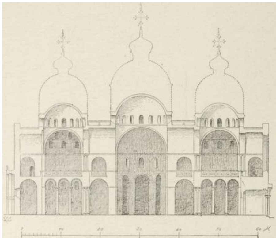
FIG. 154. — ÉGLISE DE SAINT-MARC, A VENISE. (Coupe longitudinale.)
