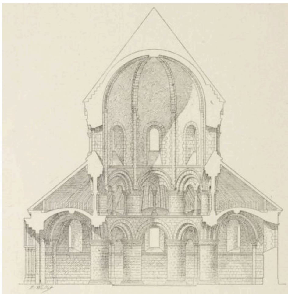
FIG. 127. — ÉGLISE DU SAINT-SÉPULCRE, A CAMBRIDGE ANGLETERRE). (Coupe.)
