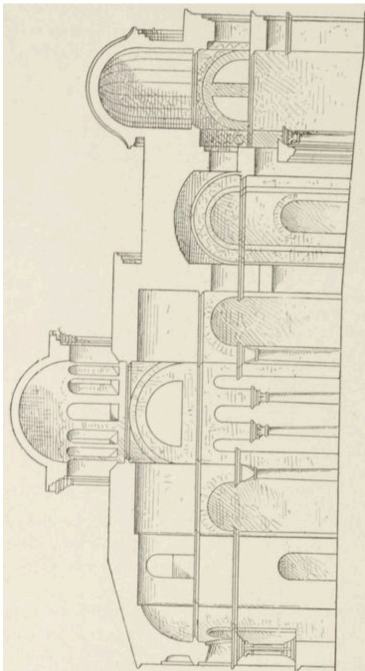
FIG. 73. — ÉGLISE DE THÉOTOCOS A CONSTANTINOPLE. (Coupe longitudinale, de l'abside au narthex.)
