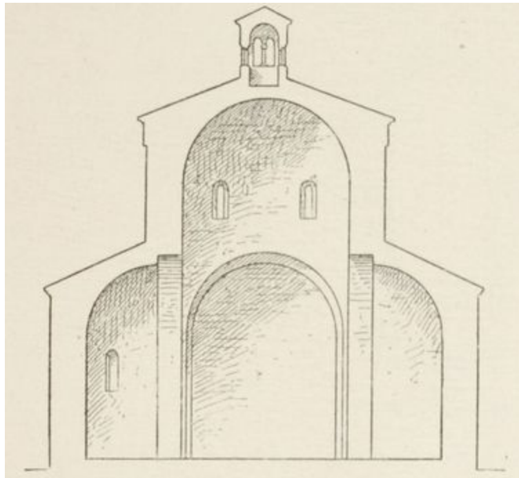
FIG. 93. — BAPTISTÈRE DE BIELLA (ITALIE). (Coupe transversale.)
