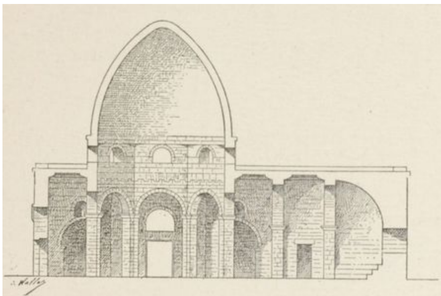
FIG. 39. — BAPTISTÈRE DE SAINT-GEORGES D'EZRA (SYRIE CENTRALE). (Coupe longitudinale.)
