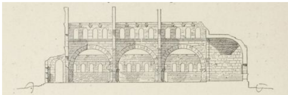
FIG. 46. — ÉGLISE DE ROUEIHA (SYRIE CENTRALE). (Coupe longitudinale.)
