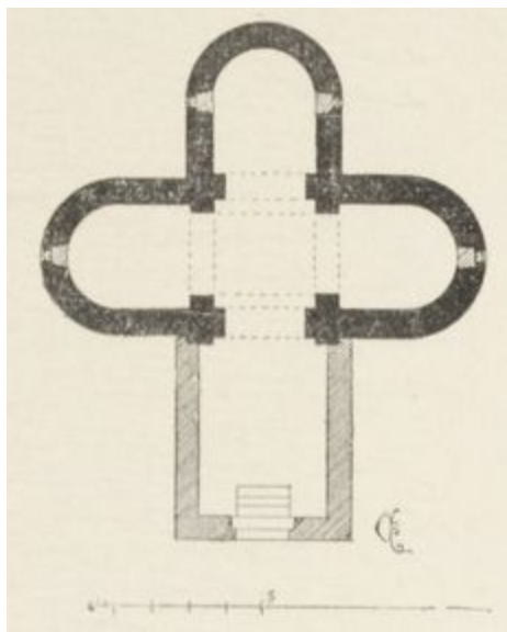
FIG. 97. CHAPELLE DE SAINT-GERMAIN A QUERQUEVILLE (PRÈS DE CHERBOURG). (Plan.)
