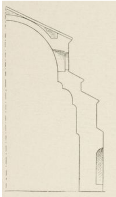
FIG. 76. ÉGLISE DE SANTA-FOSCA, A TORCELLO. (Coupe diagonale.)
