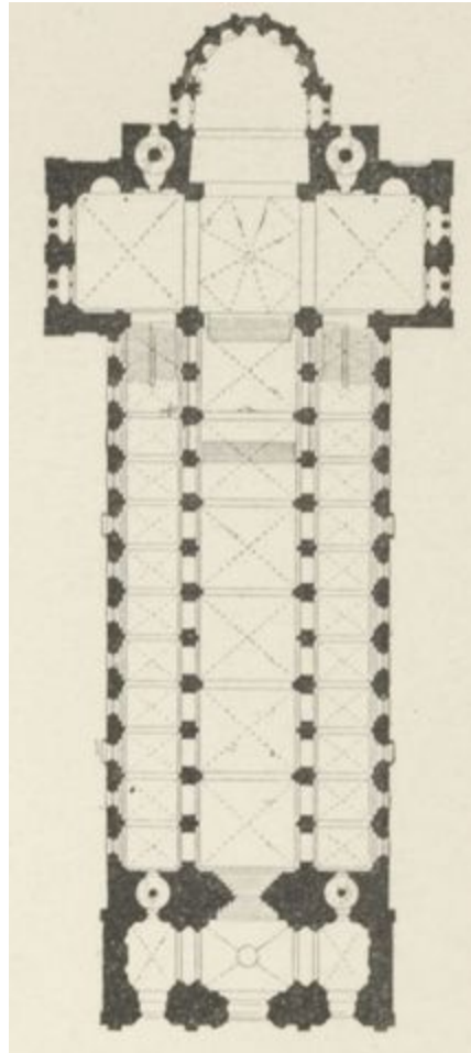
FIG. 183. ÉGLISE DE SPIRE, BAVIÈRE (ALLEMAGNE). (Plan.)
