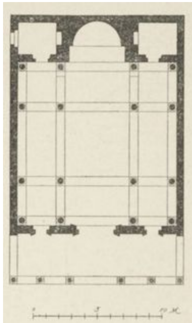
FIG. 6. PRÉTOIRE DE MOUSMIEH (SYRIE CENTRALE). (Plan )
