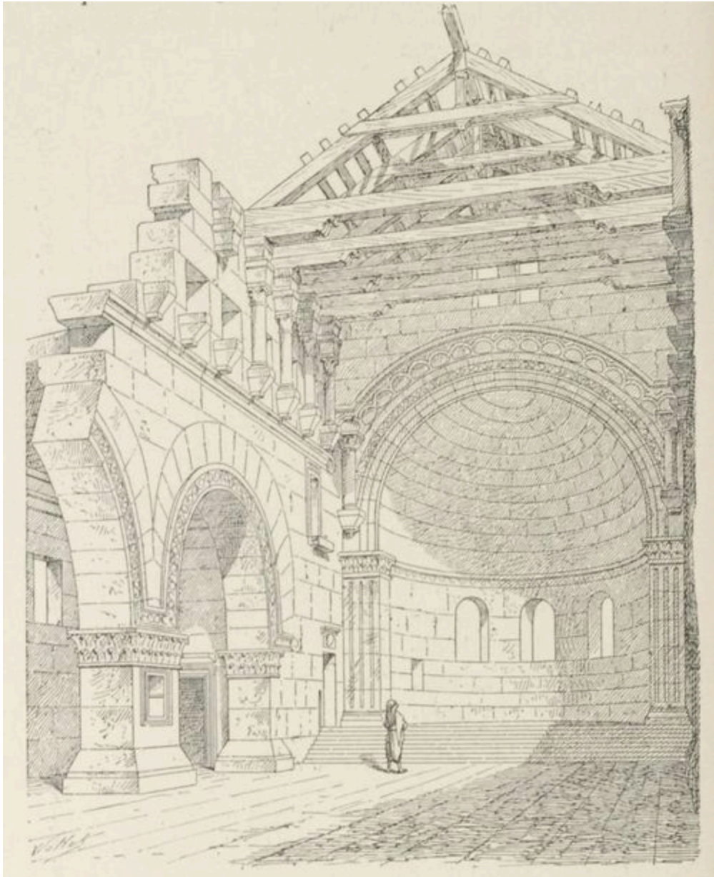
FIG. 45. — ÉGLISE DE QALB-LOUZEH (SYRIE CENTRALE). (Vue perspective intérieure vers l'abside.)
