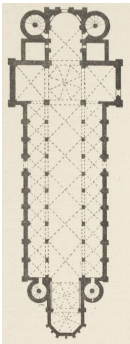
FIG. 181. — ÉGLISE DE WORMS, HESSE-DARMSTADT (ALLEMAGNE). (Plan.)
