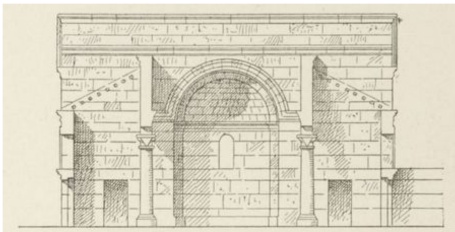
FIG. 32. — BAPTISTÈRE DE MOUDJELEIA (SYRIE CENTRALE). (Coupe transversale.)
