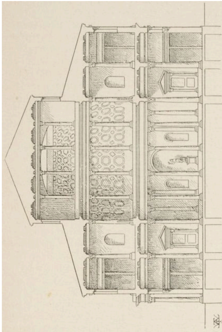
FIG. 5. — BASILIQUE ULPIENNE, A ROME (Coupe transversale.)
