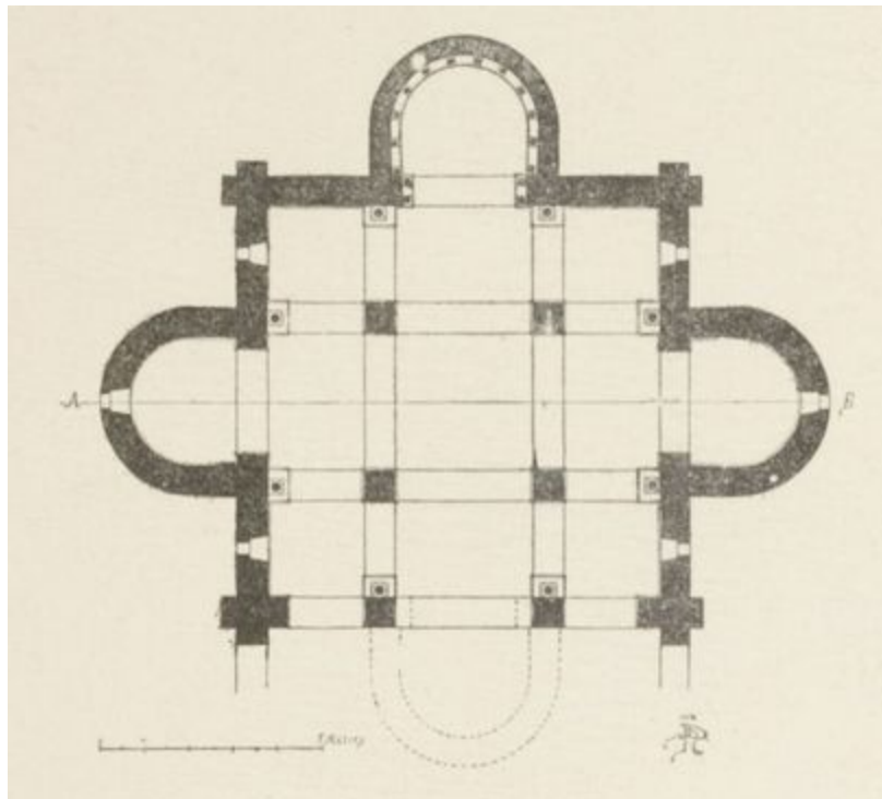
FIG 86. — ÉGLISE DE GERMINY-DES-PRÉS (FRANCE). (Plan.)
