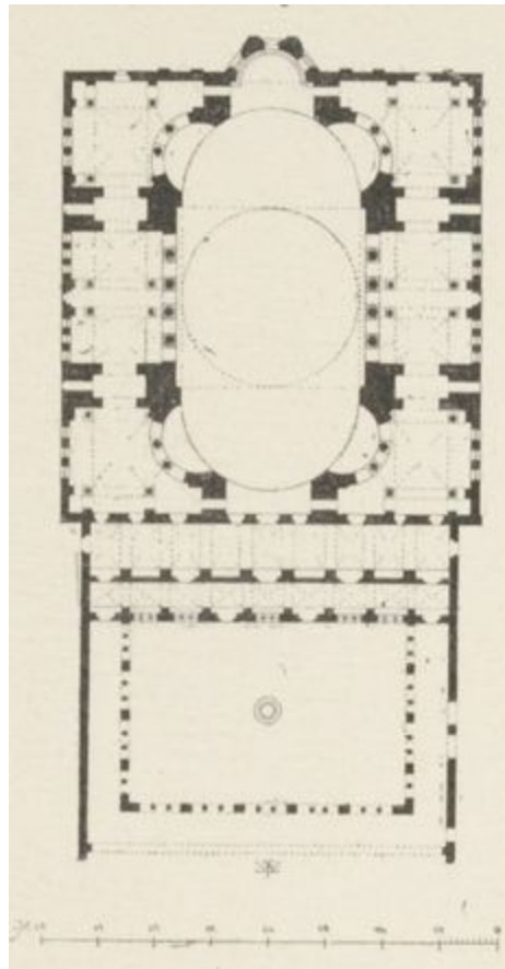
FIG. 70. ÉGLISE DE SAINTE-SOPHIE A CONSTANTINOPLE. (Plan)
