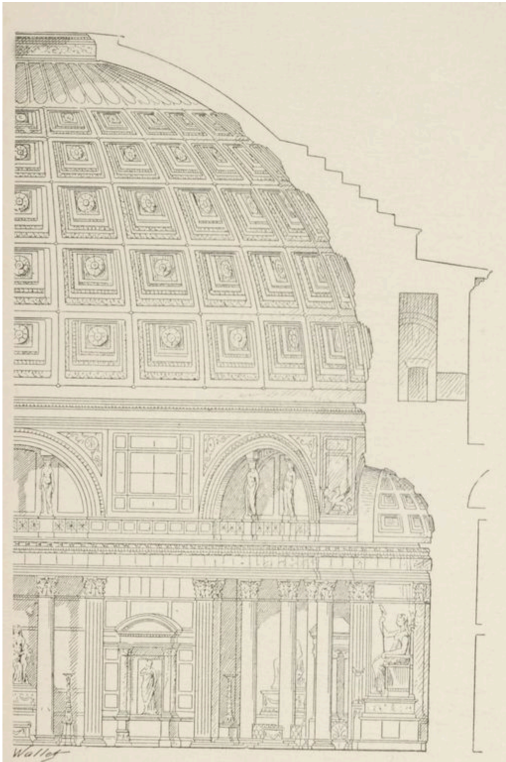
FIG. 12. LE PANTHÉON DE ROME. (Coupe longitudinale.)
