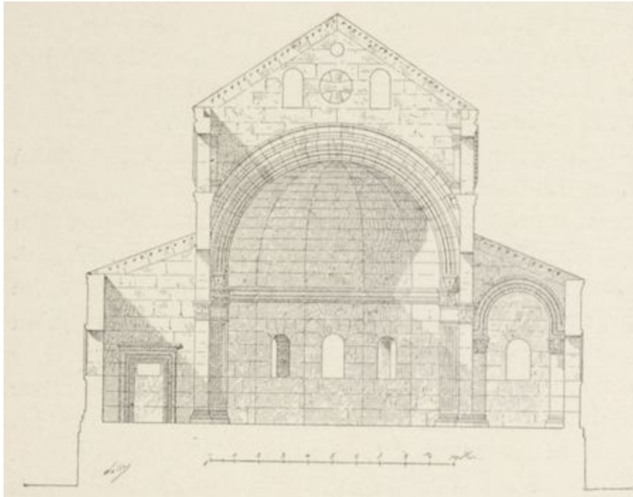
FIG. 50. — ÉGLISE DE TOURMANIN (SYRIE CENTRALE). (Coupe transversale.)
