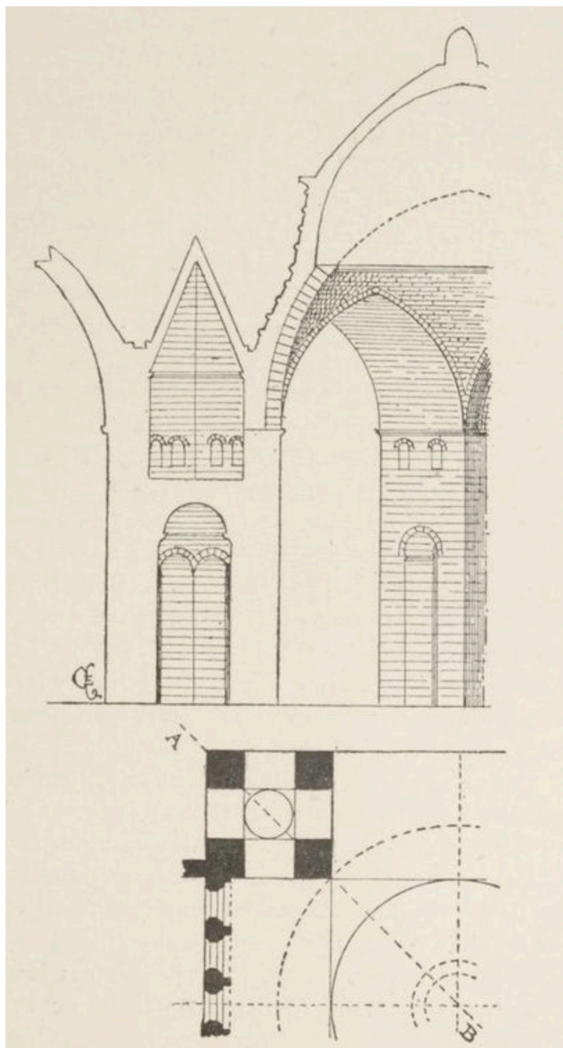
FIG. 159. — ÉGLISE SAINT-FRONT. A PÉRIGUEUX. (Coupe d'un pendentif sur la diagonale A B.)
