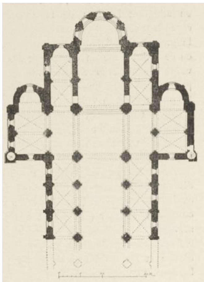
FIG. 106. ÉGLISE ABBATIALE DE CERISY-LA-FORÊT MANCHE (FRANCE). (Plan.)
