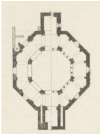
FIG. 122. — ÉGLISE D'OTTMARSHEIM (ALSACE). (Plan.)
