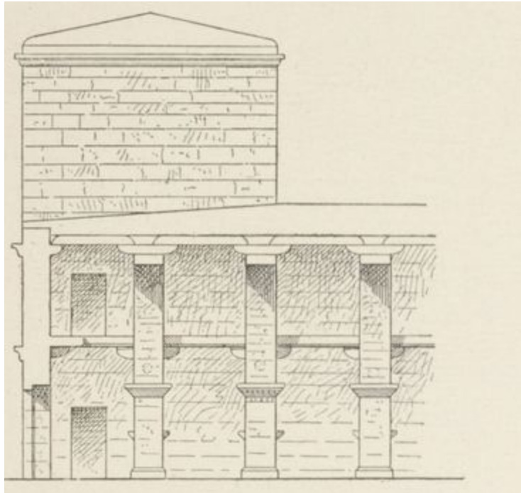
FIG. 30. — BASILIQUE DE TAFKHA (SYRIE CENTRALE). (Coupe longitudinale sur C-D du plan.)
