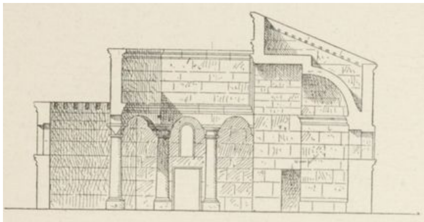
FIG. 33. — BAPTISTÈRE DE MOUDJELEIA (SYRIE CENTRALE). (Coupe longitudinale.)
