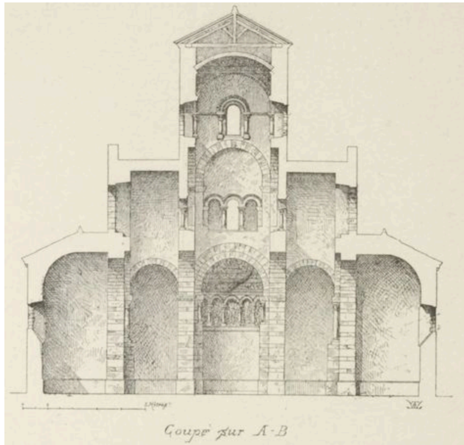
FIG. 87. — ÉGLISE DE GERMINY-DES-PRÉS (FRANCE) (Coupe transversale.)
