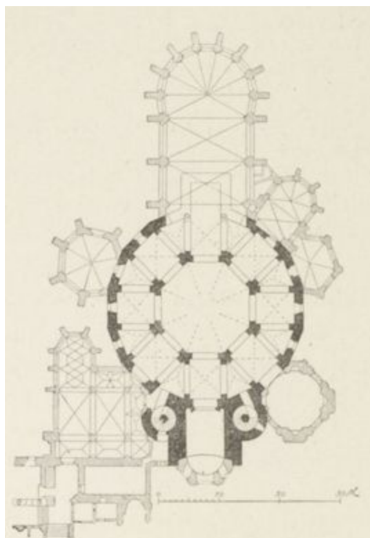
FIG. 83. CHAPELLE DU PALAIS DE CHARLEMAGNE A AIX-LA-CHAPPELLE. (Plan.)
