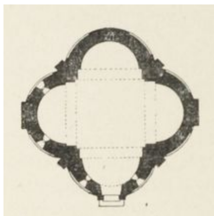
FIG. 92. — BAPTISTÈRE DE BIELLA (ITALIE). (Plan.)
