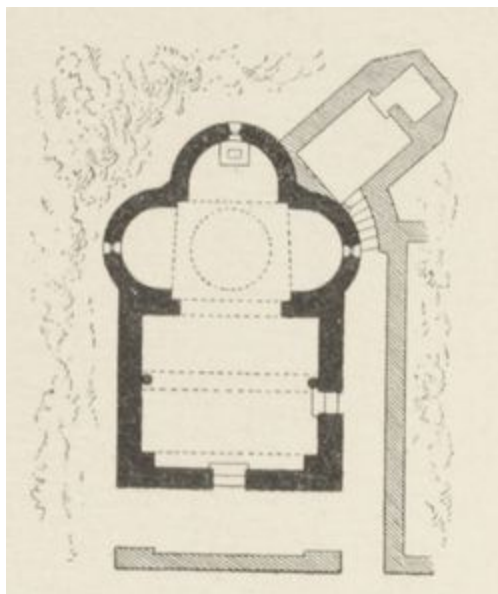
FIG. 95. CHAPELLE DE LA TRINITÉ (ILE SAINT-HONORAT DE LÉRINS (Plan.)
