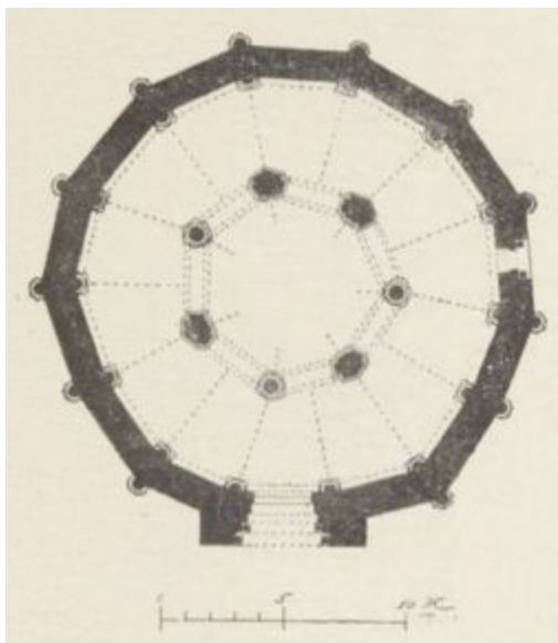
FIG. 124. — ÉGLISE DE RIEUX- MÉRINVILLE (FRANCE). (Plan.)
