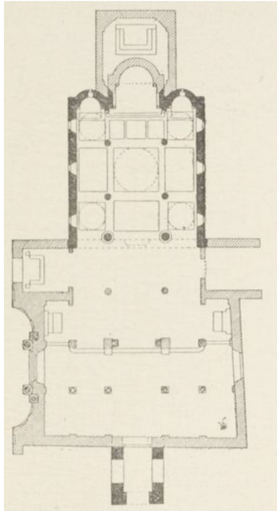
FIG. 88. — ÉGLISE DE LA MARTORANA A PALERME (SICILE). (Plan.)
