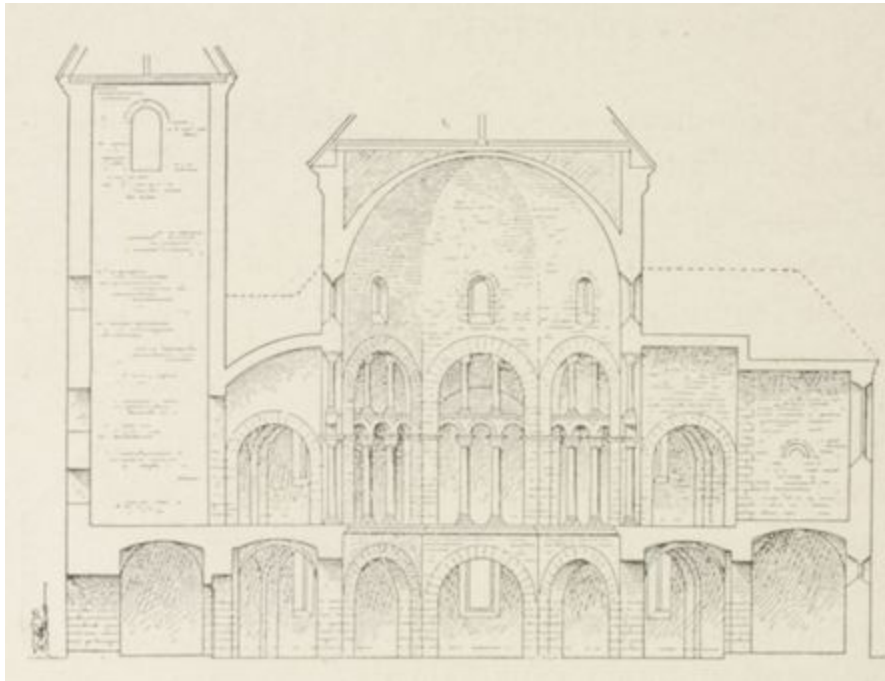
FIG. 123. — ÉGLISE D'OTTMARSHHEIM (ALSACE). (Coupe longitudinale.)
