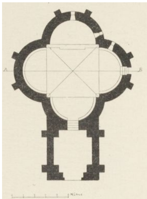
FIG. 100. CHAPELLE SAINTE-CROIX DE MONTMAJOUR (PRÈS D'ARLES). (Plan.)
