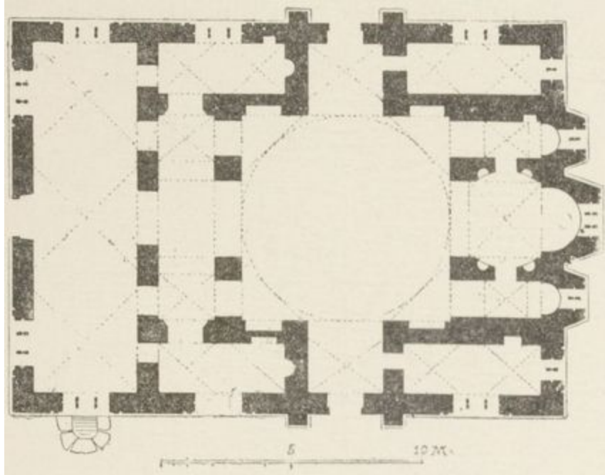
FIG. 79. — ÉGLISE DU MONASTÈRE DE DAPHNI, PRÈS D'ATHÈNES 28 , (Plan.)
