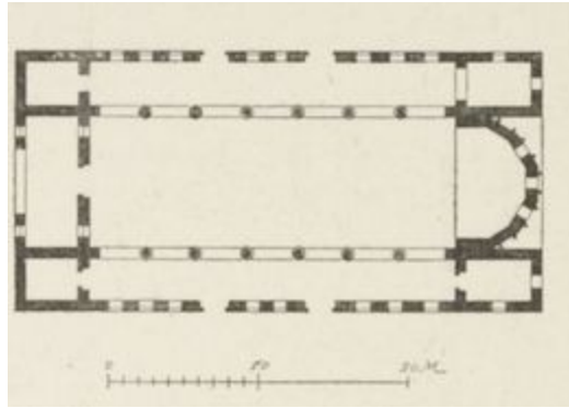
FIG. 49. — ÉGLISE DE TOURMANIN (SYRIE CENTRALE). (Plan.)
