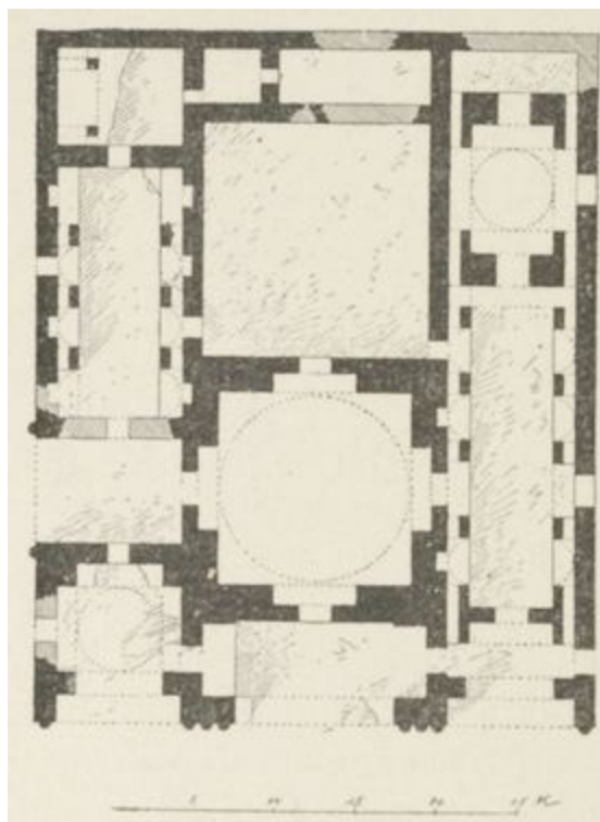
FIG. 14. PALAIS DE SARVISTAN (PERSE). (Plan.) (D'après les dessins de M. Dieulafoy.)
