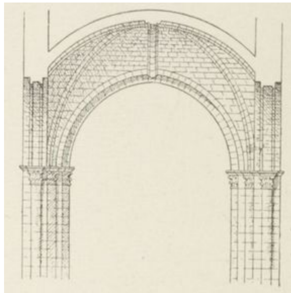
FIG. 177. — ÉGLISE DE SAUMUR. (Coupe de la voûte.)
