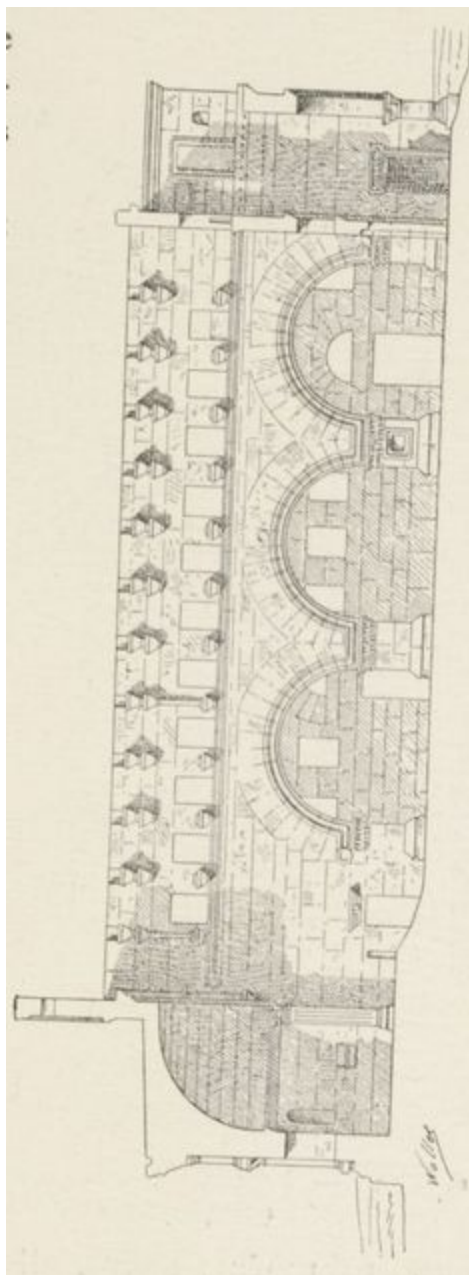
FIG. 44. — ÉGLISE DE QALB-LOUZEH (SYRIE CENTRALE). (Coupe longitudinale)
