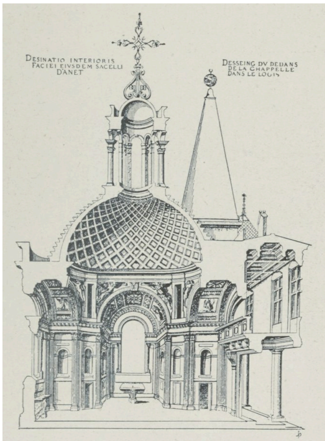
Fig. 126. – CHAPELLE DU CHATEAU D'ANET, COUPE DE L'INTÉRIEUR (PAR PHILIBERT DE L'ORME). d'après le dessin de Du Cerceau (Après 1548).
