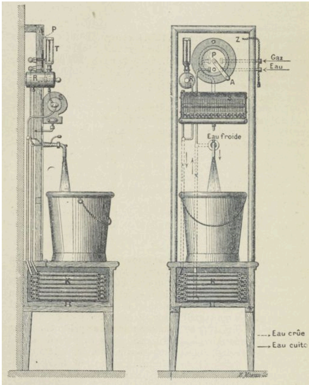
Fig. 127. — Stérilisateur de David Grove, de Berlin. K, réfrigérant ; S, chauffeur rapide ; R, réservoir ; P, disque portant manivelle ; ZA, trajet de la manivelle ; T, thermomètre.
