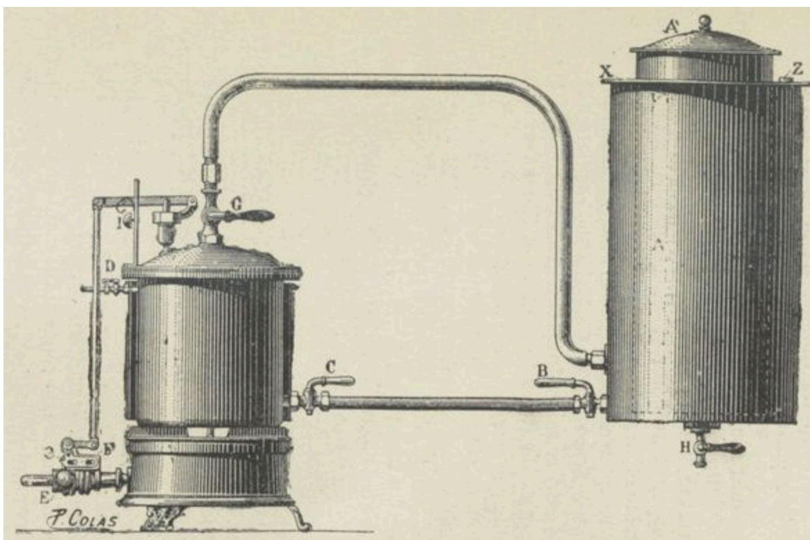
Fig. 128, — Stérilisateur de la Société de la force motrice.
