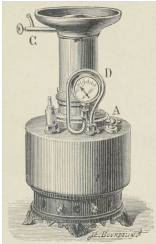
Fig. 131. — Stérilisateur domestique de Rouart, Geneste et Herscher.
