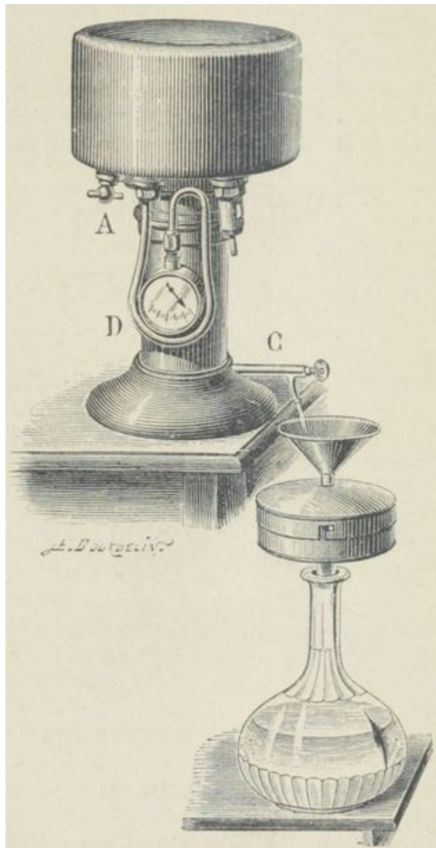
Fig. 132. — Stérilisateur en fonction.
