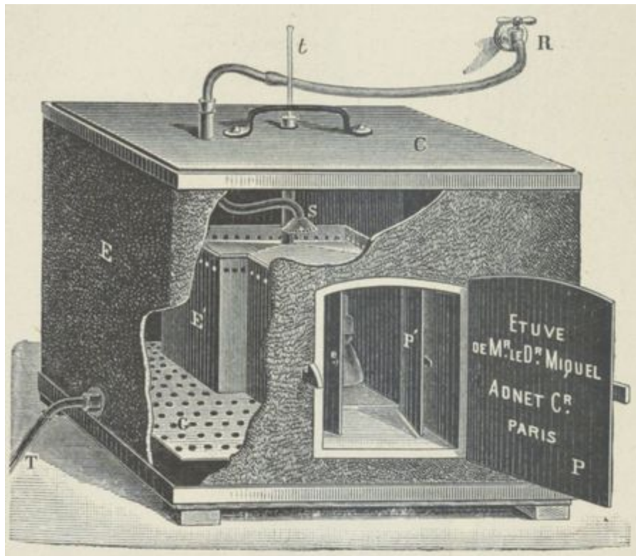
Fig. 37. — Étuve glacière à basses températures.
