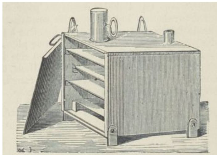
Fig. 24. — Appareil à stérilisation à air sec.
