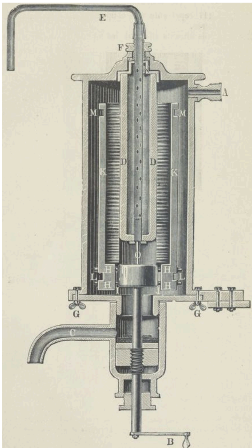
Fig. 120. — Filtre Berkefeld muni d'une brosse pour le nettoyage mécanique.
