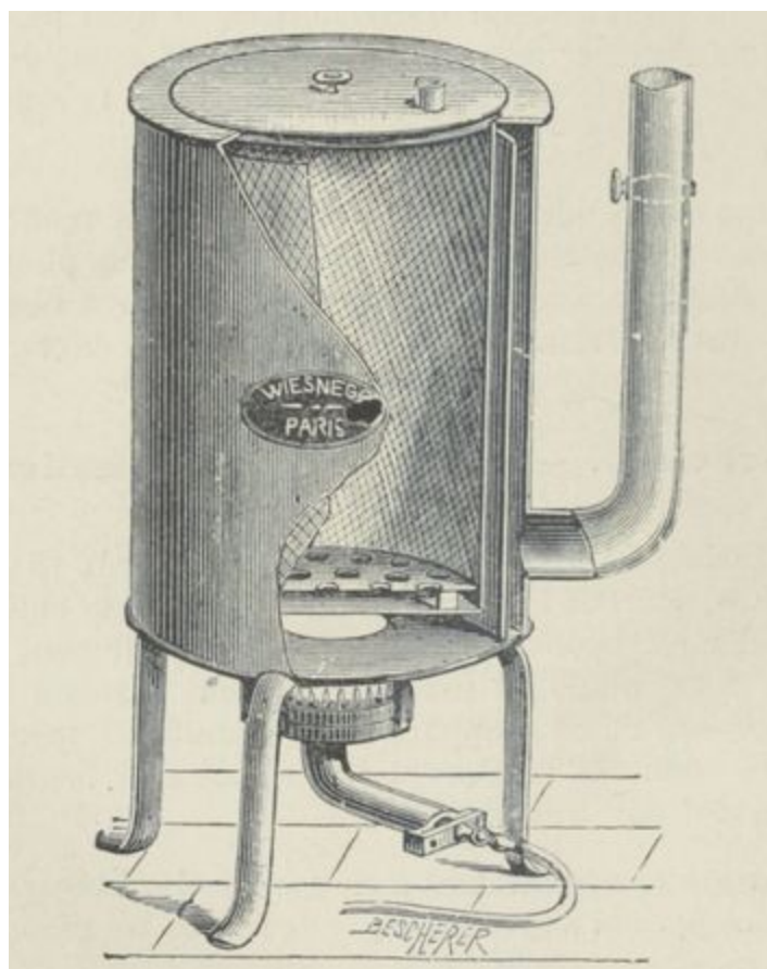
Fig. 25. — Four de Pasteur pour flamber les ballons.
