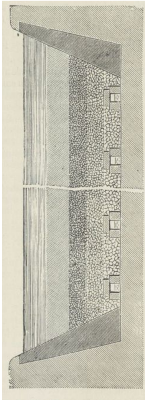
Fig. 99. — Puits de la Compagnie Lambeth, filtration de haut en bas
