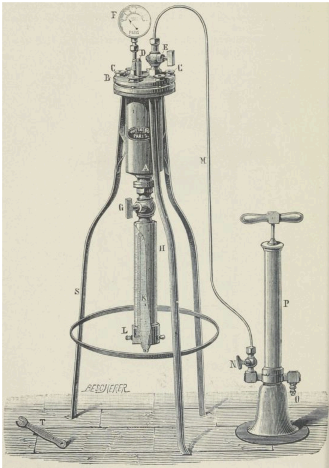
Fig. 28. — Filtre à pression graduée.
