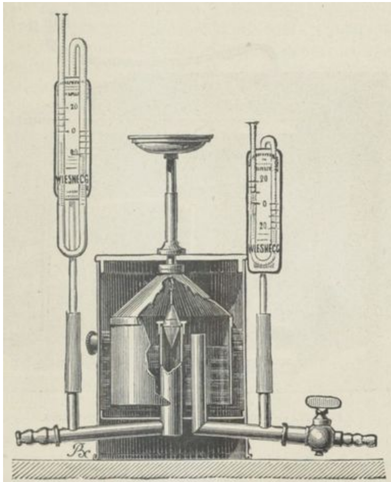
Fig. 36. — Régulateur de pression Moitessier.
