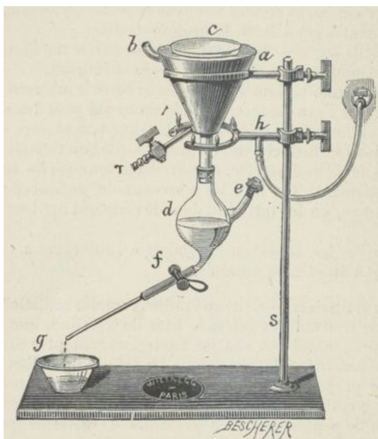
Fig. 47. — Appareil à filtration à chaud.
