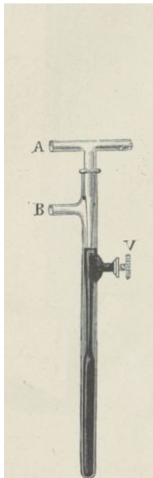
Fig. 33 . — Régulateur à mercure, de Chancel.
