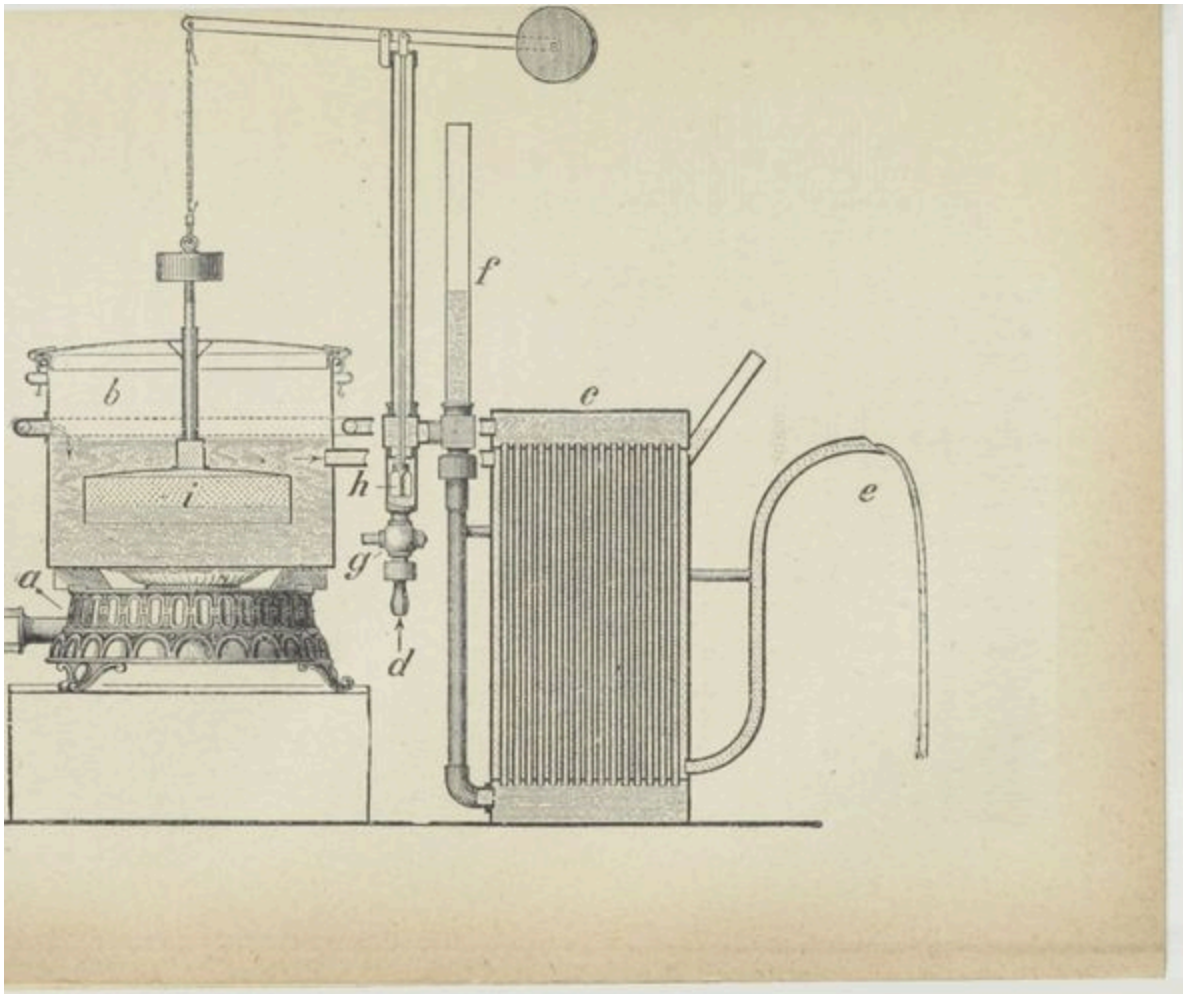
Fig. 126. Stérilisateur de Siemens.
