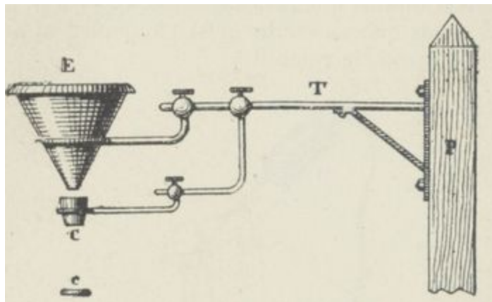
Fig. 42. — Appareil pour récolter les eaux de pluie.
