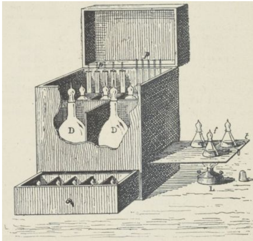
Fig. 43. — Nécessaire pour l'analyse bactériologique des eaux ;
