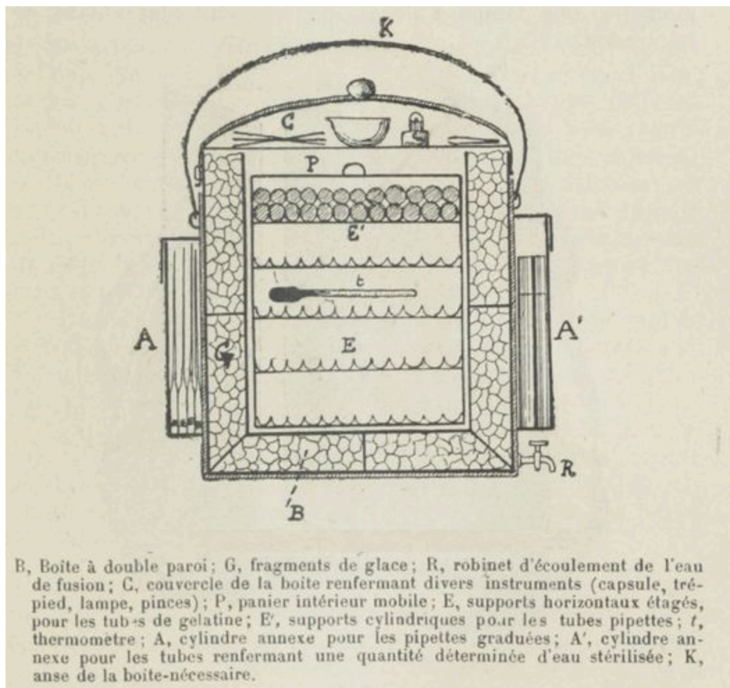
Fig. 44. — Nécessaire bactériologique du D r G. Roux.
