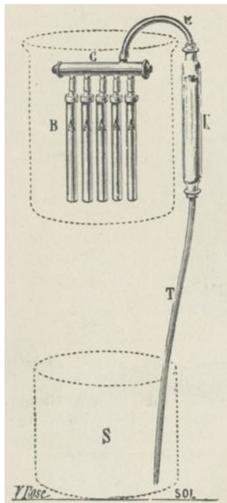
Fig. 108. — Filtre Chamberland, sans pression avec amorceur.
