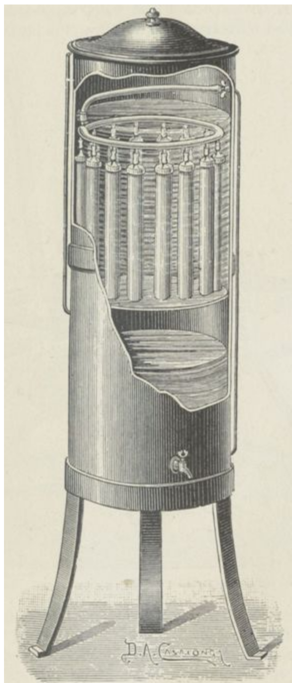
Fig. 106. — Filtre Chamberland, filtre de ménage sans pression.
