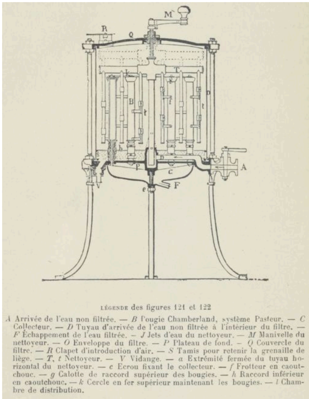
Fig. 122. — Filtre nettoyeur du système André. LÉGENDE des figures 121 et 122
