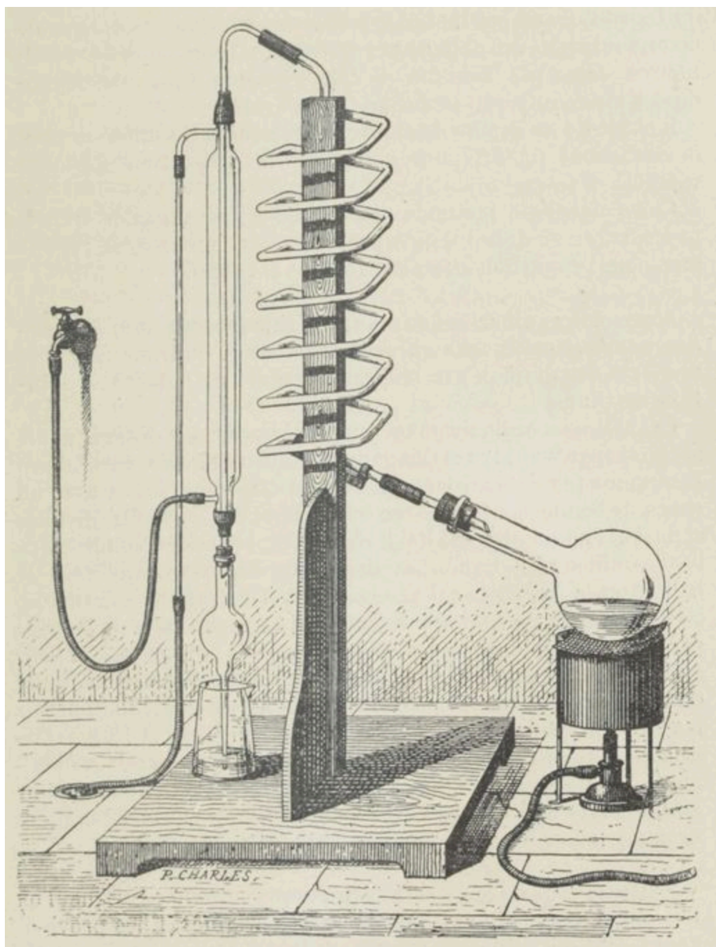
Fig. 13. — Appareil de Schlöesing.
