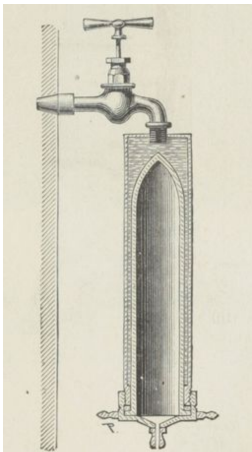
Fig. 111. — Filtre Mallie avec pression.
