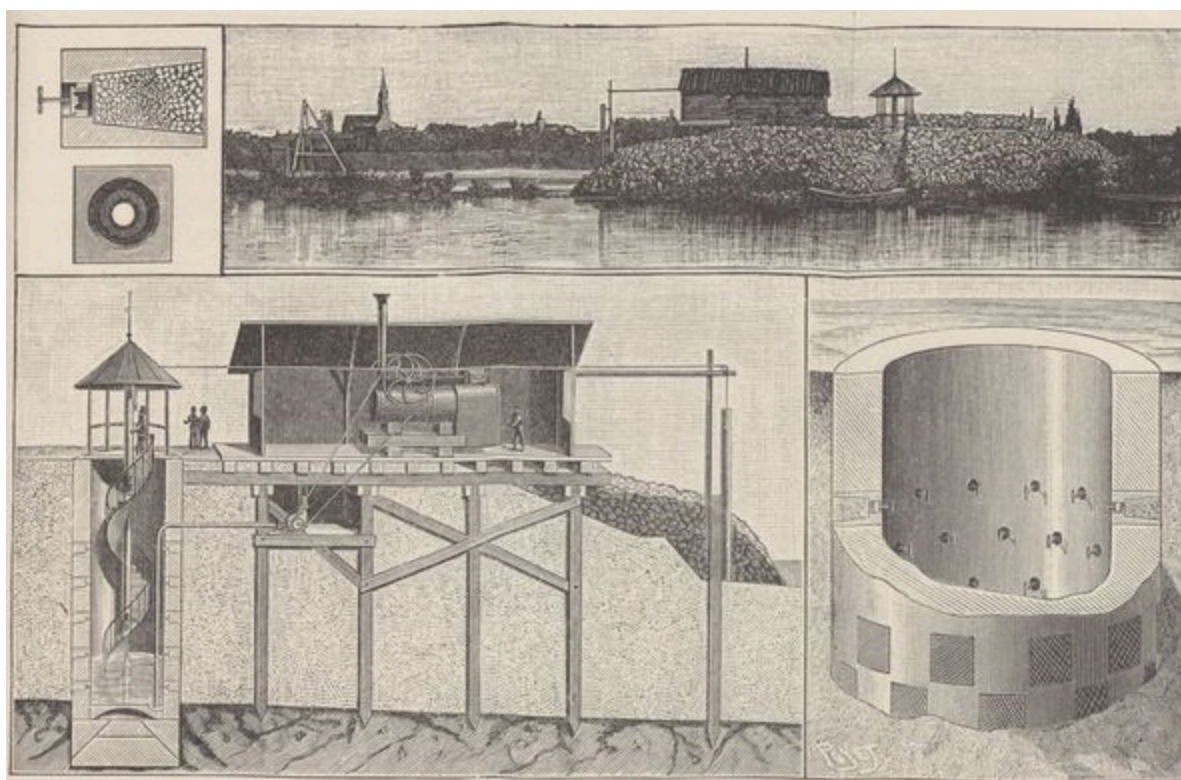
Fig. 98. — Puits filtrant Lefort.
