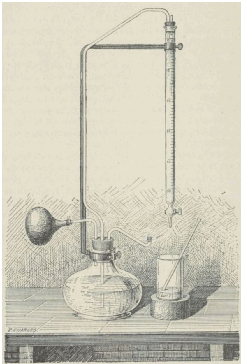
Fig. 8. — Burette automatique de Guichard.
