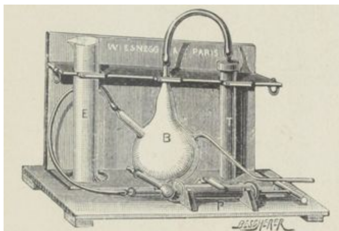
Fig. 29. — Appareil de Chamberland pour la stérilisation par filtration.
