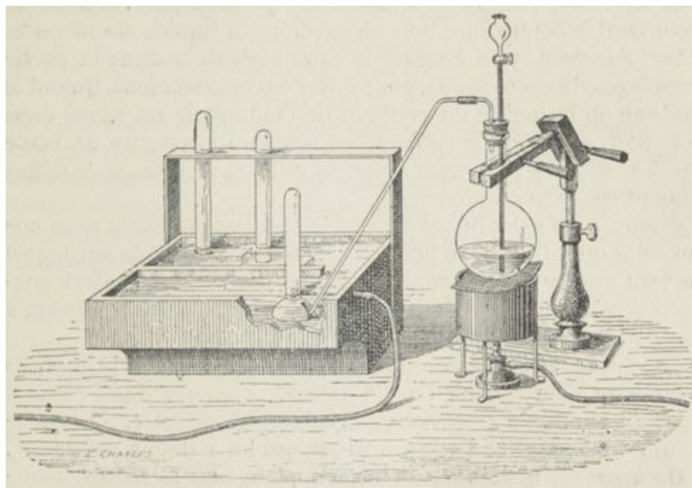
Fig. 12. — Dosage de l'acide nitrique.
