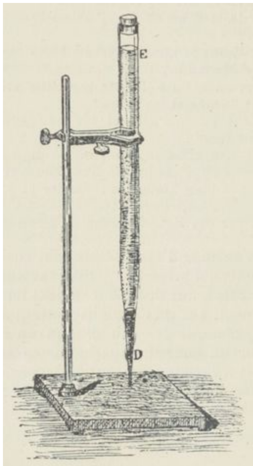
Fig. 5. — Appareil pour recueillir l'eau pour l'examen microscopique.
