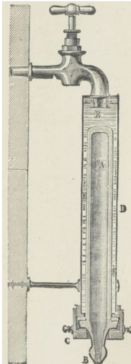
Fig. 104. — Filtre Chamberland.
