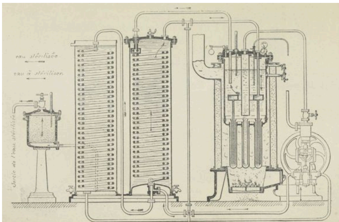
Fig. 129. — Appareil à stériliser grand modèle.
