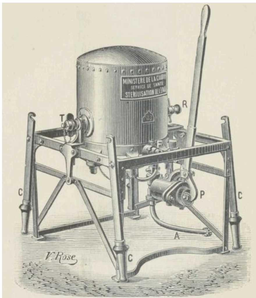
Fig. 107. — Filtre transportable ou filtre de campagne (Boulet et C ie ).
