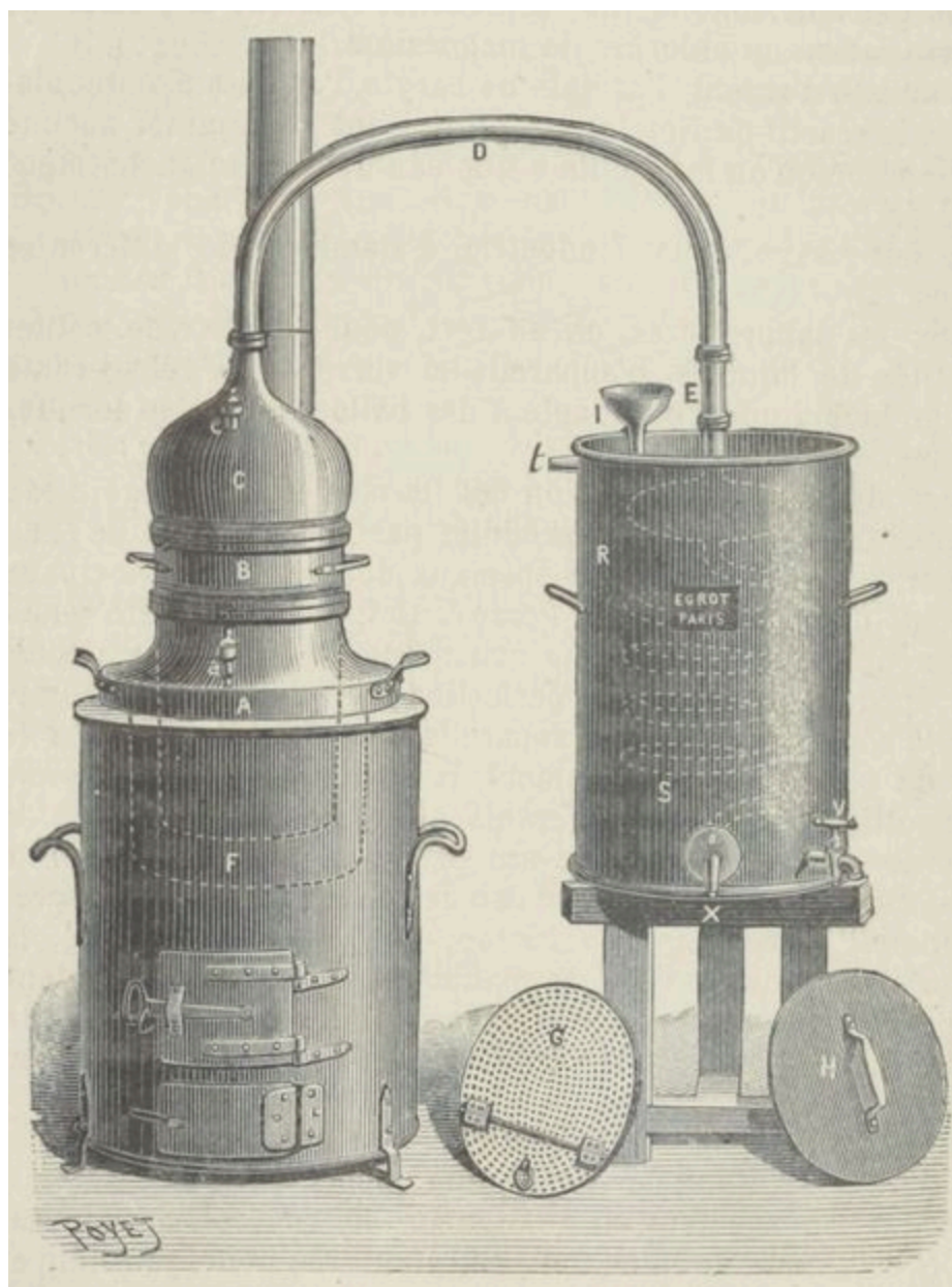
Fig. 1. — Alambic de distillerie.
