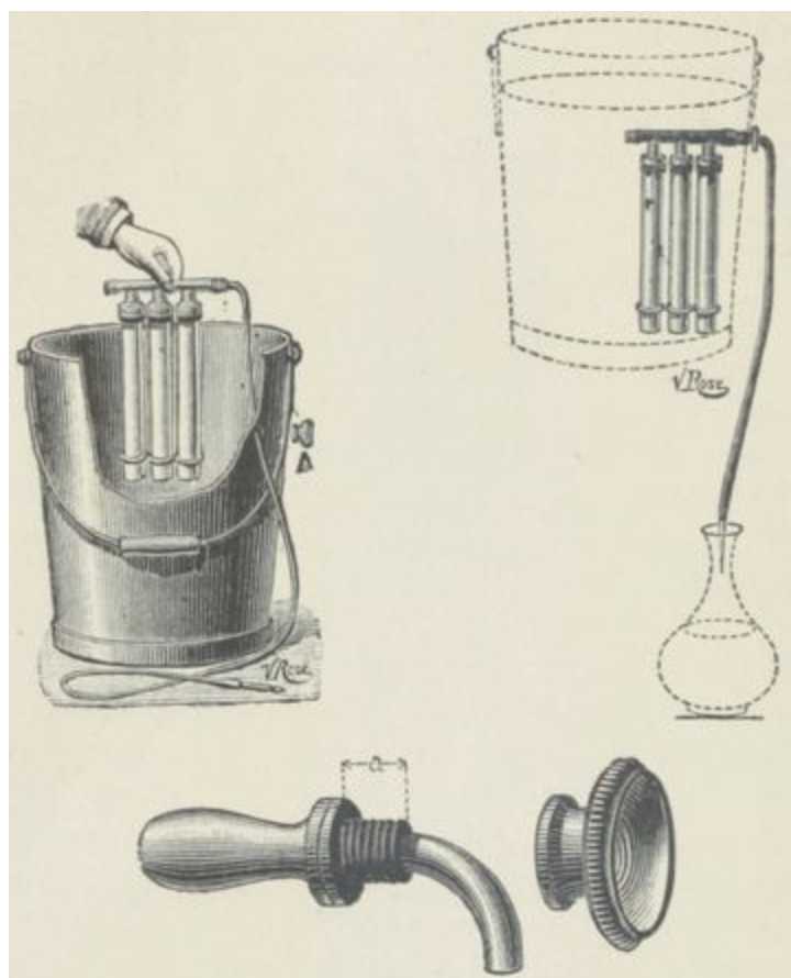
Fig. 109. — Filtre Cosmos.
