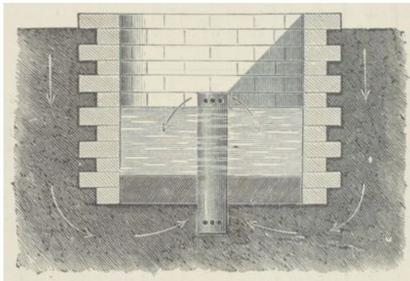
Fig. 3. — Utilisation d'un puits sans profondeur.
