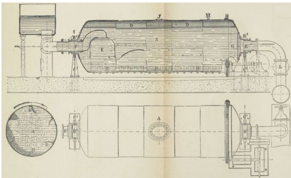
Fig. 135. — Purificateur rotatif Anderson.
