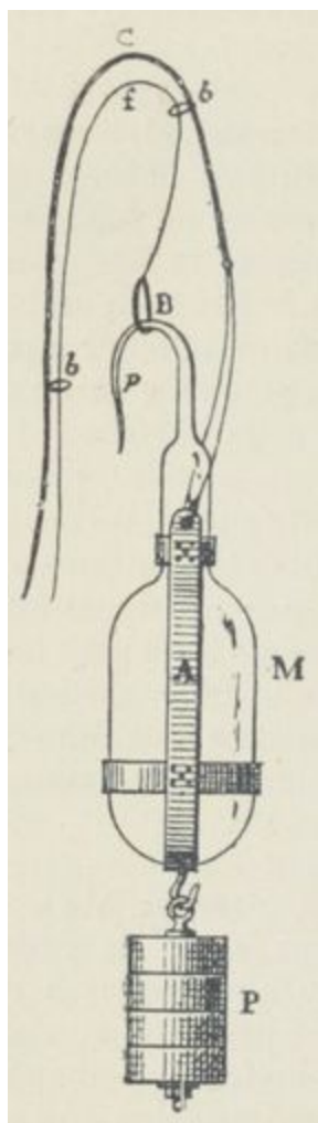
Fig. 38. — Appareil pour prélever les eaux à diverses profondeurs.
