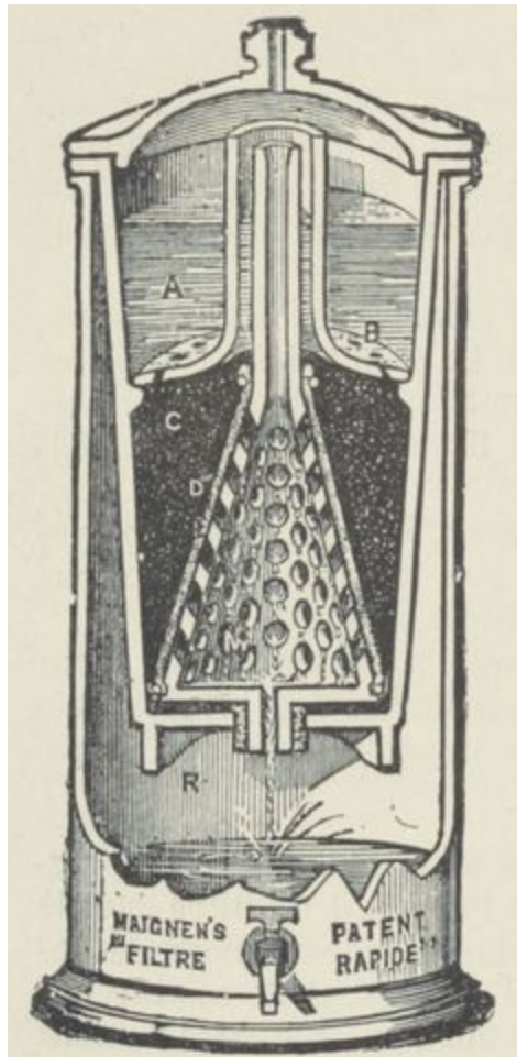
Fig. 101. — Filtre Maignen.
