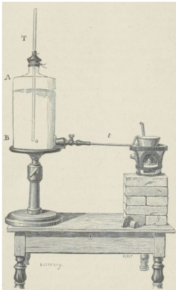
Fig. 10. — Appareil pour l'évaporation de l'eau.
