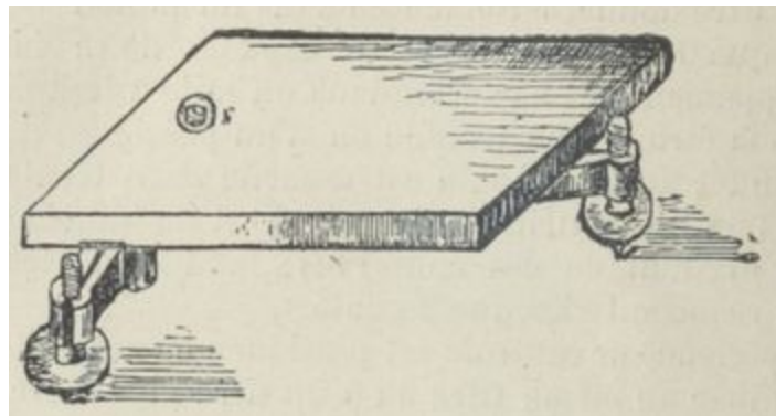
Fig. 50. — Planchette à vis calante.
