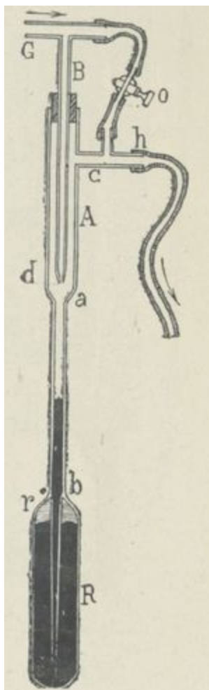
Fig. 35. — Régulateur à mercure et à éther, de M. Pittion.
