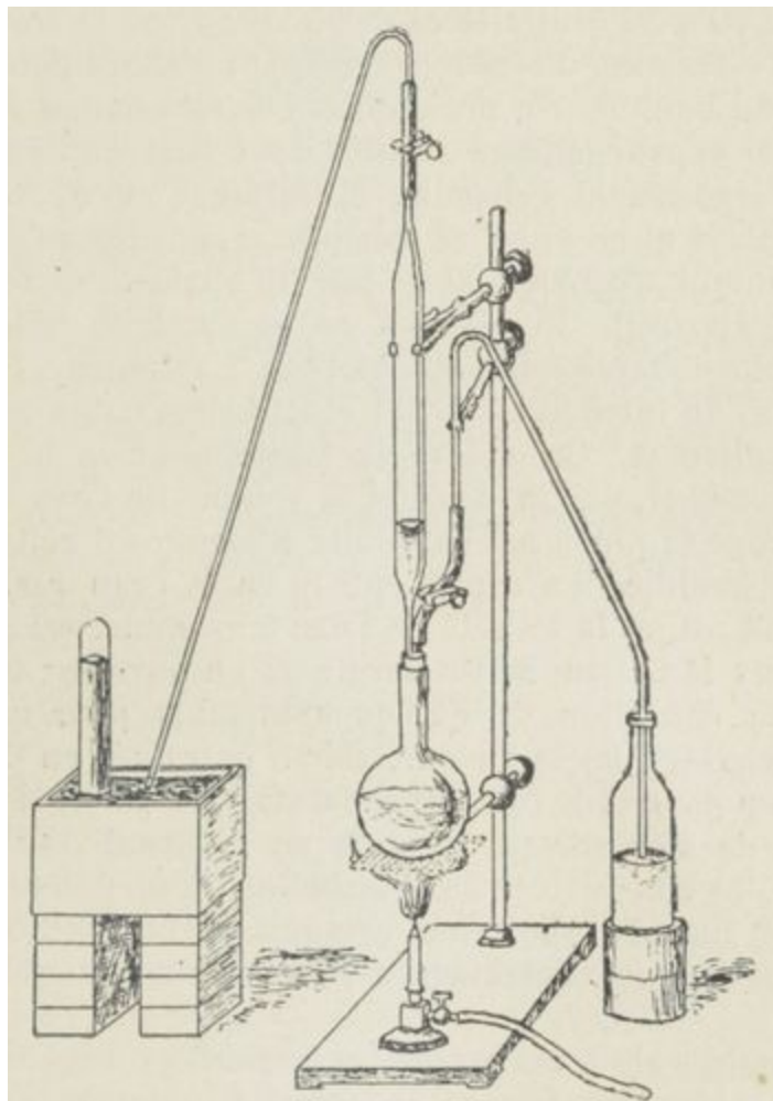
Fig. 15. — Appareil de M. Armand Gautier pour le dosage des gaz de l'eau.
