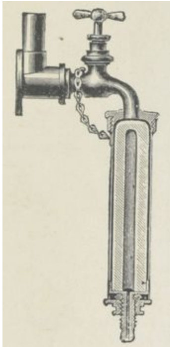
Fig. 118. — Filtre Berkefeld, filtrant de dehors en dedans.
