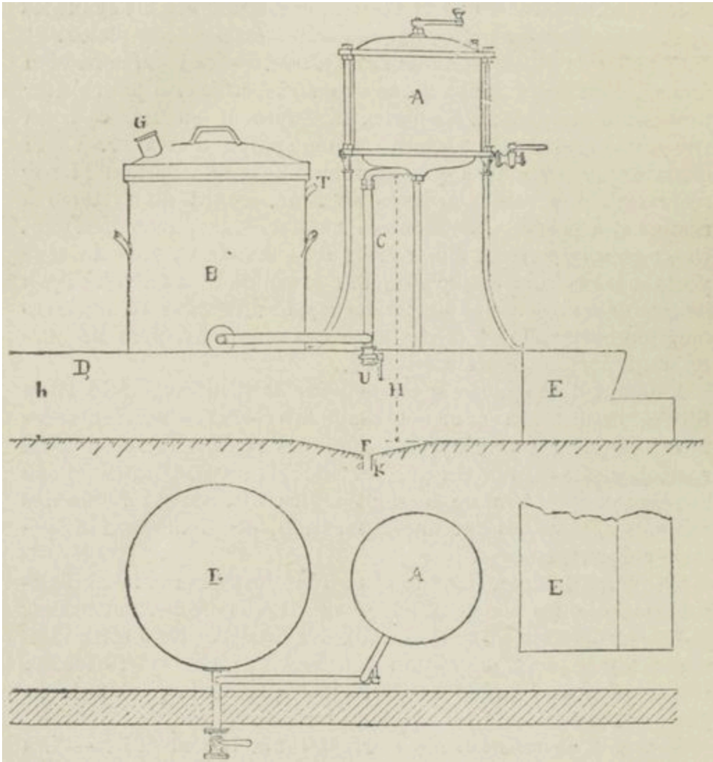
Fig. 123. — Installation des réservoirs pour filtre nettoyeur du système André.
