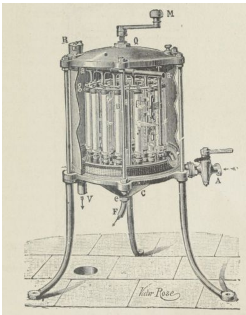
Fig. 121. — Filtre nettoyeur du système André.
