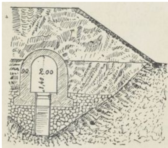
Fig. 96. — Galerie filtrante d'Angers.
