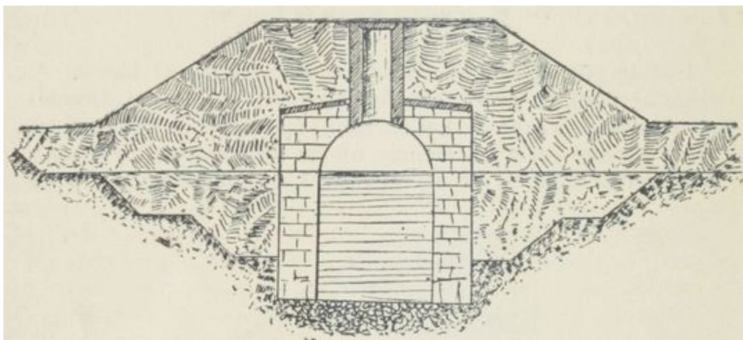
Fig. 97. — Galerie filtrante de Lyon.
