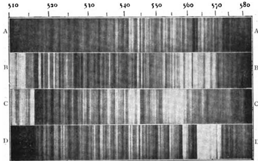
Fig. 60. — Spectres comparés d'étoiles de la 2 e , 3 e et 4 e catégorie. Photographie de l'observatoire de Yerkes. Partie verte et jaune du spectre.
