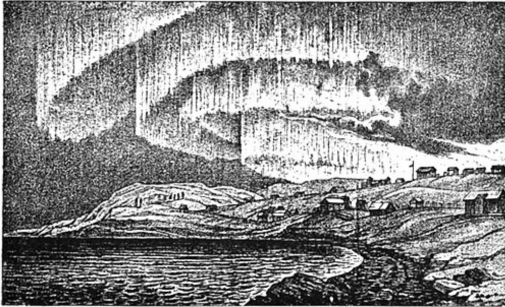
Fig. 41. — Draperies d'une aurore boréale, vue dans le Finmarken (Norvège septentrionale).
