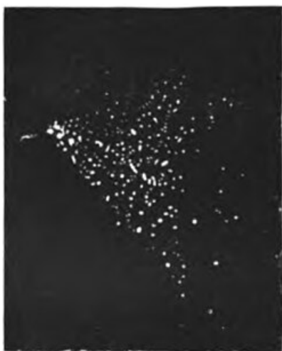
Fig. 58. — Amas d'étoiles cunéiforme, dans les Jumeaux.
