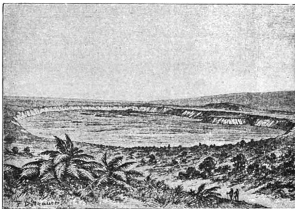
Fig. 9. — Le cratère du Kilauea, Hawaï.
