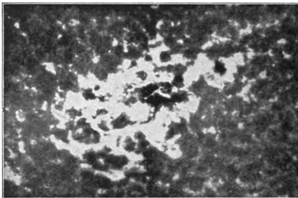
Fig. 28. — La grande tache du 9 octobre 1903. Photographie de la partie supérieure des facules de calcium, prise à l'aide de la partie moyenne de la raie H du calcium. — Les parties supérieures des facules recouvrent en grande partie la tache. Les facules s'étendent par conséquent beaucoup en s'élevant.
