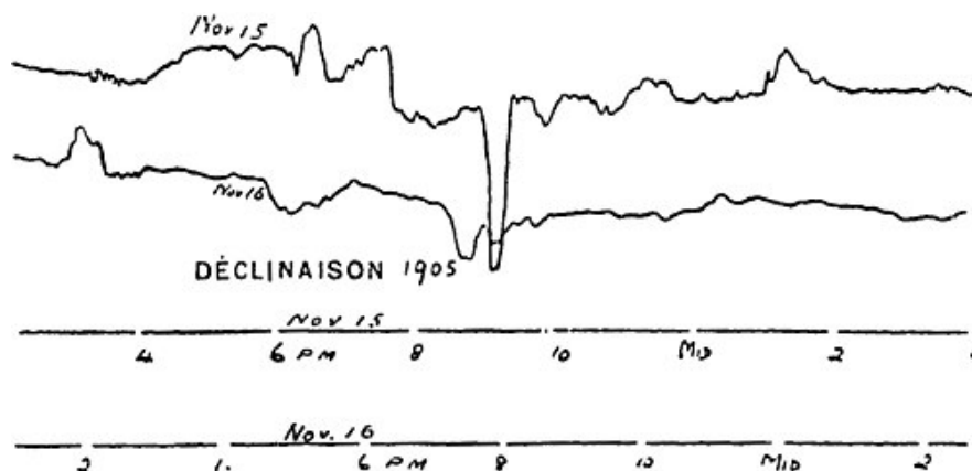
Fig. 42. — Variations de la déclinaison à Kew, près de Londres, les 15 et 16 novembre 1905. Une grande perturbation, qui se produit le 15 novembre à 9 heures du soir, correspond à la plus grande intensité de l'aurore.
