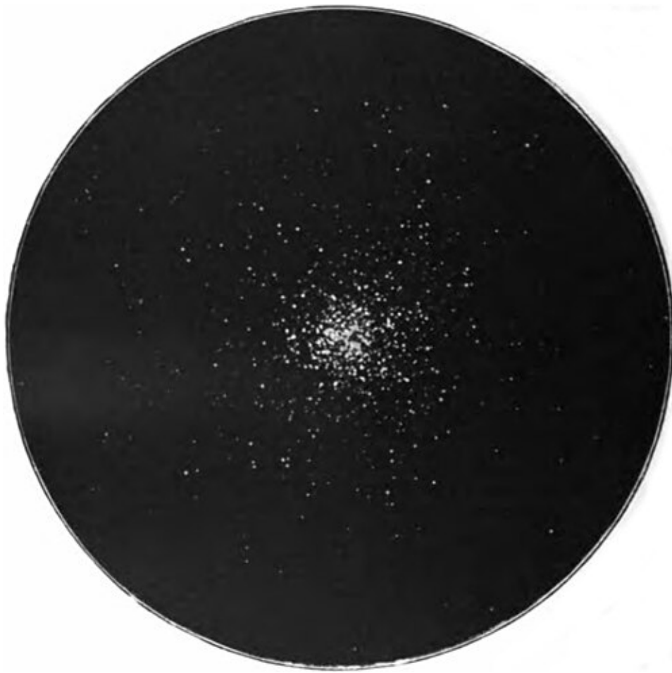
Fig. 56. — Amas d'étoiles d'Hercule (Messier 13). Photographie de l'observatoire de Yerkes. Un millimètre = 9,22 secondes d'arc.
