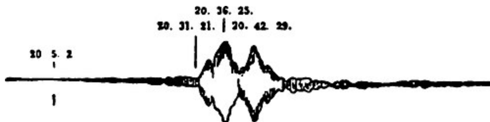
Fig. 16. — Séismogramme, relevé à Shide, dans l'île de Wight, le 31 août 1898.
