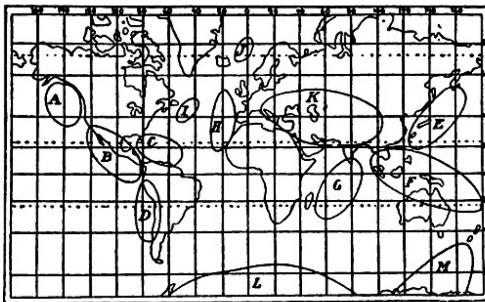
Fig. 10. — Carte des principaux centres séismiques, d'après les recherches de la British Association.
