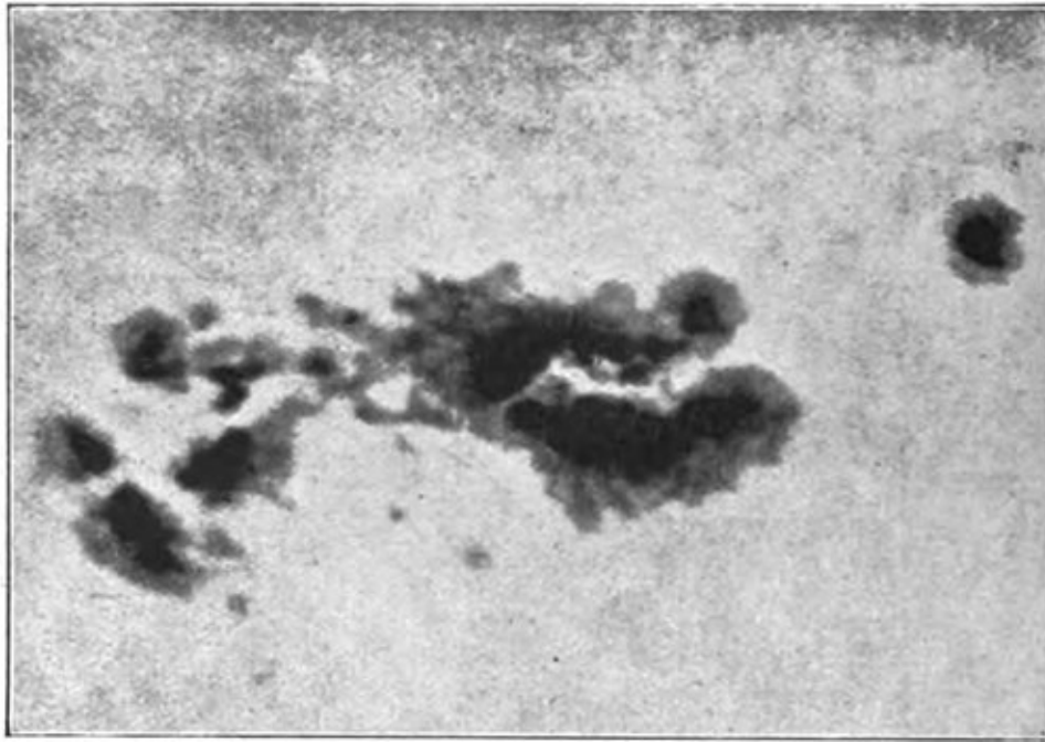
Fig. 26. — La grande tache du 9 octobre 1903, photographiée à l'aide du spectrohéliographe de Greenwich. Cette figure est photographiée comme à l'ordinaire. Elle montre la tache à la hauteur moyenne des facules de calcium. Les deux figures suivantes montrent la même tache, photographiée plus bas et plus haut dans les mêmes facules de calcium.
