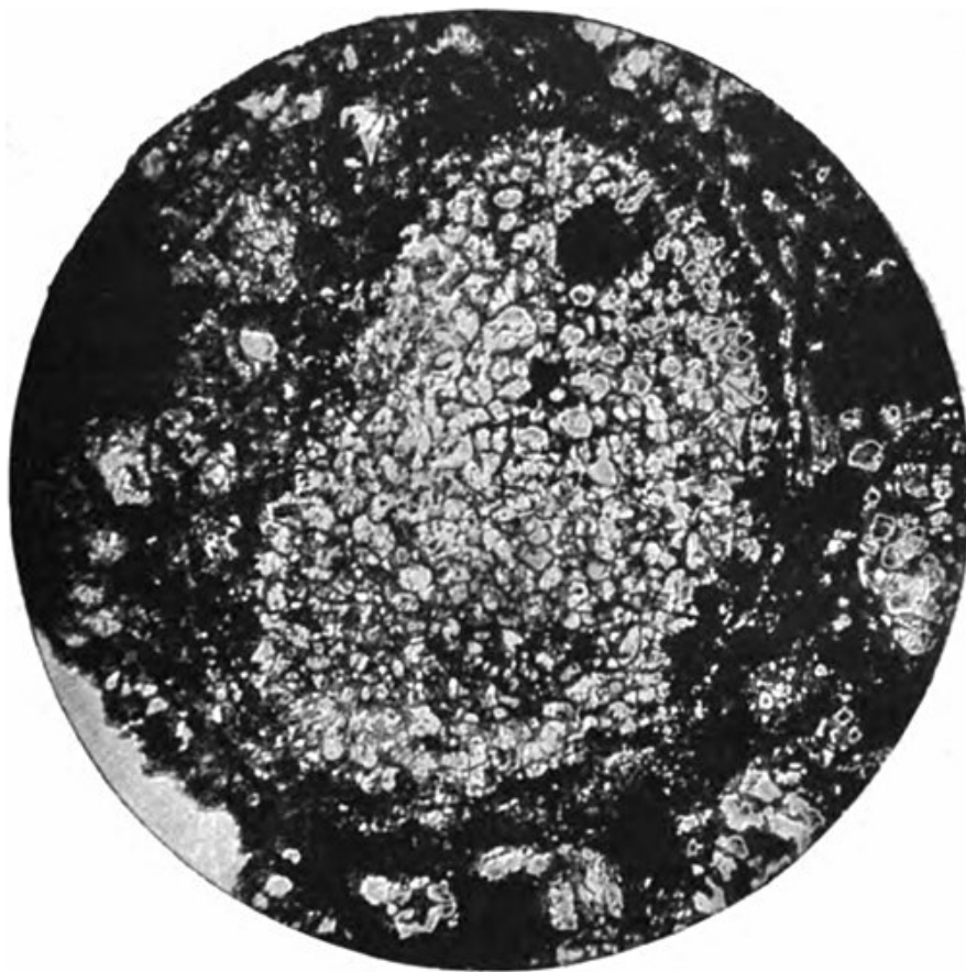
Fig. 37. — Chondrites granuleuses dans la pierre météorique de Sexes. Agrandissement 1 : 70 d'après G. Tschermak.
