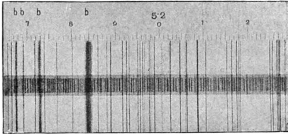
Fig. 25. — Spectre d'une tache solaire. En haut et en bas, spectre de la photosphère ; au milieu, celui de la tache, bordé de celui de la pénombre, aux bords de la tache (D'après Mitchell.)
