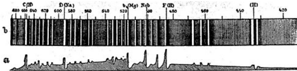
Fig. 45. — Spectre de l'étoile nouvelle du Cocher, en 1892.
