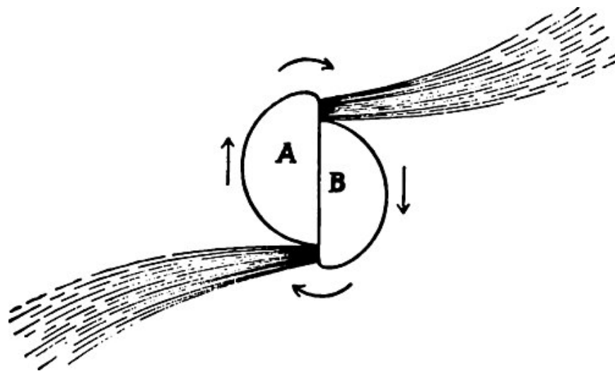
Fig. 46. — Figure schématique, indiquant les conséquences d'un choc entre deux soleils éteints A et B, qui cheminaient dans la direction des flèches. — Il en résulte une violente rotation dans le sens des flèches courbes. Deux puissants jets gazeux s'échappent par suite du dégagement de la décomposition des couches profondes contenant des combinaisons explosives, ramenées à la surface par le choc.
