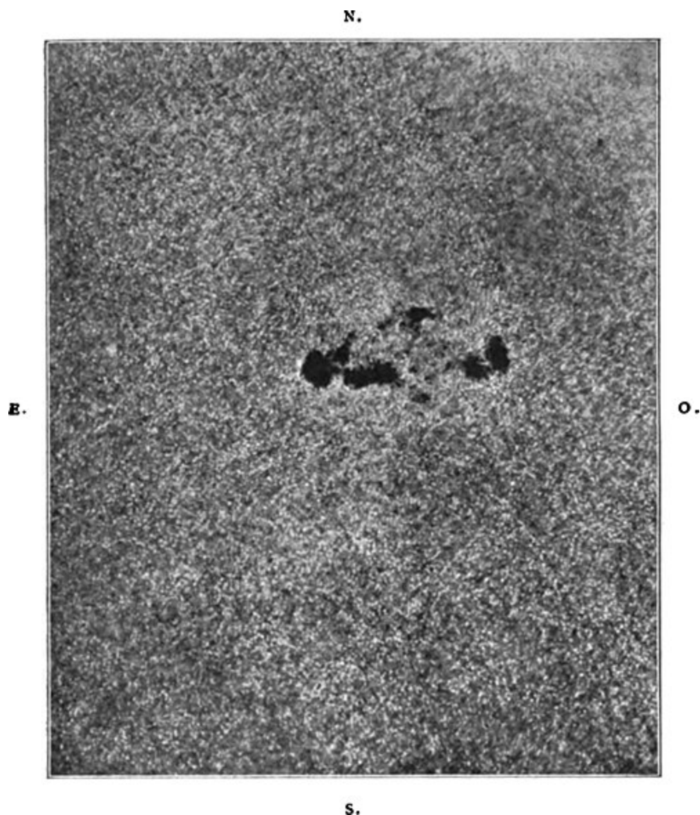
Fig. 18. — Groupe de taches solaires, et granulations. Cliché de l'observatoire de Meudon, du 1 er avril 1884.
