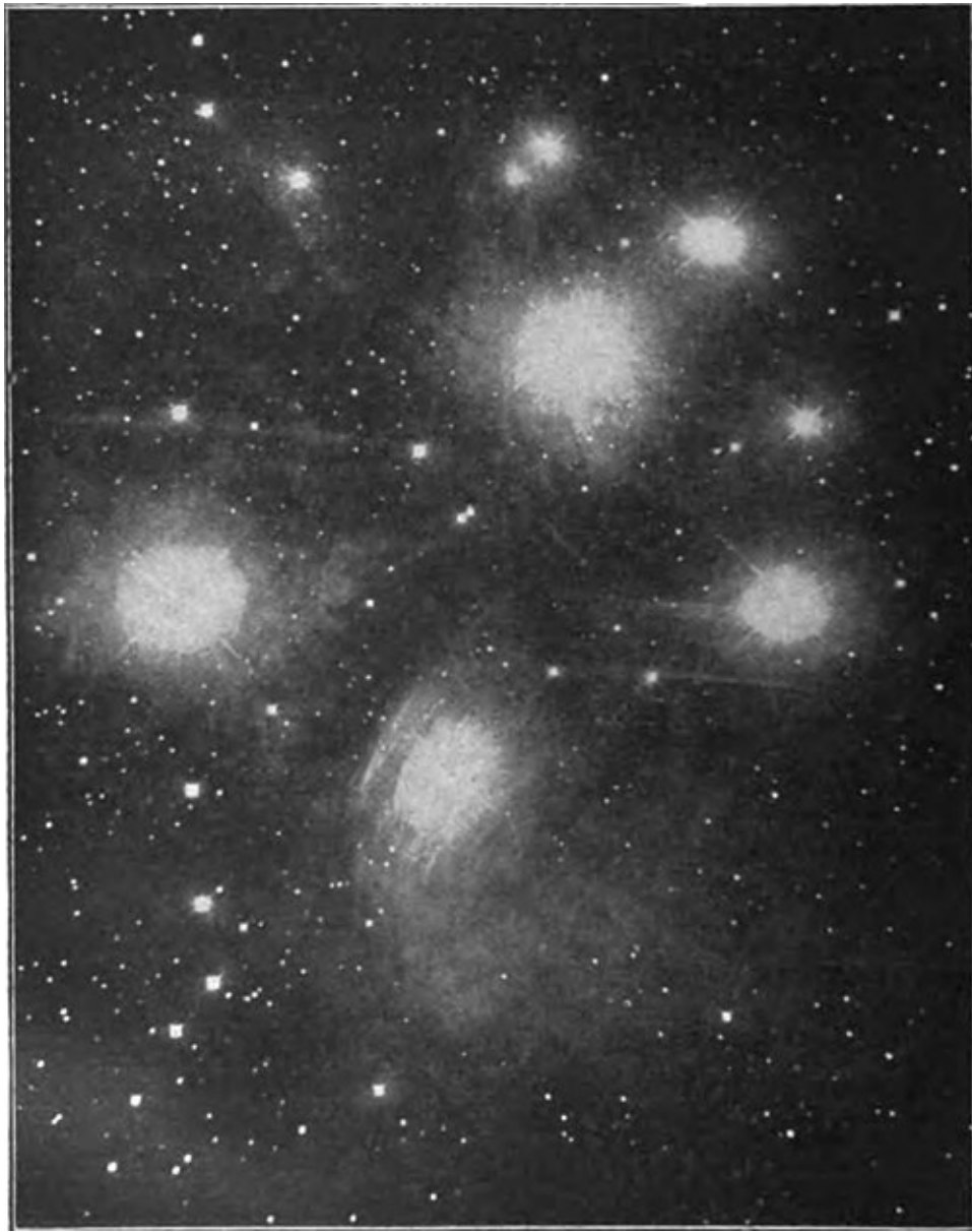
Fig. 52. — Bandes nébuleuses des étoiles des Pléiades. Photographie de l'observatoire de Yerkes du 19 octobre 1901. Un millimètre = 42,2 secondes d'arc.
