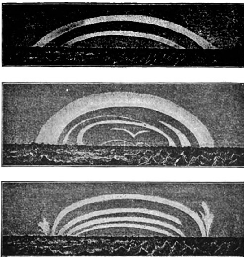
Fig. 38. — Aurores en forme d'arc, observées par Nordenskiöld, pendant l'hivernage de la Vega , près du détroit de Behring. 1879.
