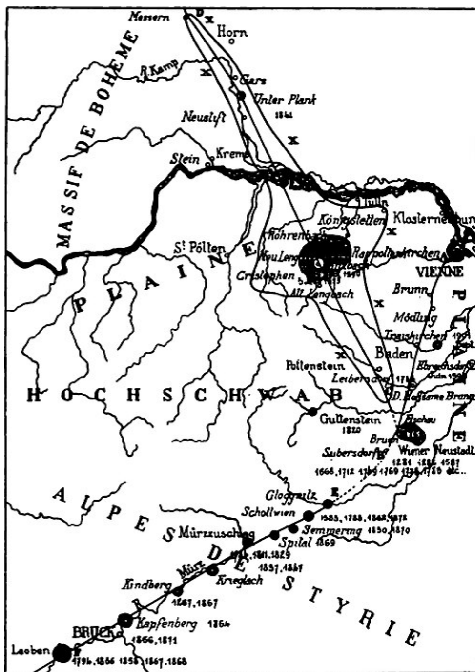
Fig. 13. — Lignes sismiques de la Basse-Autriche.
