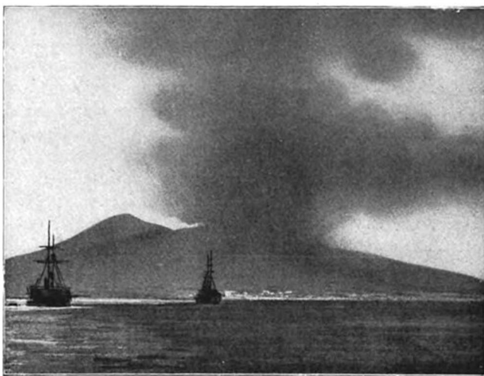
Fig. 4. — L'éruption du Vésuve de 1906, d'après une photographie. Les nuages sont constitués principalement par des cendres.
