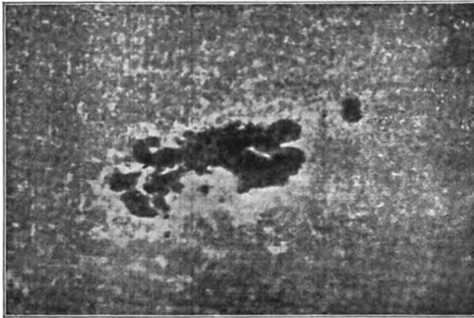
Fig. 27. — La grande tache du 9 octobre 1903. Photographie des parties inférieures des facules de calcium, obtenue à l'aide de la raie H (calcium) et au bord de cette ligne. La tache n'est pas recouverte par les facules, tout au moins pas dans la même étendue que dans les deux figures suivantes.
