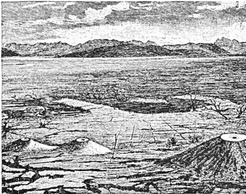
Fig. 12. — Cratères avec cônes de sable, et fentes, produites par le séisme de Corinthe en 1851. Des branches d'arbres émergent de l'eau d'inondation.
