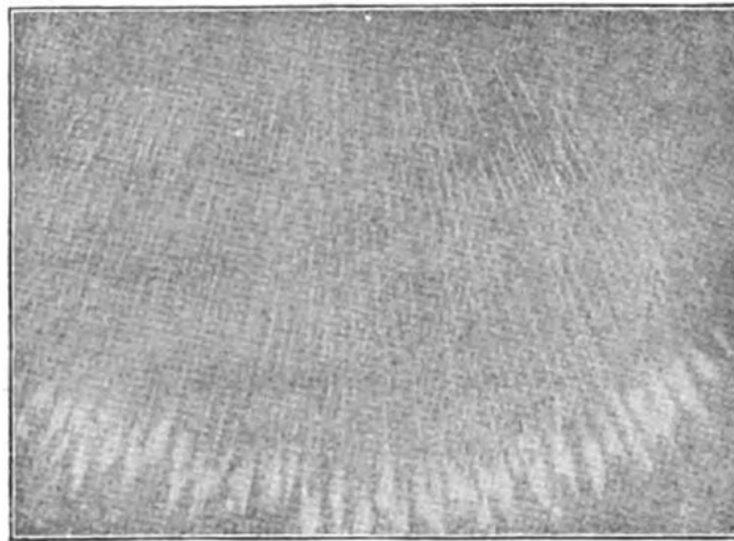
Fig. 39. — Aurore de forme rayonnante.
