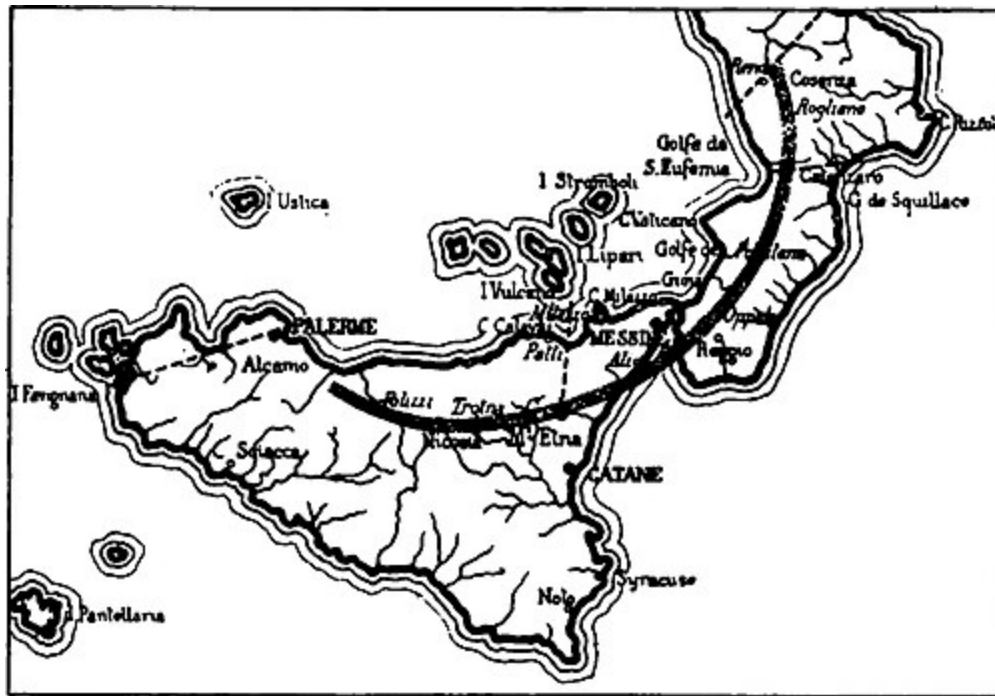
Fig. 15. — Lignes des séismes dans la région d'affaissement Tyrrhénienne.
