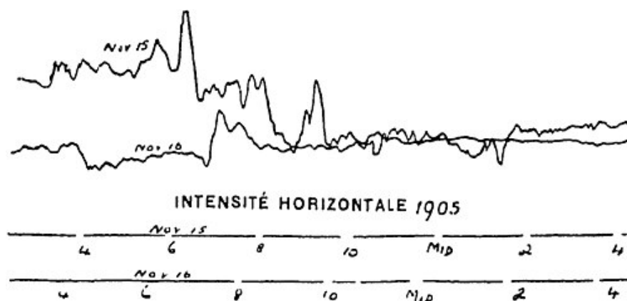
Fig. 43. — Marche de l'intensité horizontale les 15 et 16 novembre 1905, à Kew. Le 15 novembre une aurore boréale extraordinairement brillante fut observée en Galicie, Allemagne, France, Norvège, Angleterre et Irlande aussi bien qu'en Nouvelle-Écosse (Canada occidental). Son maximum eut lieu vers 9 heures du soir. Déjà vers 6 heures elle se montra exceptionnellement brillante.
