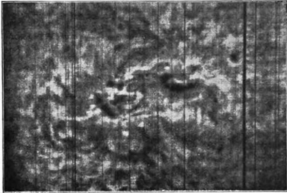
Fig. 29. — La grande tache du 9 octobre 1903. Photographie des facules d'hydrogène, faite à l'aide de la raie F de l'hydrogène. Les parties les plus accentuées de la tache sont seules visibles, les autres sont recouvertes et occultées par les masses d'hydrogène, qui montrent une violente agitation.
