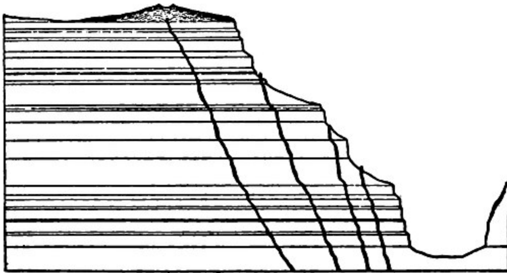
Fig. 8. — Figure schématique d'un terrain avec fissures remplies de lave, surmonté d'un cône de cendres volcaniques dans le Torowheap Cañon, sur le plateau du Colorado.
