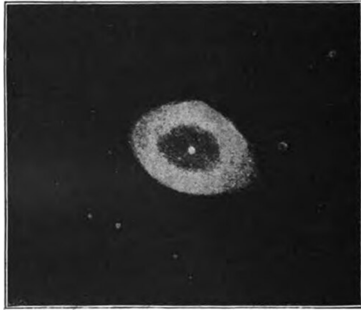
Fig. 50. — Nébuluse annulaire de la Lyre. Photographie de l'observatoire de Yerkes.
