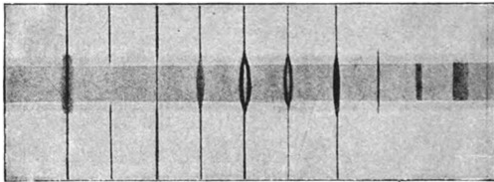
Fig. 24. — Figure schématique, montrant la différence entre le spectre d'une tache et celui de la photosphère. Certaines lignes se trouvent agrandies dans la tache, d'autres sont affaiblies. Au milieu, deux « inversions », à droite, deux « bandes ». (D'après Mitchell.)
