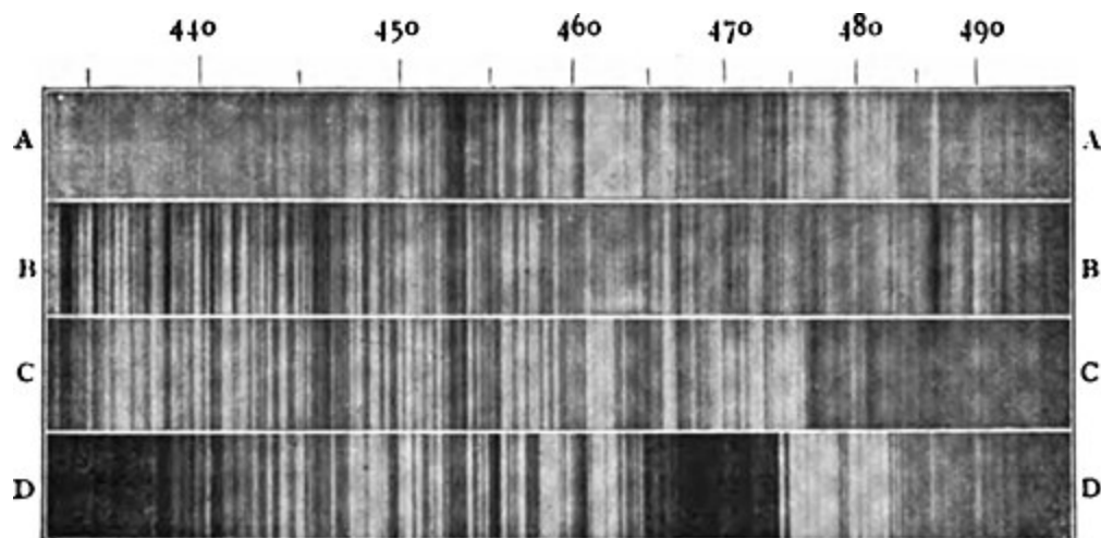
Fig. 59. — Spectres comparés d'étoiles de la 2 e , 3 e et 4 e catégorie. Photographie de l'observatoire de Yerkes. Partie bleue du spectre.
