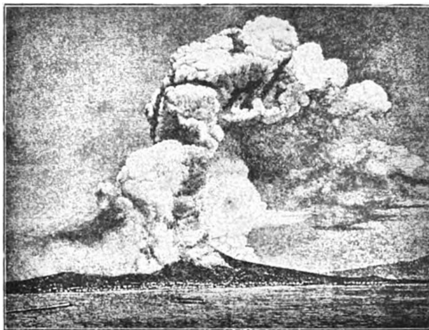
Fig. 3. — L'éruption de 1872, d'après une photographie.
