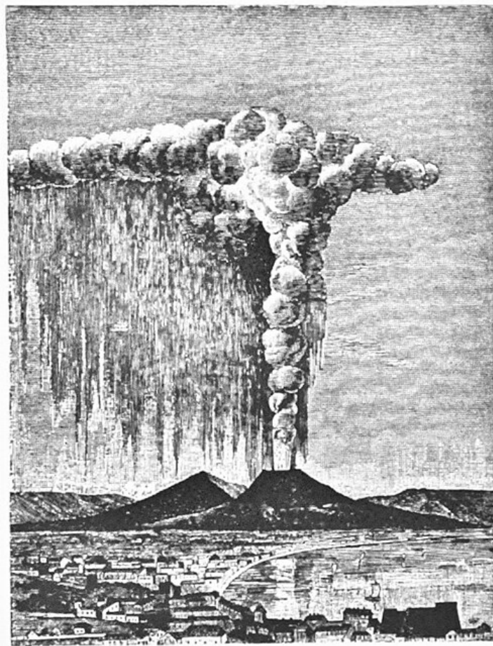
Fig. 2. — L'éruption du Vésuve de 1822, d'après un dessin fait sur place par Poulett-Scrope.
