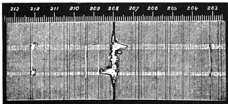
Fig. 19. — Partie du spectre solaire, du 3 janvier 1875, d'après Langley. Les deux lignes claires horizontales sont données par des protubérances. Au centre, la ligne de l'hydrogène F, très déformée par suite d'énormes mouvements gazeux.
