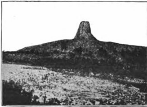
Fig. 7. — Mato Tepee, dans le Wyoming. Un type de neck volcanique.
