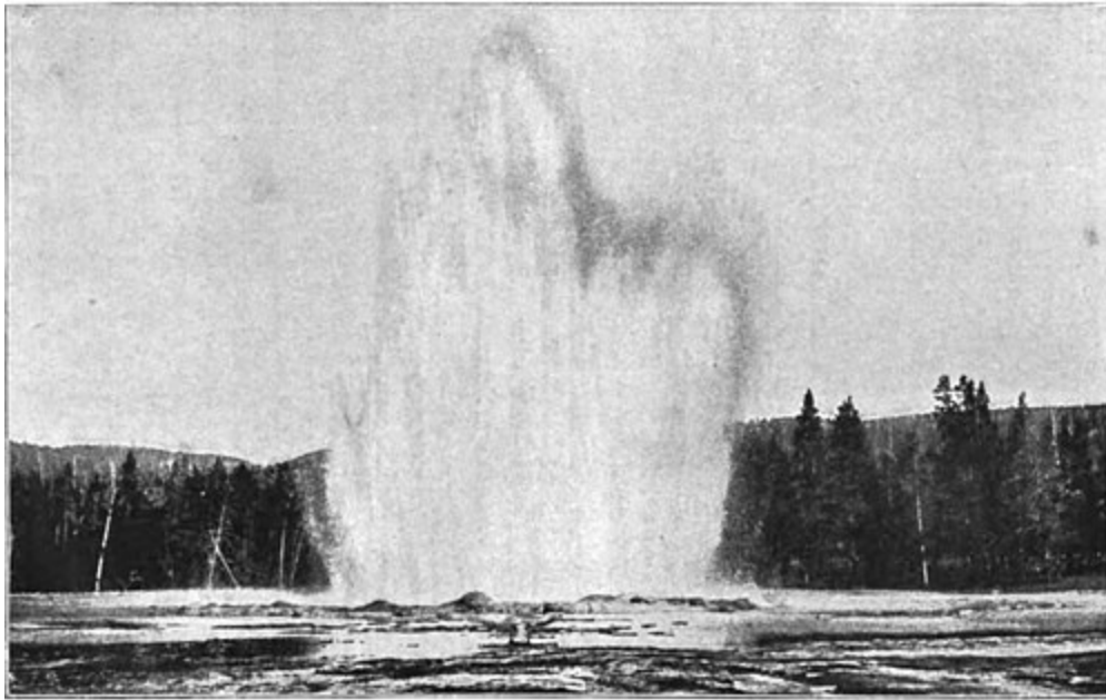
Fig 6. — Le geyser « Excelsior », dans le Yellowstone-Park, Wyoming. Reliquat d'une puissante action volcanique pendant l'époque tertiaire.
