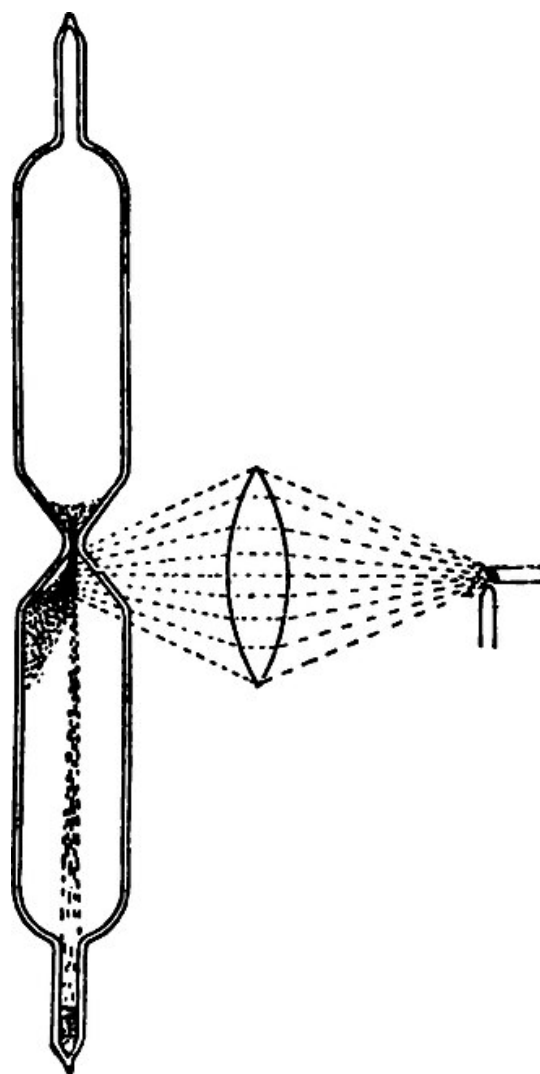
Fig. 36. — Expérience de Nichols et Hull, pour la reproduction des effets des queues de comète. La lumière d'une lampe à arc est projetée à travers une loupe, sur de fines poussières tombant d'un orifice.
