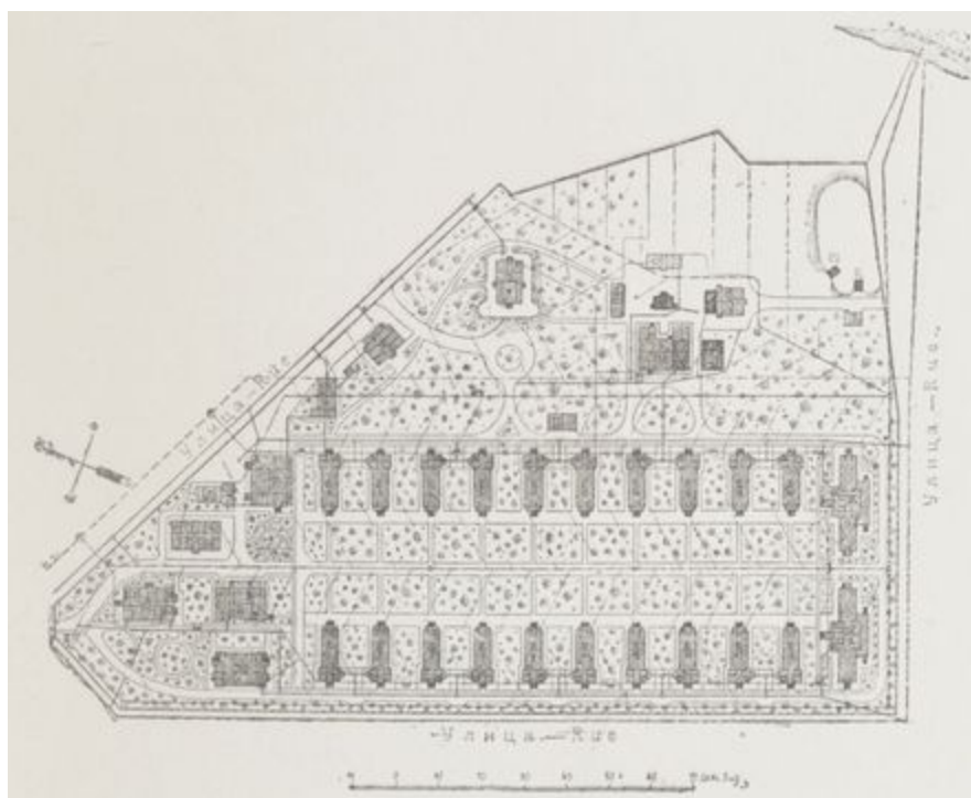
Fig. 25. Plan de l'hôpital Alexandre.
