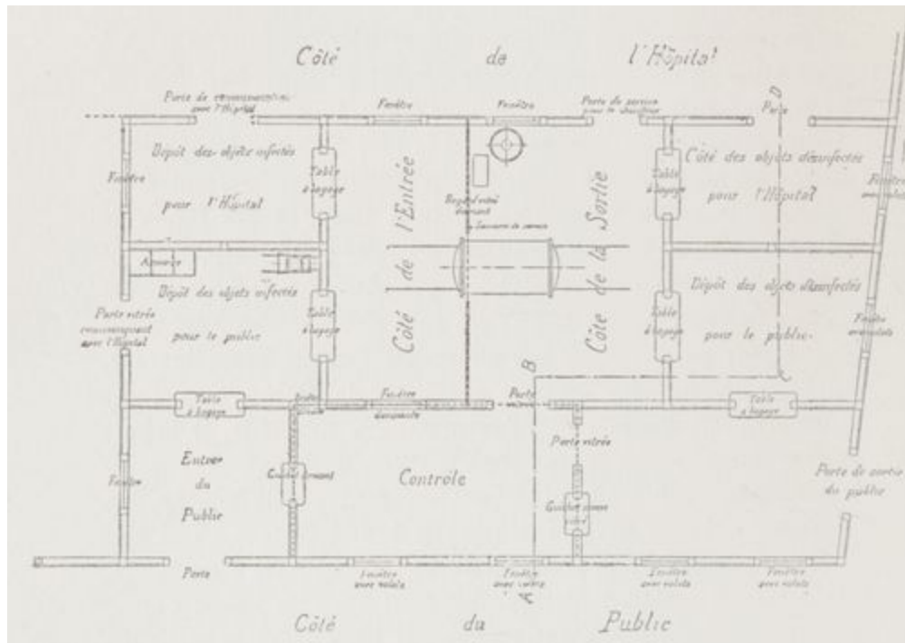
Fig. 24. — Plan d'un pavillon de désinfection.
