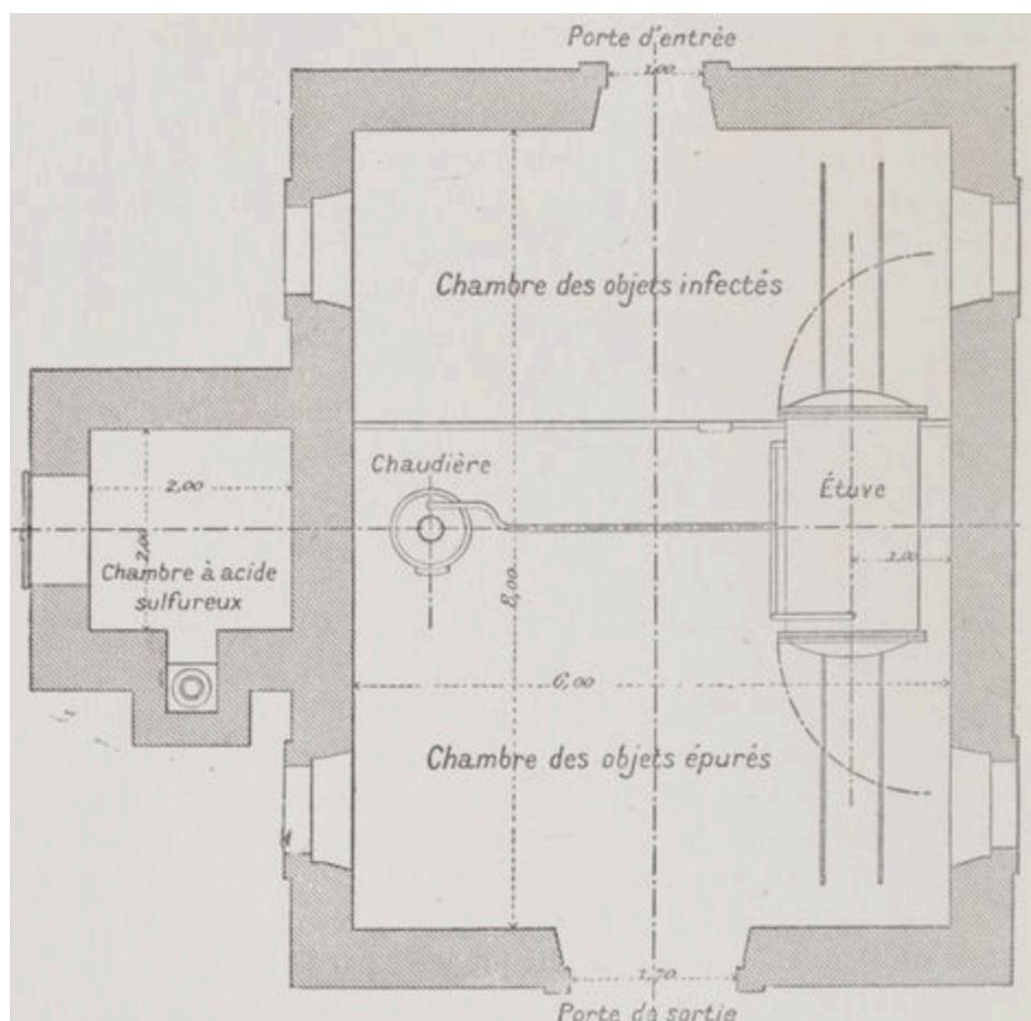
Fig. 23. — Plan d'un bâtiment à désinfection.
