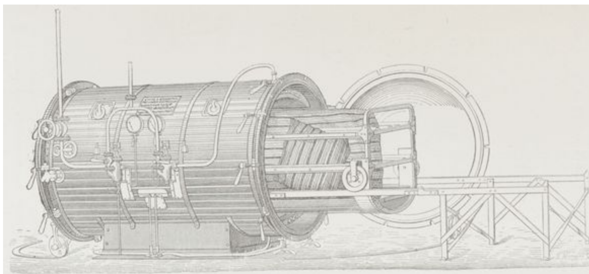
Fig. 20. — Etuve fixe à désinfection (modèle Geneste et Herscher).
