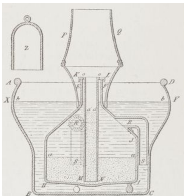
Fig. 16. — Brûleur de sulfure de carbone.
