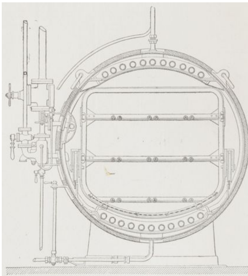
Fig. 21. — Coupe de l'étuve à désinfection.
