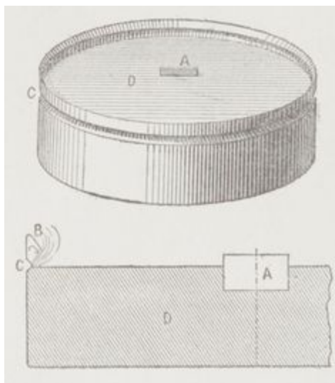
Fig. 18. — Brûleur de soufre de Deschiens.
