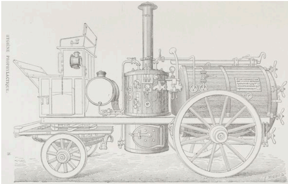
Fig. 22. — Etuve mobile à désinfection (modèle Geneste et Herscher).
