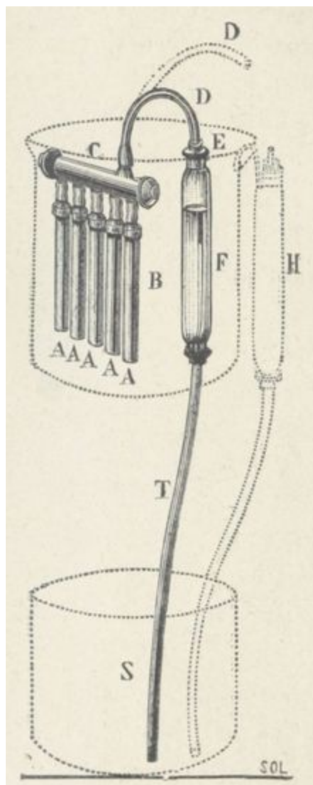
FIG. 2. — Filtre de Chamberland,
