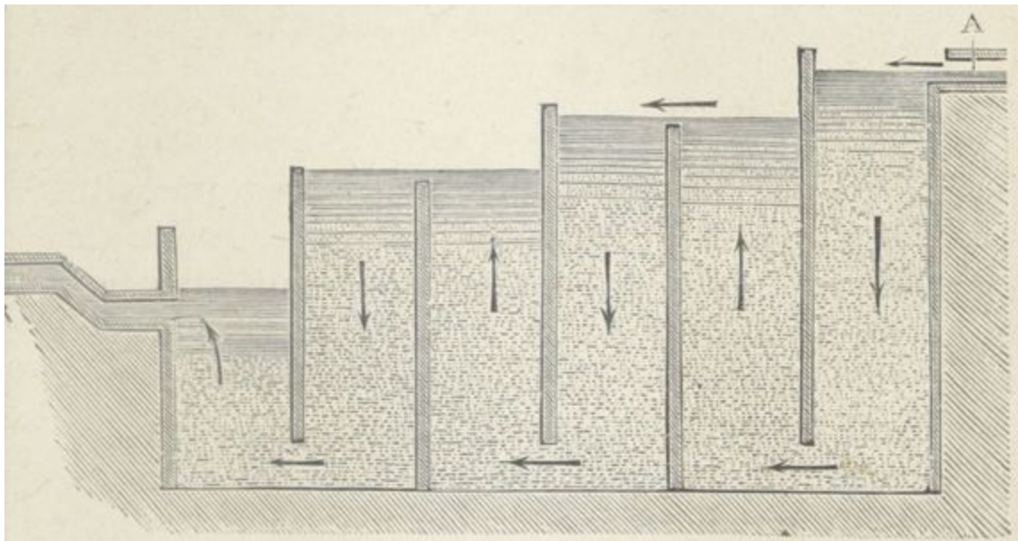
FIG. 1. — Bassin filtrant de M. Charles Garnier. A, conduite d'amenée. — R, conduite de distribution.
