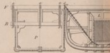
Coupe transversale de l'appareil au milieu
