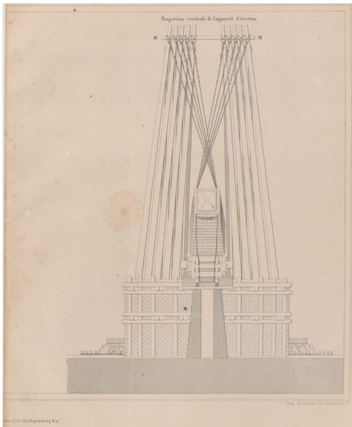
L'Obélisque de Luxor PROJECTION VERTICALE DE L'APPAREIL D'ÉRECTION, PI : XII.
