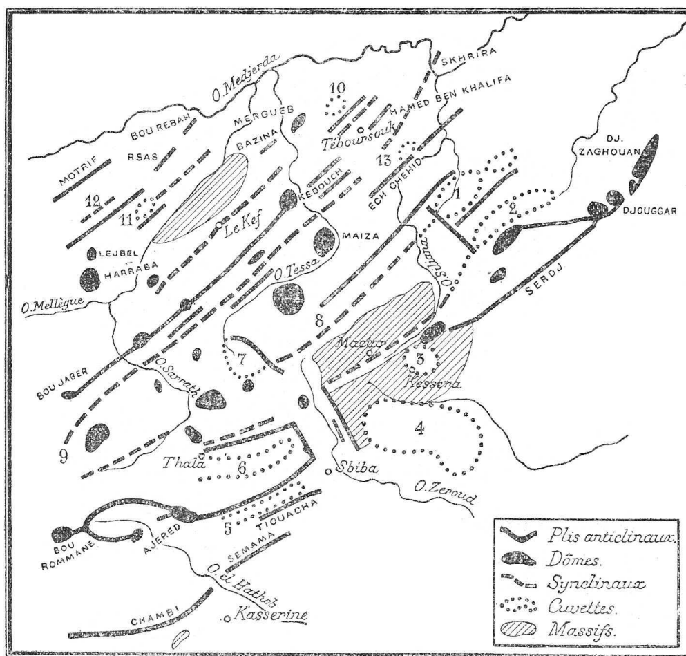
Carte 3. — CARTE OROTECTONIQUE SCHÉMATIQUE DU HAUT TELL
