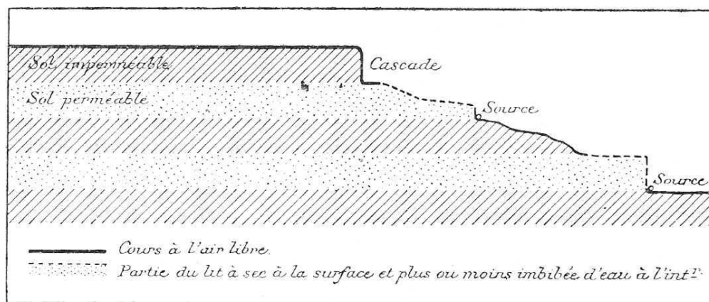
Figure 4. — HYDROLOGIE — LE RÉGIME A ÉCLIPSES
