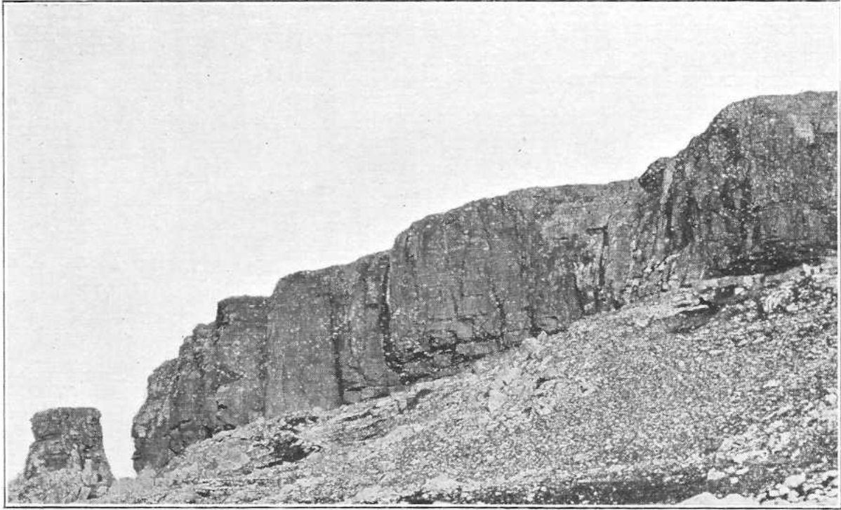
IV — FALAISE DE LA KALAAT SENANE VUE PRISE DU SUD-EST. (Cliché Olivier.)
