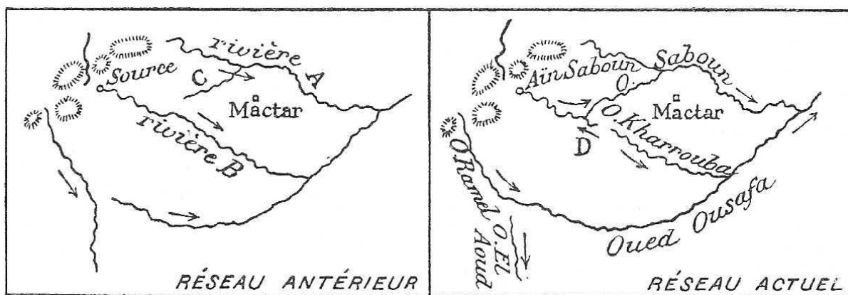
Carte 8. — CAPTURE D'OUEDS SUR LE HAUT OUSAFA
