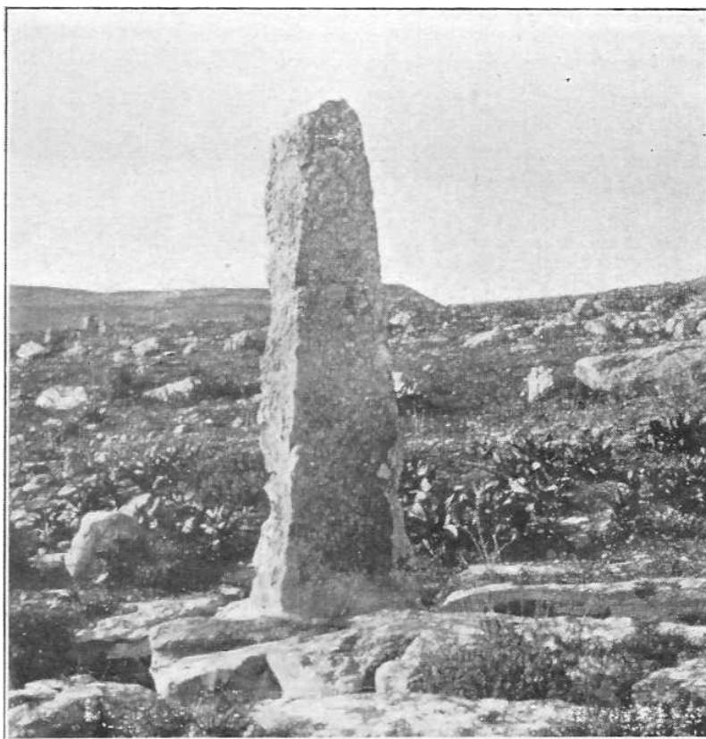
XVI — MENHIR AVEC INSCRIPTION LIBYQUE A MÉDOUDJA. (Cliché Monchicourt.)
