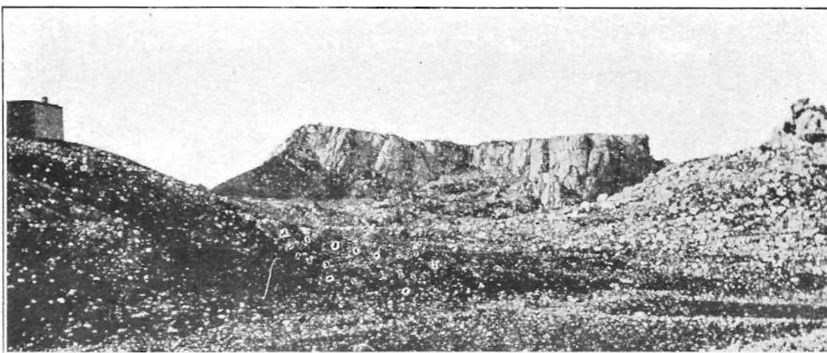
VI — LE DYR DU KEF, VUE PRISE DE LA DIRECTION DE NEBEUR. (Cliché Olivier.)
