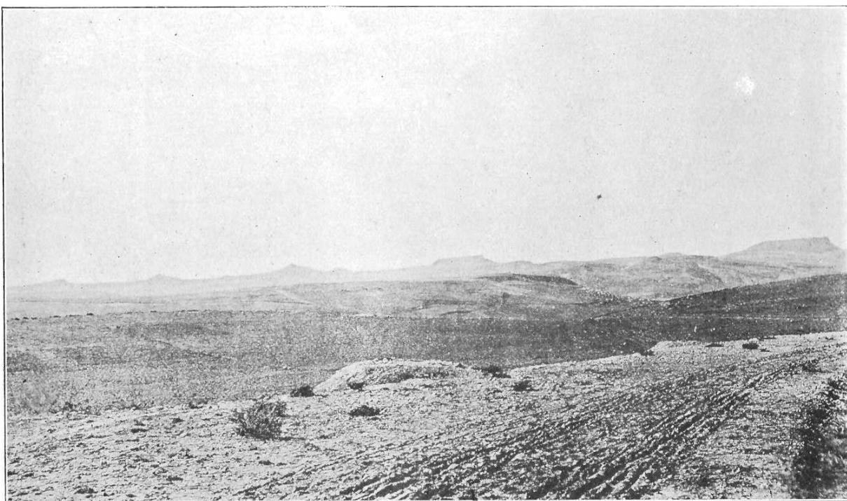
VIII — LA CHAÎNE DES KALAATS (PARTIE OCCIDENTALE) : DU KEF BDIRI A L'OUEST A LA KALAAT EL-HARAT A L'EST (HAMADAT DES OULED-AYAR). (Cliché Monchicourt.)
