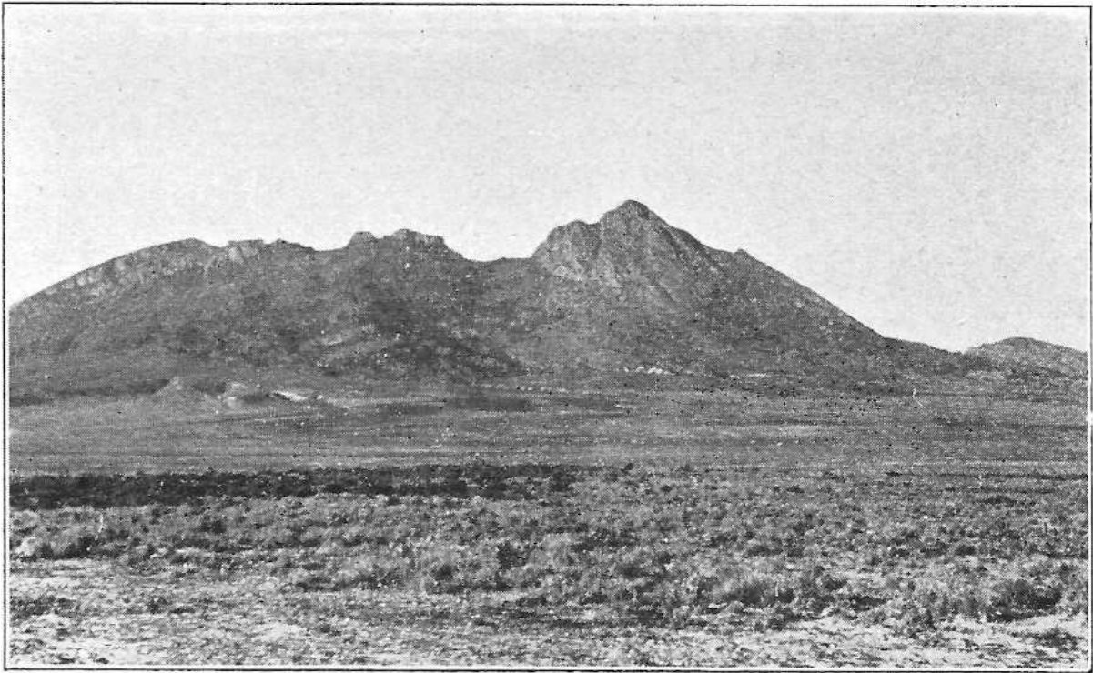
I — LE DJEBEL SLATA VU DU SUD-EST. (Cliché Olivier.)
