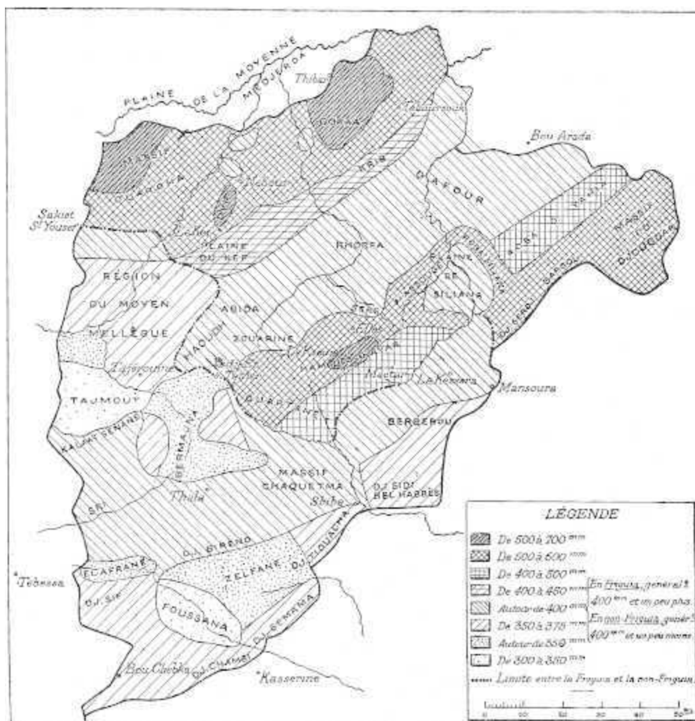
Carte 5. — ESSAI DE CARTE DE LA DISTRIBUTION DES PLUIES DANS LE HAUT-TELL
