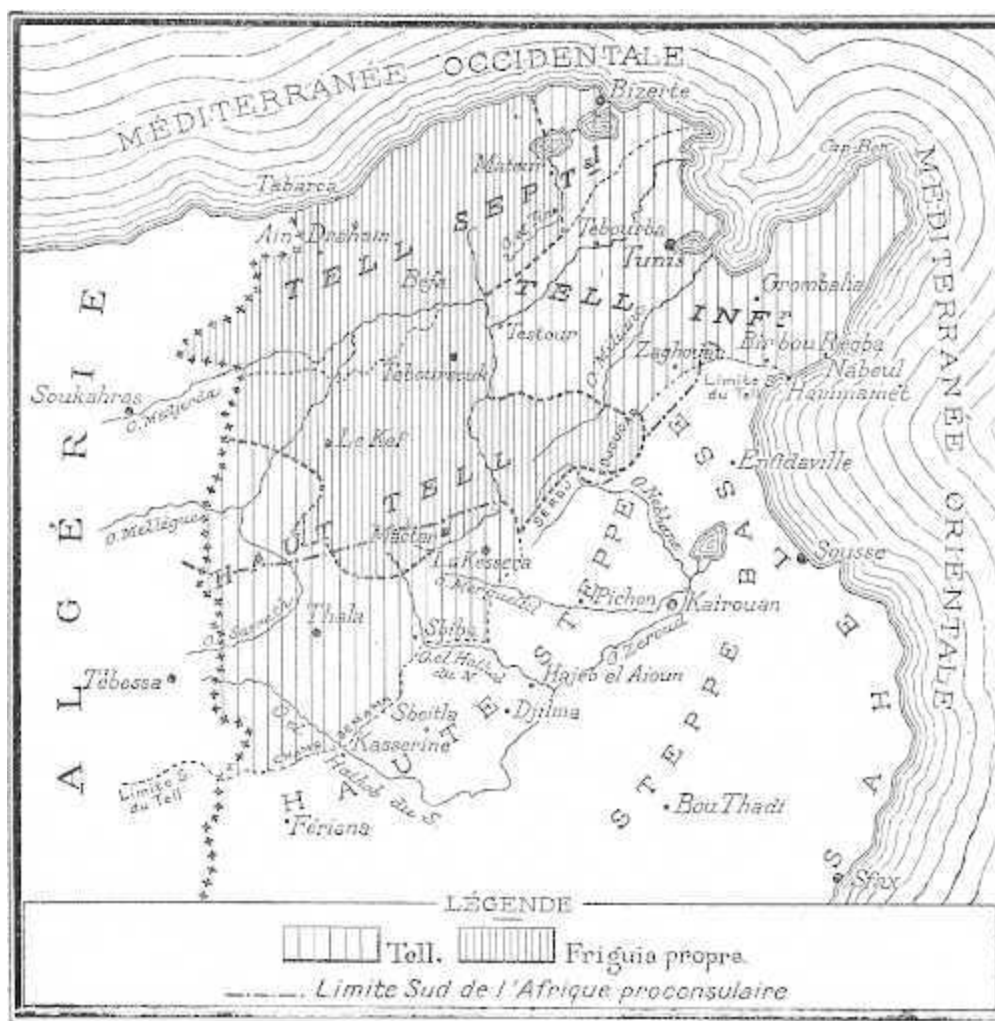
Carte 1. — LES GRANDES DIVISIONS NATURELLES DE LA TUNISIE
