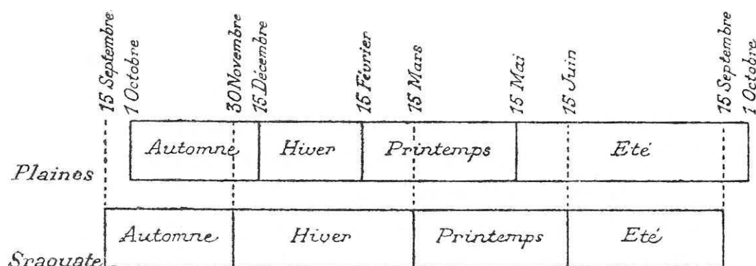
Figure 3. — RÉPARTITION DES SAISONS DANS LES PLAINES ET SUR LES SRAOUATE
