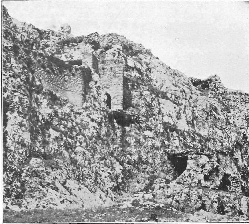
XIX — L'ESCALIER DE LA KALAAT SENANE. (Cliché Monchicourt)
