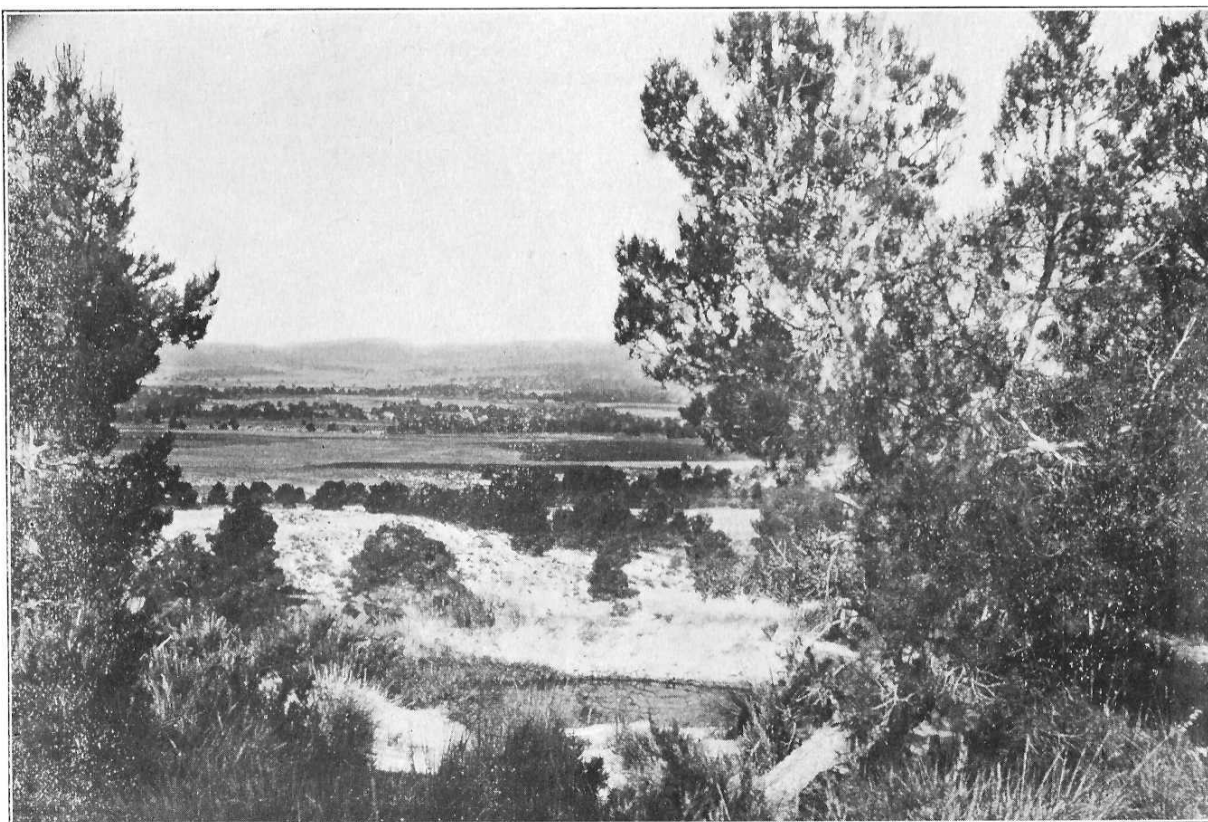
IX — LE TELL DES FRÉCHICH — LE PAYS AU NORD DE L'AÏN MIDOUN. (Cliché Monchicourt.)
