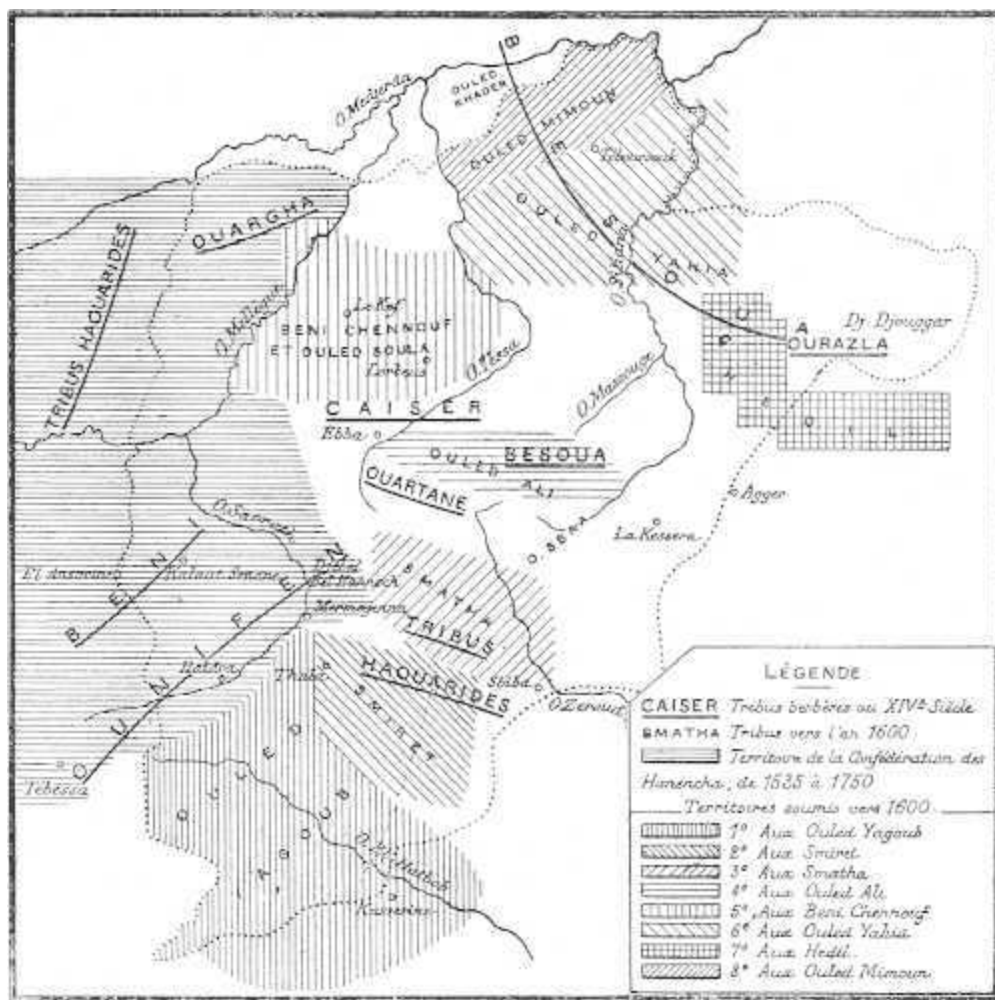
Carte n° 10. — LES TRIBUS DU HAUT-TELL A L'ÉPOQUE ARABE ET TURQUE
