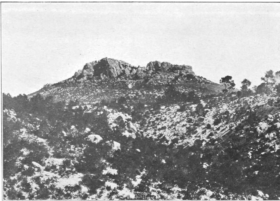
XII — LA KALAAT FRARHA (CHAQUETMA) ET LA FORÊT SOUS-JACENTE. PINS SUR ROMARIN ET GENÊTS. (Cliché Monchicourt.)
