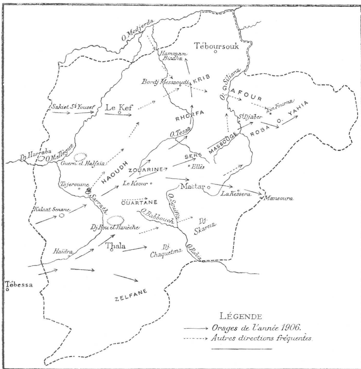
Carte 6. — CARTE DE LA DIRECTION DES ORAGES DE GRÊLE
