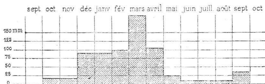
Figure 2. — PLUIE — DIVERS TYPES D'ANNÉES A MACTAR. Type A
