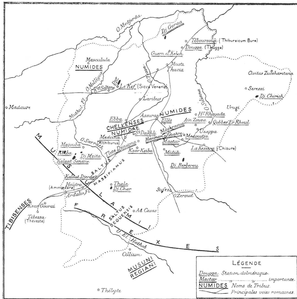
Carte n° 9. — LE HAUT-TELL DANS L'ANTIQUITÉ
