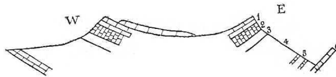
Figure 1. — DISTRIBUTION DES TERRAINS AU DJEBEL MEIDA DES OUARGHA (communiqué par ABADIE)
