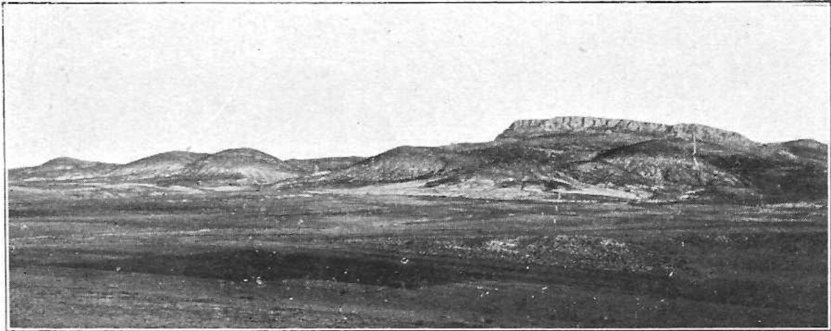
VII — CONTRASTE DE L'ÉOCÈNE INFÉRIEUR DU KEF BERDA (BORD OUEST DU HAODH) ET DU SÉNONIEN SOUS-JACENT. (Cliché Olivier.)
