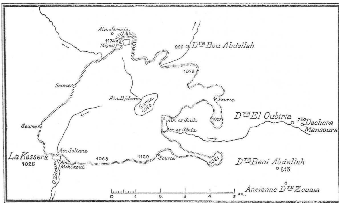
Carte 7. — LA HAMADAT DE LA KESSERA
