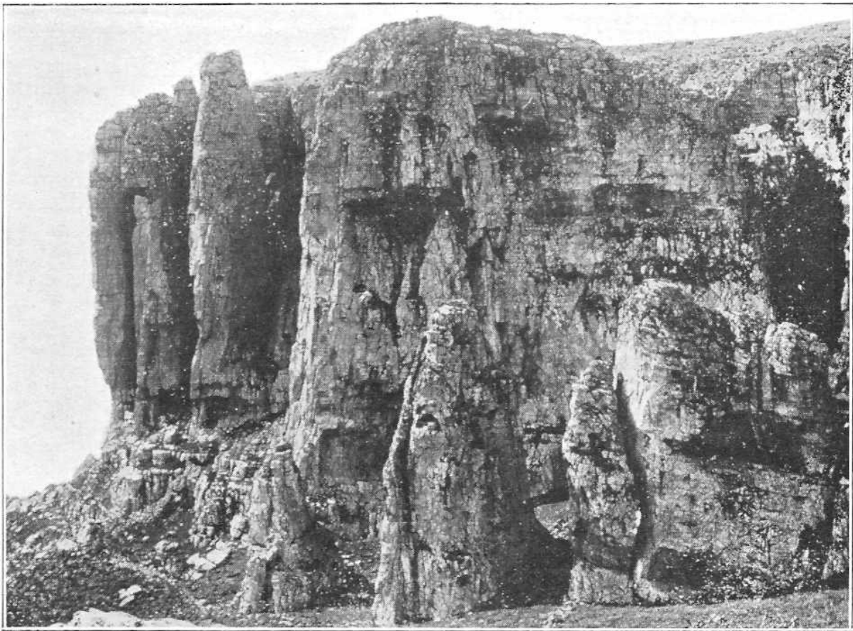
III — FALAISE DE LA KALAAT SENANE. LES FAHOUL DE L'ANGLE NORD-EST. (Cliché Monchicourt.)
