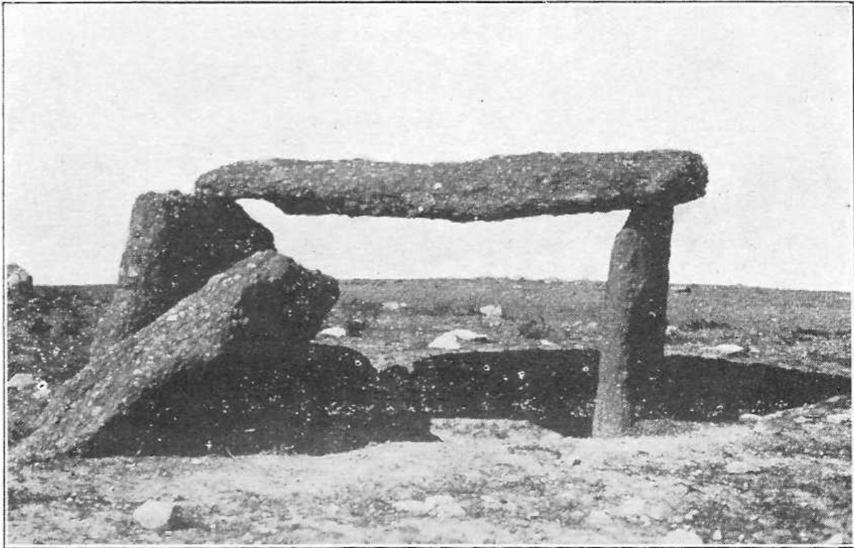
XVII — DOLMEN EN CONGLOMÉRAT DE LUMACHELLES DE L'ÉOCÈNE MOYEN (MACTAR). (Cliché Monchicourt.)
