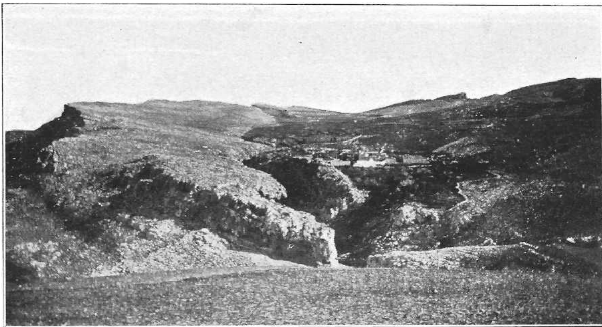
V — LE SYNCLINAL DU DYR DU KEF ET LA ZAOUIA DE SIDI MANSOUR EL GAIAS VUS EN PLAN. (Cliché Olivier)
