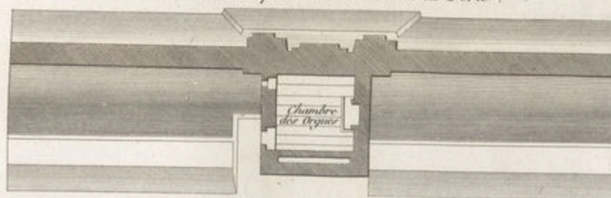
Élévation Intérieure de la Porte. Fig. 6
