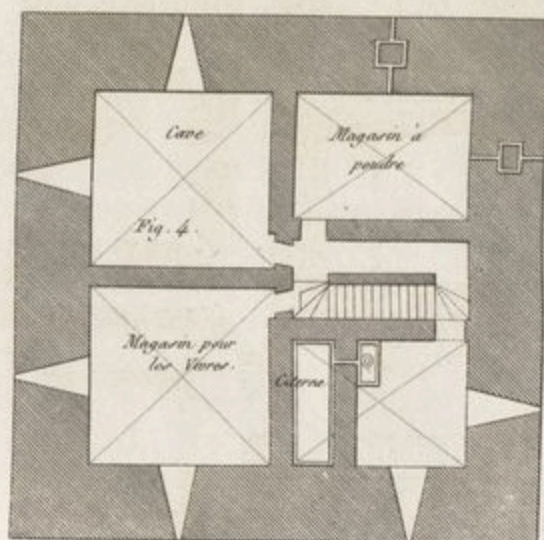
Parce de la Redoute.
