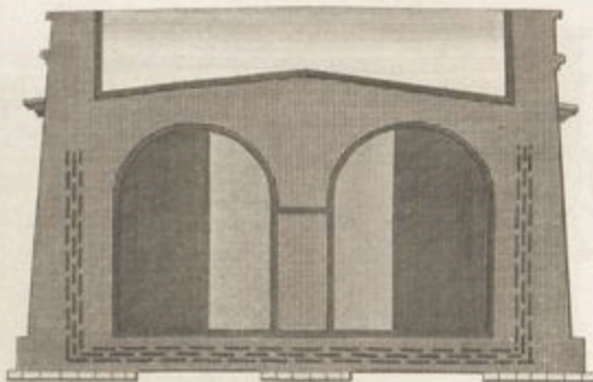
Echelle des dessins qui représentent des Four.
