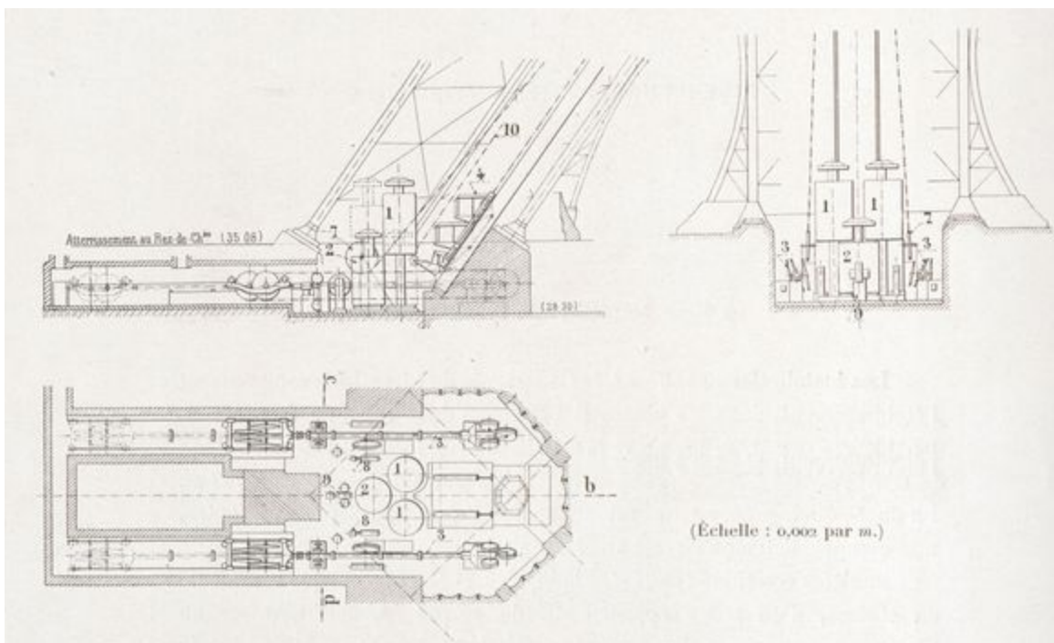
Fig. 5. — Ensemble des appareils placés dans le sous-sol du pilier. (Échelle : 0,002 par m.)
