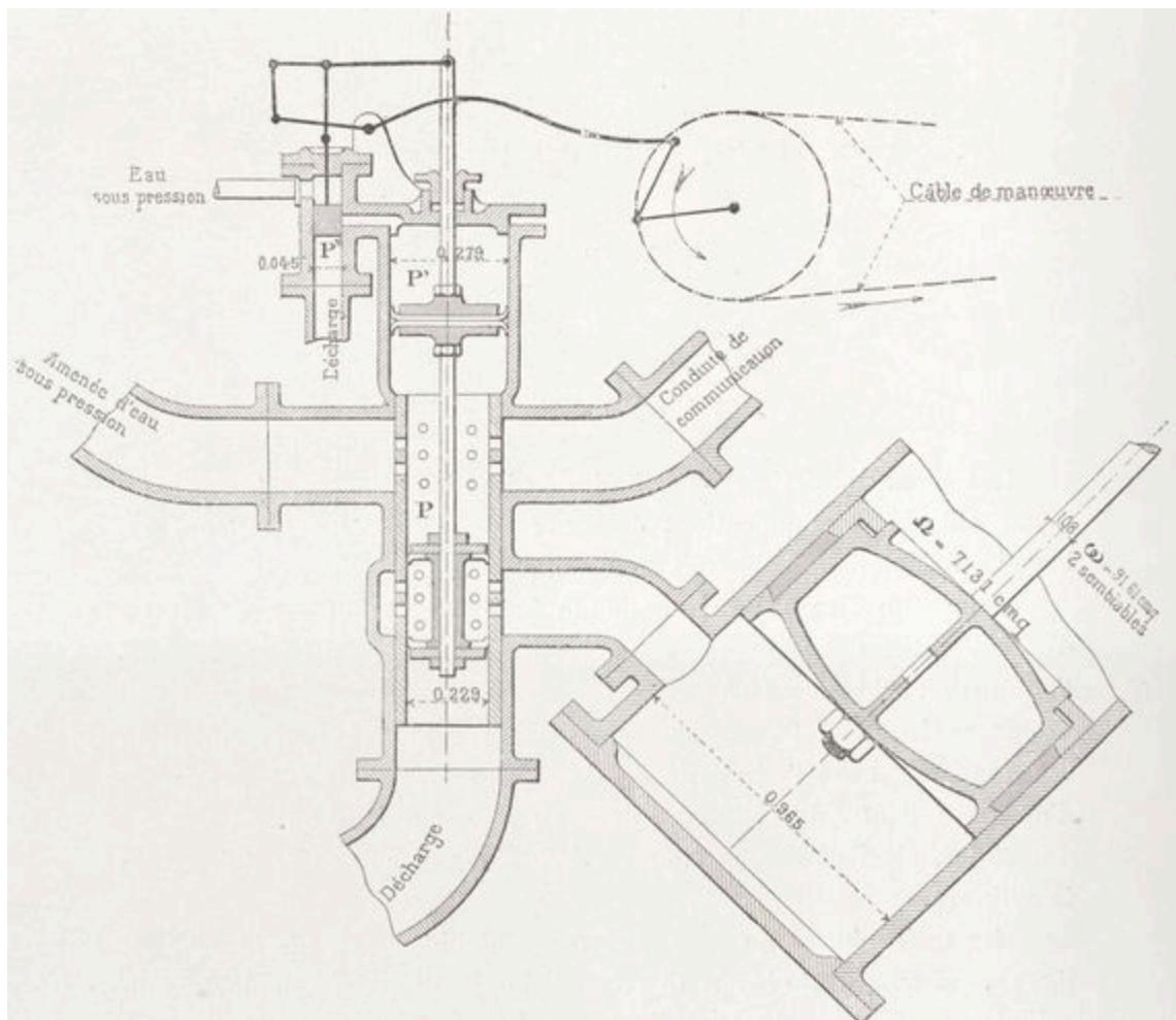
Fig. 52. — Schéma du distributeur. (Position de l'arrêt.)
