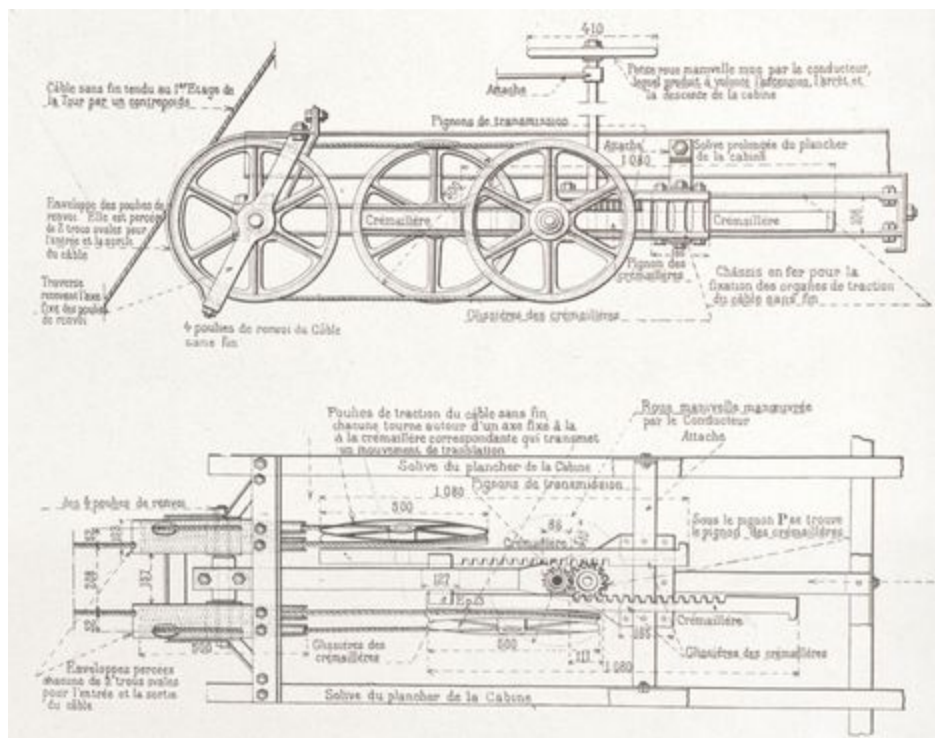
Fig. 61. — Élévation et plan de l'appareil de manœuvre.
