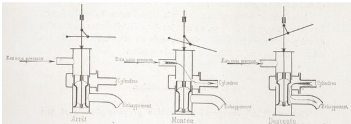
Fig. 25 . — Schémas des positions du distributeur.
