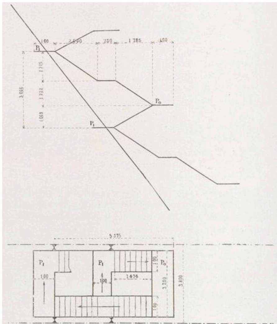
Fig. 30 — Schéma d'une révolution entre le sol et le 1er étage. (Échelle : 1/100.)
