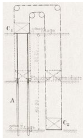
Fig. 4. — Schéma de l'ascenseur Edoux.
