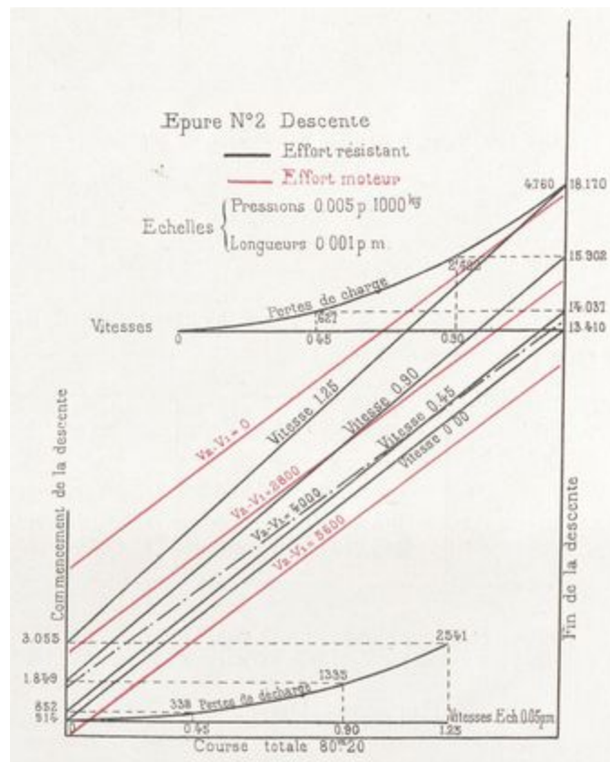
Fig. 66. — Épure de la descente.
