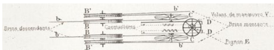
Fig. 60. — Vue en plan de l'appareil de manœuvre du véhicule.
