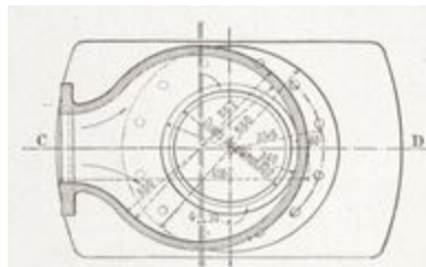
Fig. 20. — Coupe horizontale de la tête du cylindre par l'axe de la tubulure.
