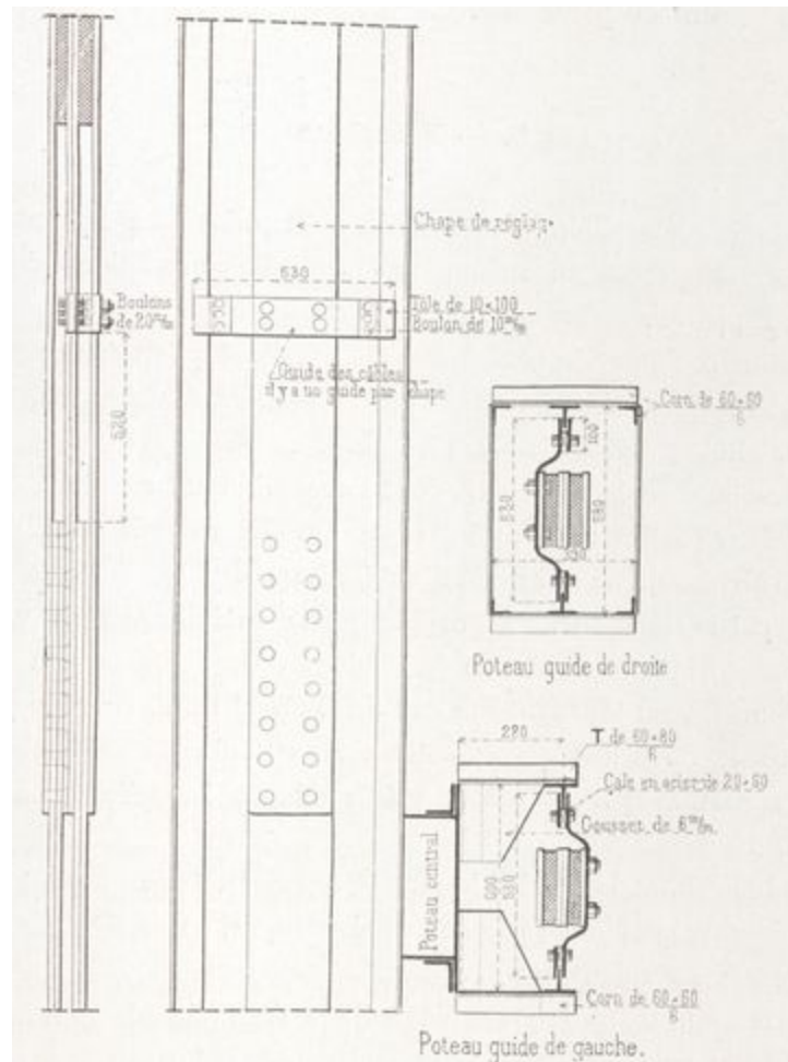
Fig. 28. — Poteaux-guides des câbles du côté de la cabine B entre l'étage intermédiaire et le sommet.
