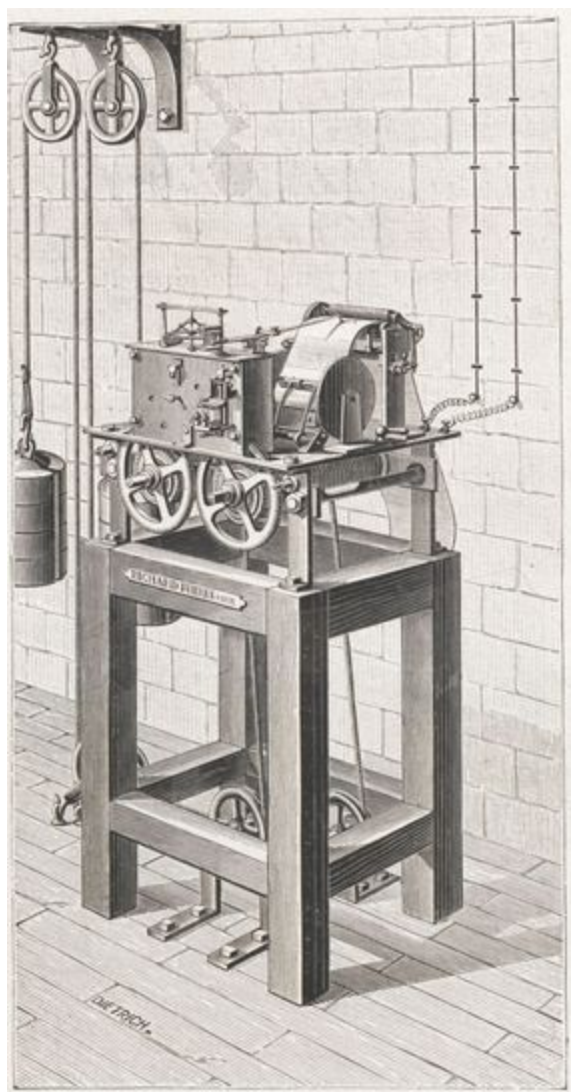
Fig. 50 ter. — Anémo-Cinémographe à indications instantanées.
