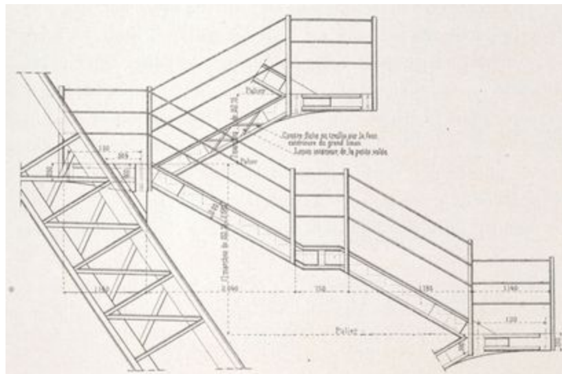
Fig. 31. — Détail d'une travée de l'escalier du pilier Sud.
