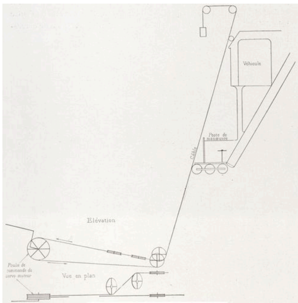
Fig. 59. — Schéma du câble de manœuvre.
