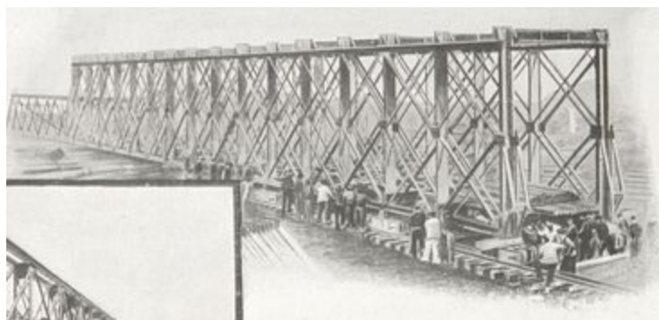
FIG. 89. — PONTS DÉMONTABLES POUR VOIES FERRÉES.
