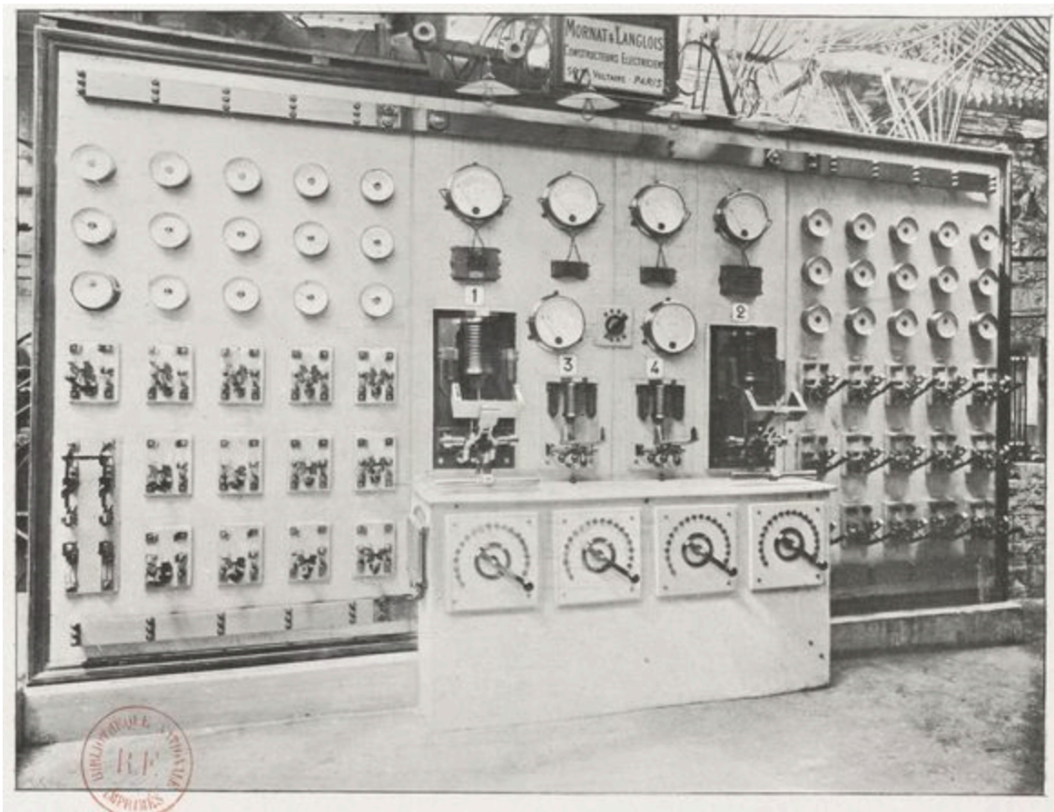
Fig. 33. — Vue générale du tableau de distribution électrique.
