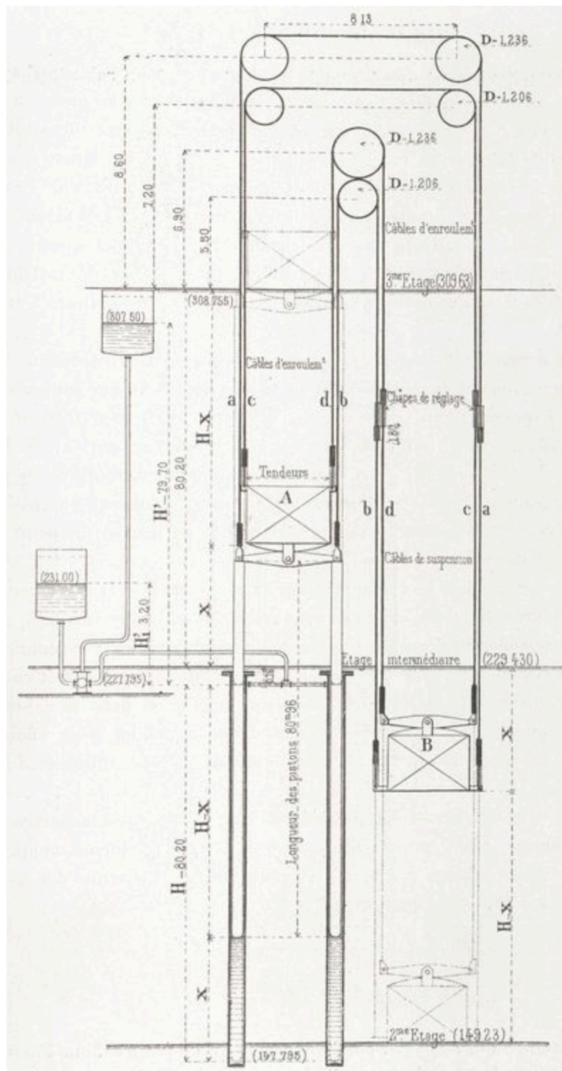
Fig. 18. — Ensemble schématique de l'ascenseur un Edoux.
