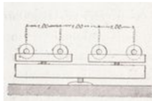
FIG. 69. — CHASSIS DE LANÇAGE A BASCULE A 4 GALETS.
