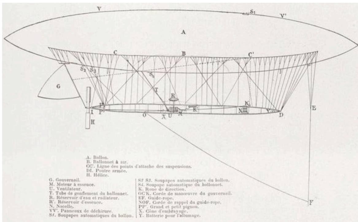
Dessin schématique du Santos-Dumont n° 6. (Échelle de 1/185 e .)
