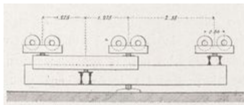
FIG. 70. — CHASSIS DE LANÇAGE A BASCULE A 6 PAIRES DE GALETS
