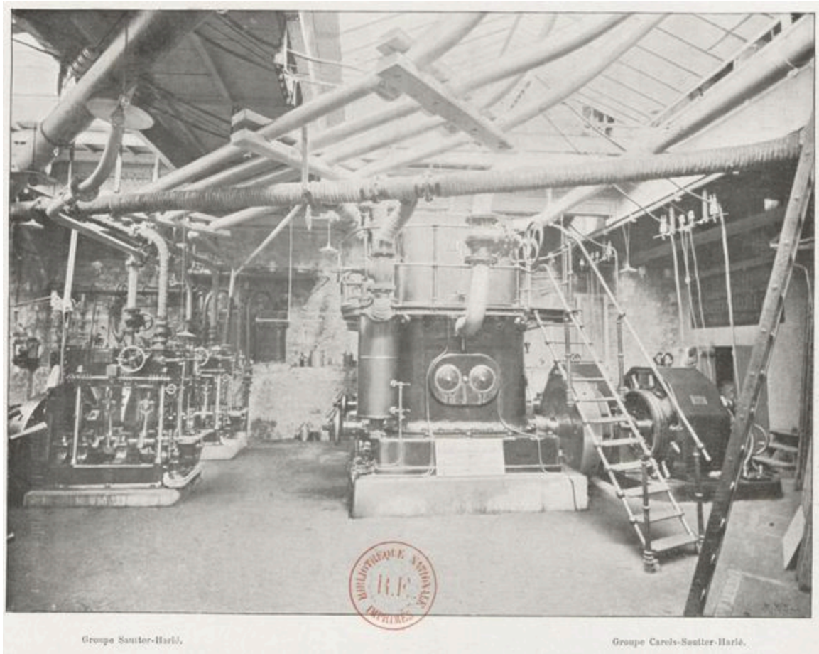
Fig. 32. — Vue des groupes électrogènes.
