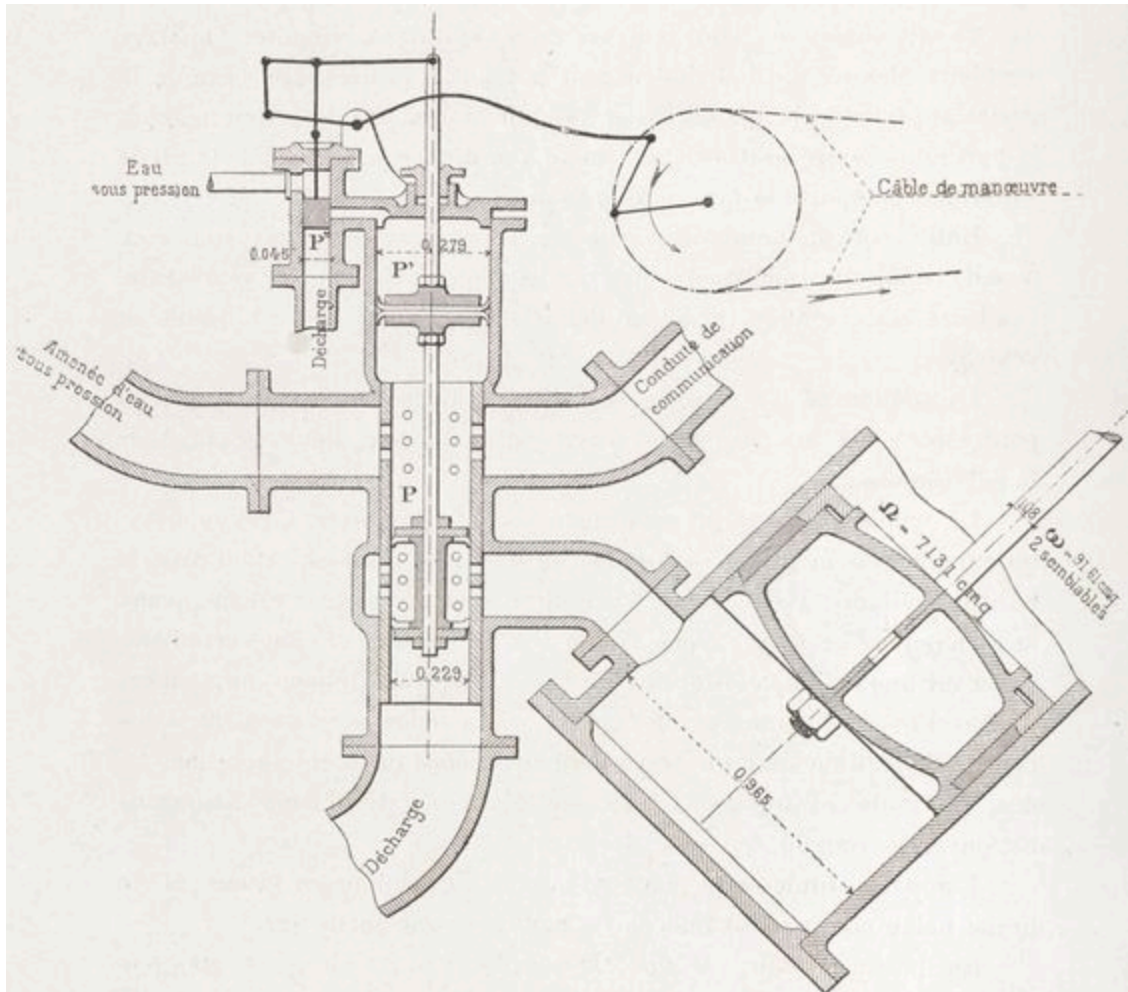
Fig. 13. — Schéma du distributeur.
