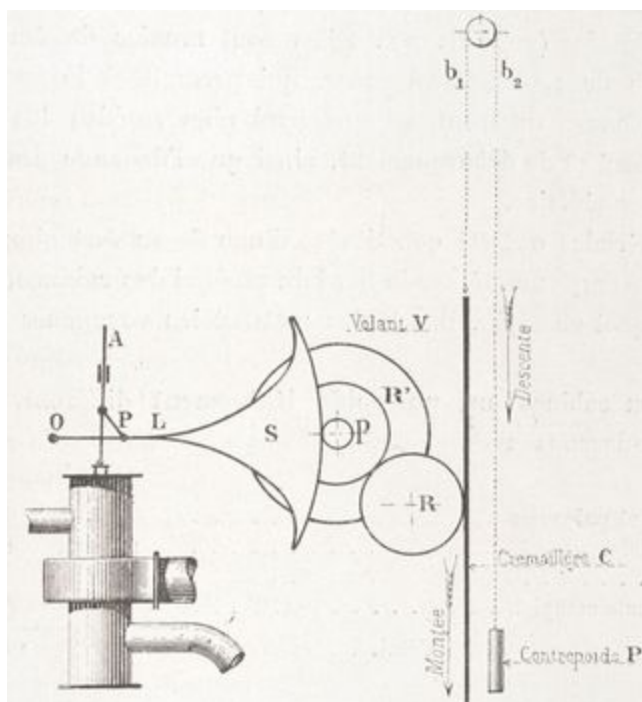
Fig. 26. — Commande des distributeurs.
