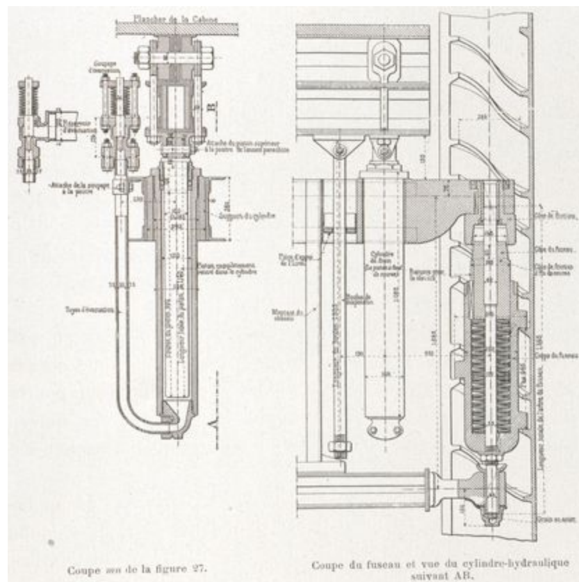
Fig. 29. — Parachute de la cabine B.
