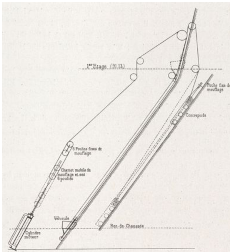
Fig. 11. — Ensemble de l'ascenseur Otis transformé.
