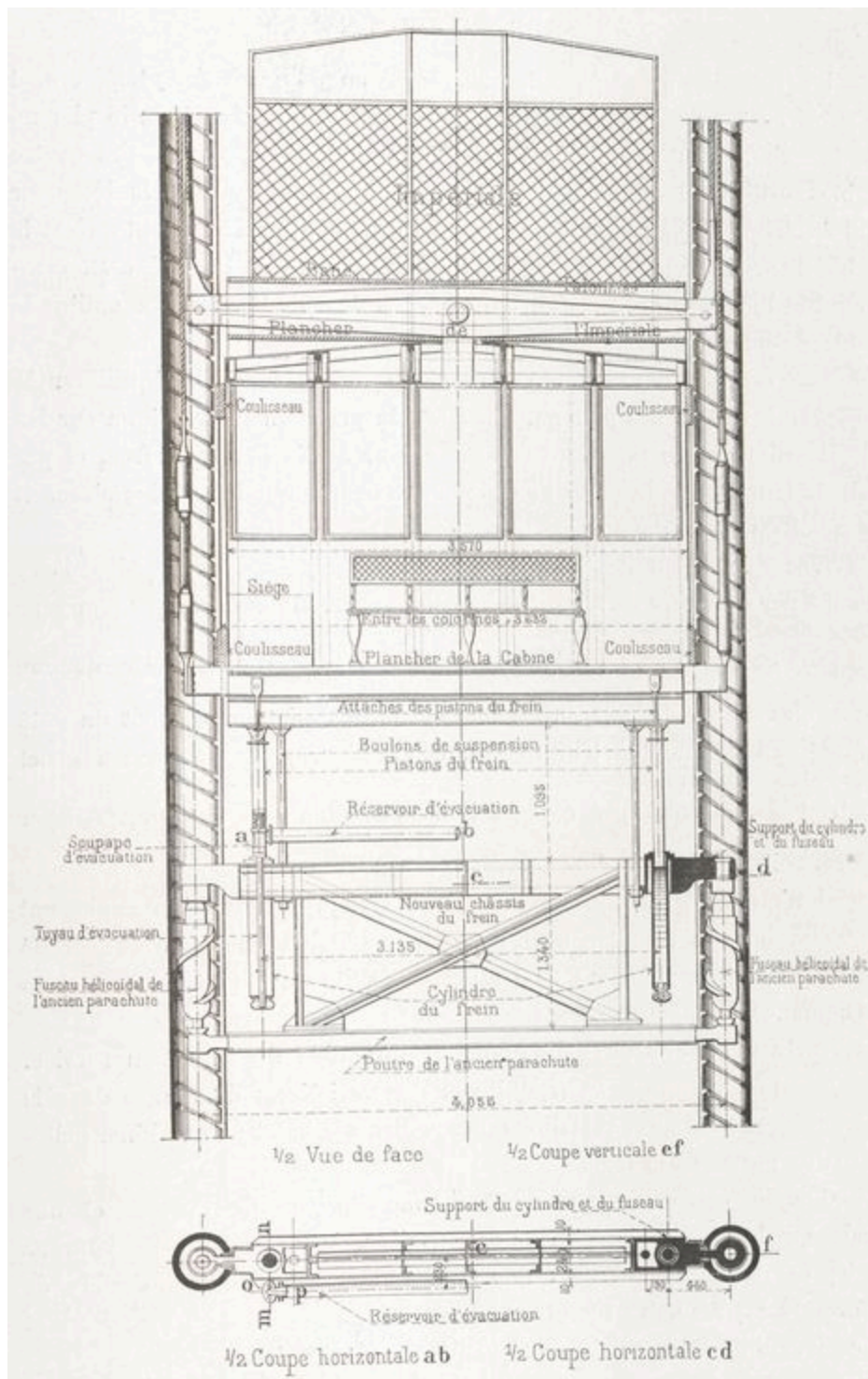
Fig. 27. — Cabine contrepoids B, avec son parachute complet.
