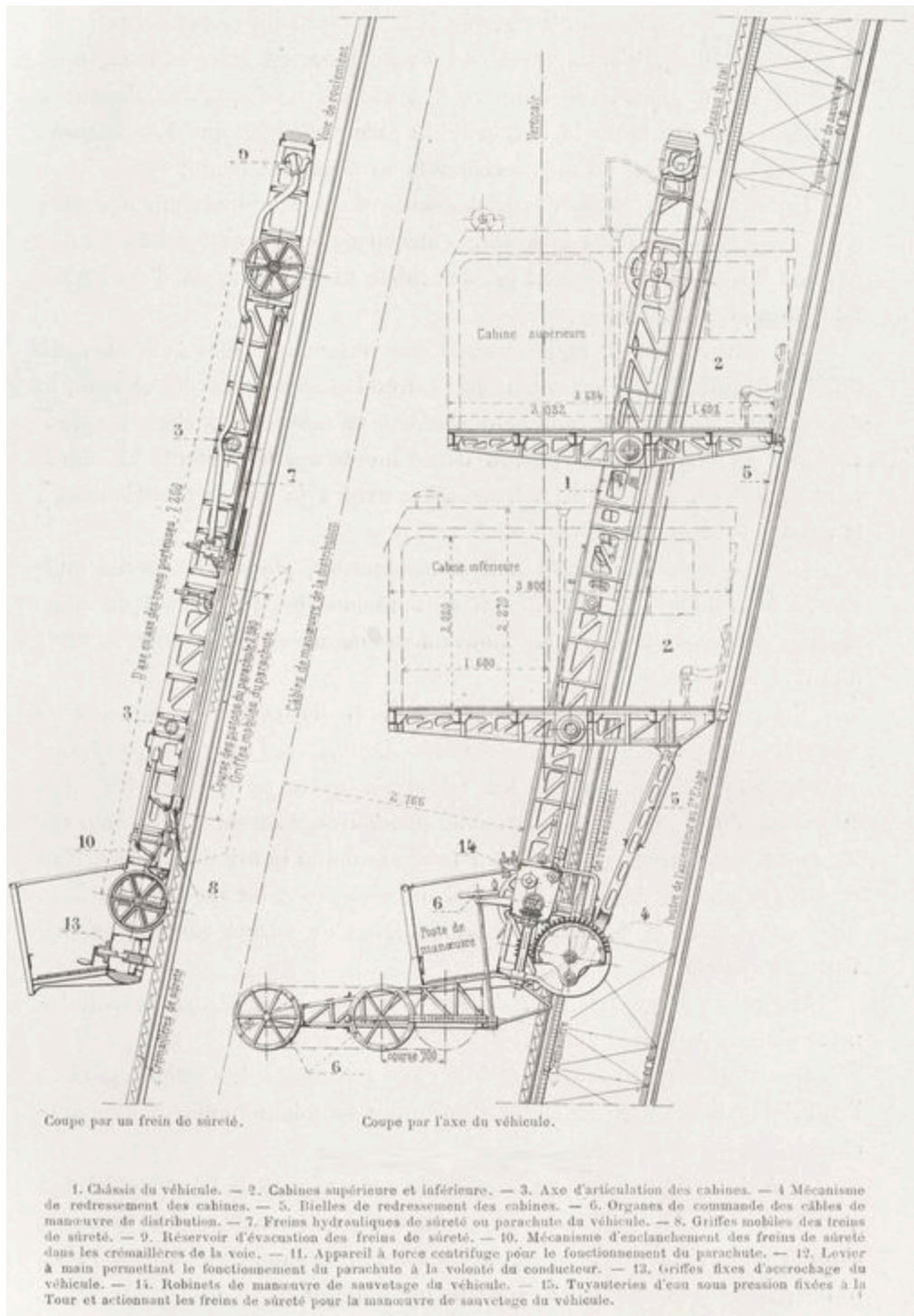
Fig. 10. — Détail du véhicule.
