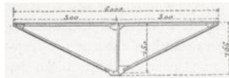
FIG. 87. — ÉLÉMENT TRIANGULAIRE D'UN PONT DÉMONTABLE.
