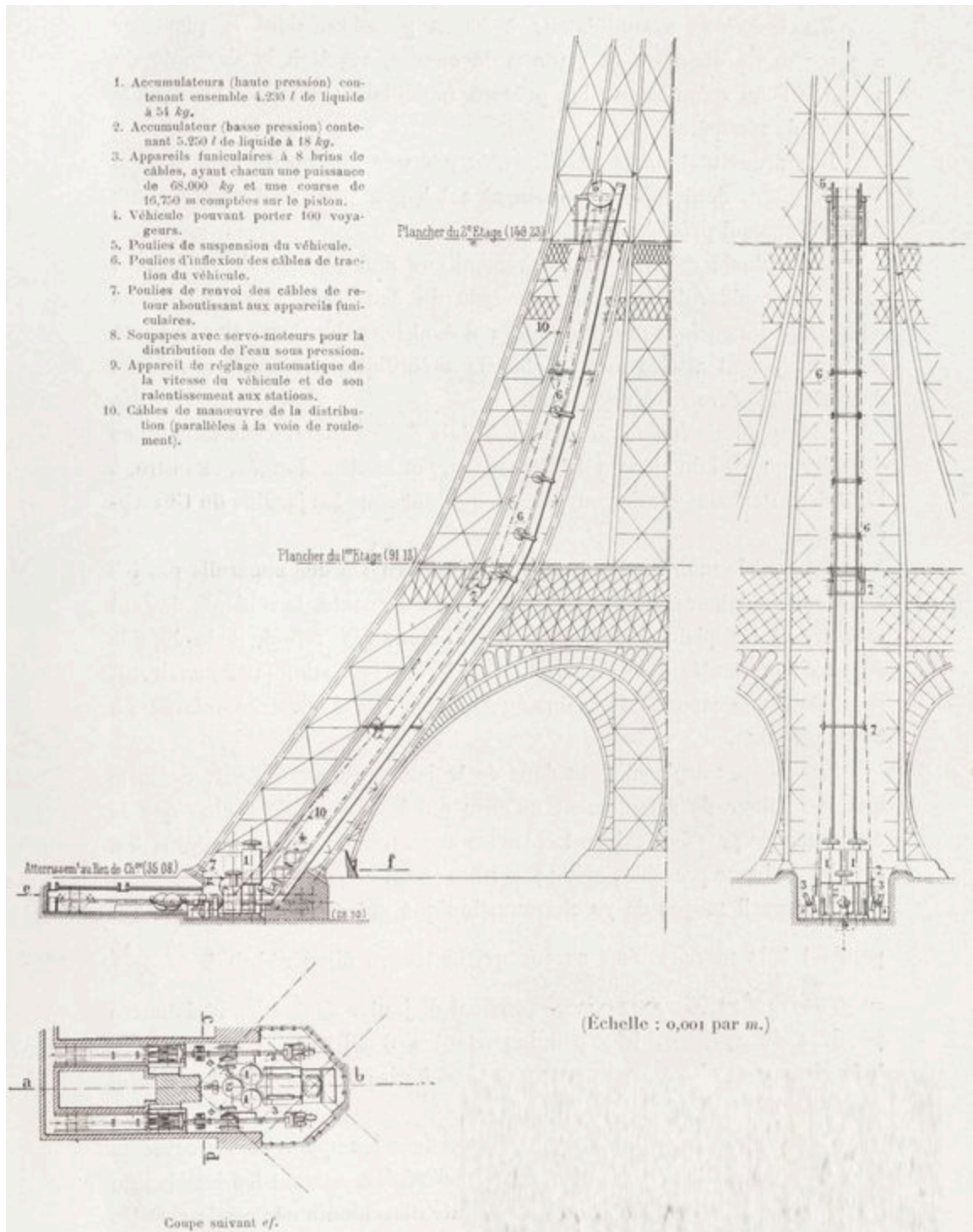
Fig. 6. — Ensemble de l'ascenseur. (Échelle : 0,001 par m.)
