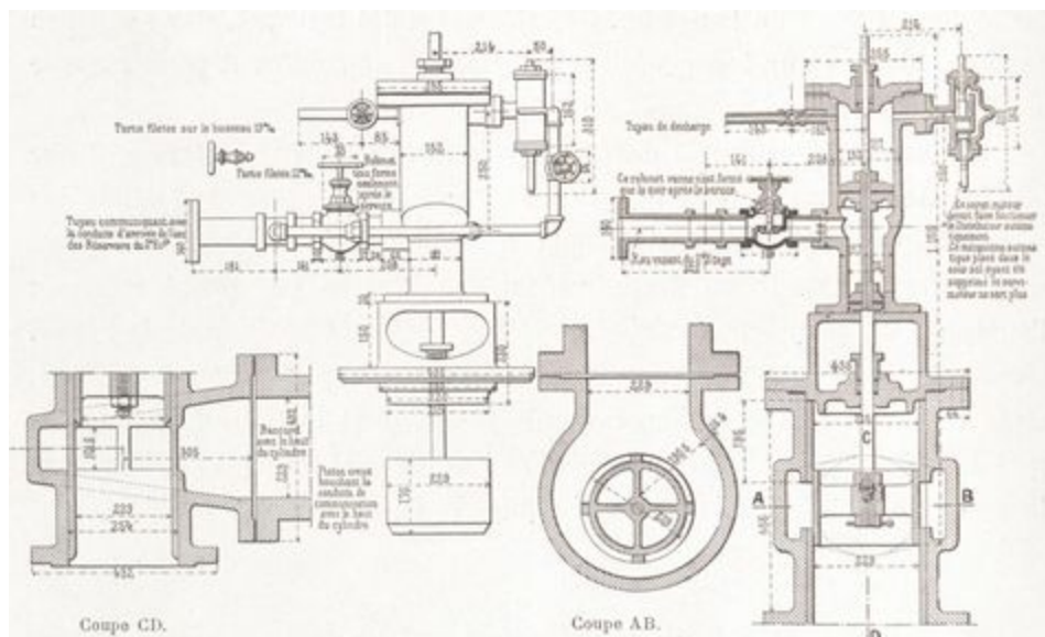
Fig. 58 . — Détail du distributeur de sûreté.
