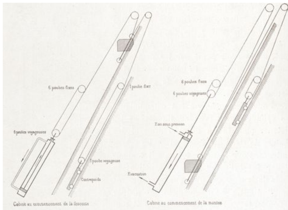
Fig. 3. — Schéma de l'ascenseur.
