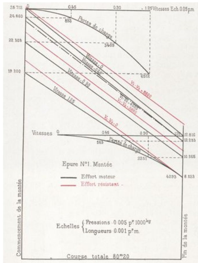
Fig. 65. — Épure de la montée.
