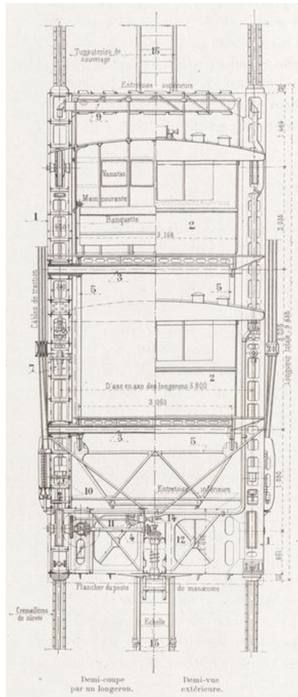
Fig. 9. — Détail du véhicule. (Échelle : 0,015 par m.)
