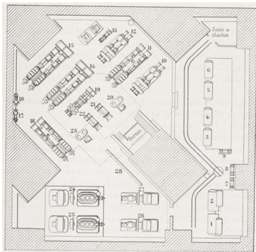
Fig. 35. — Plan général de la salle des machines.
