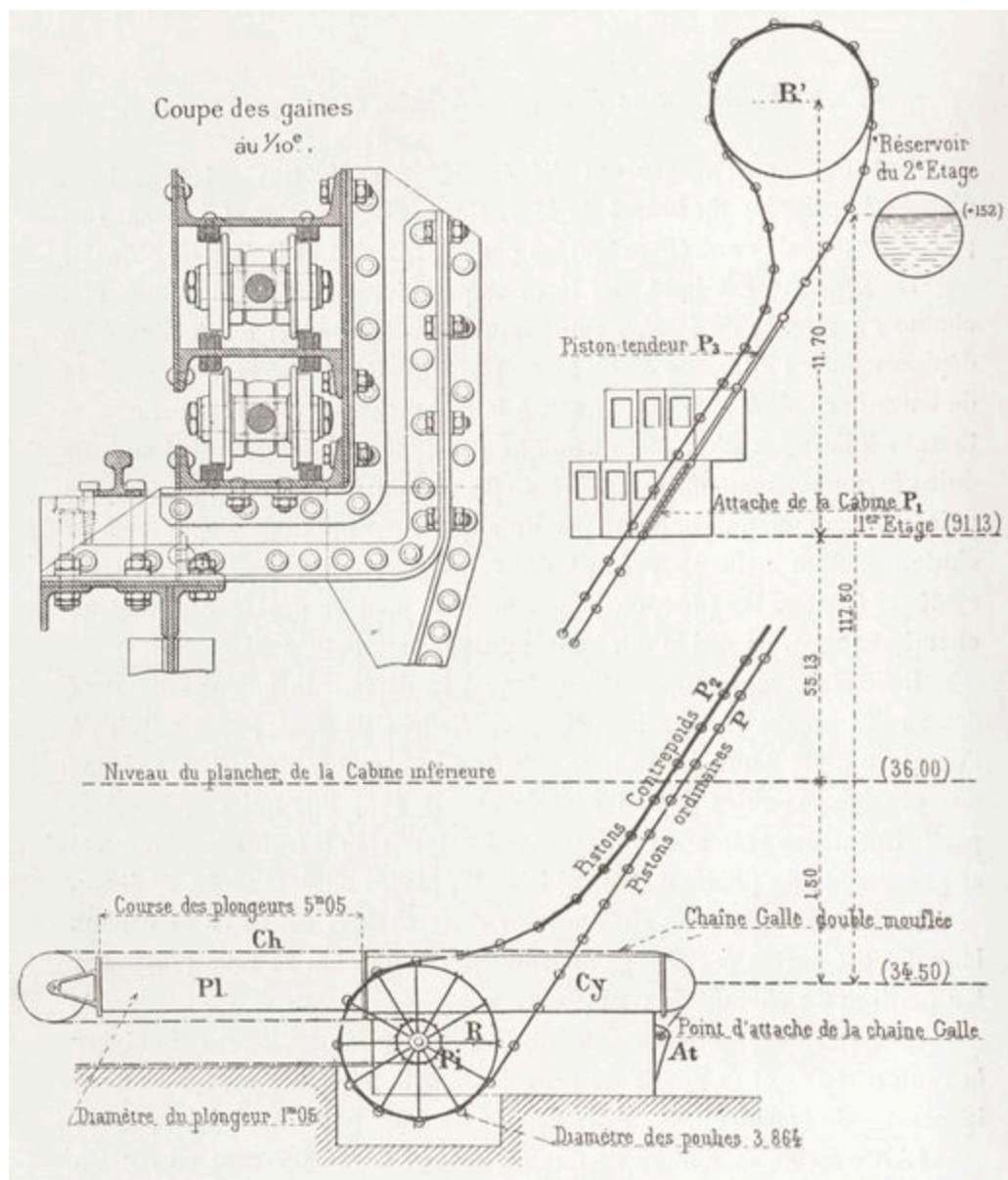
Fig. 1. — Schéma de l'ascenseur Combaluzier.
