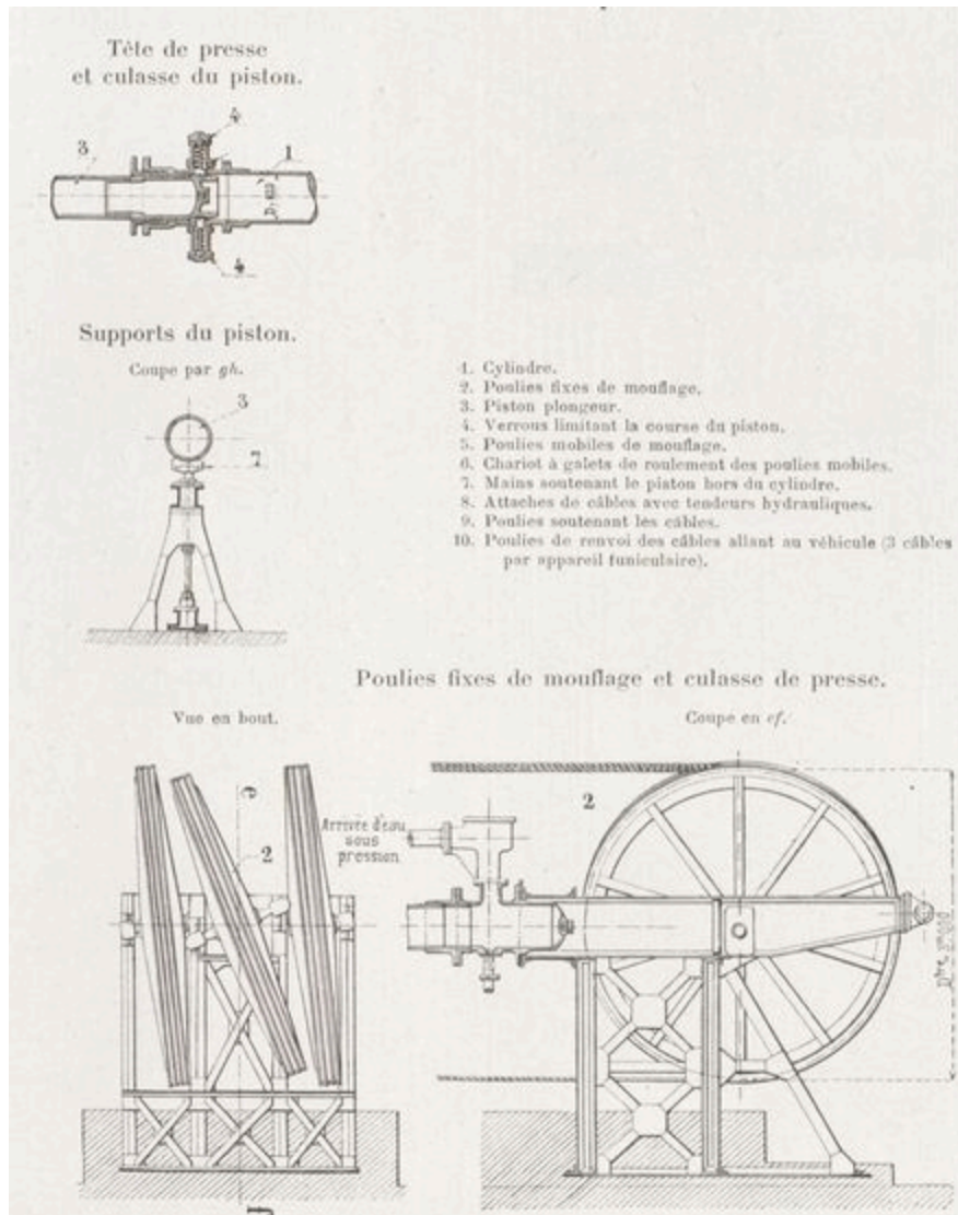
Fig. 8. — Détail de l'appareil funiculaire. (Échelle : 0,015 par m.)
