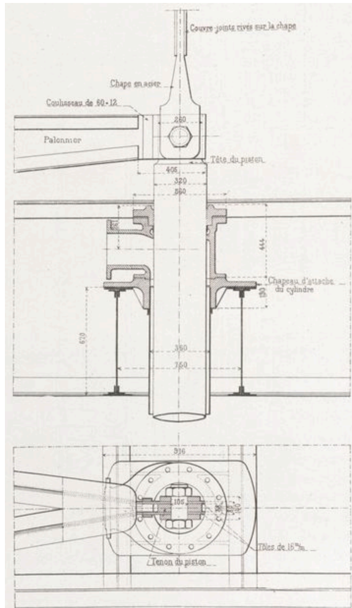
Fig. 19. — Plan et coupe verticale de la tête d'un cylindre.
