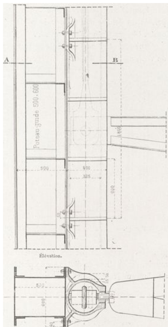
Fig. 21. — Colonnes-guides des pistons.
