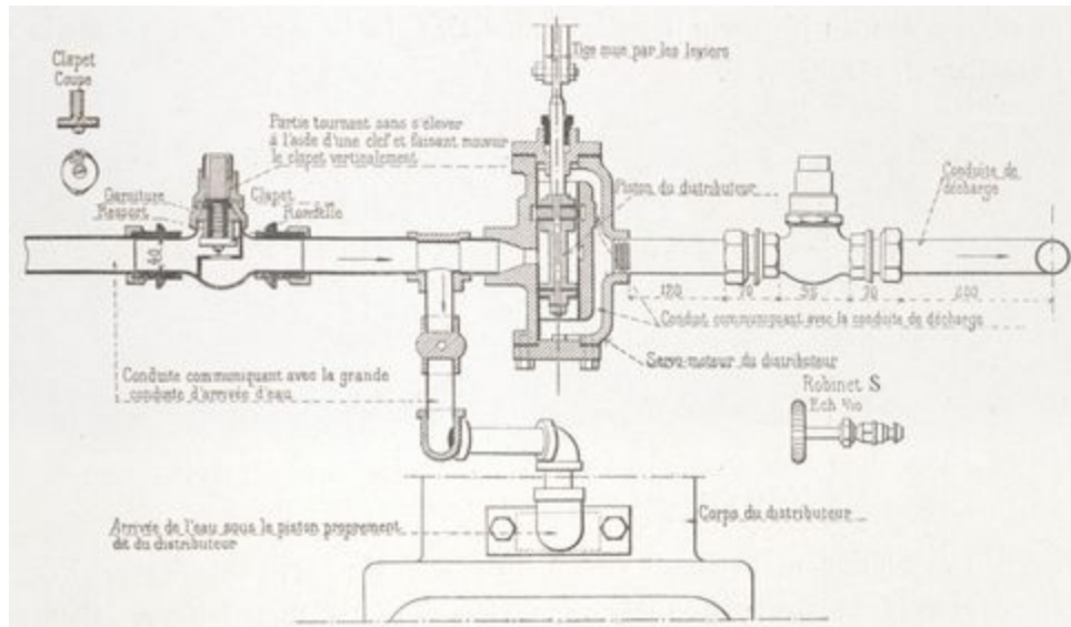
Fig. 54. — Tuyauterie du distributeur.
