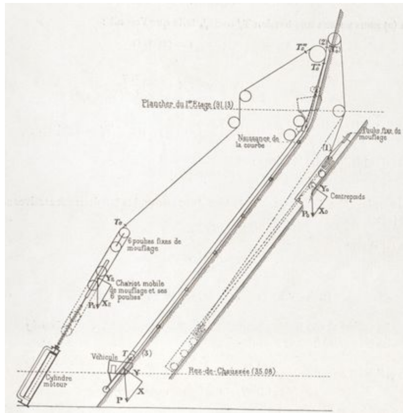
Fig. 63. — Ensemble de l'appareil.
