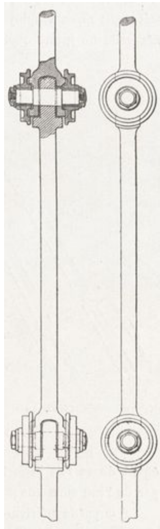
Fig. 2. — Pistons articulés au 1/10 e .
