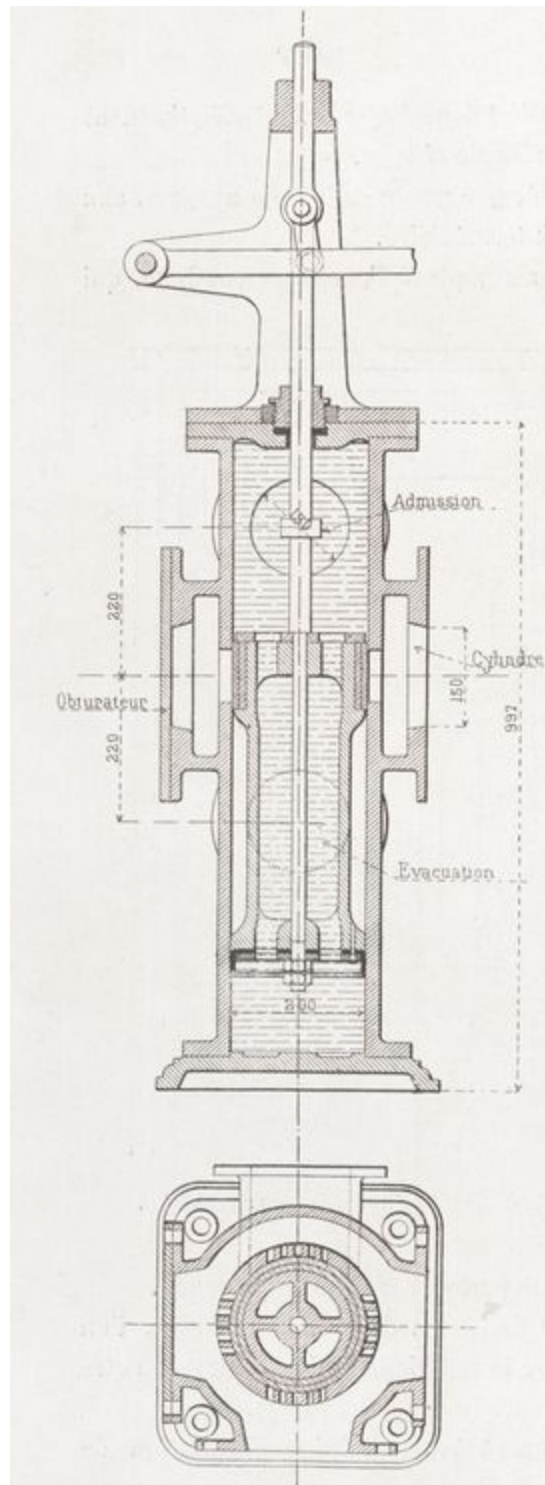
Fig. 24. — Distributeur (coupes horizontale et verticale).
