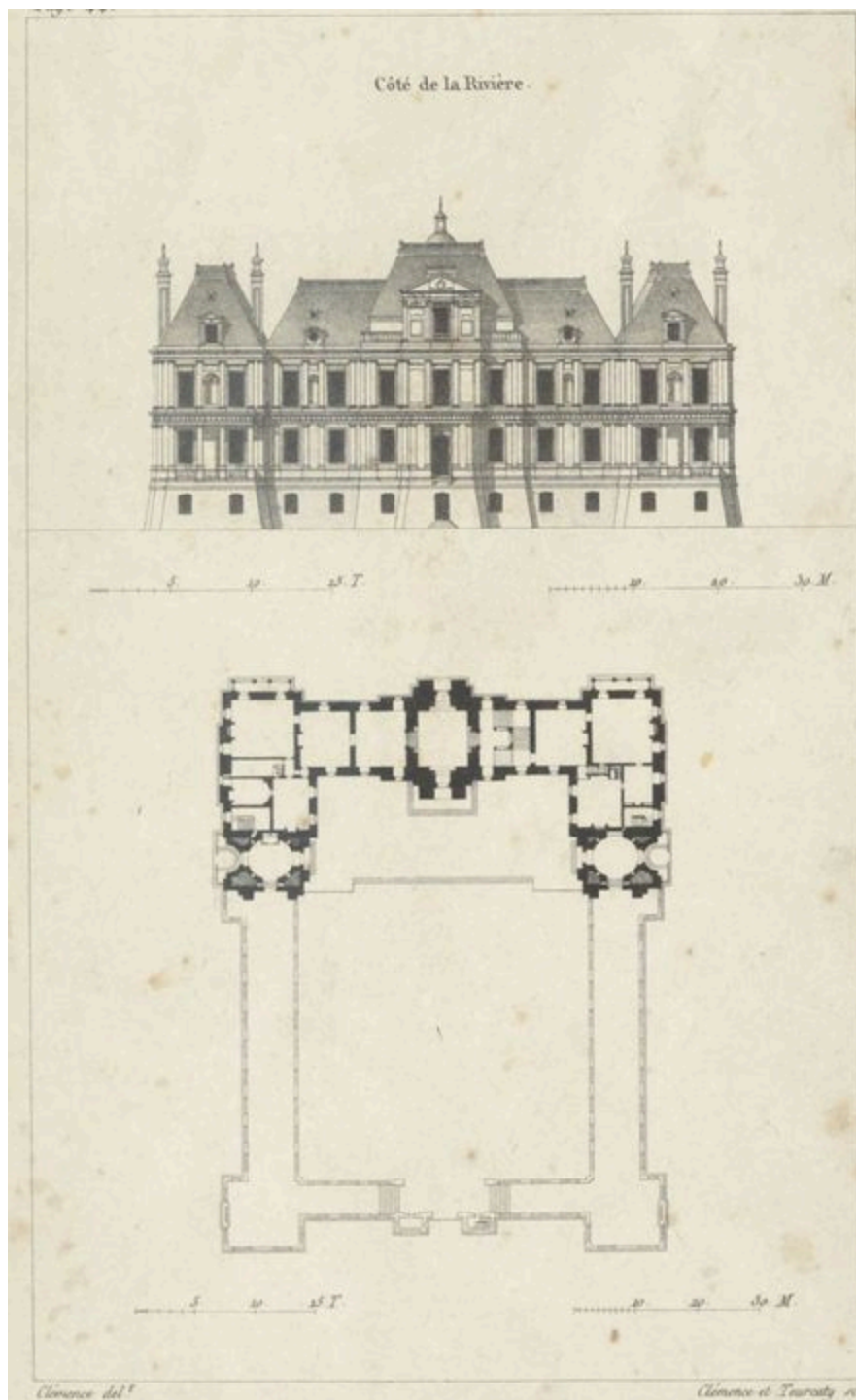
Plan et Elévation du Château de Maisons.
