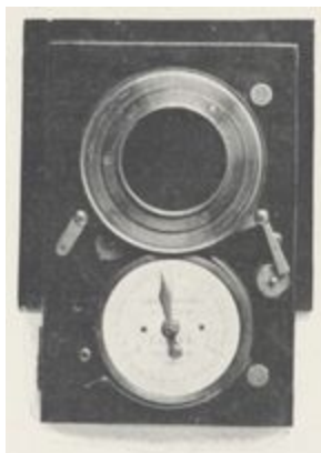
Obturateur P. Boca.
