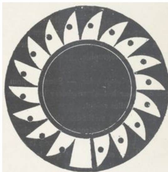
Passage de Vénus sur le soleil (1874). Cliché obtenu par le revolver photographique de M. Janssen.
