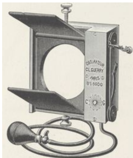
Obturateur Guerry, à double volet.
