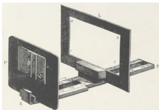
Chercheur focimétrique de M. Davanne.
