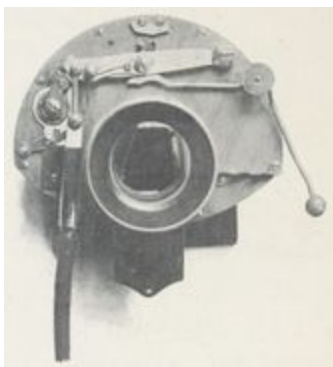
Obturateur Bezu et Hauser.
