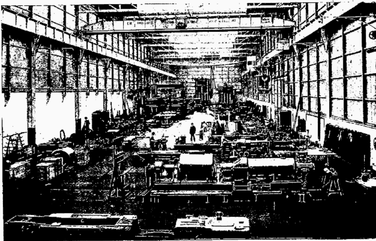
Vue intérieure des usines de Fives-Lille.
