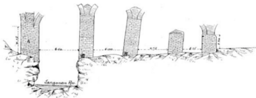
Fig. 18. — Pont-aqueduc de Langonan.
