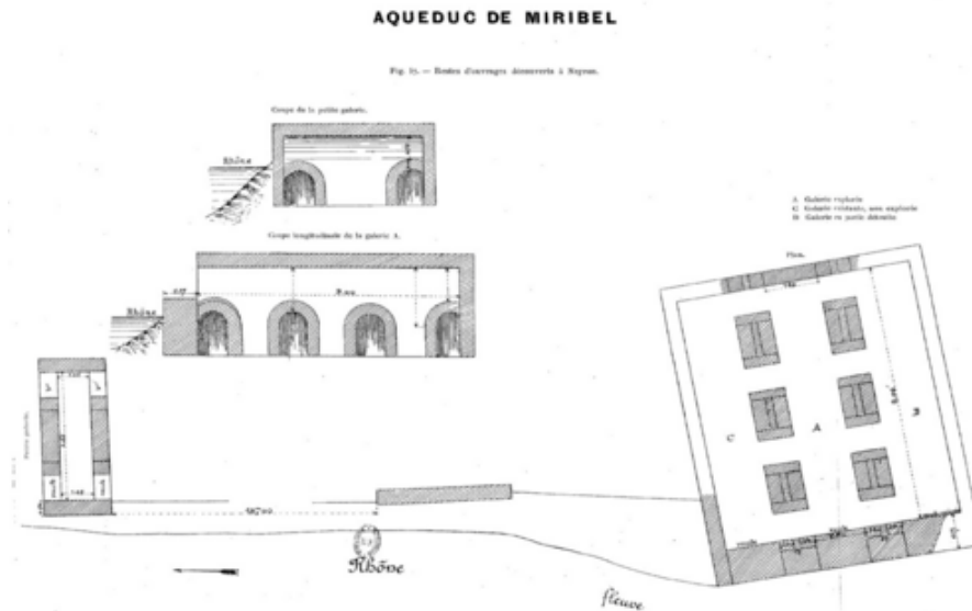
Fig. 03. — Restes d'ouvrages découverts à Neyron.
