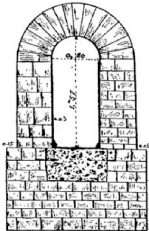
Fig. 10. — Coupe de l'aqueduc à La Valsonnière.
