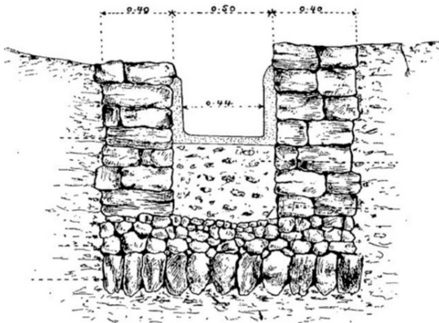
Fig.5. — Section de l'aqueduc à Vaugneray.
