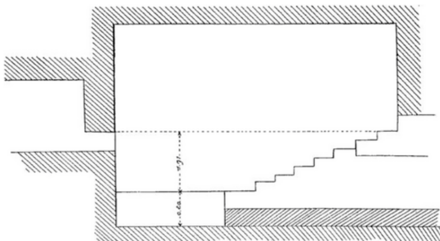
Fig. 64. 2 e réservoir d'Arche. Coupe longitudinale.
