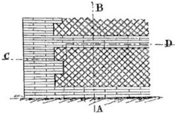
Fig. 91. — Opus reliculatum (comportant toujours le blocage intérieur).
