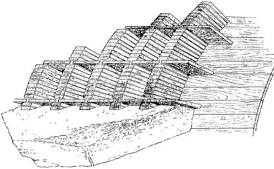
Ossature des voûtes romaines (D'après M. A. Choisy, L'art de bâtir chez les Romains .)
