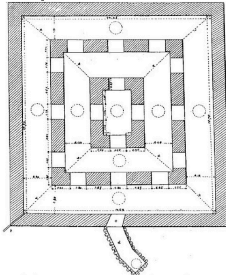
Fig. 126. — Citerne romaine du Grand-Séminaire de Lyon.
