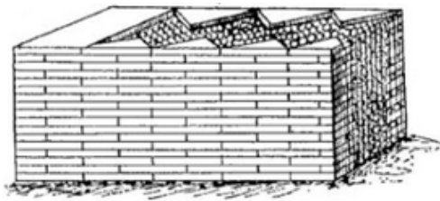
Fig. 96. — Opus latericium. (Maçonnerie de briques).
