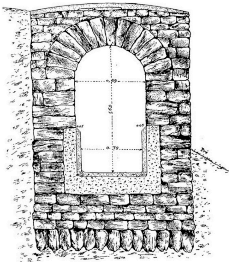
Fig. 11. — Coupe de l'aqueduc près de Chevinay ( aux Thus ).
