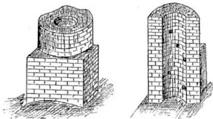
Fig. 112. — Regards à l'aqueduc de Dougga.
