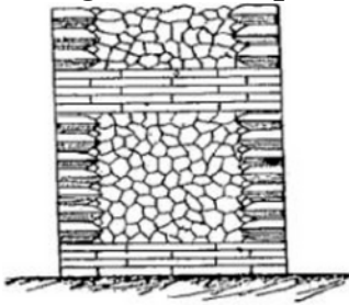
Coupe suivant A B.
