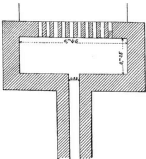
Fig. 20. — Réservoir de chasse de Saint-Genis (coupe horizontale au niveau des orifices).
