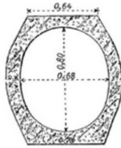
Fig. 110. — Section de l'aqueduc de Rochefort.
