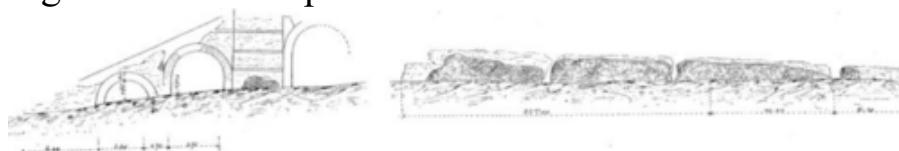
Fig. 39. — Siphon du Garon. Réservoir de fuite.
