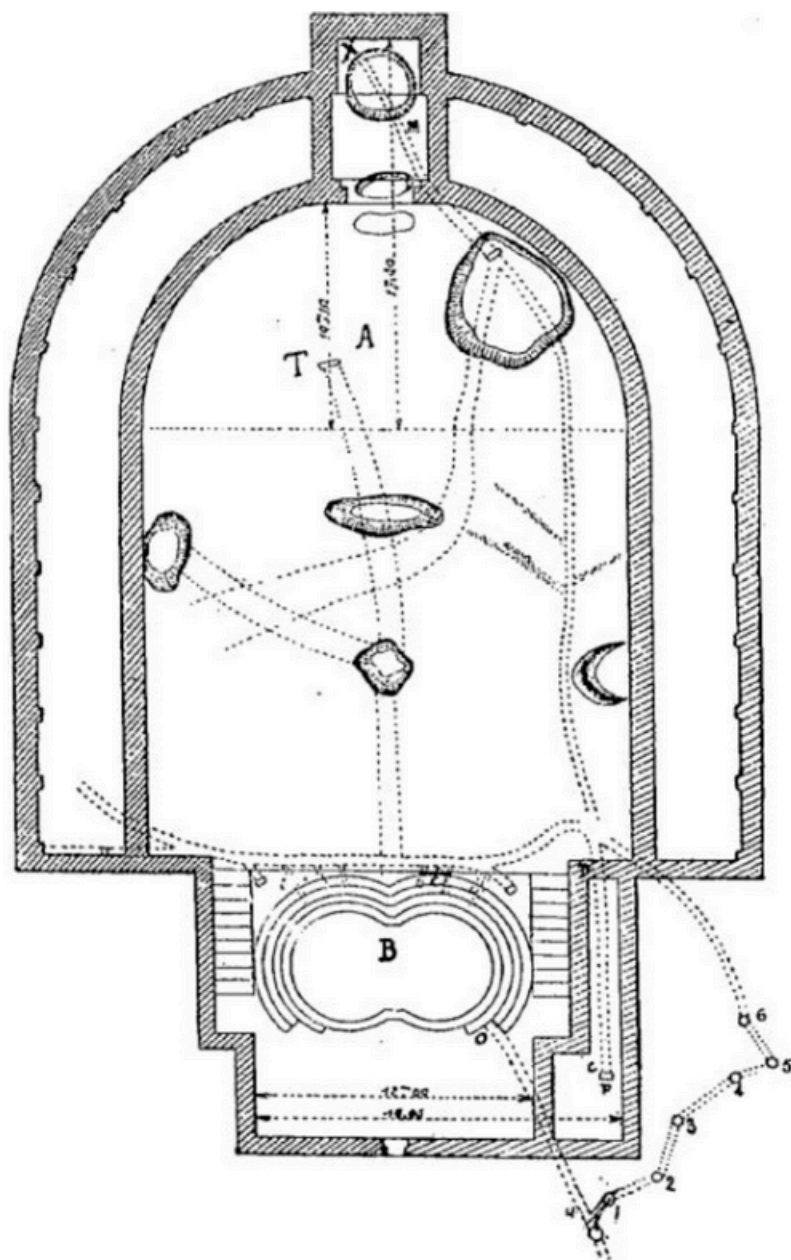
Fig. 61. — Nymphée de Zaghouan, avec prise d'eau souterraine.
