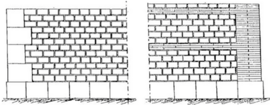
Fig. 88. — Structure en moyen appareil.
