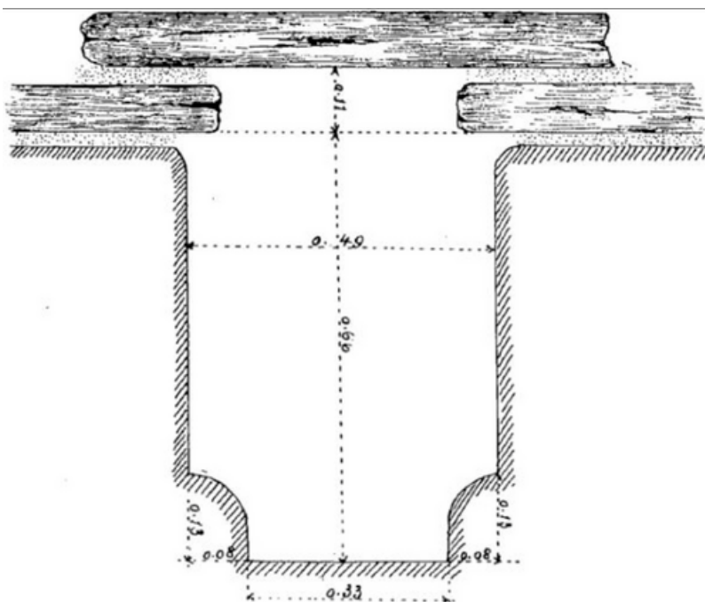
Fig. 4. — Section de l'aqueduc à Saint-Cyr (d'après M. Gabut).
