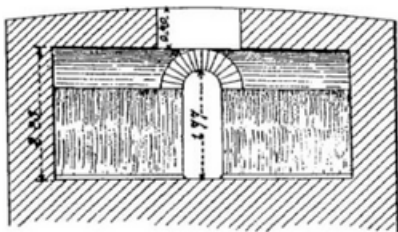
Fig. 29. — Réservoir de chasse du siphon de Soucieu. Coupe horizontale au niveau des orifices.
