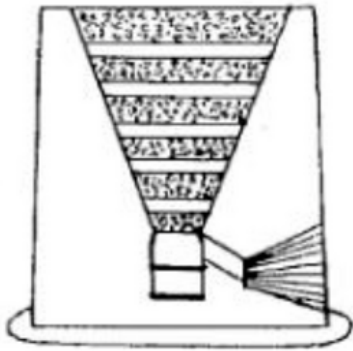
Fig. 105, — Four à chaux primitif, à feu continu.
