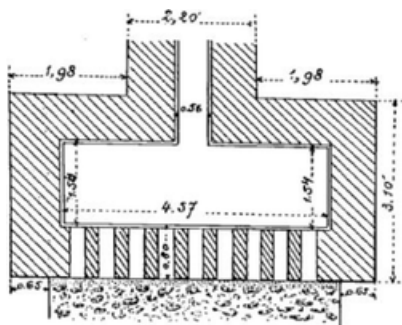
Fig. 30. — Réservoir de chasse du siphon de Soucieu. Coupe longitudinale.
