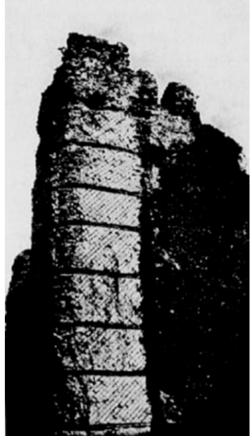
Fig. 95. — Siphon de Beaunant. Pile de support du réservoir de chasse, face arrière.
