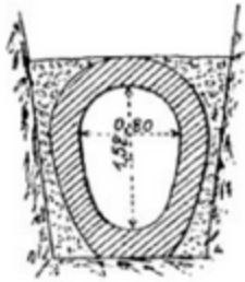
Fig. 109. — Section de l'aqueduc de Rochetaillée (Saint-Étienne).
