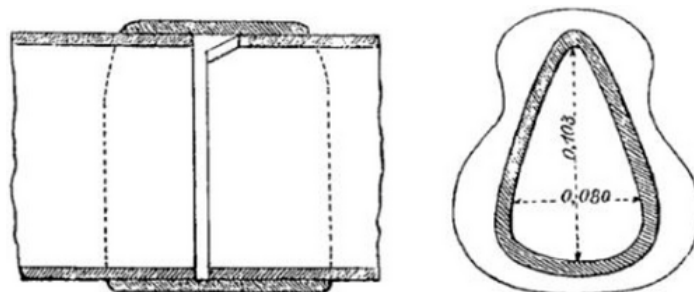
Fig. 77. — Tuyau découvert rue Gay-Lussac.
