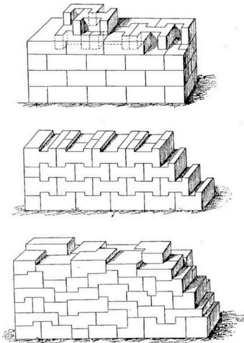
Fig. 90. — Opus revinctum.
