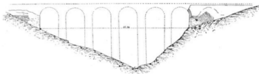
Fig. 22. — Pont sur le Feloing.
