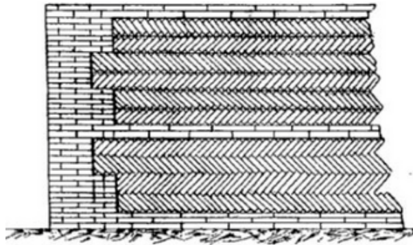
Fig. 92. — Opus spicatum.
