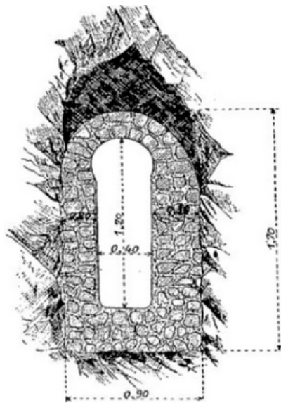
Fig. 115. — Aqueduc de Sens. Section de l'aqueduc en tunnel.
