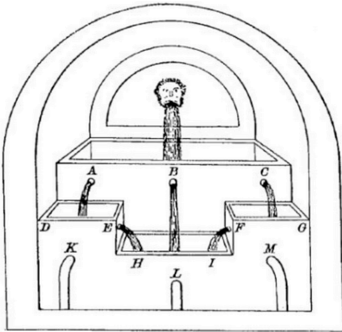
Fig. 123. — Distribution théorique au château d'eau. Dessin de Perrault, d'après Vitruve.
