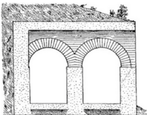
Fig. 56. - Aqueduc de Miribel. Chambre voûtée où aboutissent les galeries jumelles.
