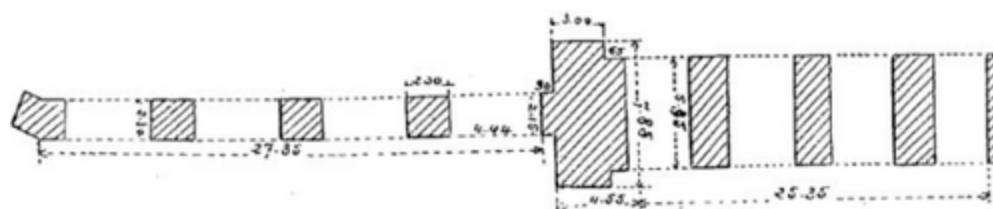
Fig. 43. — Réservoir de chasse du siphon de Beaunant. Plan de l'ensemble et des abords.
