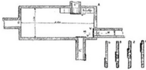
Fig. 125. — Chambre de distribution, à Tebourba (Tunisie).
