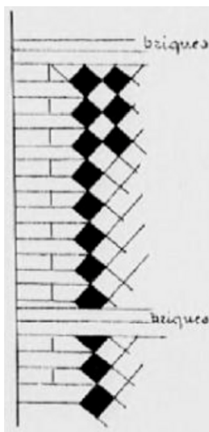
Fig. 37. — Pont du Garon. Détail du parement.
