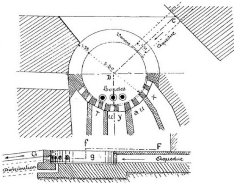
Fig. 124. Chambre de distribution ( Castellum divisorium ) de Nîmes.
