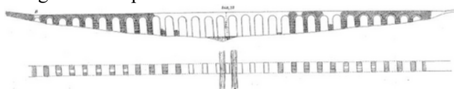
Fig. 40. — Pont-siphon de Beaunant. Ensemble des arcades.
