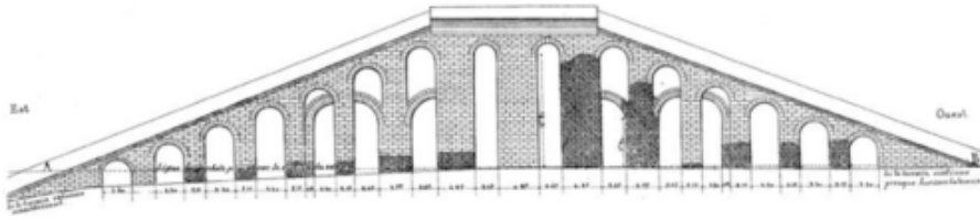
Fig. 8. — Reconstitution du monument des tourillons, par M. Gabut.
