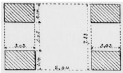
Fig. 48. — Piles évidées. Plan.
