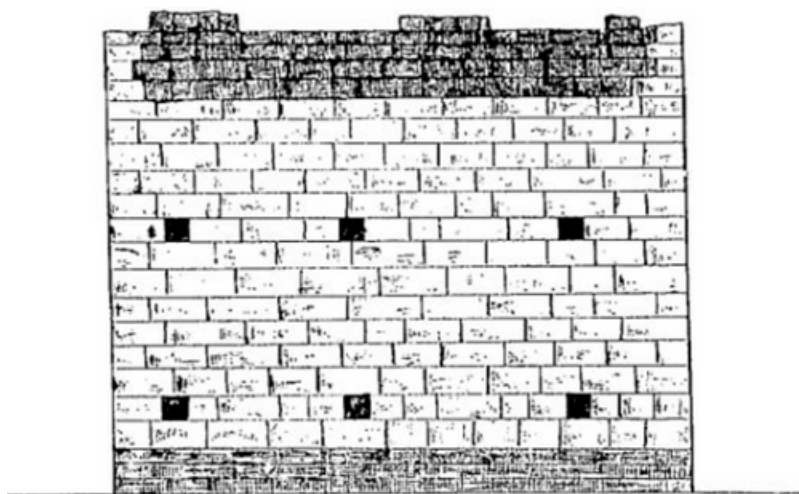
Fig. 97. — Pile du pont de Grange-Blanche. Parement en petit appareil rectangulaire, avec trous d'échafaudages.
