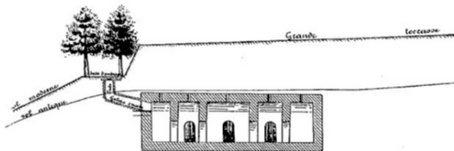
Fig. 127. — Citerne du Grand-Séminaire. Situation par rapport au sol du jardin.
