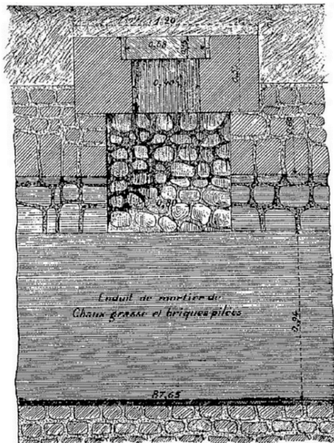
Fig. 113. — Regards à l'aqueduc de Sens.
