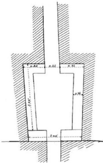
Fig. 63. — Premier réservoir d'Arche. Plan.
