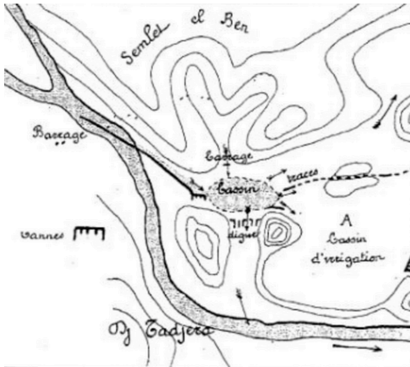
Fig. 66. — Barrage de l'oued Hallouf.
