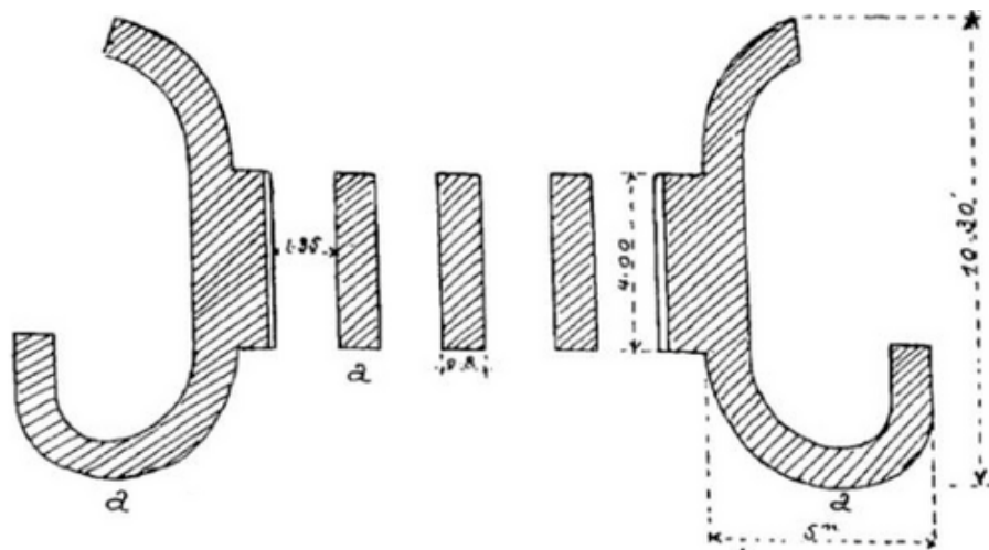
Fig. 65. — Barrage de l'Henchir Saïd (Tunisie).
