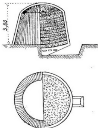
Fig. 107. — Four à chaux en meule.
