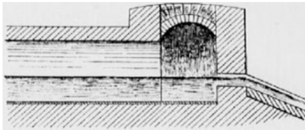
Réservoir de Soucieu. Coupe transversale.
