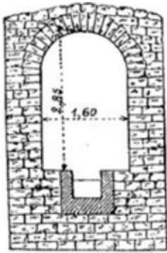
Fig. 111. — Section de l'aqueduc de Montpellier.
