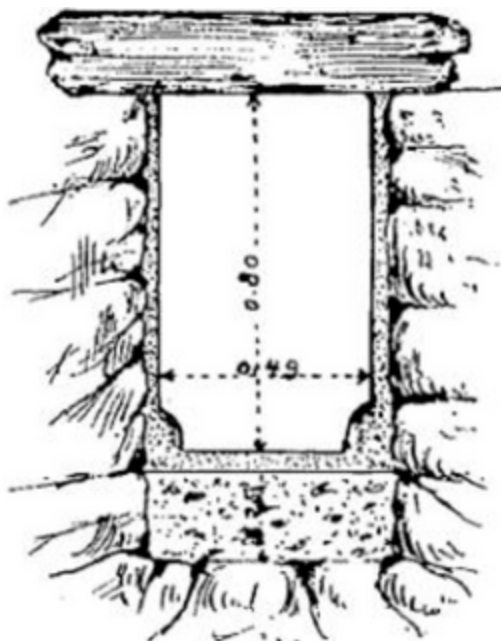
Fig. 3 — Profil de la section aux carrières de la Blache.
