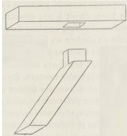
Fig. 60. Tenon biais.
