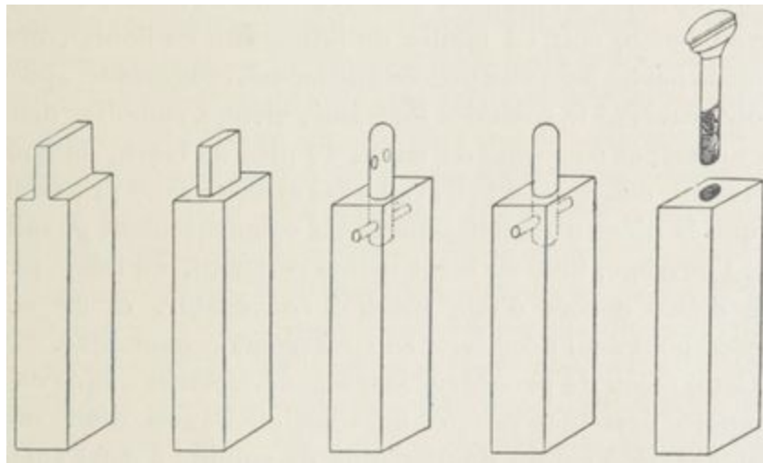
Fig. 46 à 50. — Diverses sortes d'assemblages usités dans la confection des grilles. — Assemblage à tenon d'épaisseur, — à tenon réduit, — à tenon rapporté, — à tenon rapporté et à prisonnier, — à vis.
