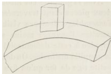
Fig. 59. — Tenon greffé sur un fer courbe.
