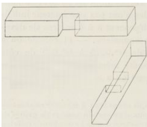
Fig. 51. — Assemblage à demi-fer.
