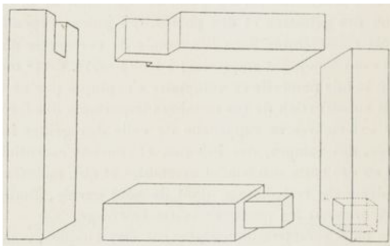
Fig. 56 et 57. — Assemblage de grilles par enfourchement et à tenon et mortaise.
