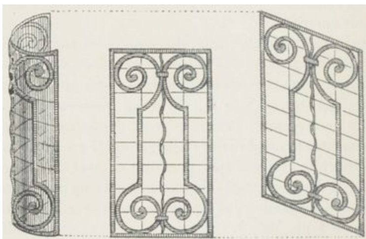
Fig. 71 à 73. — Manière d'incliner ou de recourber les panneaux de rampe.
