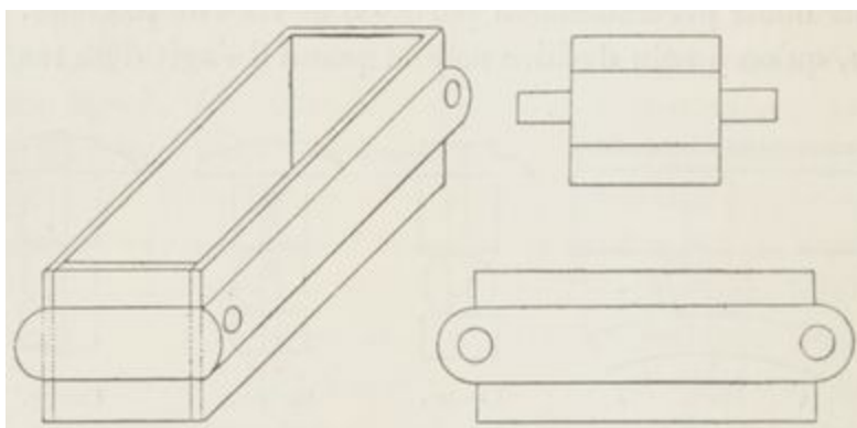
Fig. 65 à 67. — Collier à cordon : le collier monté et les côtés avant l'assemblage.
