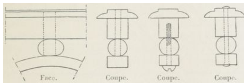
Fig. 61 à 64. — Diverses sortes d'assemblages à boules : assemblage à tenon, à vis, à goupille.
