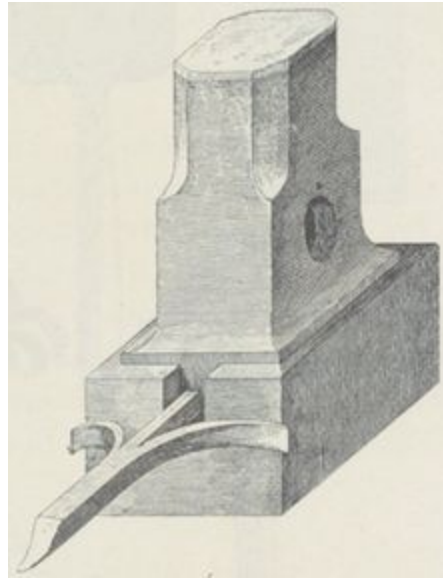
Fig. 25. — Étampe fermée.
