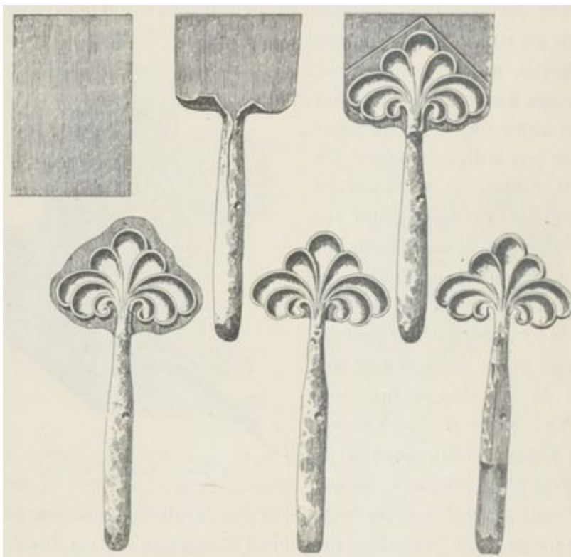
Fig. 26 à 31. — Passes successives d'un fleuron estampé. — La masse forgée. — La masse dégrossie. — Premier passage à l'étampe. — Le fleuron ébarbé. — Le fleuron découpé. — Le fleuron dégagé et terminé à la lime.
