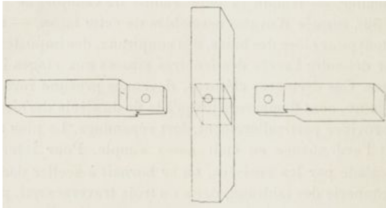
Fig. 53. — Assemblage en deux parties.
