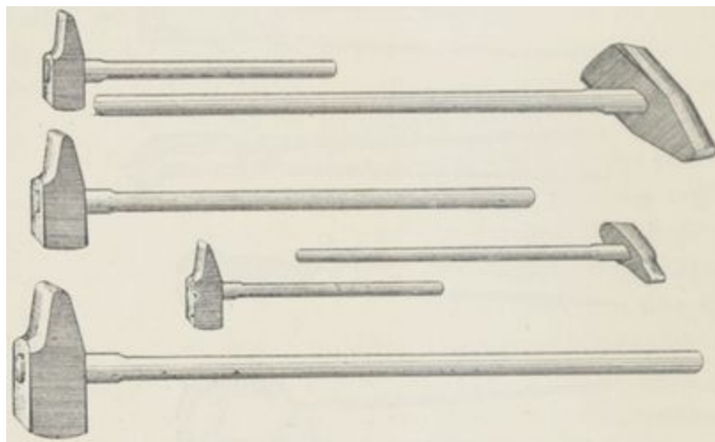
Fig. 12 à 17. — Marteau à main pour forgeron. — Marteau à devant panne en long. — Petit marteau à devant panne en travers. — Marteau à main à bigorne. — Marteau rivoire pour ajusteur. — Grand marteau à devant panne en travers.
