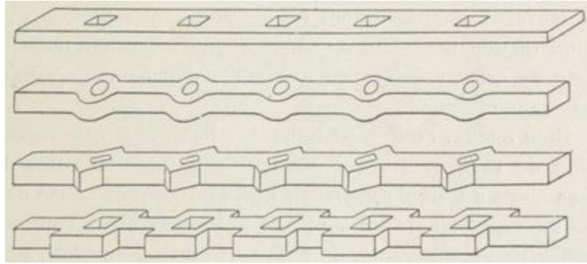
Fig. 41 à 44. — Sommiers préparés pour recevoir les barreaux d'une grille.
