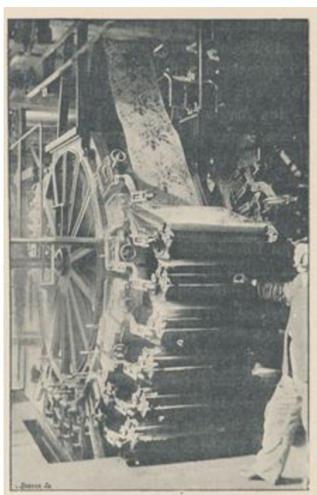
Machine à papier peint en 24 couleurs (vue de côté) Manufactures Gillou & fils
