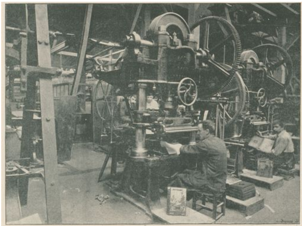
Presser pour le tirage en couleur des couvertures Maison Lenègre
