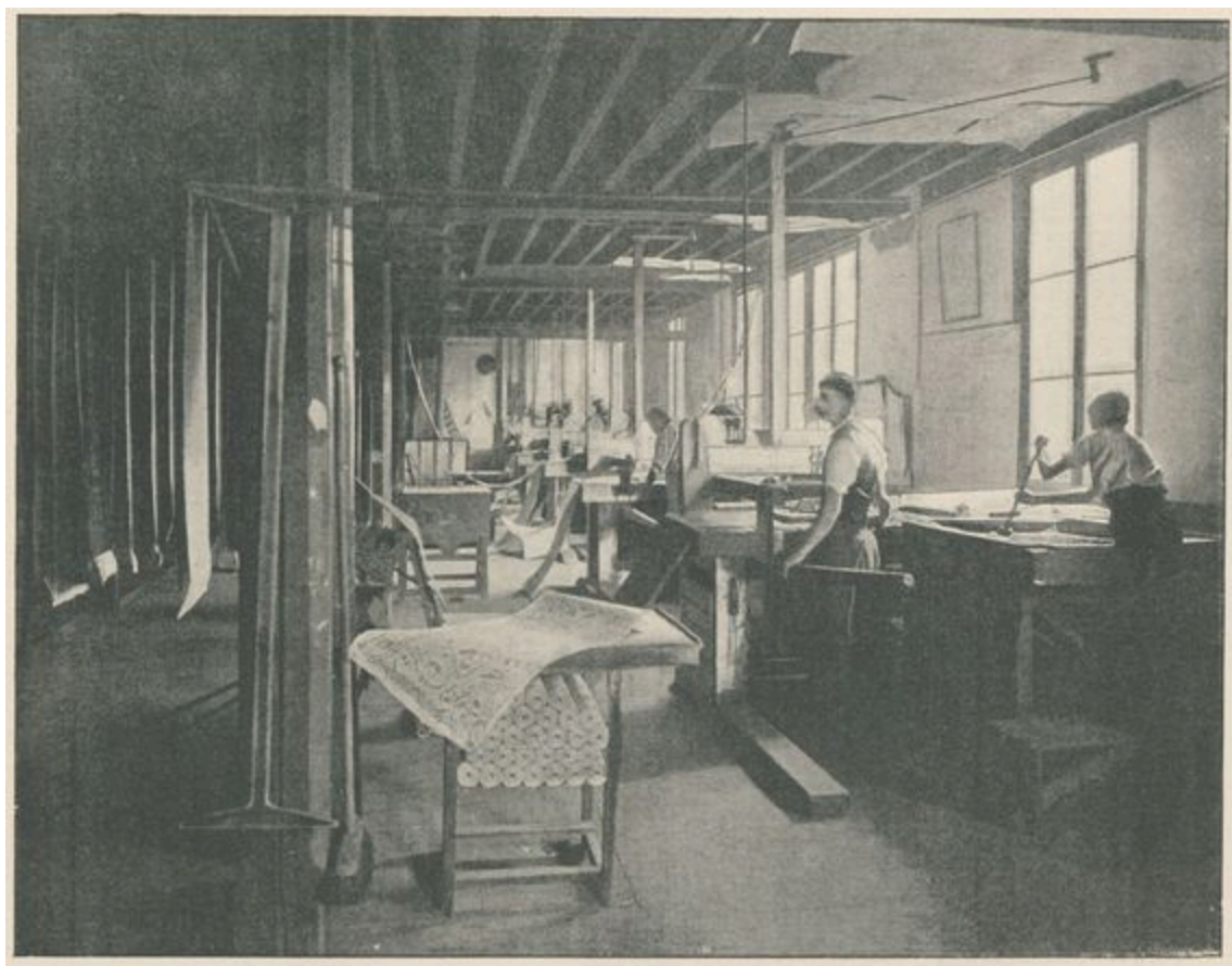
Un Atelier d'impression du papier peint Fabrique Jouanny
