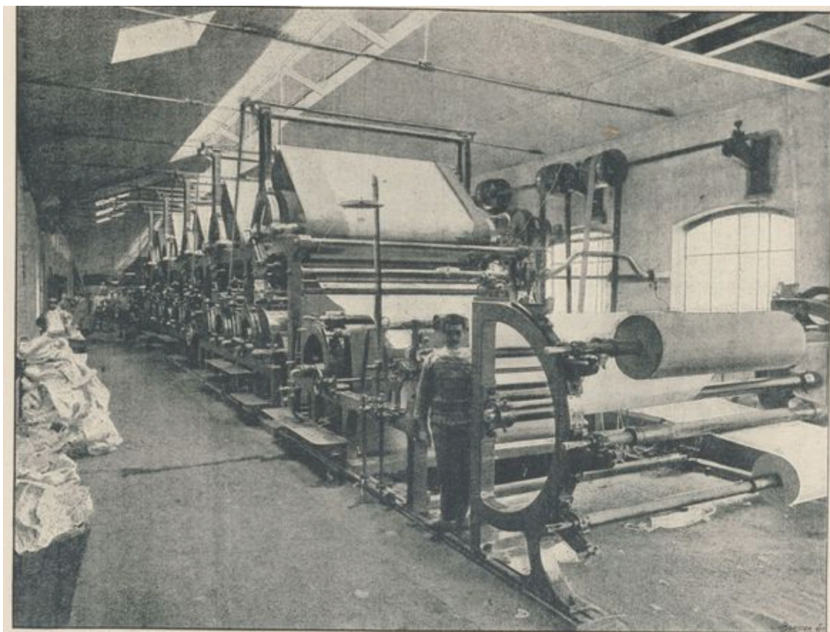
Machine Lhuillier à fabriquer le papier : la Sécherie Usine Firmin-Didot
