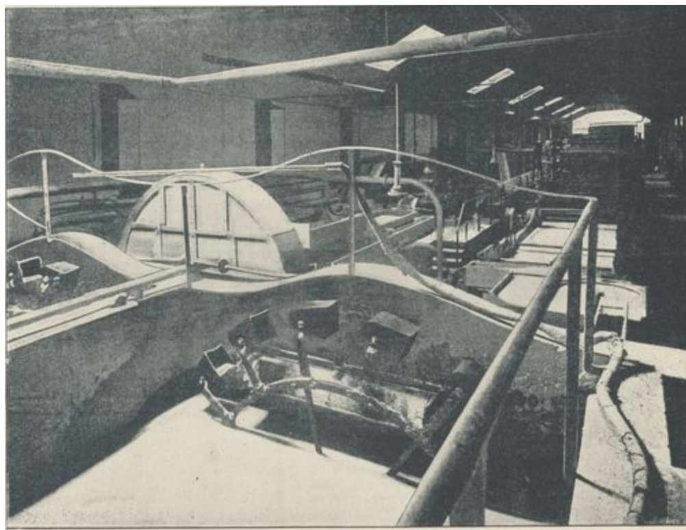
Machine à fabriquer le papier & le carton. Cuver & Epurateurs Usine Vacquerel
