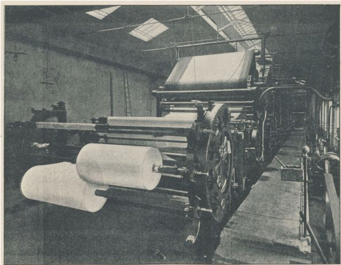
Machine Lhuillier à fabriquer le papier : Vue d'ensemble Usine Firmin-Didot
