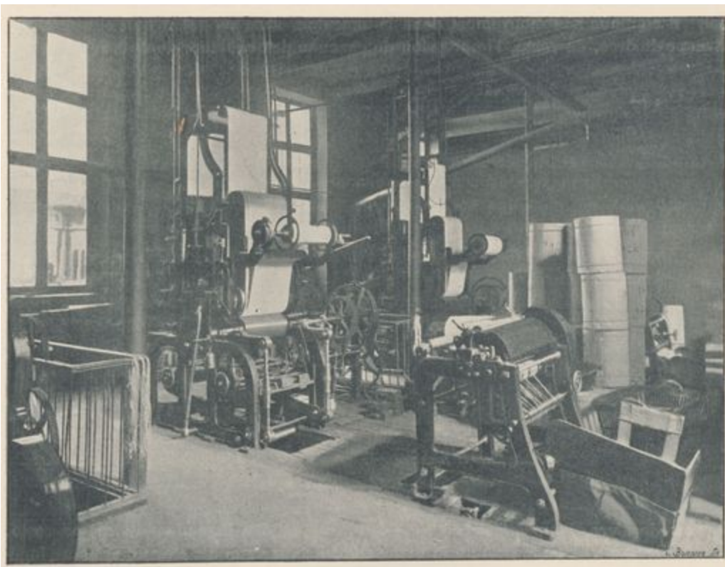
Machine Godchaux à imprimerie en taille-douce les cahiers scolaire
