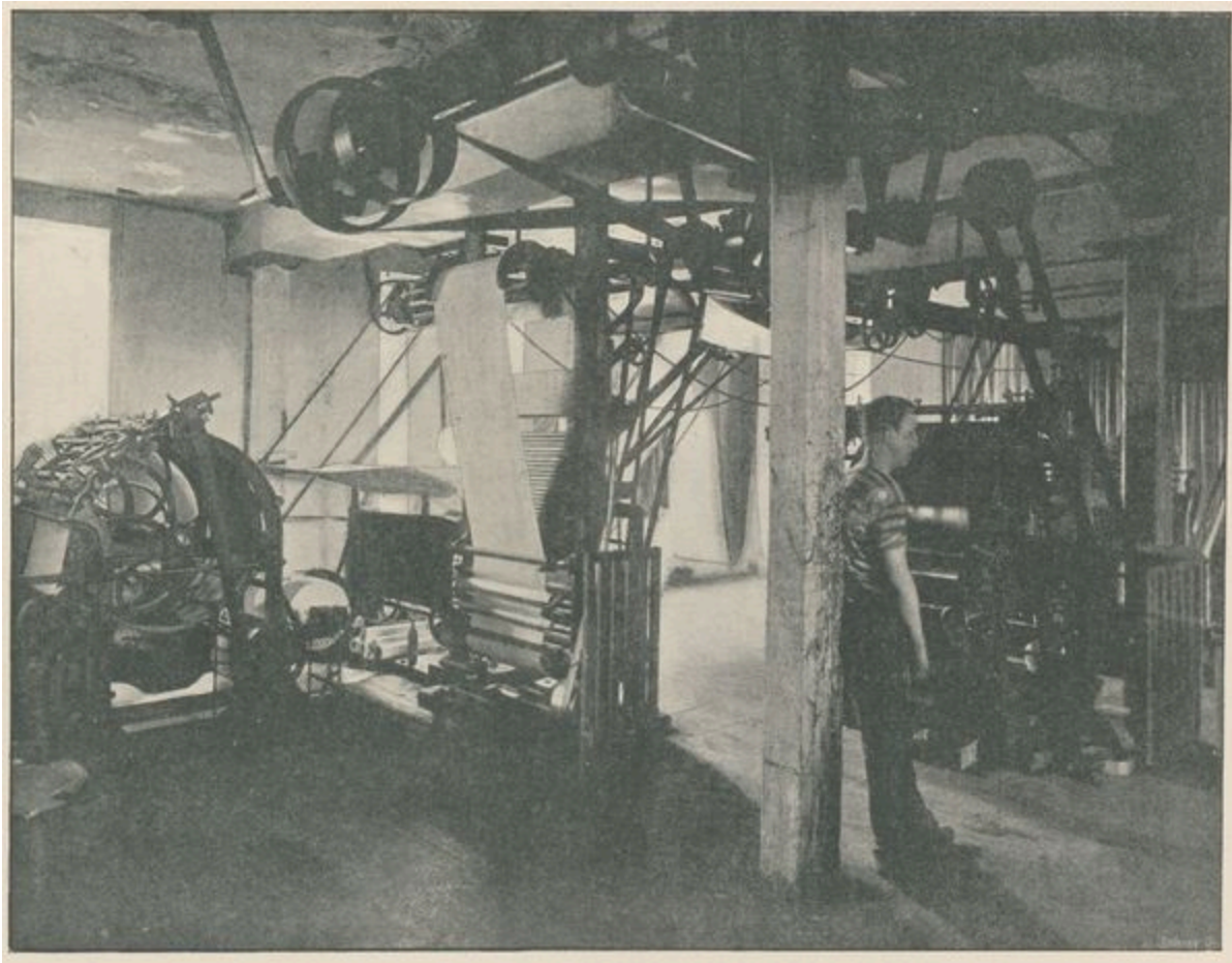
Fabrication mécanique du papier de fantaisie : Machines à foncer, avec accrocheuses & bobineuses Usine Vacquerel
