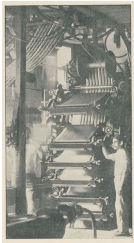
Machine à papier peint en 24 couleurs (vue de face) Manufactures Gillou & fils
