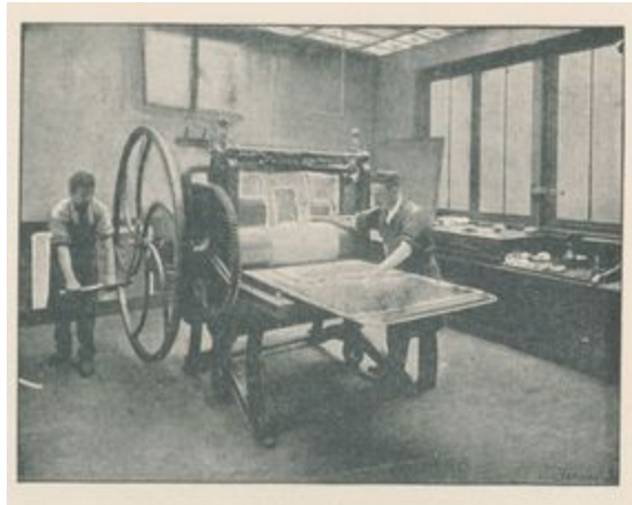
Une presse en taille-douce Imprimerie Wittmann
