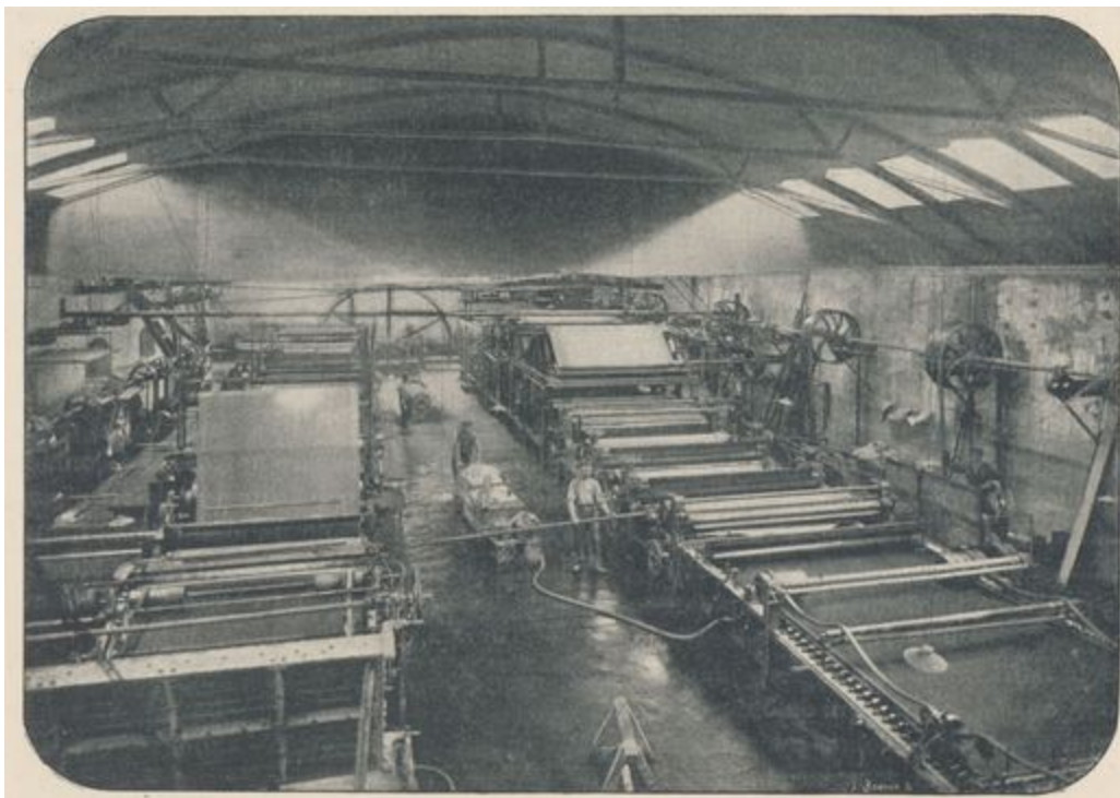
Atelier des machines à fabriquer le papier Papeterie de La Haye-Descartes
