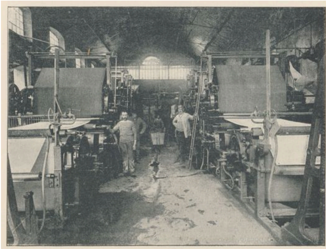
Machines à fabriquer le papier Usine Firmin-Didot
