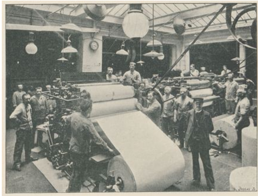
Les Machines rotatives du « Petit Journal »
