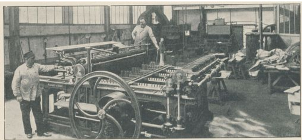
Machine à imprimer les billets de banque Ateliers Alauzet & Tiquet
