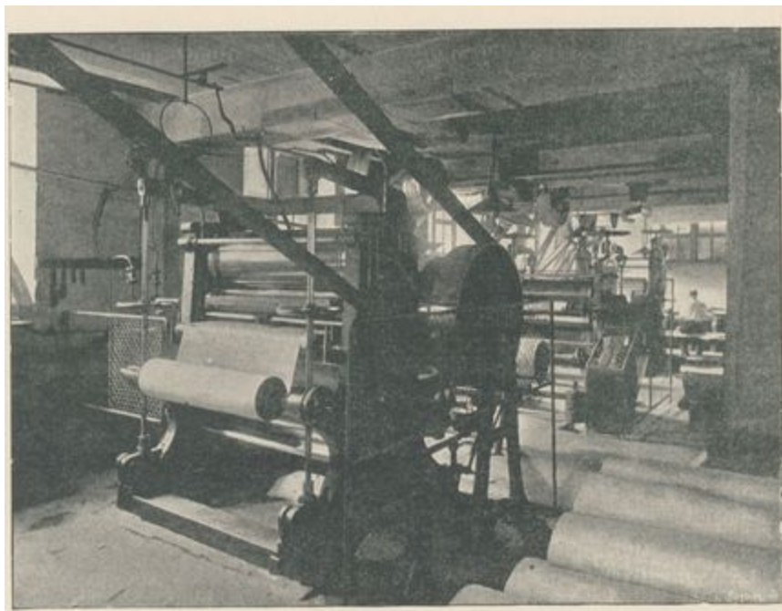
Fabrication du papier de fantaisie Atelier des calandres. Usine Vacquerel
