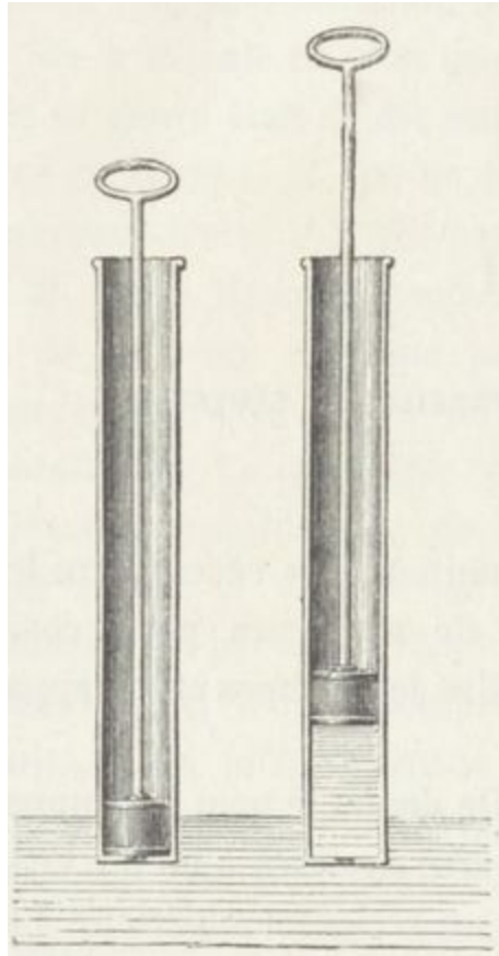
Fig. 19. — Principe de la pompe.
