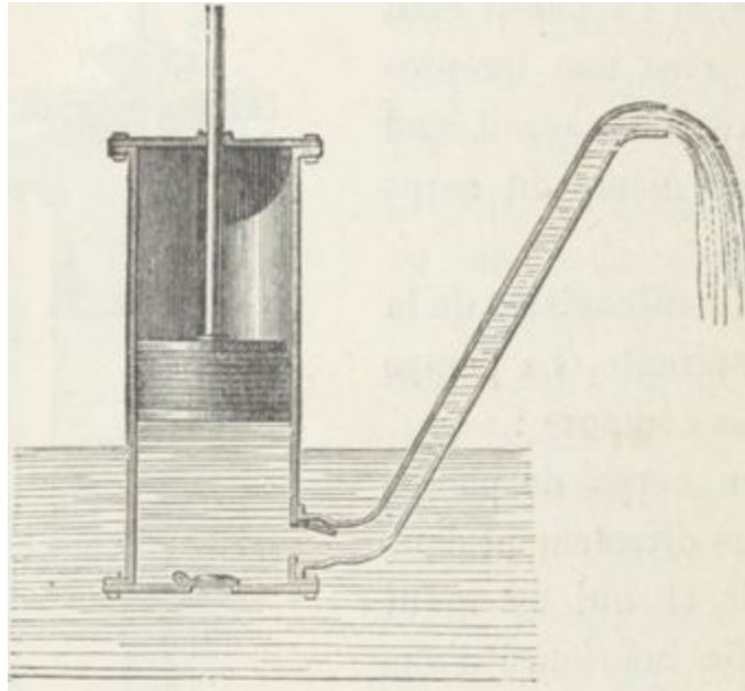
Fig. 21. — Pompe foulante.
