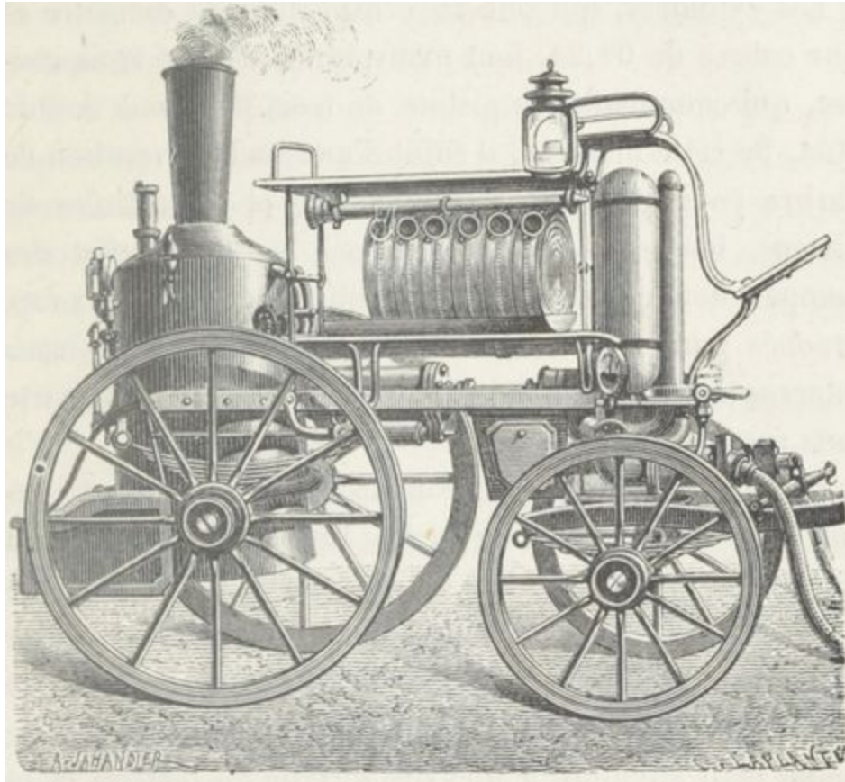
Fig. 26. — Pompe à incendie à vapeur.
