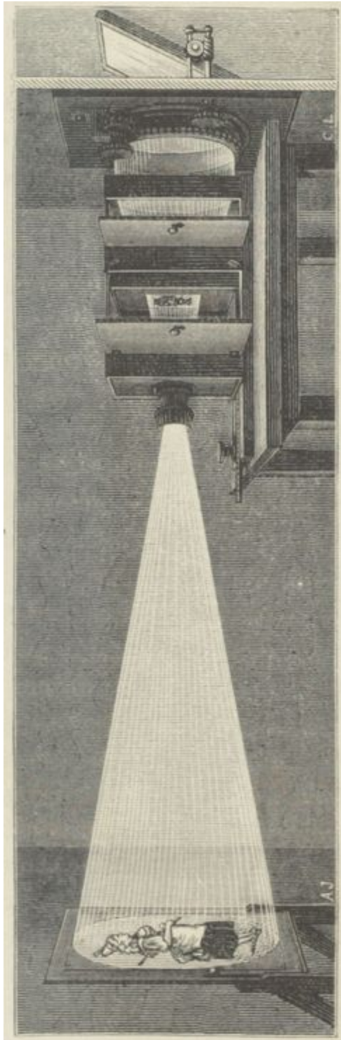
Fig.32 – Appareil d’agrandissement de M. Monckhoven.
