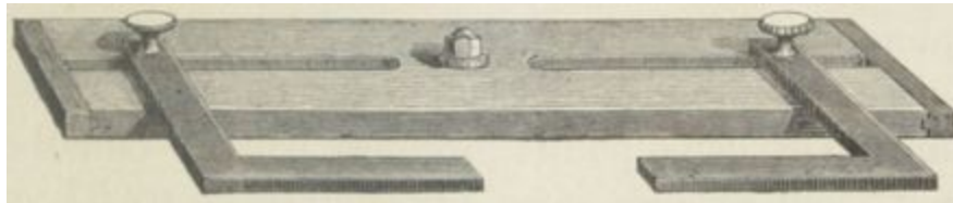
Fig. 62. — Planchette de la chambre noire pour la prise des vues stéréoscopiques.
