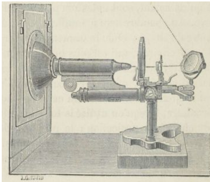
Fig. 38. — Microscope incliné adapté à la chambre noire.
