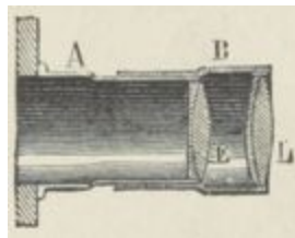
Fig. 13. — Détail de l'objectif.
