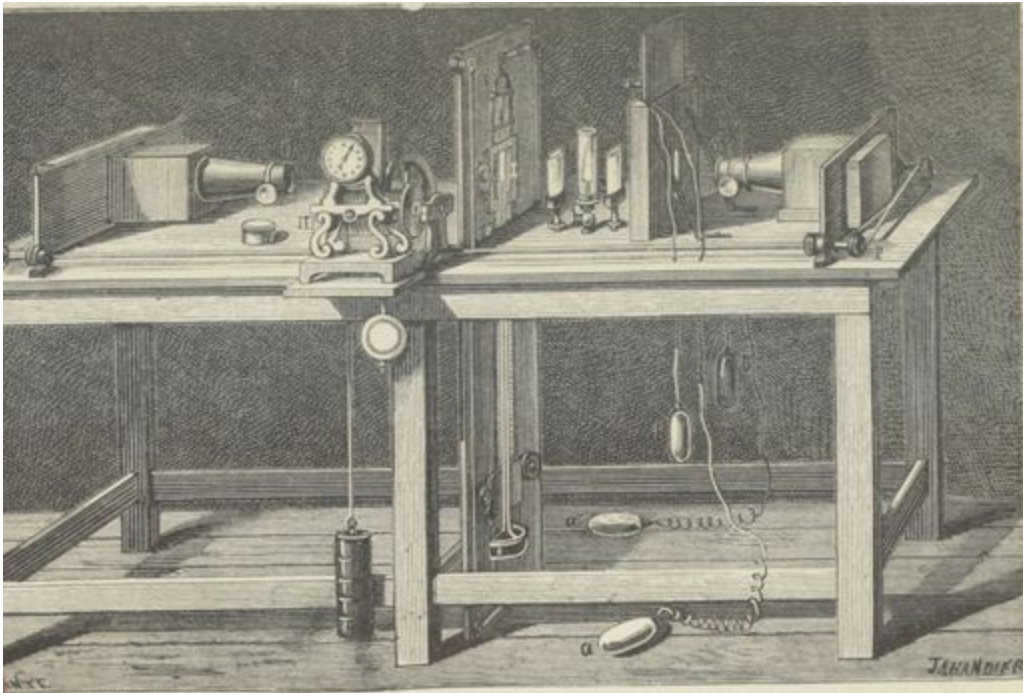
Fig. 55. — Barométrographe et thermométrographe photographiques de M. Salleron.
