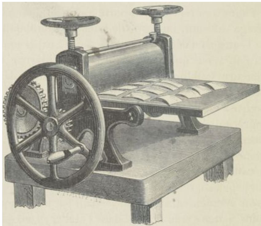
Fig. 29. — Presse à satiner les épreuves positives.
