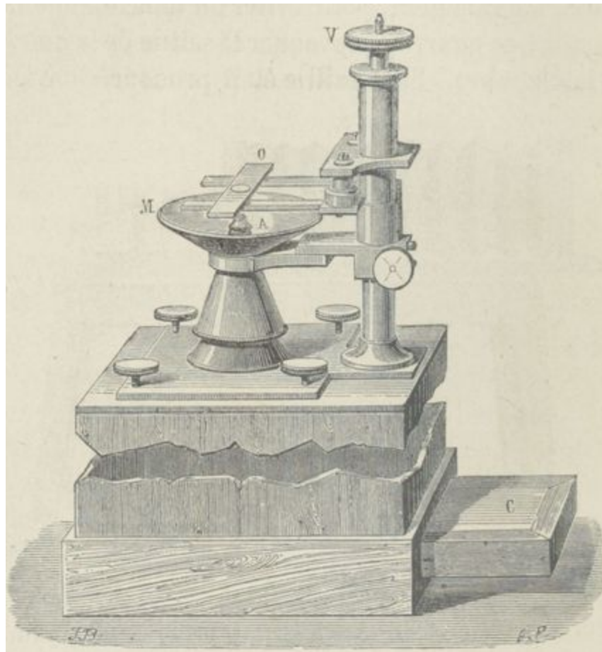
Fig. 40. — Microscope vertical adapté à la chambre noire pour la photomicrographie.
