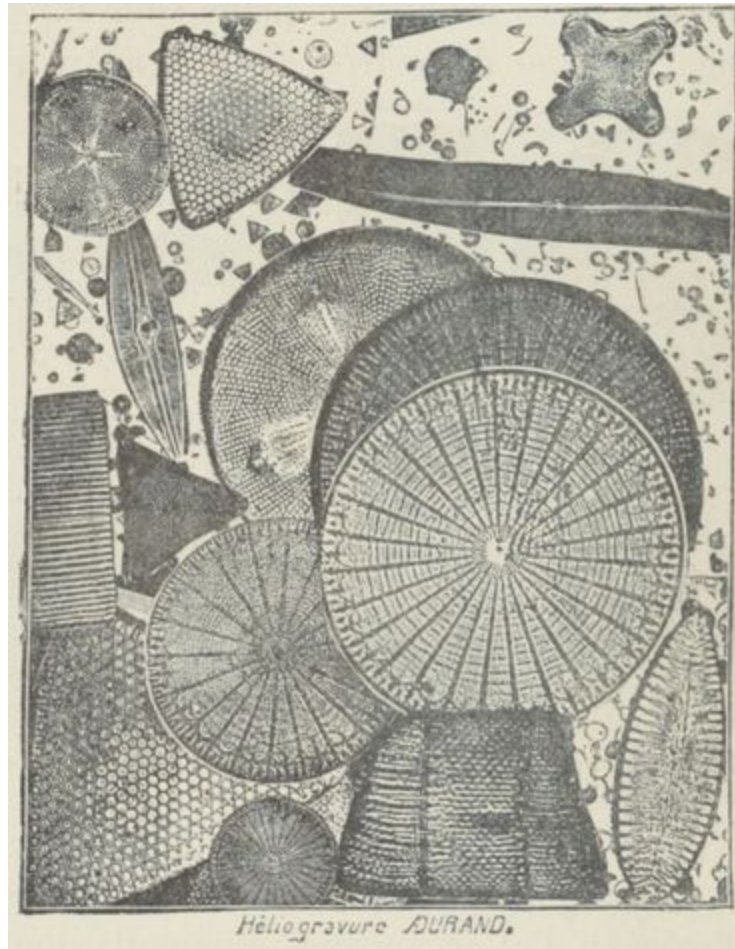
Fig. 45. — Diatomées groupées.
