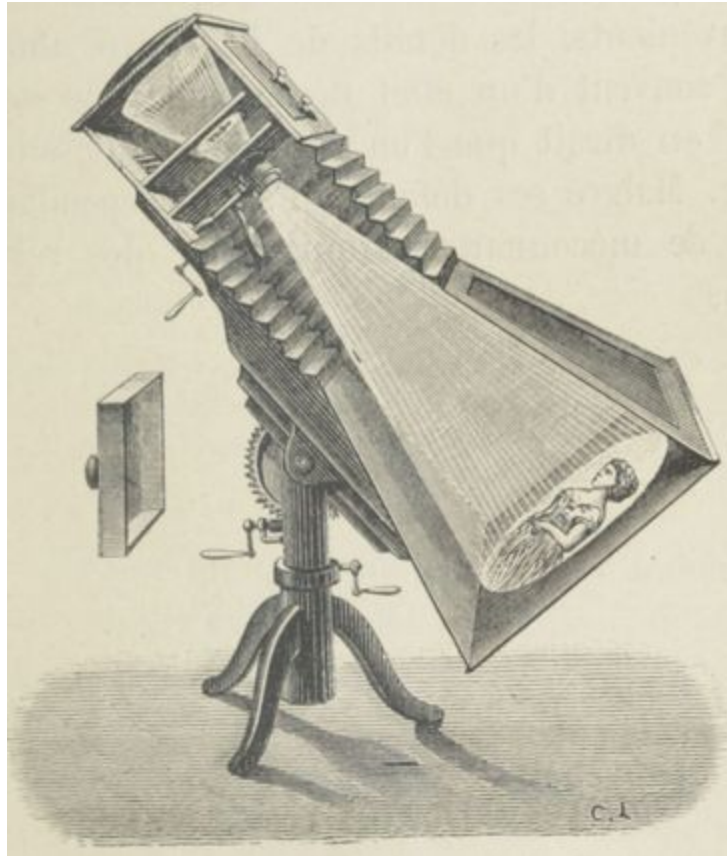
Fig. 33. — Chambre solaire universelle.
