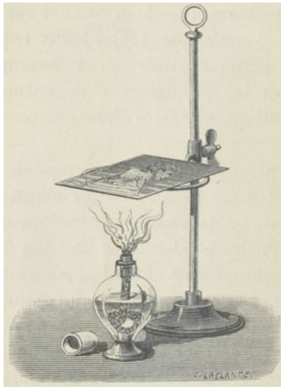
Fig. 8. — Dorure de la plaque daguerrienne.
