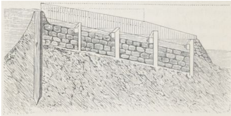
Coupe d'une échelle pour poissons migrateurs.
