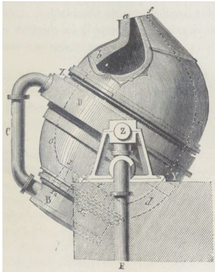
Convertisseur Bessemer.
