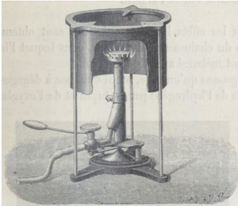
Fourneau à gaz des laboratoires.
