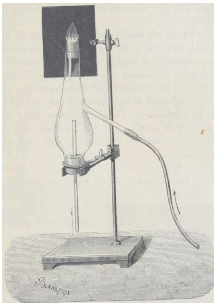
Appareil à renversement de la flamme.
