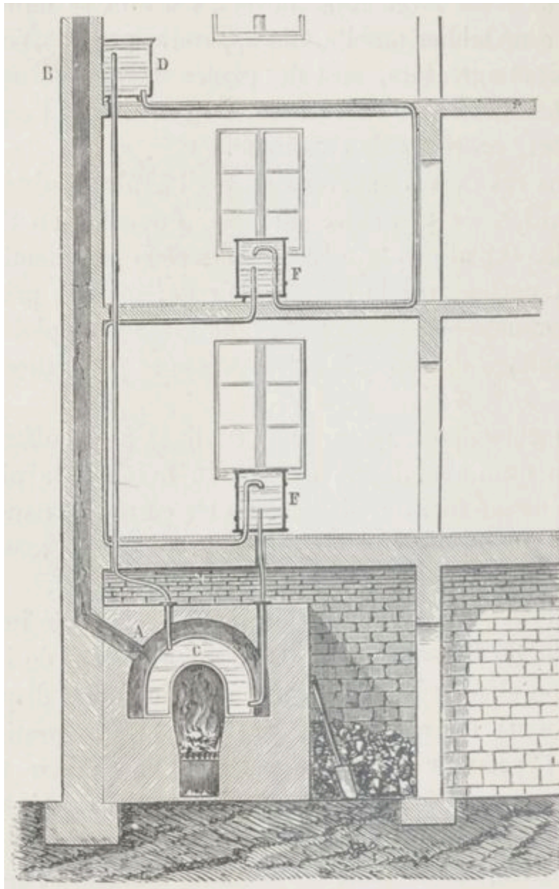
Calorifère à eau chaude.
