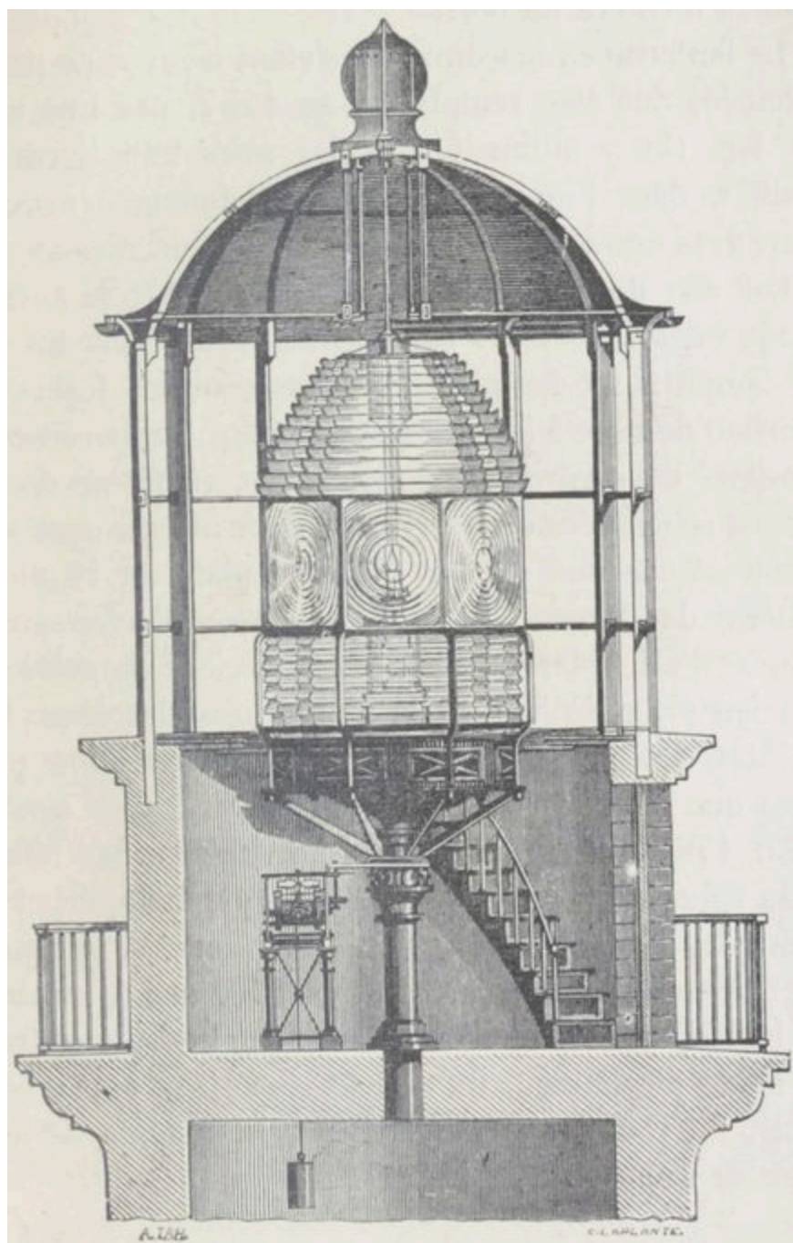
Lanterne d'un phare à réfraction.
