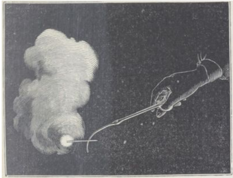
Combustion du magnésium dans l'air.
