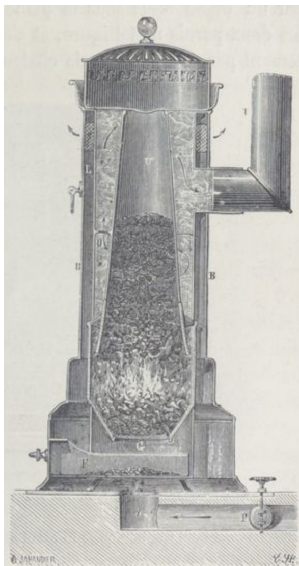
Poêle calorifère et ventilateur.
