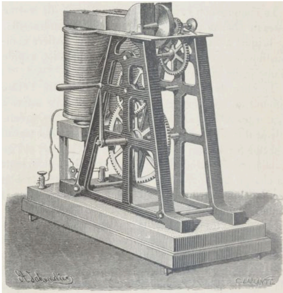
Électro-aimant de Foucault.
