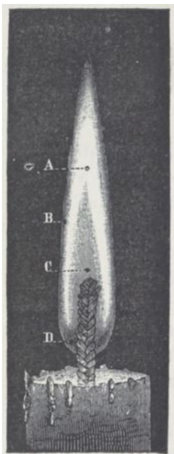
Intérieur de la flamme d'une bougie
