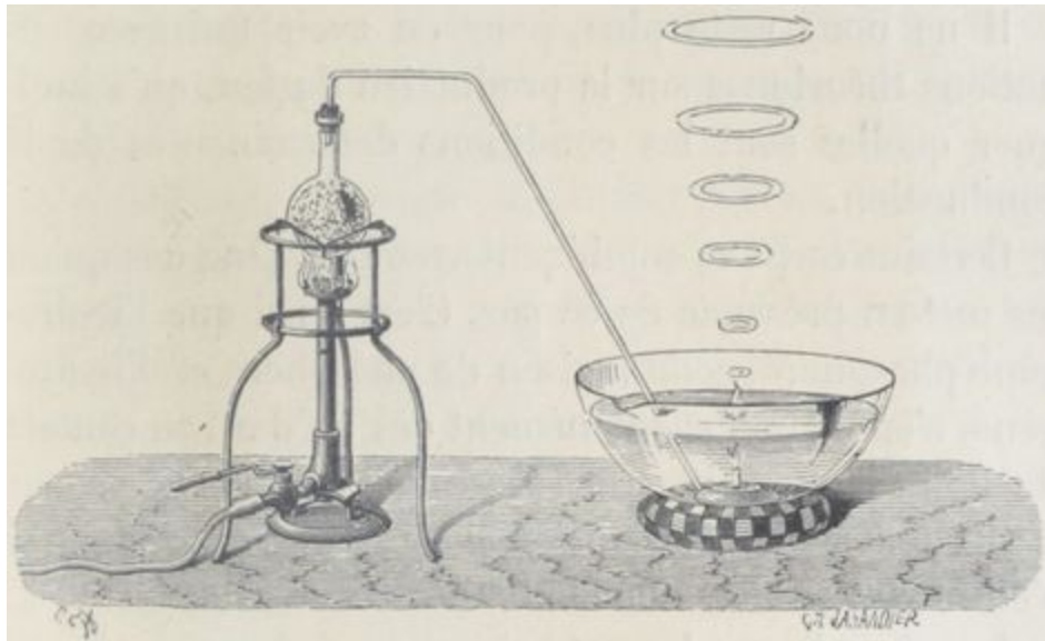
Inflammation spontanée de l'hydrogène phosphore.
