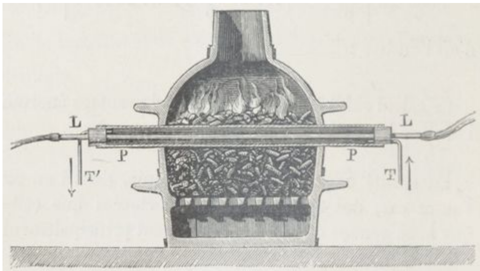
Dissociation de l'eau.
