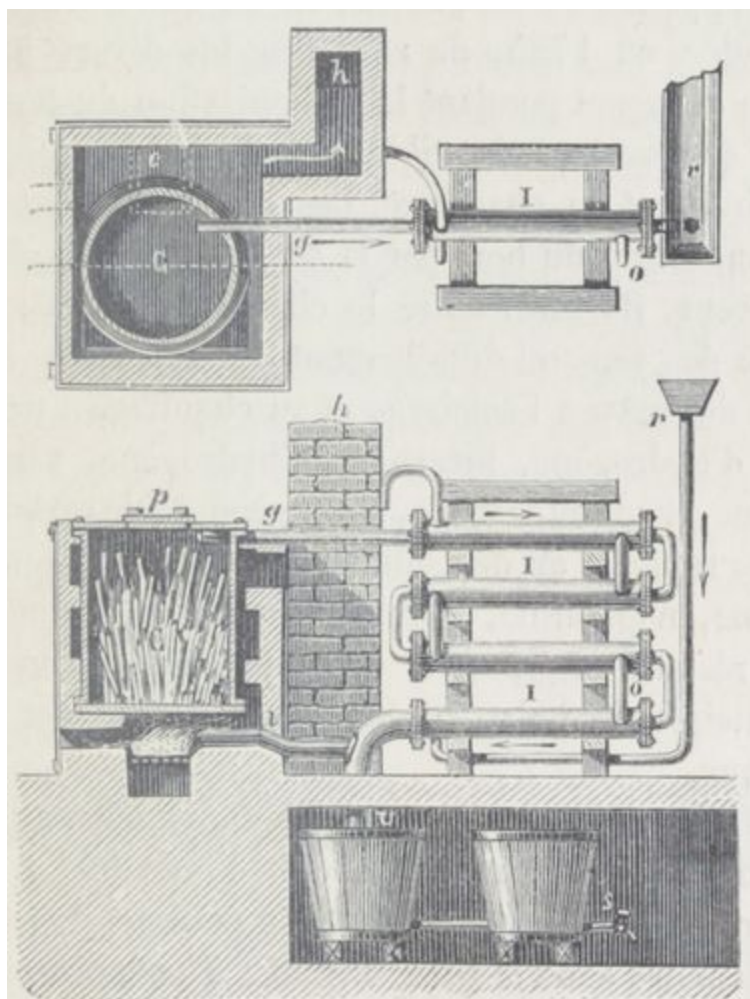
Distillation du bois en vase clos.
