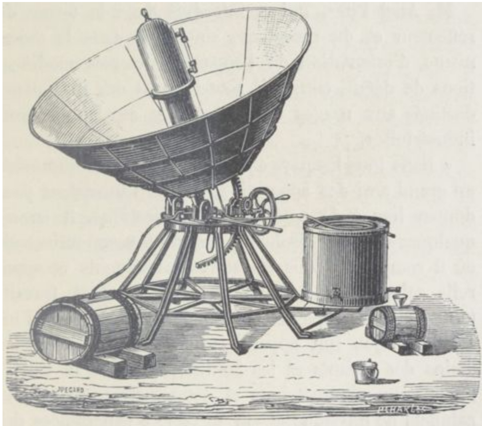
Appareil Mouchot.
