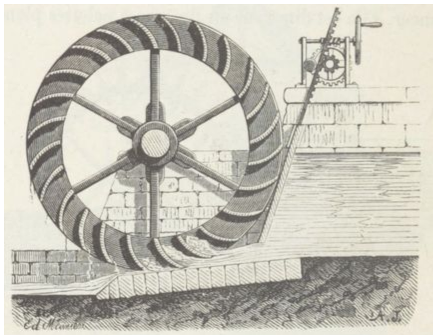
Fig. 19. — Roue Poncelet à palettes courbes.
