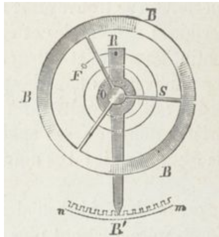
Fig. 24. — Ressort.
