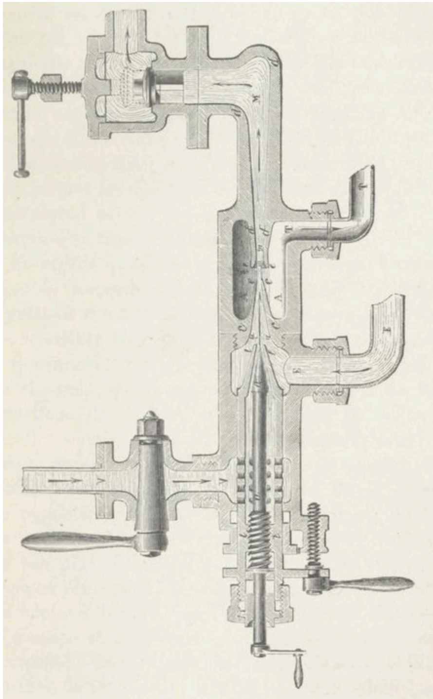
Fig. 58. — Coupe de l'injecteur Giffard.
