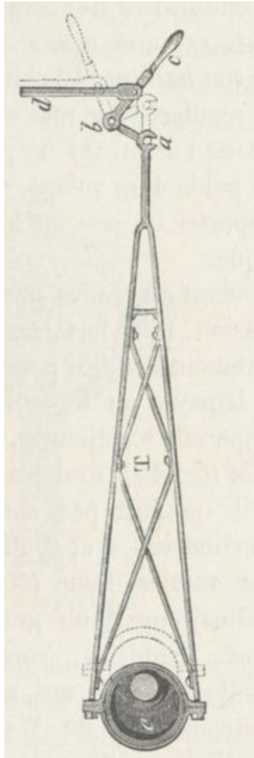
Fig. 49. Tige-bielle d'excentrique.
