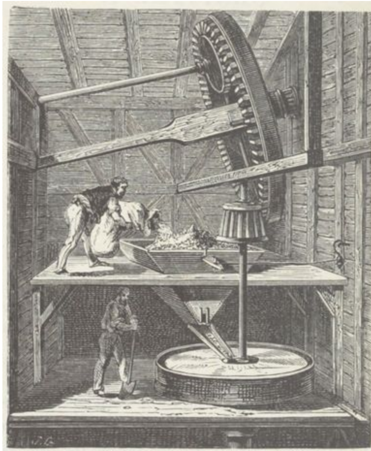
Fig. 8. — Intérieur d'un moulin à vent.
