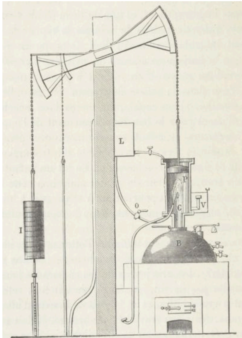
Fig. 40. — Machine de Newcomen.
