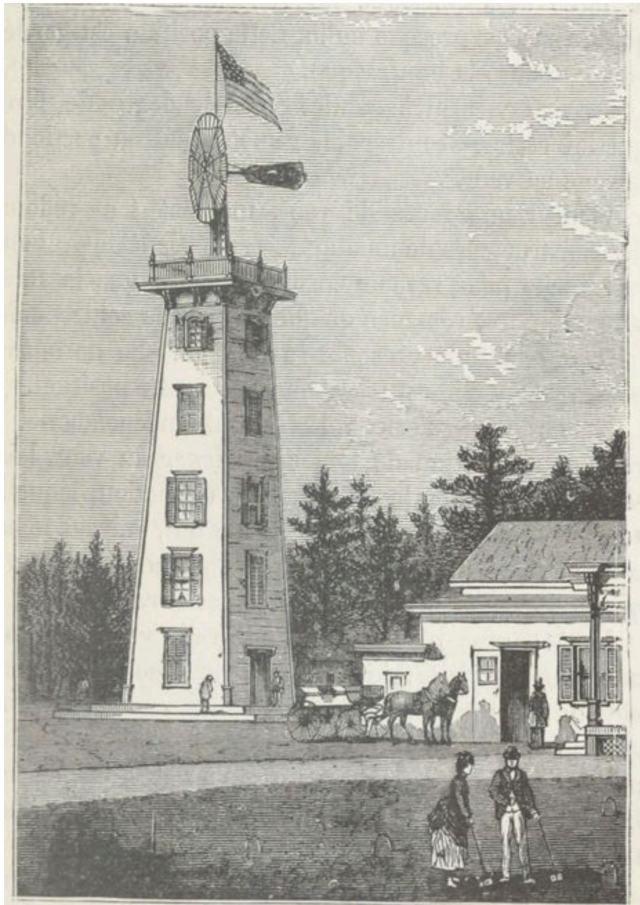
Fig. 10. — Moulin automoteur l'Éclipse.
