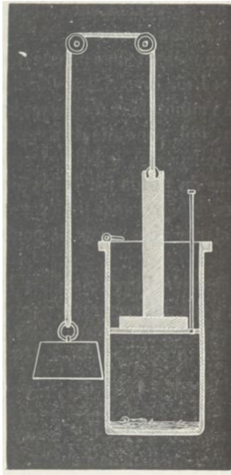
Fig. 29. — 1 re machine de Papin.
