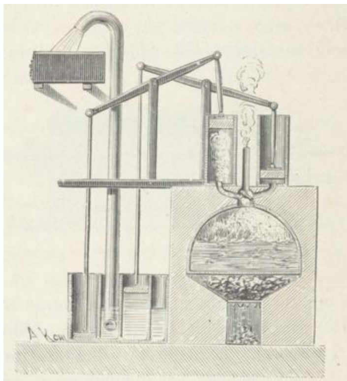
Fig. 43. — Machine de Leupold.
