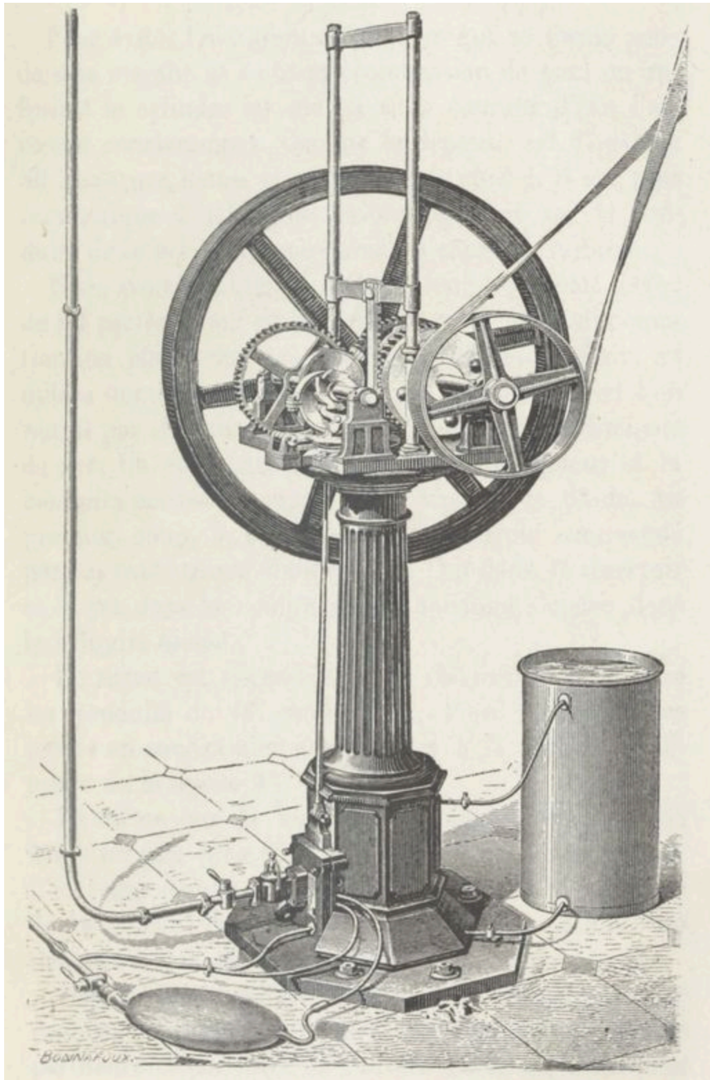
Fig. 97. — Moteur a gaz Otto el Laugu.
