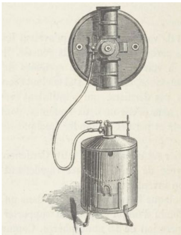
Fig. 106. — Moteur à ammoniac Cordenons.
