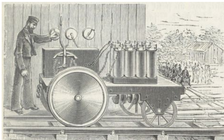
Fig. 94. — Locomotive électrique au repos en charge.
