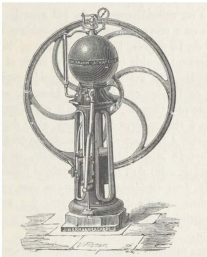
Fig. 102. — Saturateur pour boissons gazeuses.
