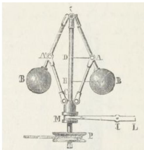
Fig. 57. — Modérateur de Watt à force centrifuge.
