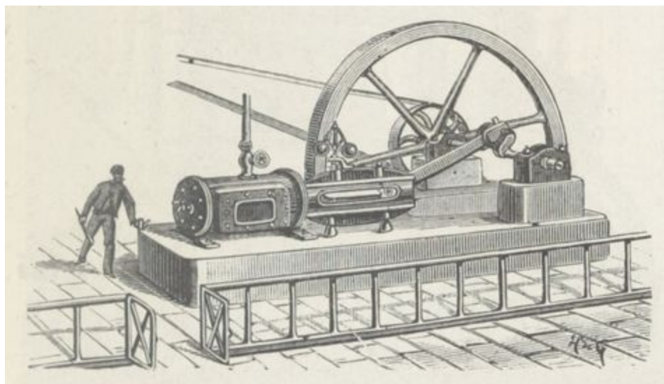
Fig. 80. — Machine d'atelier Farcot.
