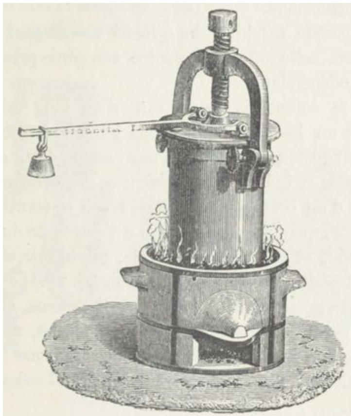
Fig. 37. — Le « New Digester » du docteur Papin.
