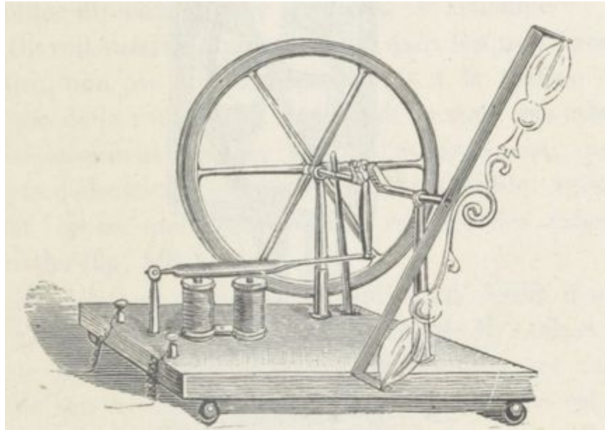
Fig. 88. — Moteur Loiseau.
