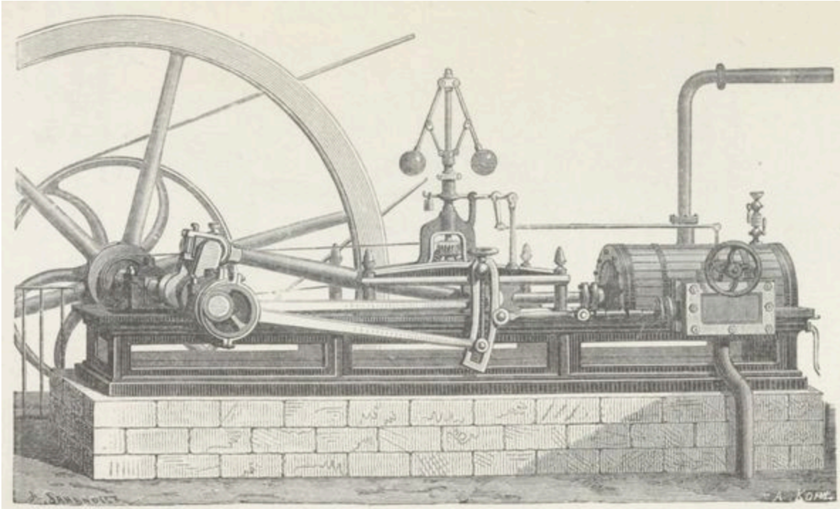
Fig. 69. — Machine à vapeur horizontale munie de la coulisse de Stephenson.
