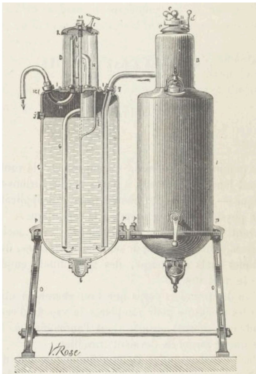
Fig. 100. — Appareil pour boissons gazeuses ; producteur et épurateur.
