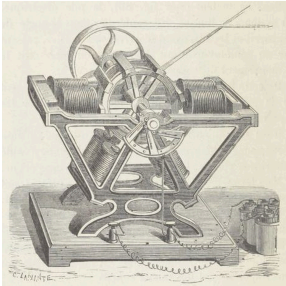
Fig. 87. — Moteur Froment (Dessus enlevé).
