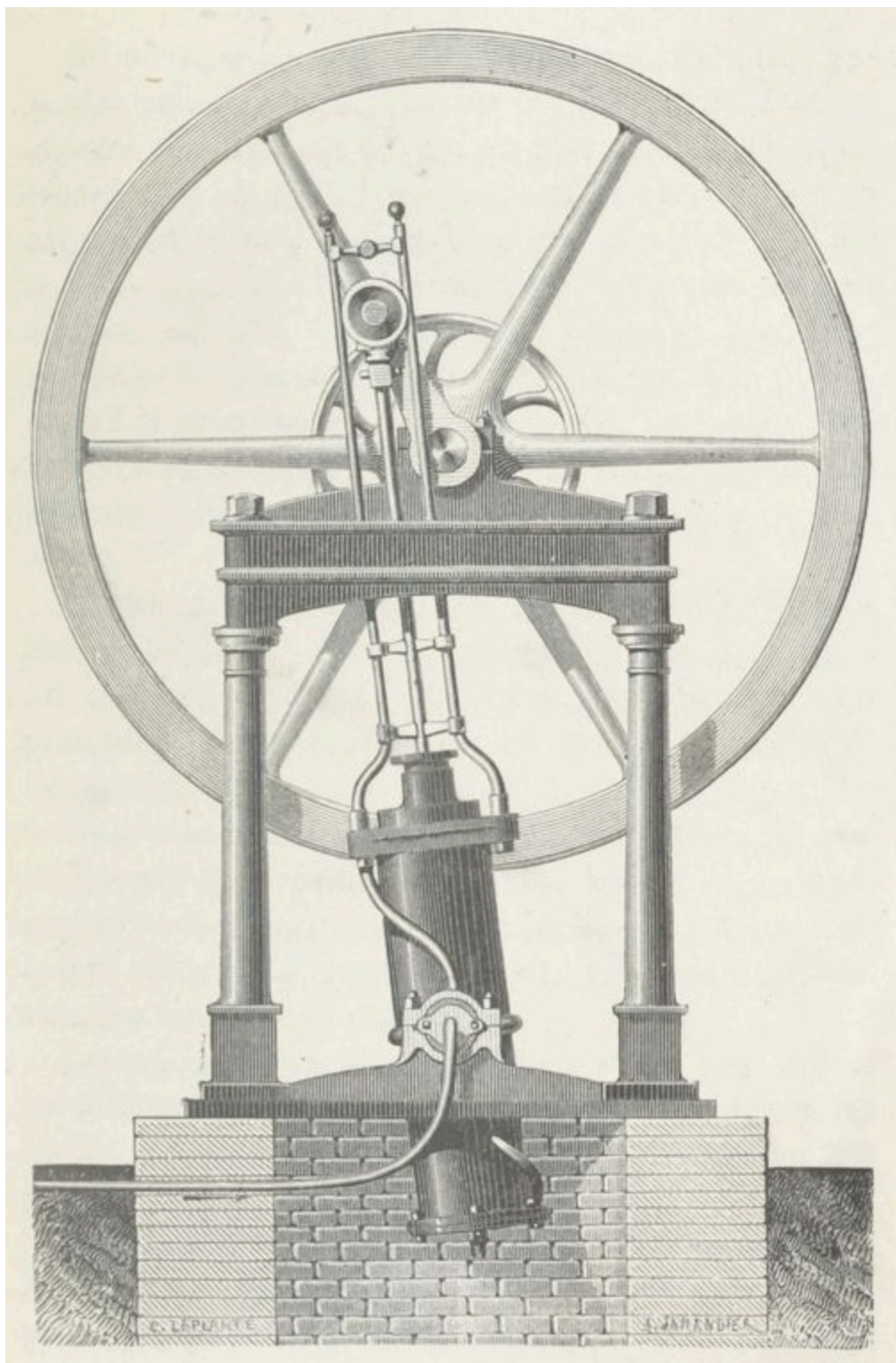
Fig. 64. — Machine à cylindre oscillant Cavé.
