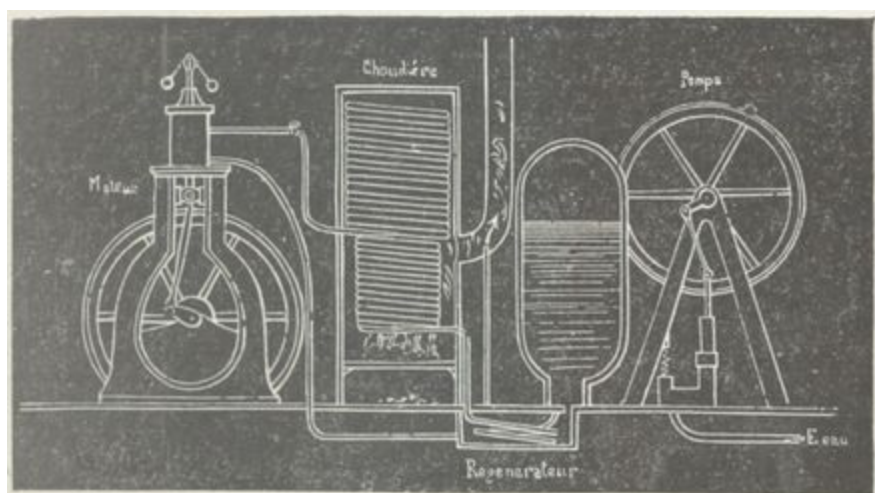
Fig. 68. — Diagramme du moteur Tyson.
