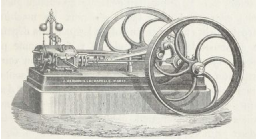
Fig. 59. — Machine horizontale à deux volants.
