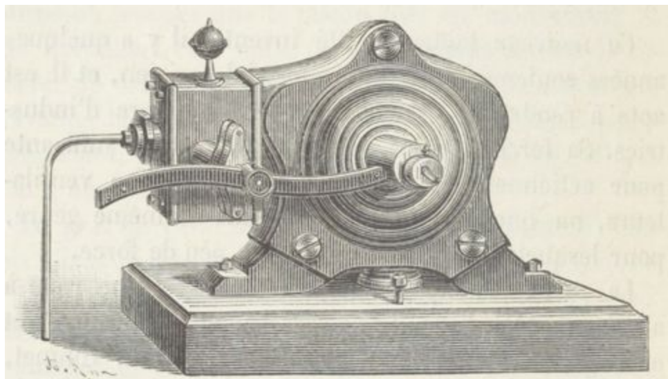
Fig. 22. — Moteur Dufort.
