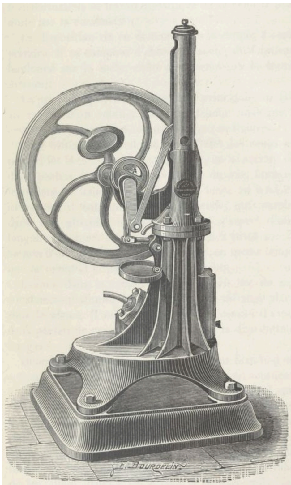
Fig. 99. — Moteur à gaz Bisschop.
