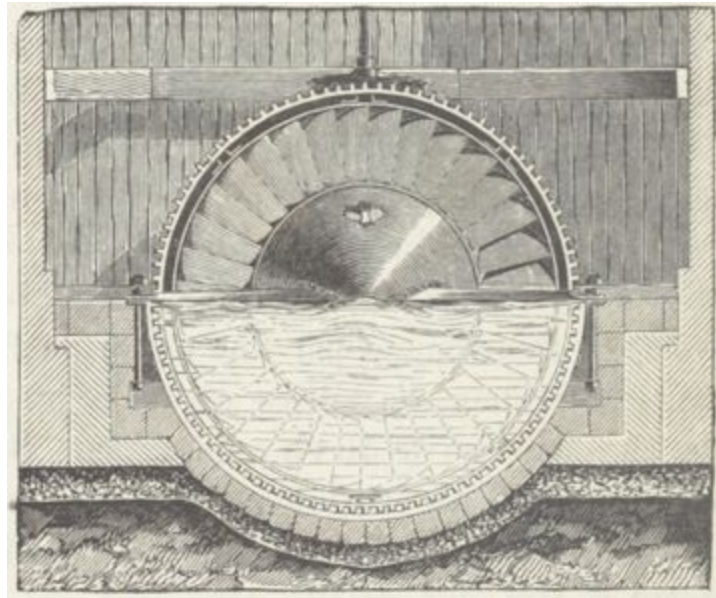
Fig. 21. — Roue hélice Girard.
