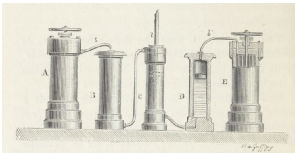
Fig. 103. — Machine de Brunel.
