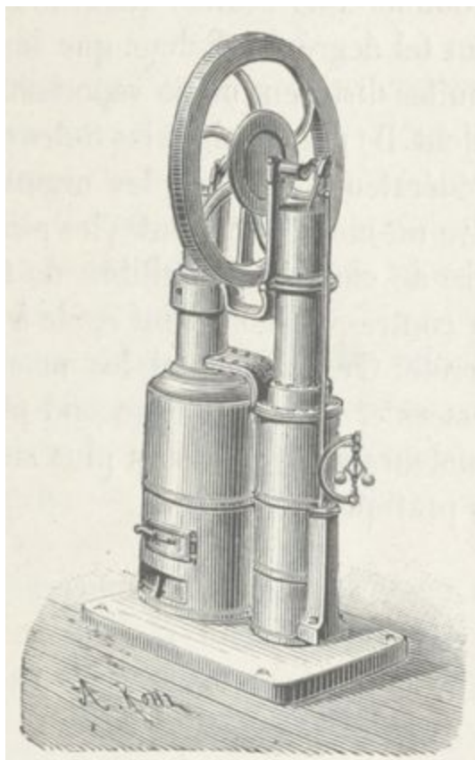
Fig. 32. — Machine Daulton.
