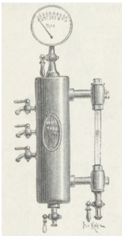
Fig. 56. — Porte-tube séparateur Damourette.
