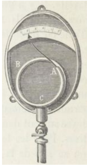
Fig. 54. — Manomètre métallique Bourdon.
