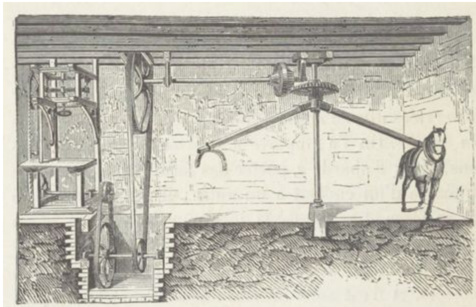
Fig. 3. — Scie à ruban.
