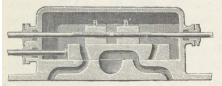
Fig. 42. — Détente Meyer.
