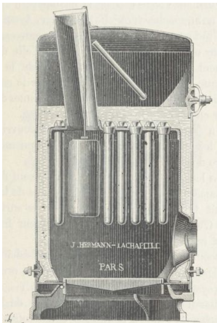
Fig. 45. — Coupe de la chaudière Field.
