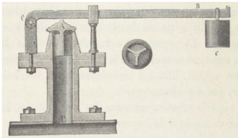
Fig. 51. — Soupape de Papin.
