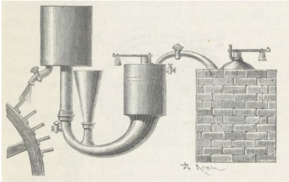
Fig. 38. — 2 e Machine de Papin.
