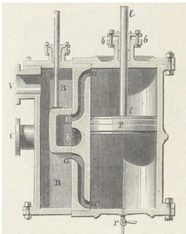
Fig. 47. — Tiroir à coquille.
