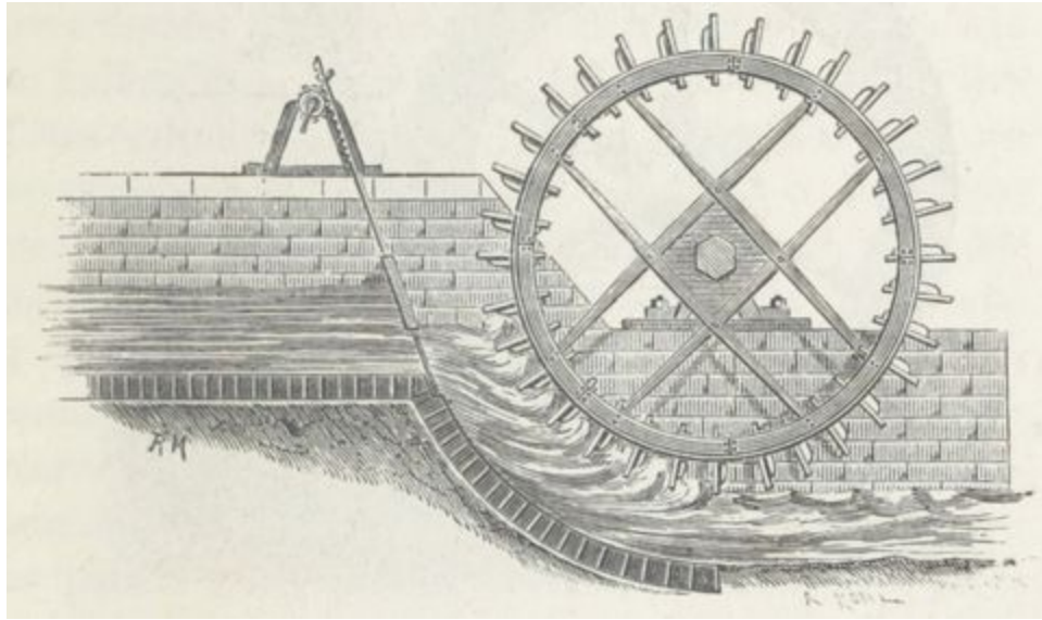
Fig.18. — Roue hydraulique à coursier circulaire.
