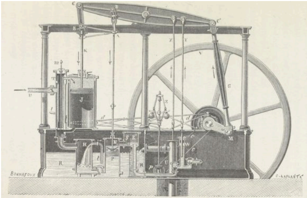
Fig. 11. — Machine de Watt.
