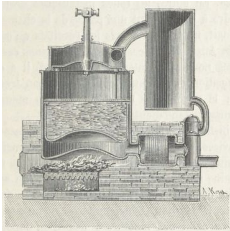
Fig. 30. — Moteur à air chaud d'Ericcson.
