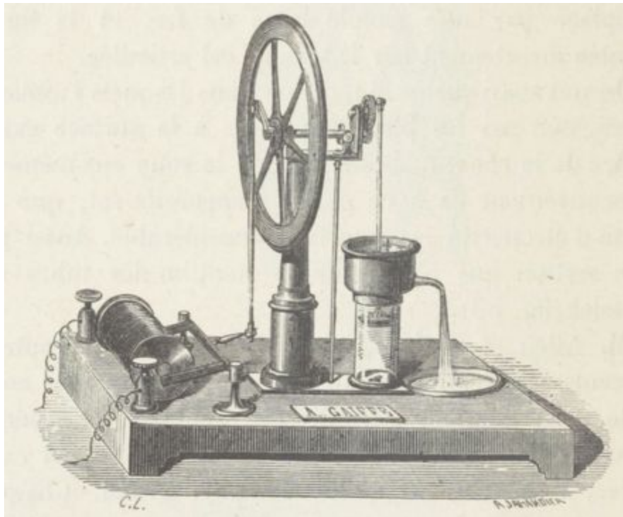
Fig. 90. Moteur électrique de M. Gaiffe.
