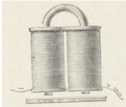
Fig. 84. — Électro-aimant en fer à cheval.
