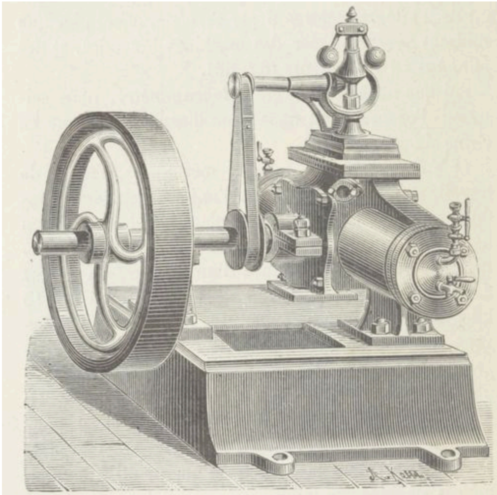
Fig. 70. — Moteur rationnel.
