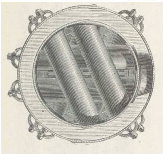
Fig. 46. — Coupe en plan de la chaudière à bouilleurs entre-croisés Hermann-Lachapelle.
