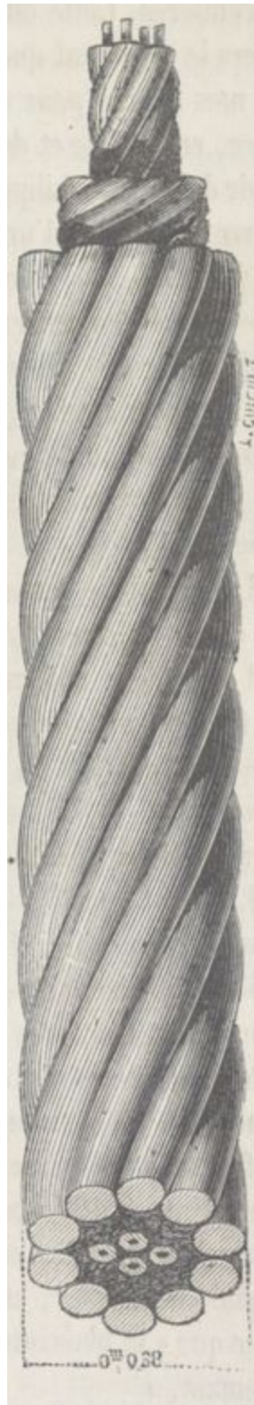
Fig. 38. — Cable de Douvres à Calais (1851).
