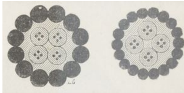
Fig. 96. — Câble de Cagliari à Bône.
