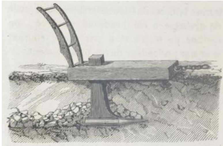
Fig. 213. — Charrue taupe.
