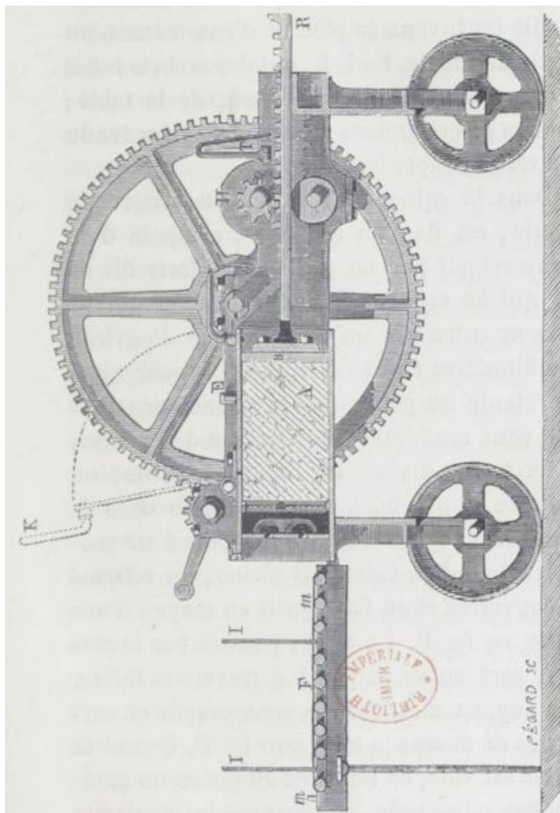
Fig. 33. — Machine de Williams (coupe longitudinale).
