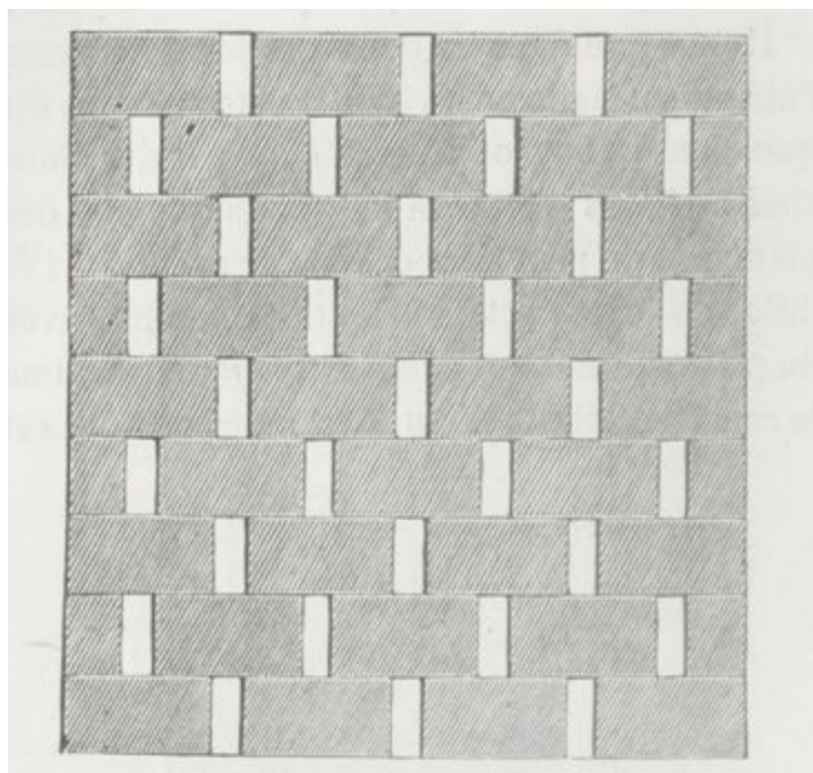
Fig. 67. — Mur à jour pour séchoir avec briques à section de rectangle.
