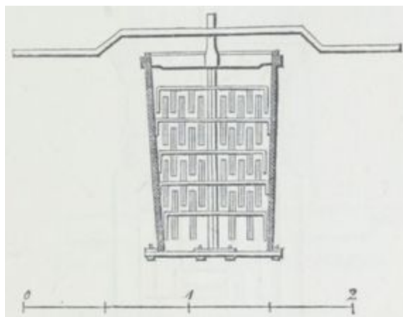
Fig. 14. — Tonneau malaxeur.
