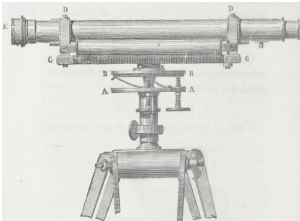
Fig. 118. — Vue de profil du niveau d'Égault.
