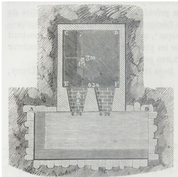
Fig. 94. — Four de M. Vincent (plan).
