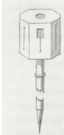
Fig. 108. Équerre d'arpenteur.
