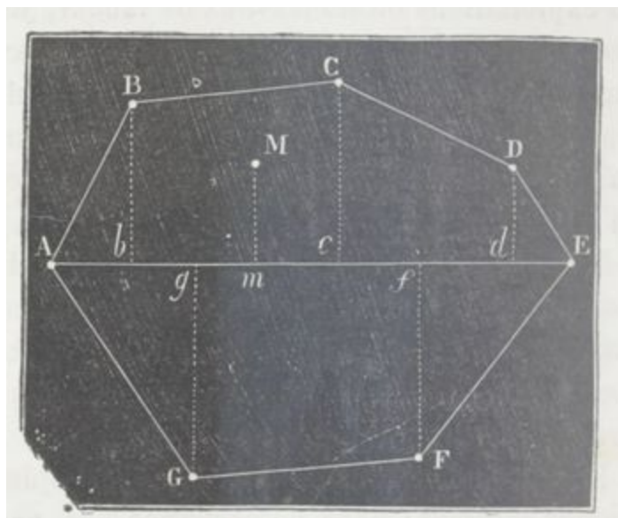
Fig. 104. — Méthode de levé d'un plan.
