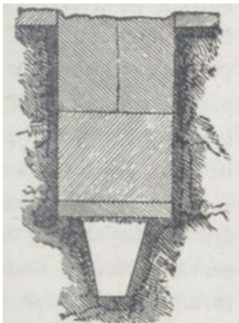
Fig. 208. — Tranchée garnie de tourbe.
