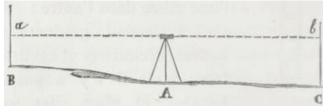
Fig. III. — Nivellement simple.
