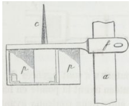
Fig. 10. — Couteau râcleur (élévation).
