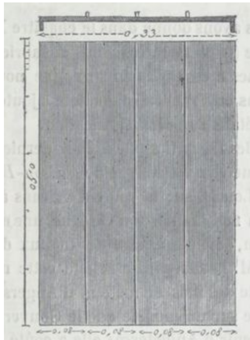
Fig. 87. — Élévation de la planchette à faire les colliers. Fig. 86. — Plan de la planchette à faire les colliers.
