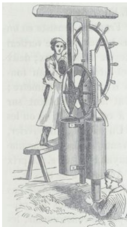
Fig. 53. — Machine d'Exall.
