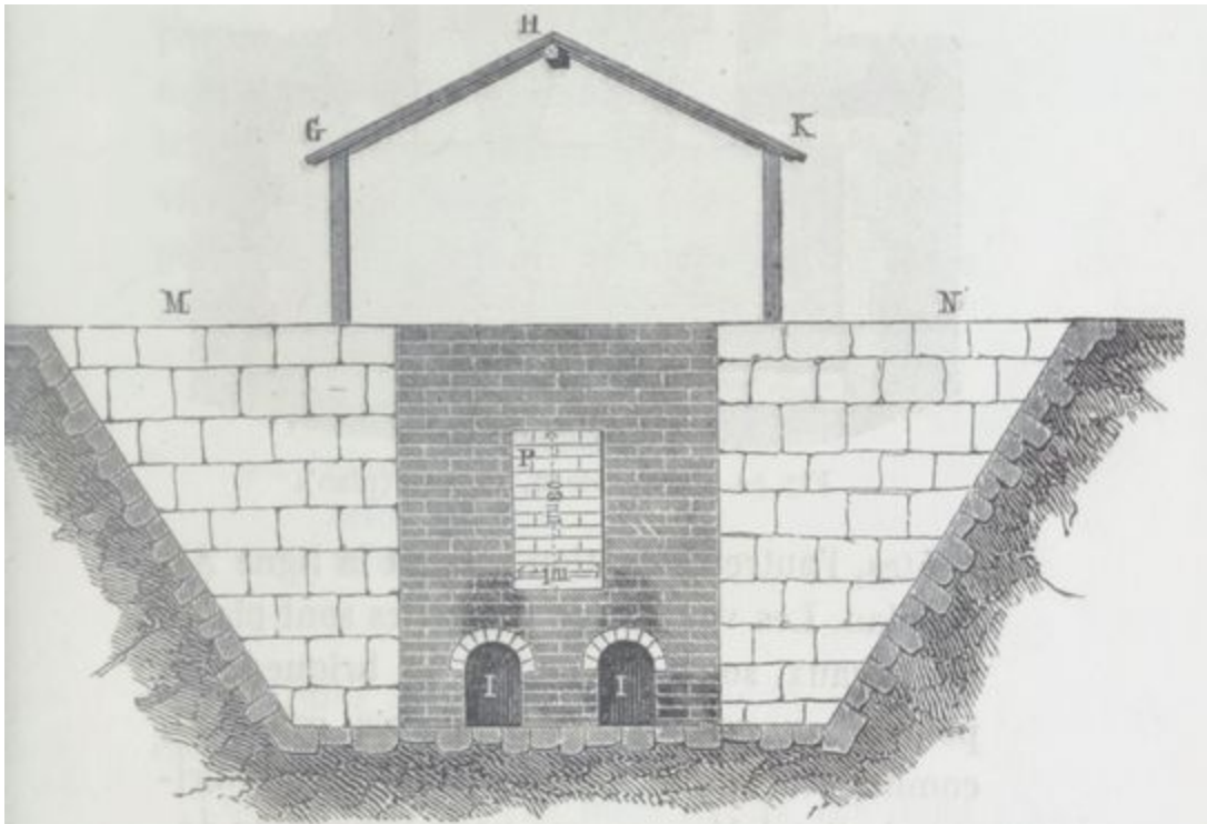
Fig. 93. — Four de M. Vincent (élévation).
