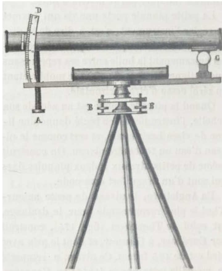
Fig. 175. — Niveau de pente de Thompson.
