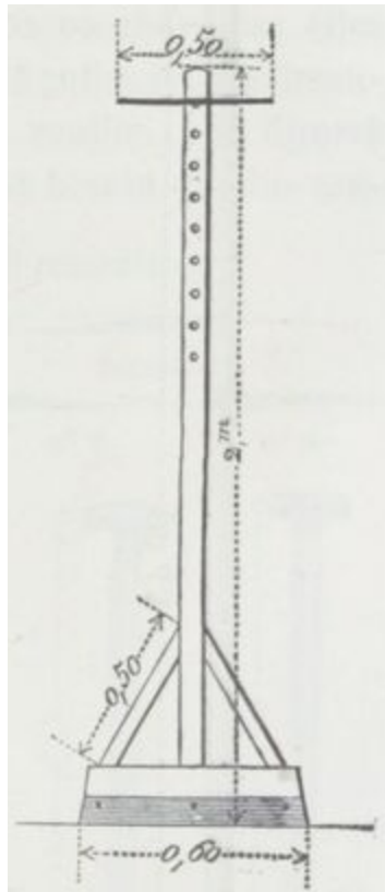
Fig. 153. — Fouloir en bois de M. Laurel.
