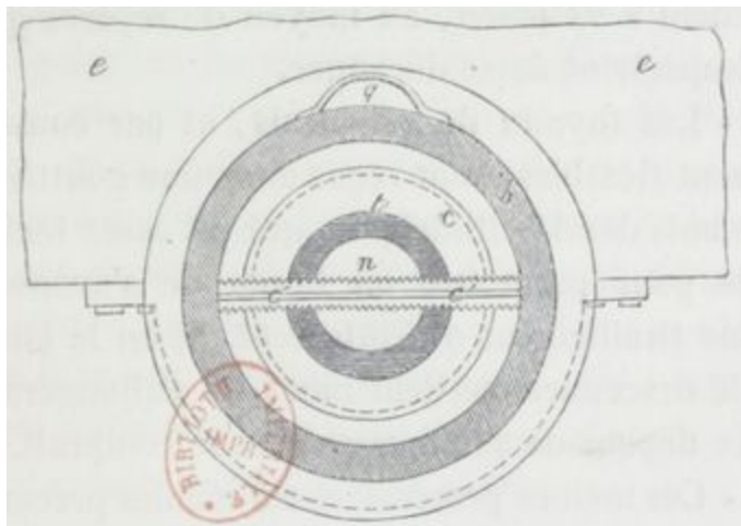
Fig. 27. — Presse à faire les tuyaux (plan).
