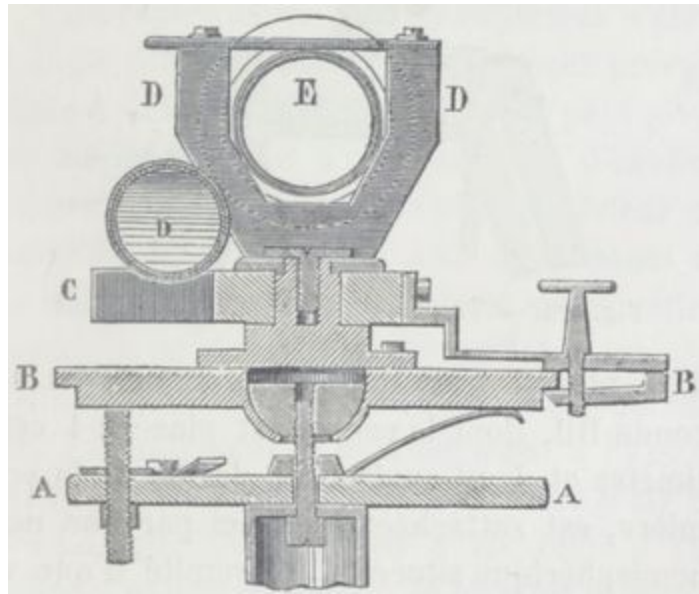
Fig. 117. — Coupe du niveau d'Égault.
