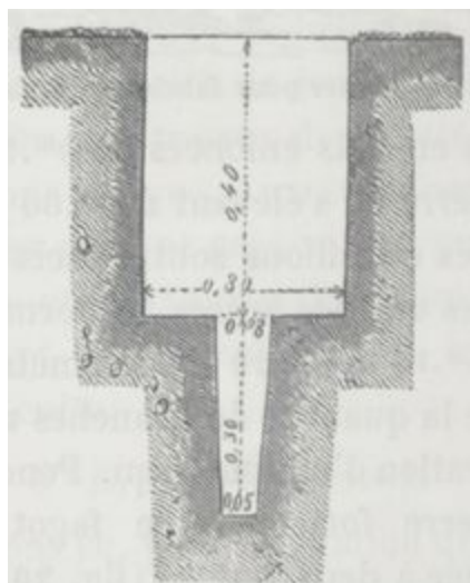
Fig. 205. — Drain disposé pour être garni de fascines.
