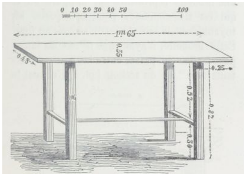
Fig. 82. — Table pour rouler les tuyaux.
