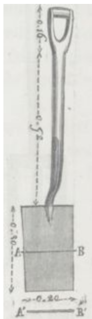
Fig. 139. — Bêche plate à poignée intérieure.
