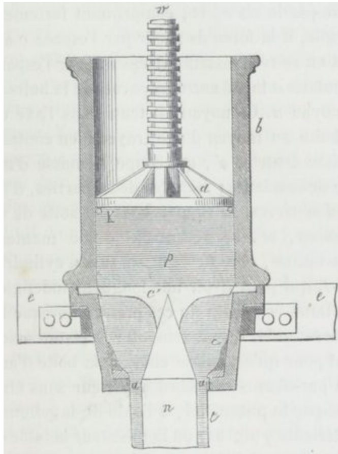
Fig. 26. — Presse à faire les tuyaux de grès (coupe).
