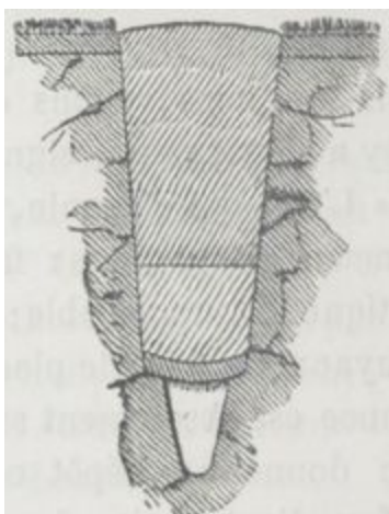
Fig. 207. — Tranchée garnie de gazon.
