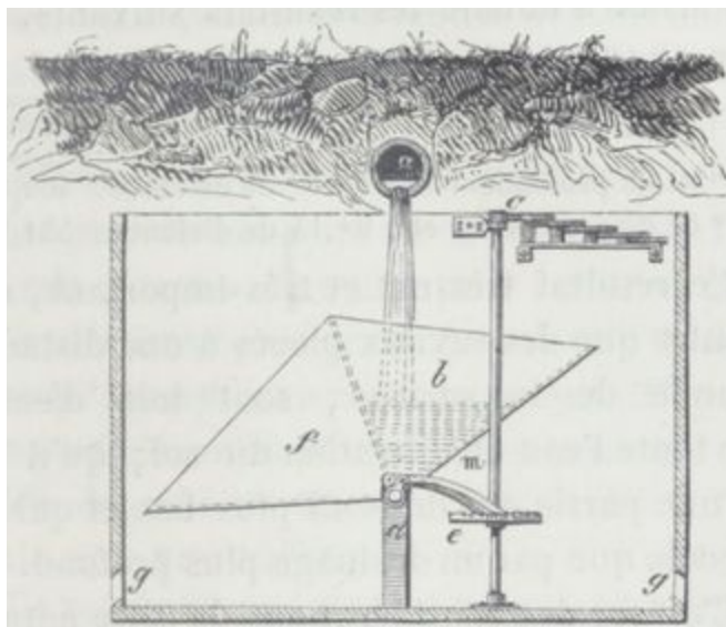
Fig. 225. — Appareil pour jauger l'eau écoulée d'un drainage.
