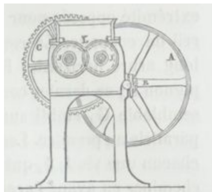
Fig. 57. — Section du cylindre a pétrir de la machine de Randell et Saunders.
