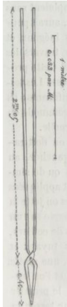
Fig. 183. — Pince en bois pour garnir les joints des tuyaux.
