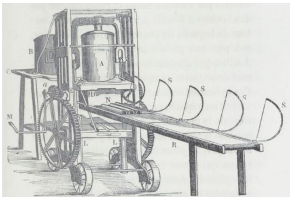
Fig. 20. — Machine verticale de Clayton à décharge horizontale.
