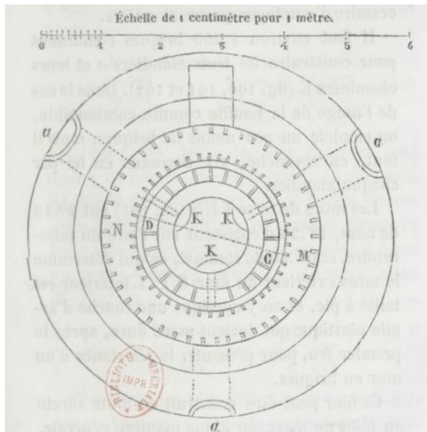
Fig. 102. — Four temporaire en terre (projection sur le plan supérieur,).
