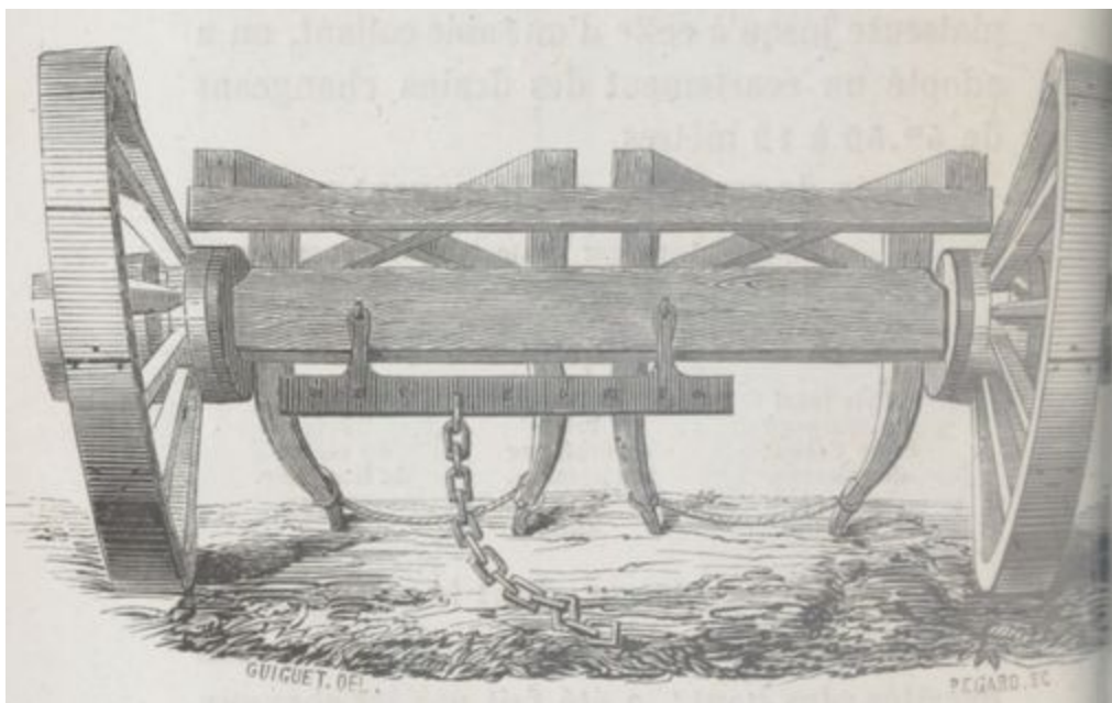
Fig. 217. — Avant-train de la charrue sous-sol.
