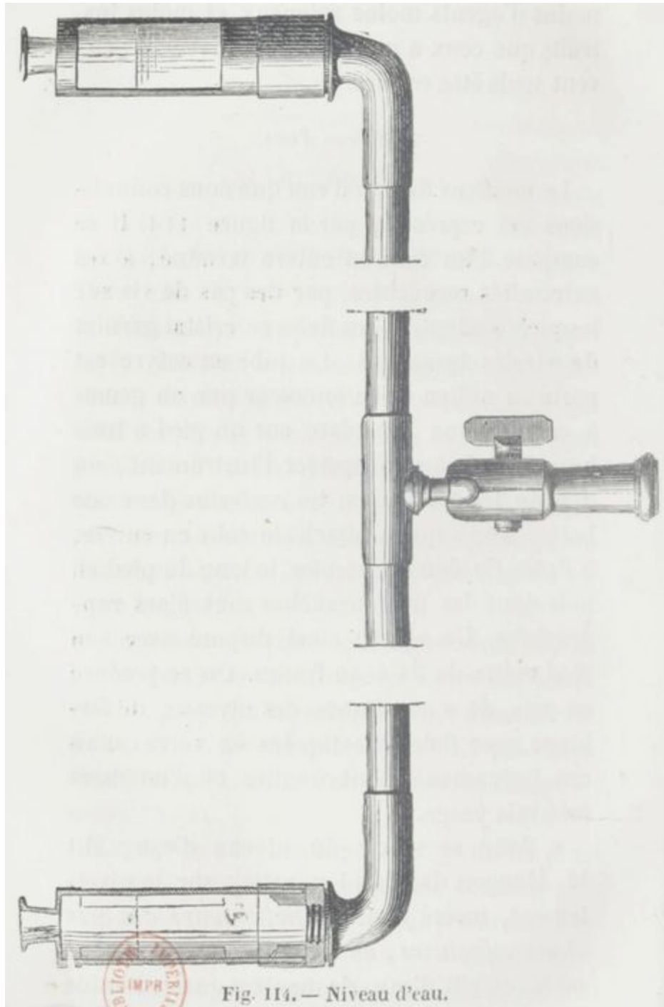
Fig. 114. — Niveau d'eau.
