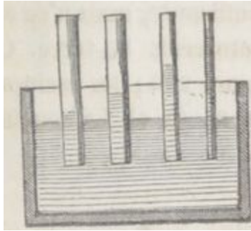
Fig. 219. — Élévation de l'eau par la capillarité.
