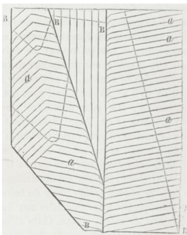
Fig 121. — Plan de drainage avec lignes horizontales de niveau, d'une contenance de 4 hectares.
