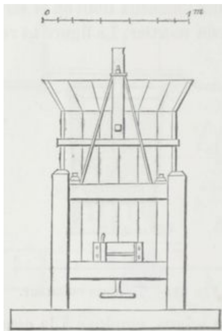
Fig. 15. — Tonneau broyeur élévation).
