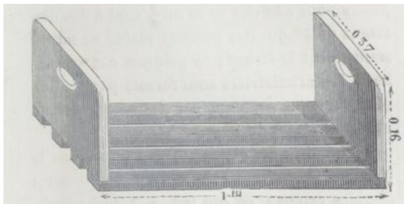
Fig. 64. — Claie pour placer les tuyaux.
