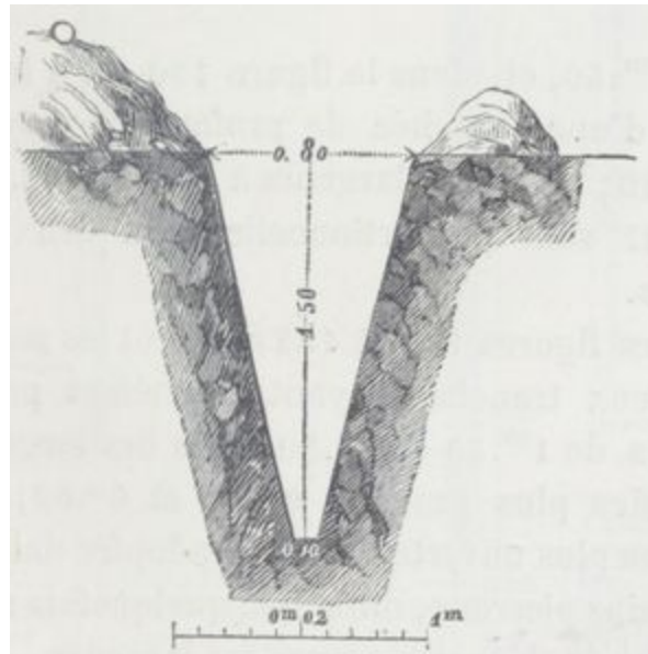
Fig. 131. — Tranchée profonde pour les terrains pierreux.
