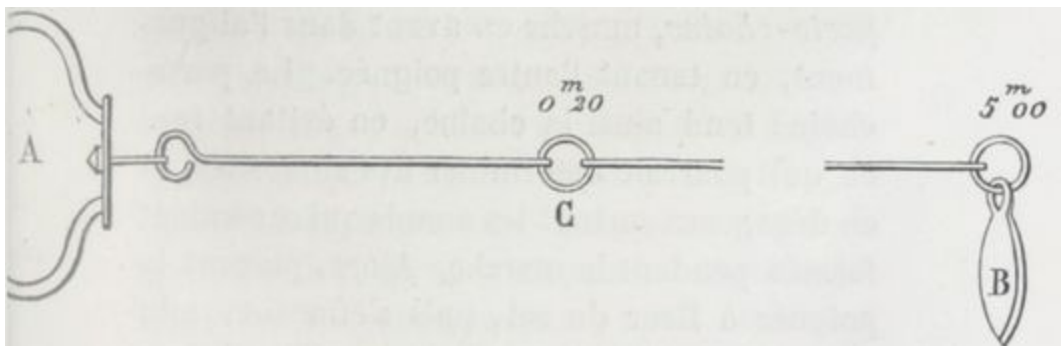
Fig. 105. — Chaîne d'arpenteur.
