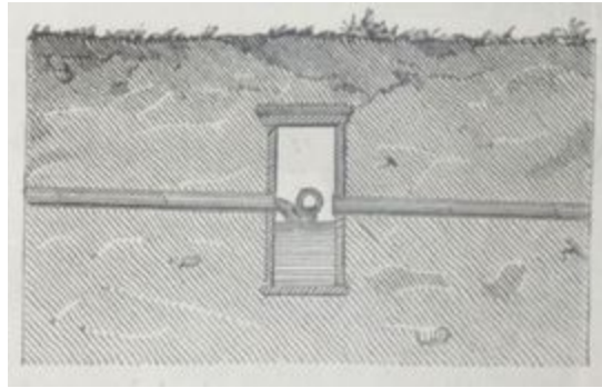
Fig. 187. — Regard pour vérifier le fonctionnement du drainage.
