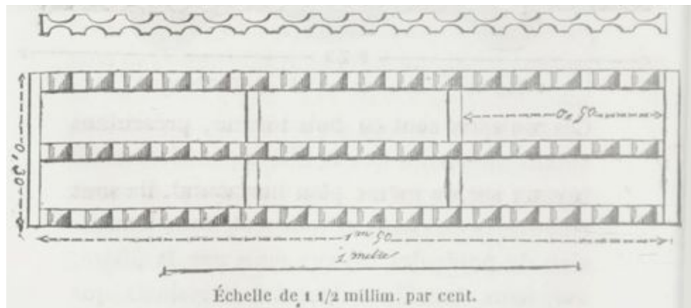
Fig. 80. — Élévation longitudinale d'une claie de M. Vincent. Fig. 81. — Projection horizontale d'une claie de M. Vincent.
