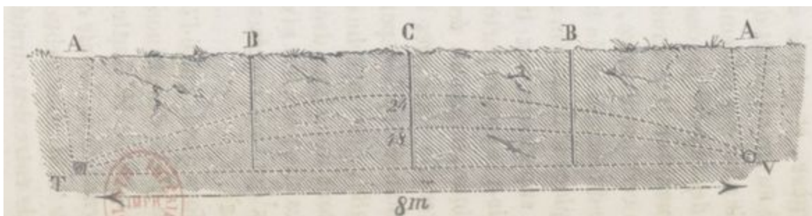
Fig. 231. — Courbes figurant la situation de l'eau dans un terrain drainé à 8 mètres de distance, 24 et 48 heures après une pluie.
