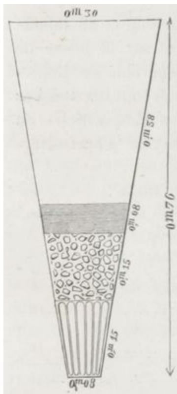
Fig. 215. — Tranchée empierrée ordinaire.
