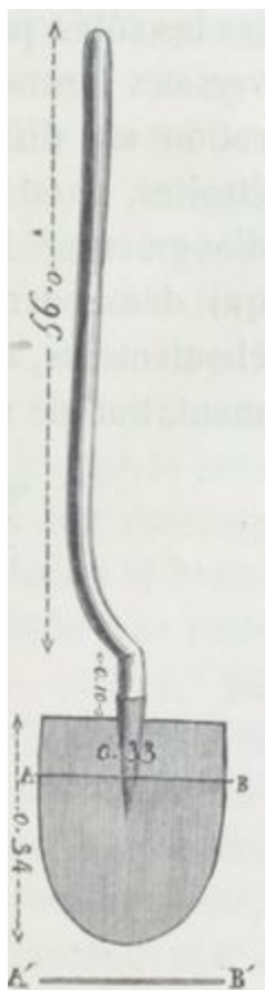
Fig. 164. — Pelle pour déblayer.
