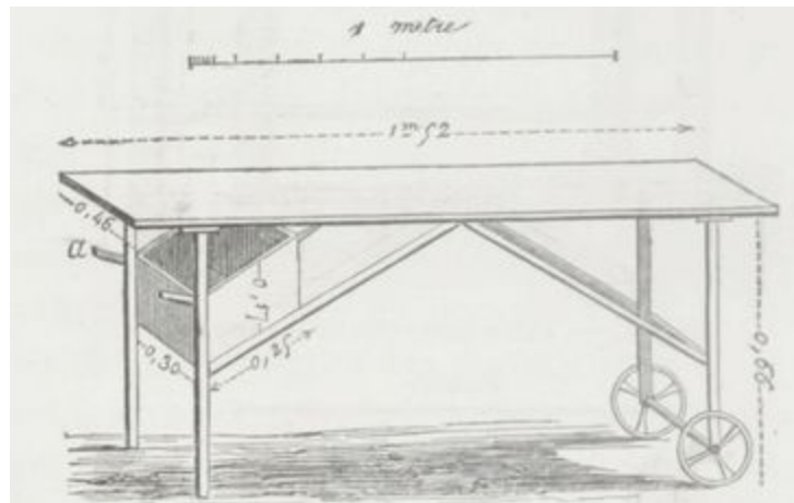
Fig. 84. — Table à roulettes pour rouler les tuyaux.
