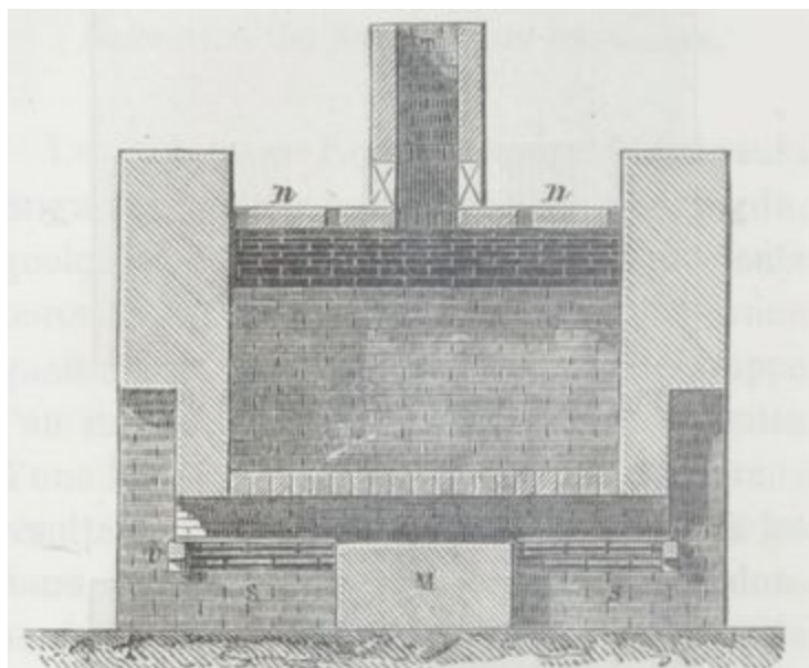
Fig. 32. — Four de Saint-Meuge (coupe suivant la ligne yy du plan).
