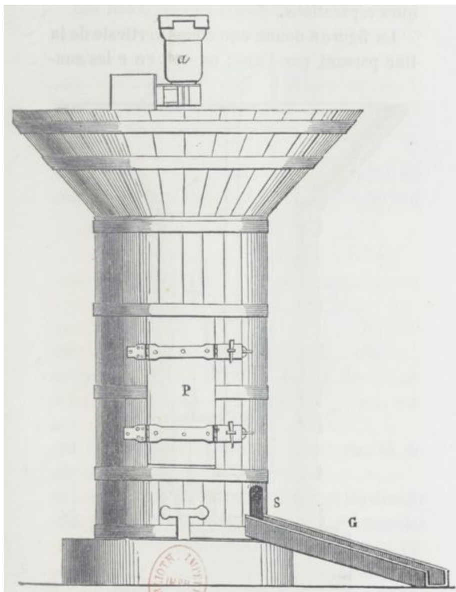
Fig. 7. — Tinc à moulures (élévation).
