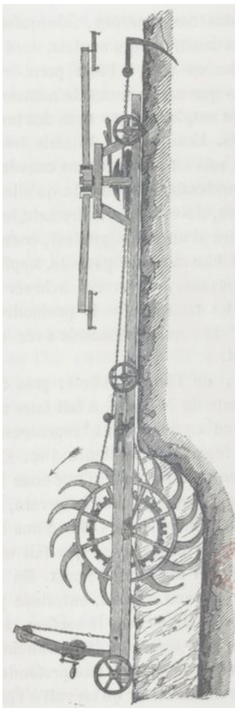
Fig. 196. — Charrue de drainage de M. Paul.
