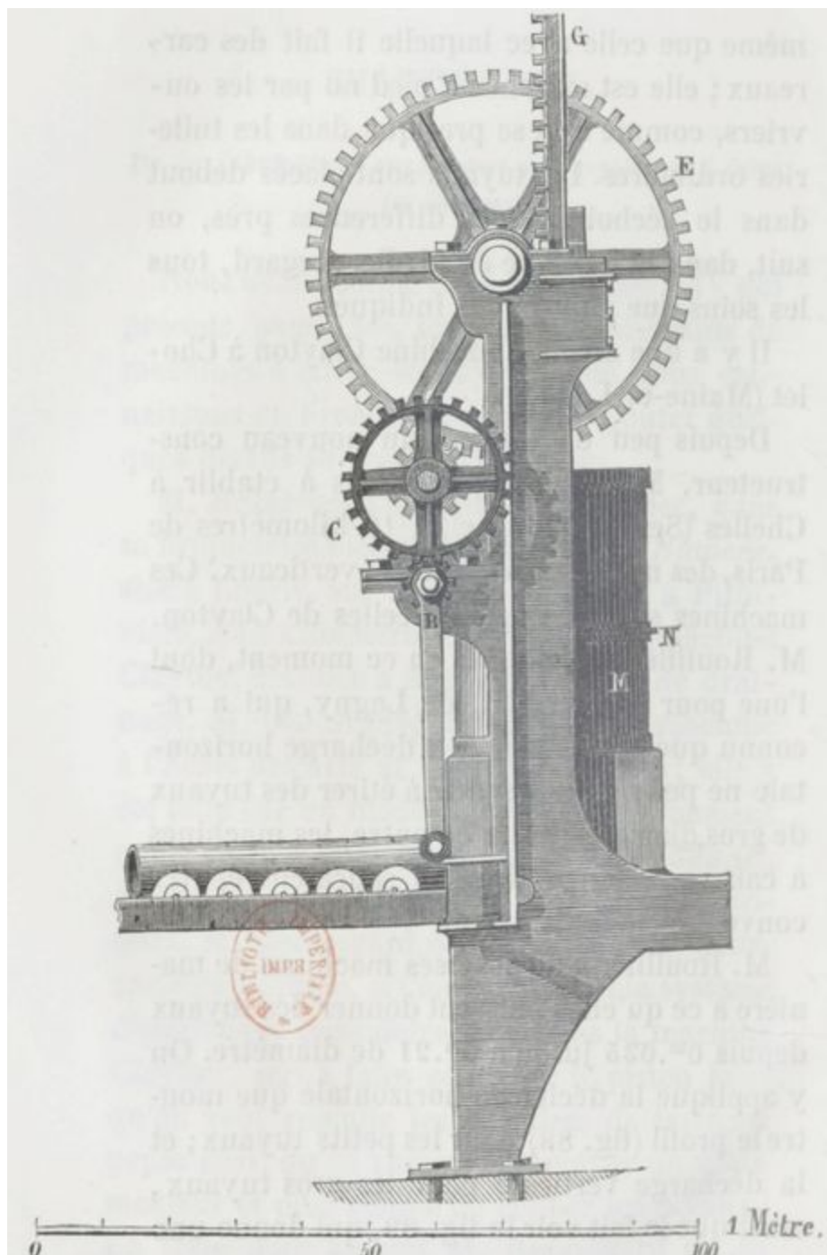
Fig. 88. — Machine à décharge horizontale de M. Rouillier.
