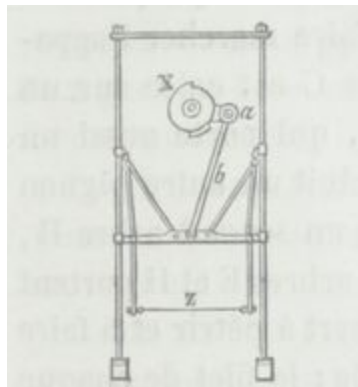
Fig. 56. — Élévation de la machine de Randell et Saunders vue par devant.
