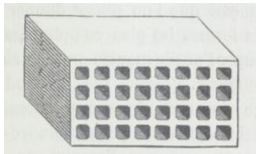
Fig. 61. — Brique tubulaire dite boutisse.
