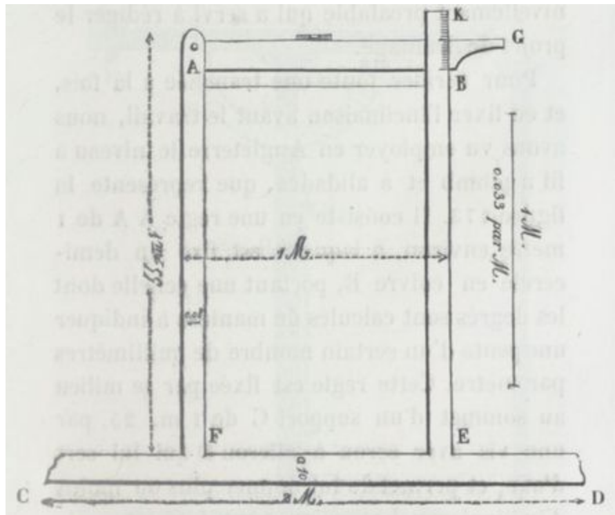
Fig. 172. — Niveau de pente de M. Laurel.
