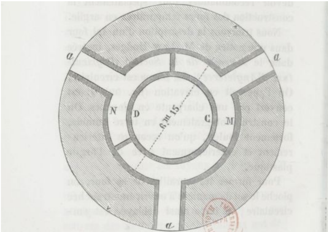
Fig. 100. — Four temporaire en terre (plan suivant la ligne AB de la coupe).
