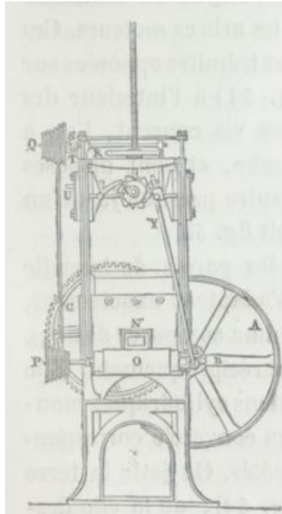
Fig. 58. — Élévation complète de la machine de Randell et Saunders du côté du moule.
