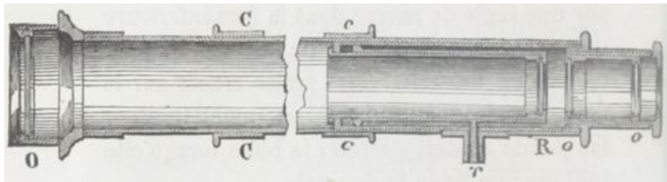
Fig. 116. — Détails de la lunette des niveaux.
