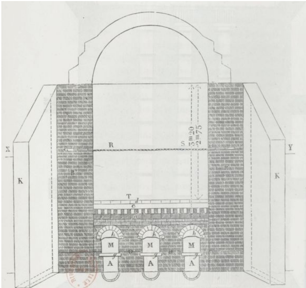
Fig. 96. — Four Clayton (élévation du côté des foyers).
