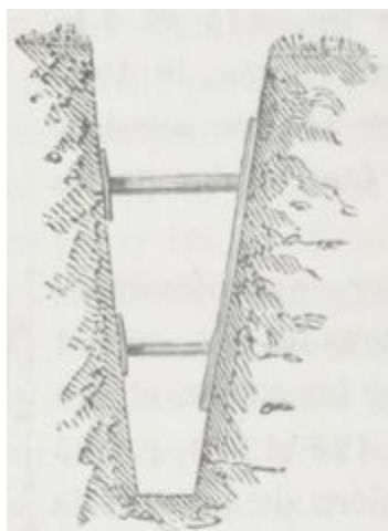
Fig. 165. — Tranchée étançonnée dans un terrain très-meuble.
