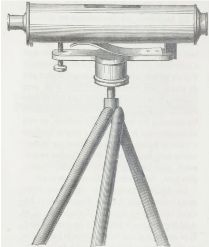
Fig. 120. — Niveau de drainage anglais.
