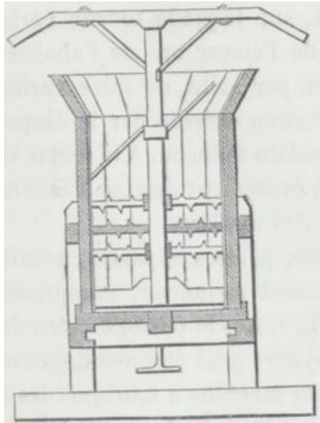
Fig. 16. — Tonneau broyeur (coupe).
