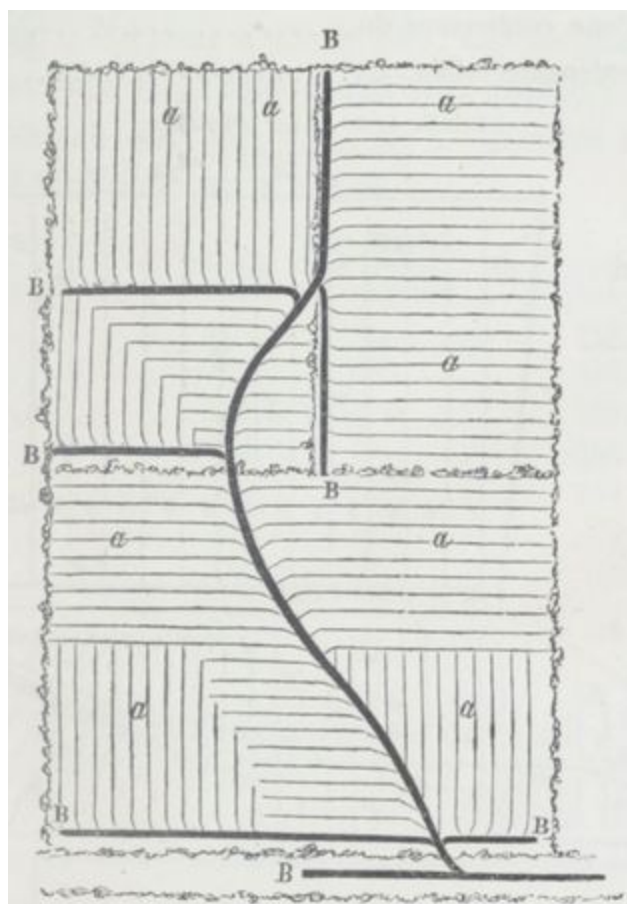
Fig. 122. — Drainage d'un champ très-accidenté.
