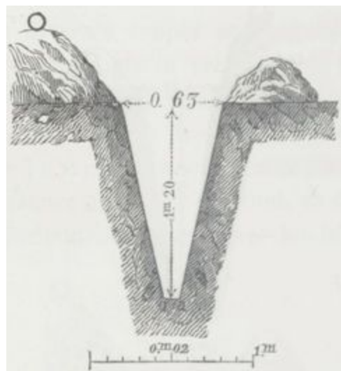
Fig. 132. — Tranchée moyenne pour les terrains pierreux.
