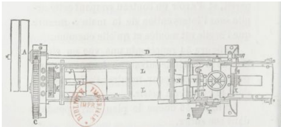
Fig. 55. — Plan de la machine de Randell et Saunders dans le sens de la longueur.
