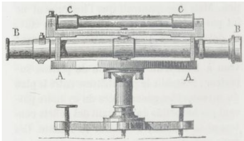
Fig. 119. — Niveau de Lenoir.
