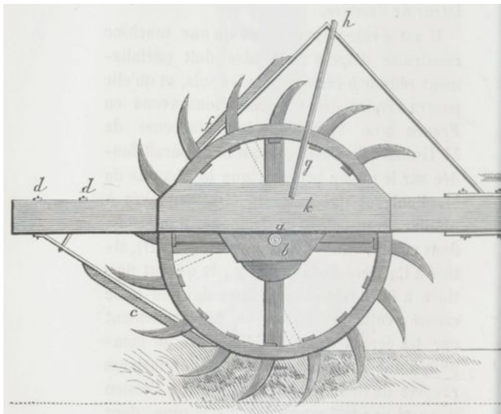
Fig. 197. — Défonceuse Guibal.
