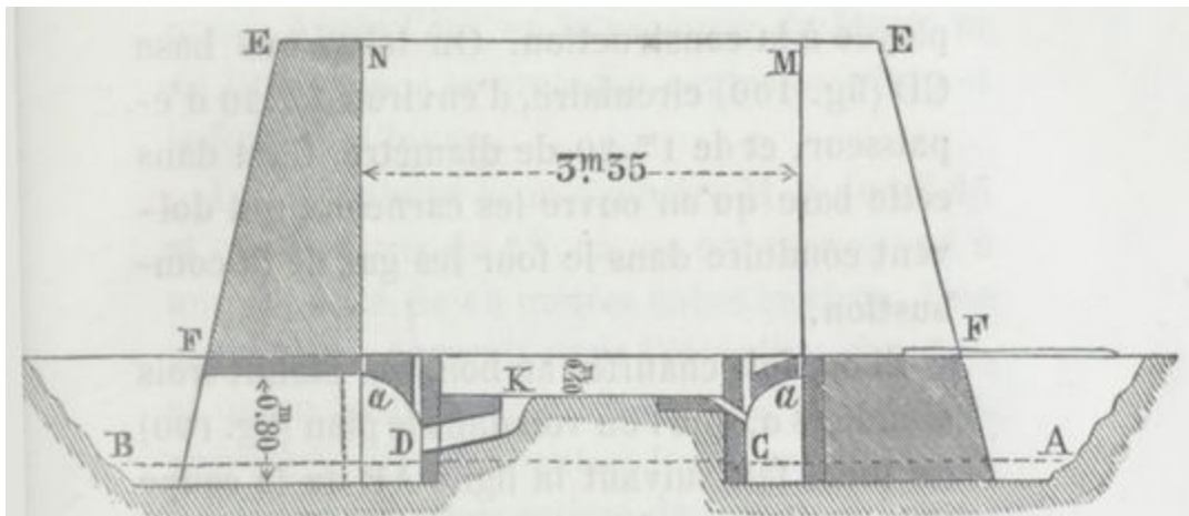
Fig. 101. — Four temporaire en terre (coupe).
