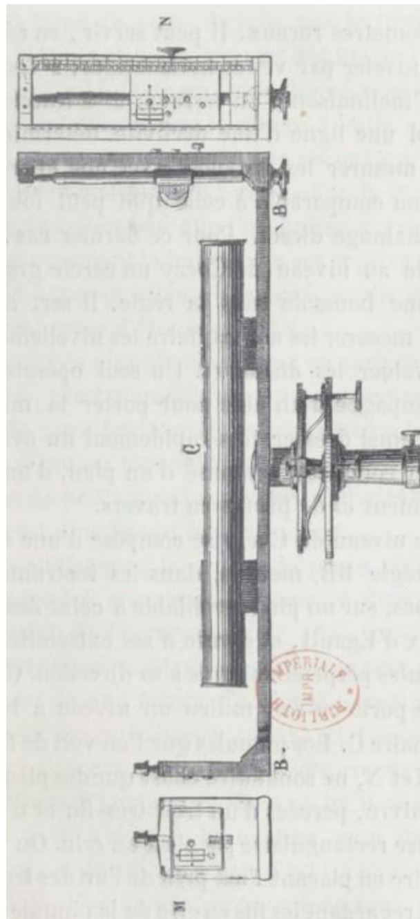
Fig. 174. — Niveau de pente de Chezy.
