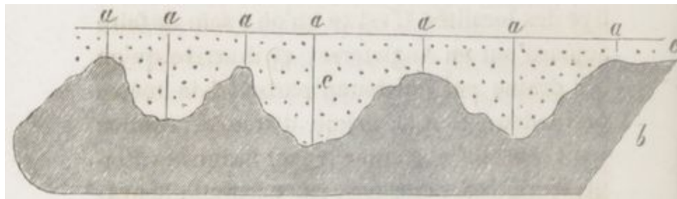
Fig. 228. — Coupe géologique de Keythorpe.
