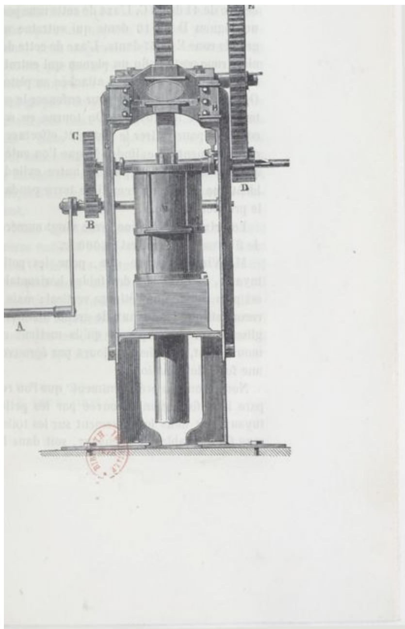
Fig. 89. — Machine à décharge verticale de M. Rouillier.
