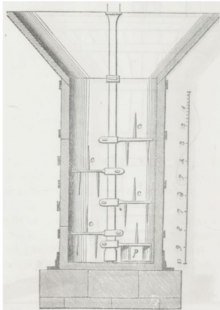
Fig. 8. — Tine à malaxer (coupe).
