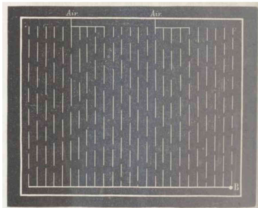
Fig. 222. — Plan d'un drainage à circulation d'air.
