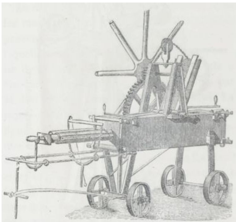
Fig. 31*. — Machine de Webster.
