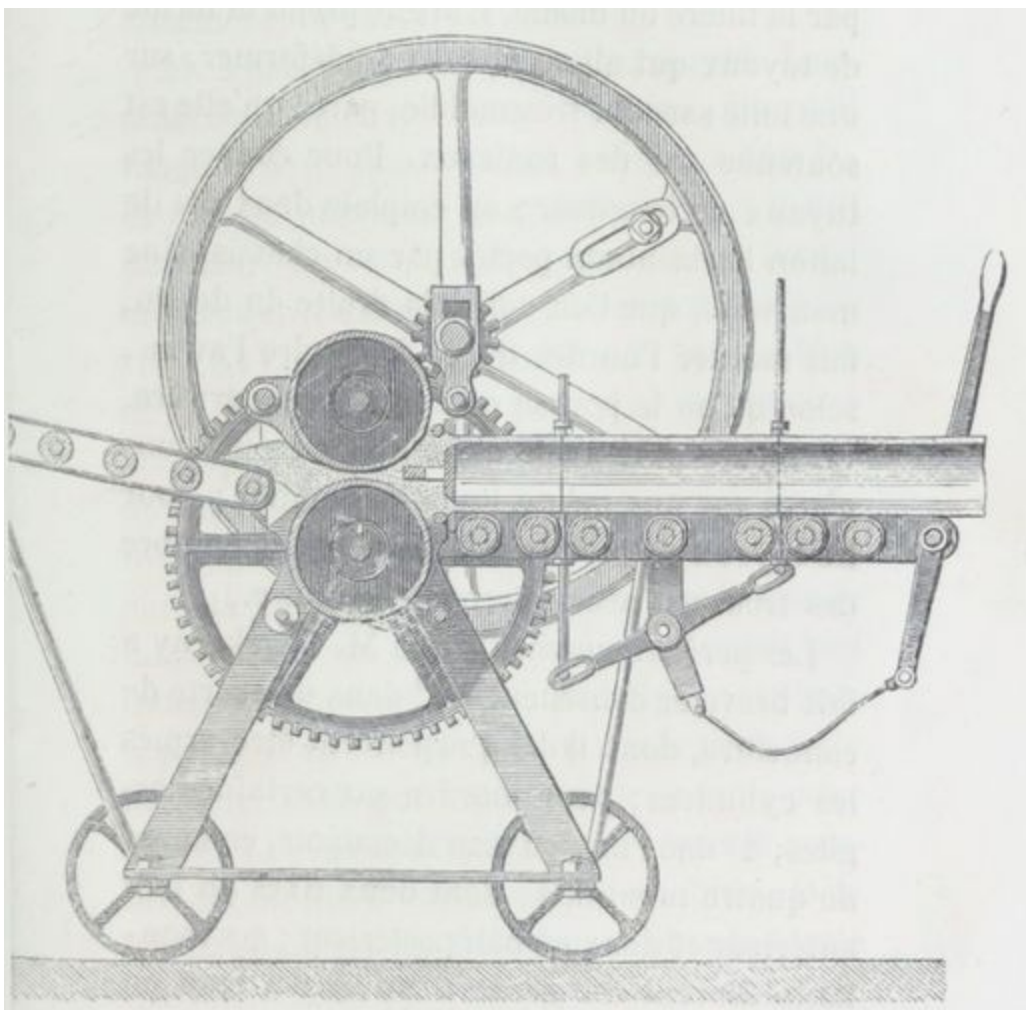
Fig. 43. — Machine d'Ainslie.
