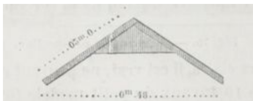
Fig. 77. — Coupe du toit couvrant les claies. superposées.
