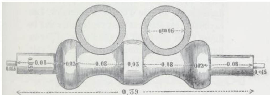
Fig. 79. — Rouleau mobile de M. Vincent.
