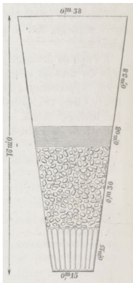
Fig. 216. — Tranchée empierrée principale.
