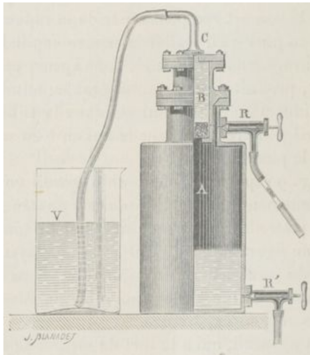
Fig. 10. Appareil filtrateur à hautes pressions.
