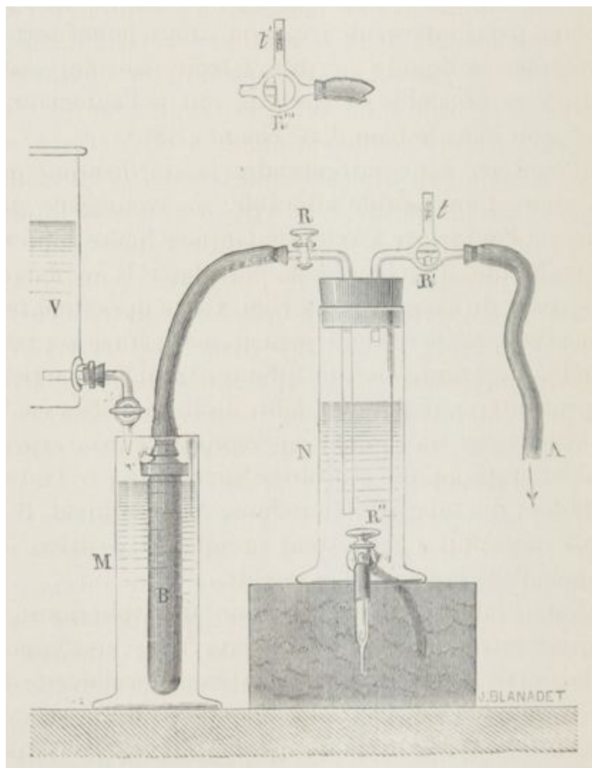
Fig.11. Appareil filtrateur construit avec une bougie Chamberland.
