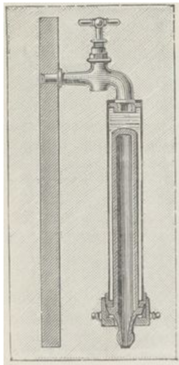
Fig. 23. Filtre Chamberland à une bougie.
