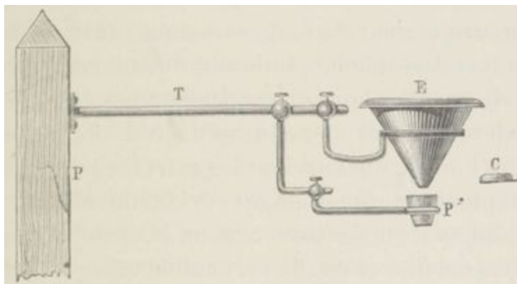
Fig. 2. Appareil pour récolter les eaux de pluie.
