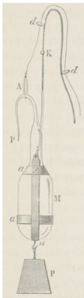
Fig. 1. Appareil pour prélever les eaux à diverses profondeurs.
