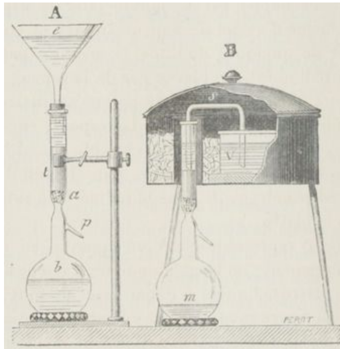
Fig. 9. Filtres de plâtre.
