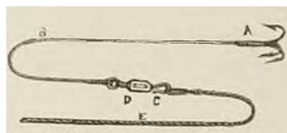
FIG. 103. — Avancée et ligne à brochet.
