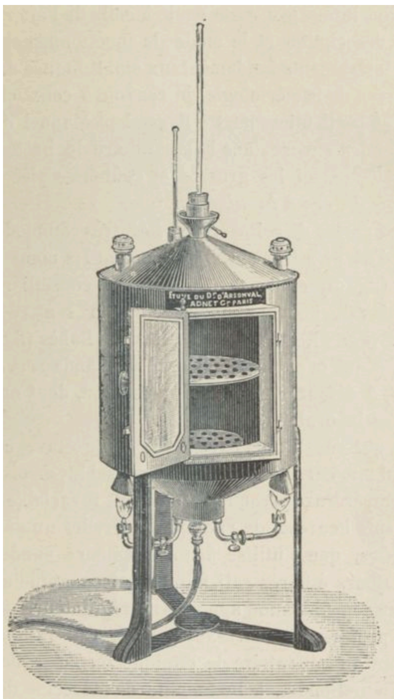
FIG. 6. — Nouvelle étuve auto-régulatrice de d'Arsonval.
