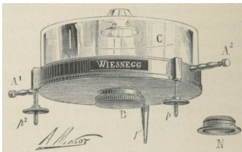
FIG. 27. — Appareil pour plaques de gélatine.
