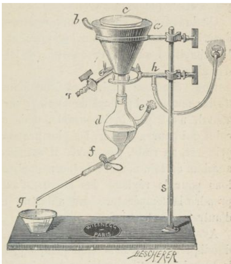
FIG. 10. — Appareil à filtration à chaud.
