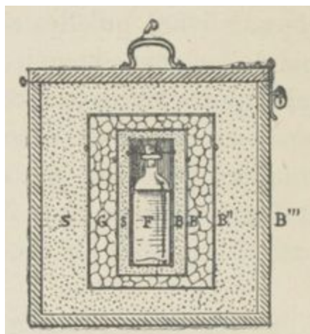
FIG. 19. — Glacière pour les long voyages.
