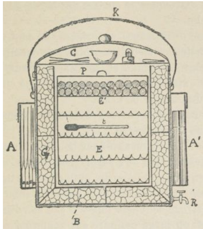
FIG. 20. — Nécessaire bactériologique du D r G. Roux.
