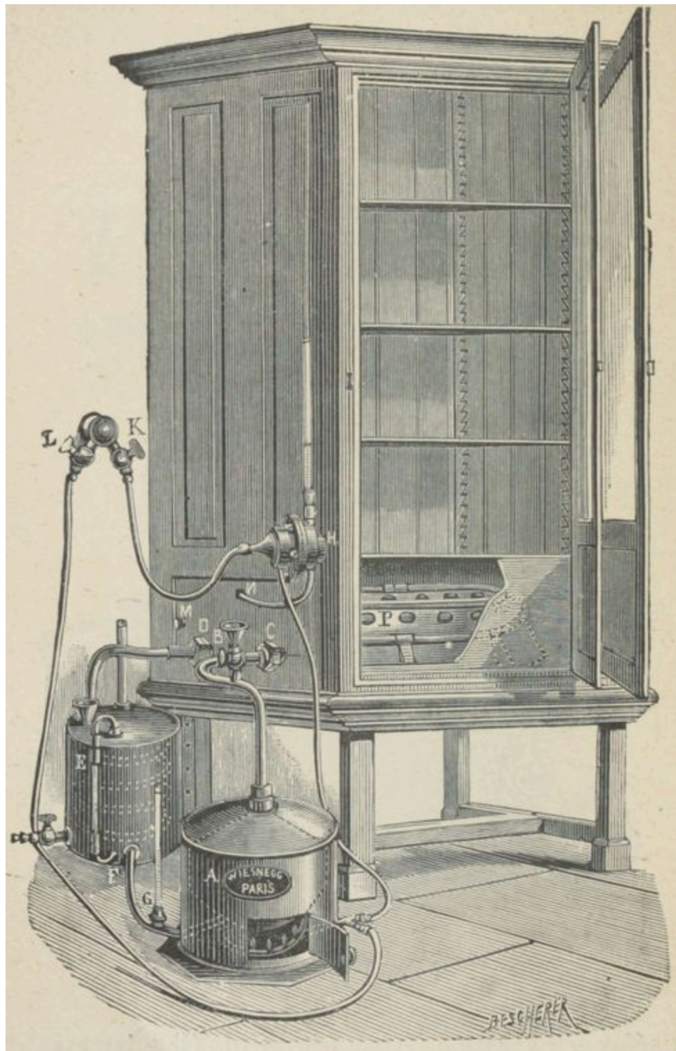
FIG. 5. — Etuve de Pasteur.
