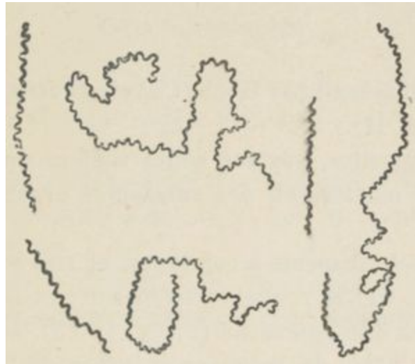
FIG. 61. — Spirillum plicatile .
