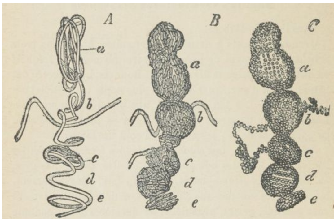
FIG. 60. — Bacillus Zopfii .
