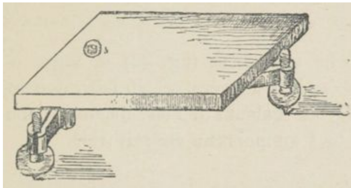
FIG. 26. -- Planchette à vis calantes.
