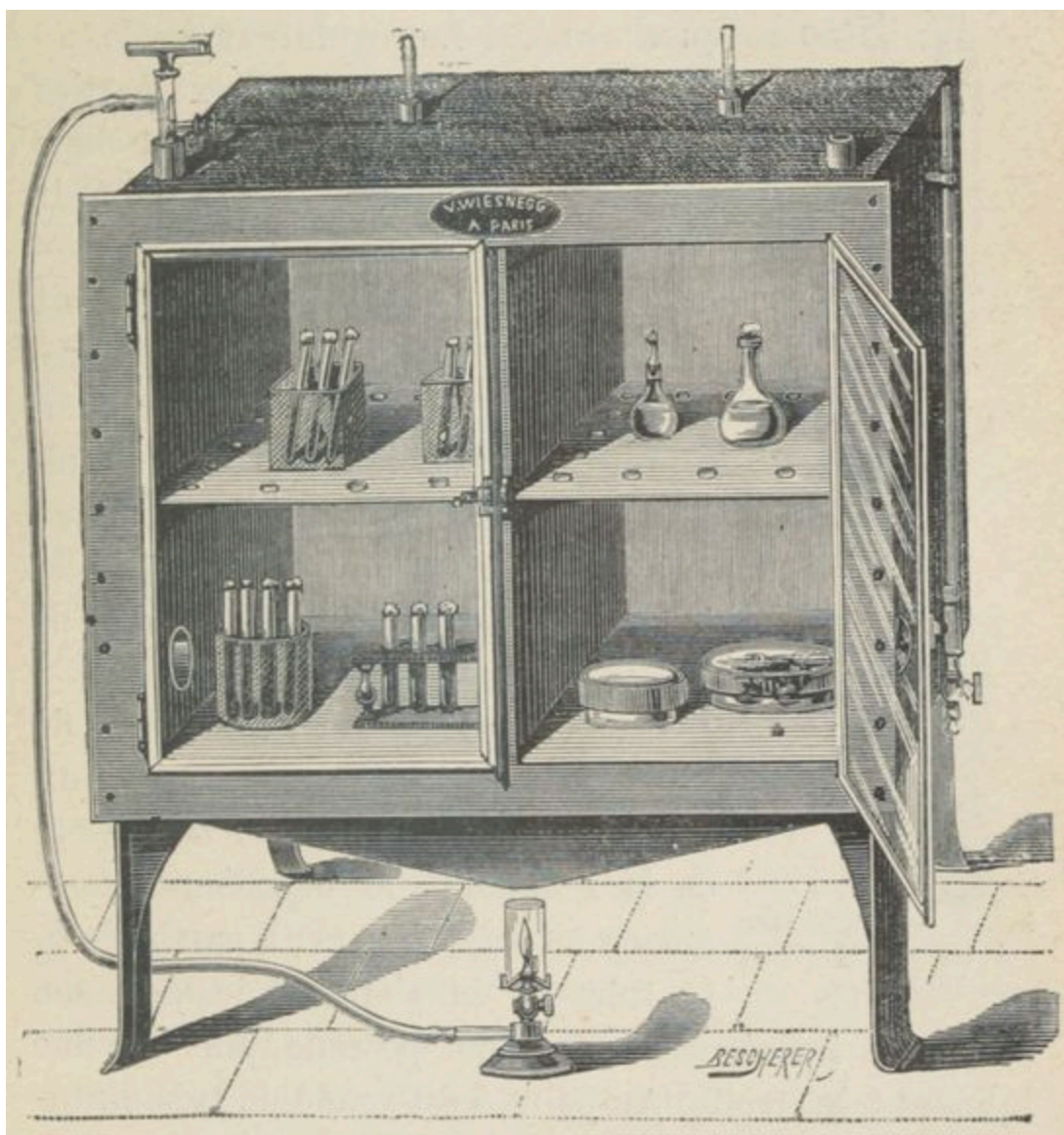
FIG. 7. — Grande étuve, modèle Babès, à deux compartiments.
