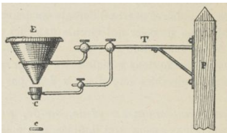
FIG. 18. — Appareil pour récolter les eaux de pluie.
