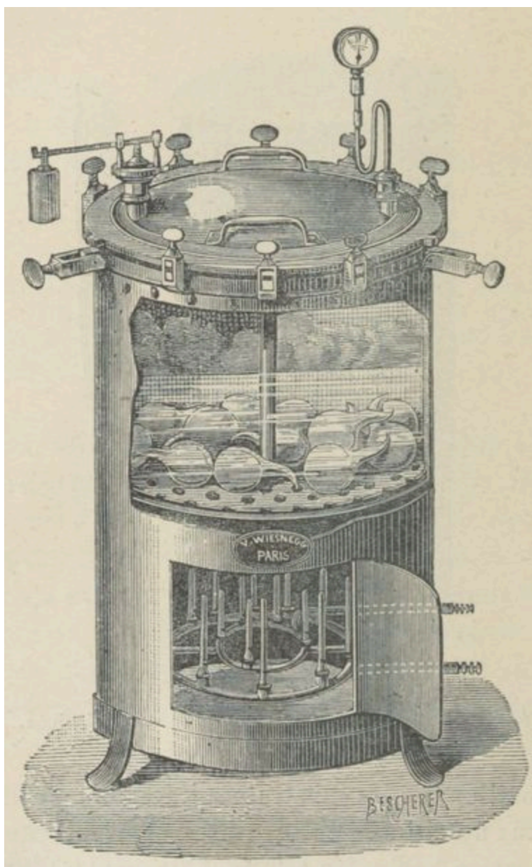
FIG. 3. — Autoclave de Chamberland.
