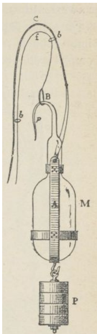
FiG.16. — Appareil pour prélever les eaux à diverses profondeurs.
