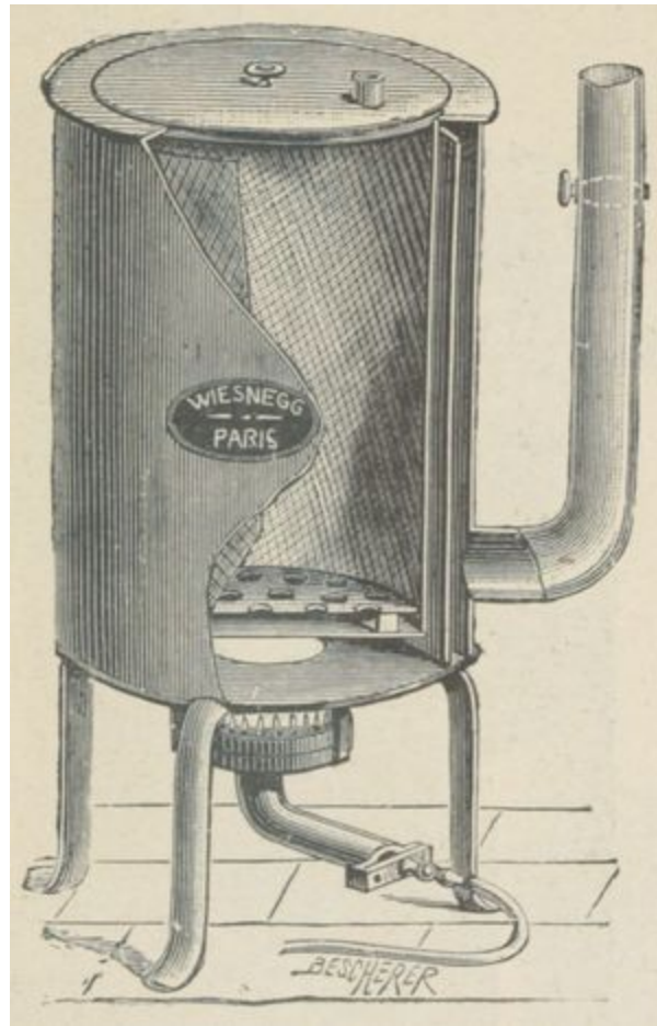
FIG. 2. — Four de Pasteur, pour flamber les ballons.
