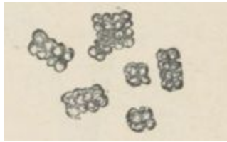
FIG. 49. — Sarcina ventriculi. 900/1.
