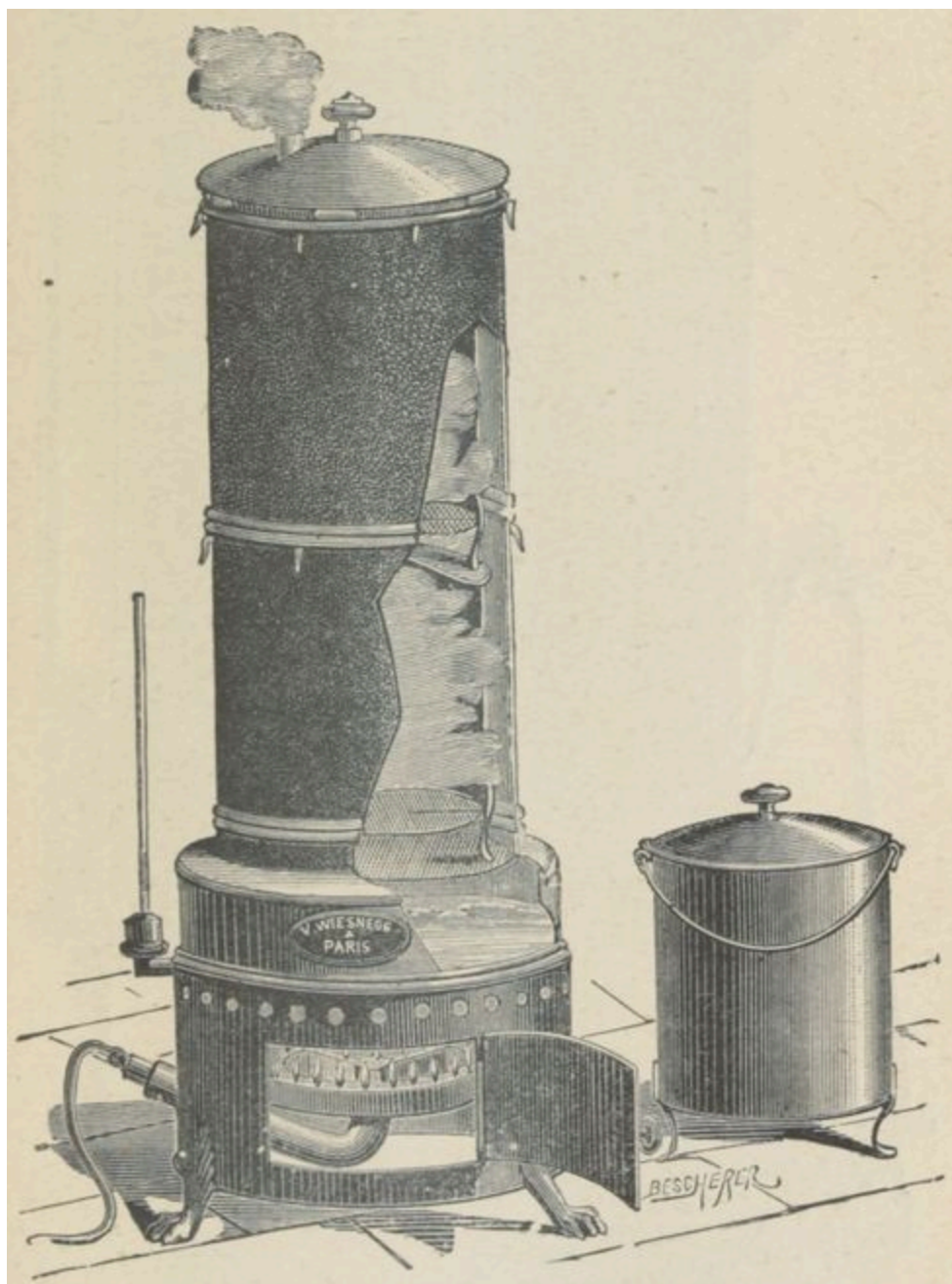
FIG 4. — Stérilisateur à vapeur de Koch
