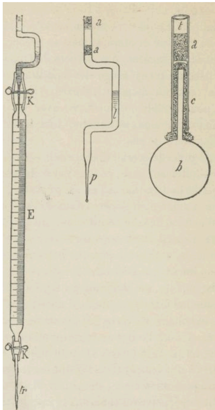
FIG. 25. — Appareils de Fol, pour l'analyse de l'eau.
