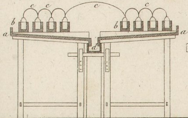
Fig. 1 re Coupe suivant la ligne A B.
