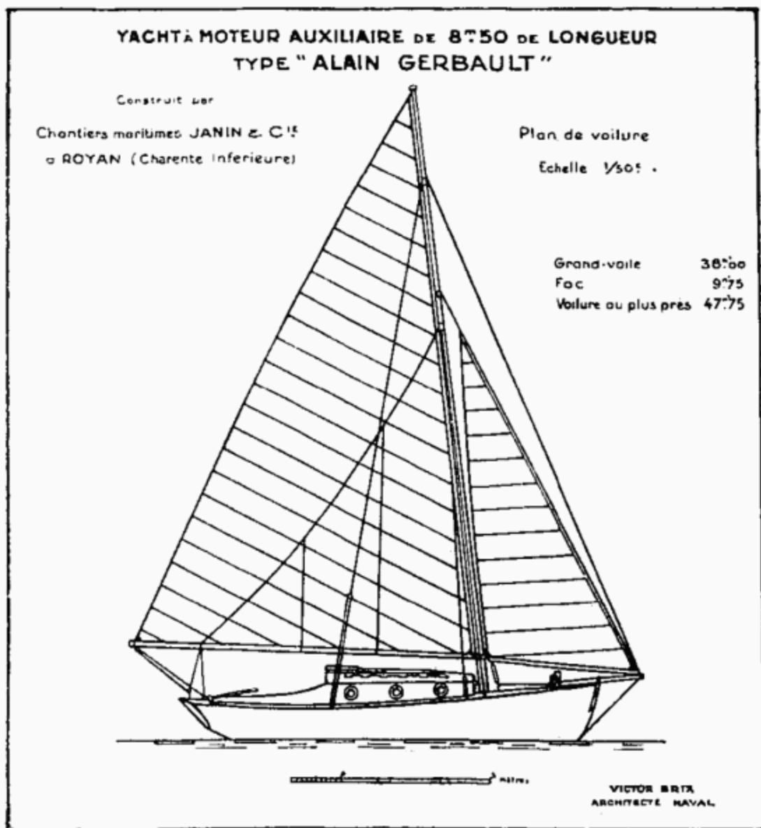
PLAN DU YACHT à moteur TYPE "ALAIN GERBAULT" Construit par Les Chantiers Maritimes JANIN et Cie à ROYAN
