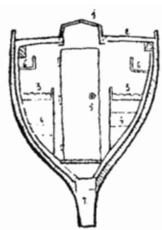
COUPE DE LA CABINE Regardant vers l'avant
