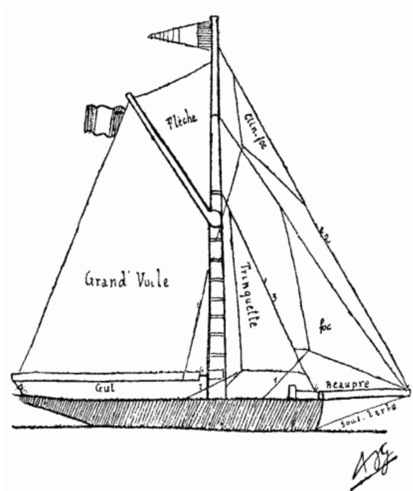
LE PLAN DE VOILURE DU Firecrest (dessiné par Alain Gerbault).
