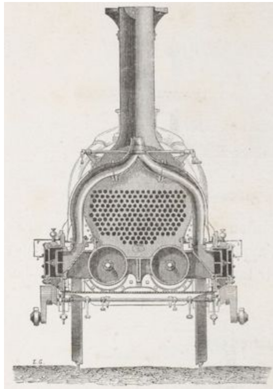
BOITE A FUMÉE D'UNE LOCOMOTIVE.
