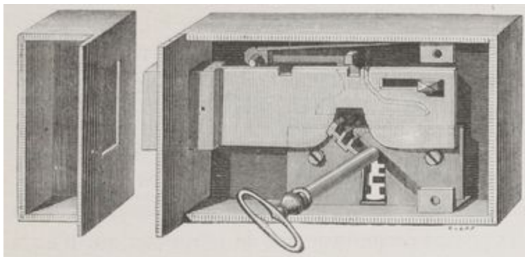
SERRURE A UN TOUR.
