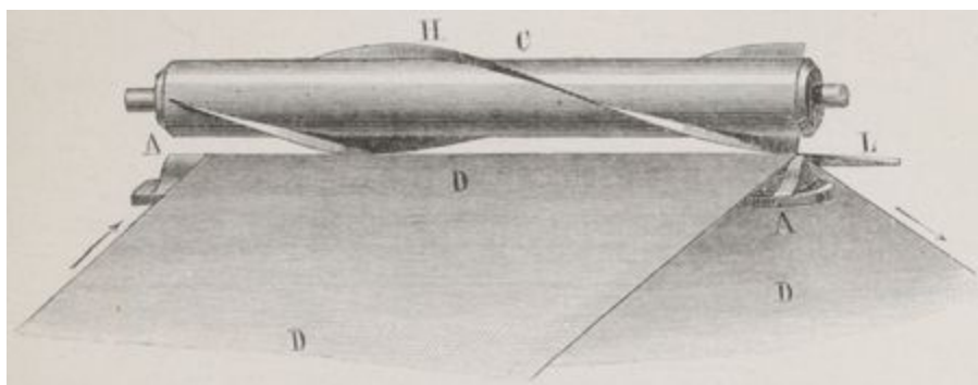
TONDAGE DES ÉTOFFES.
