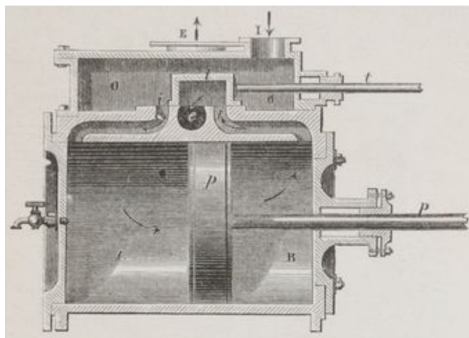
TIROIR (première position).
