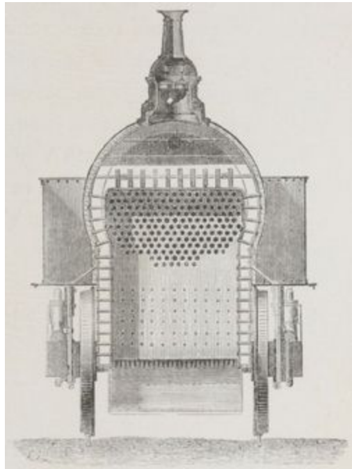
BOÎTE A FEU D'UNE LOCOMOTIVE.
