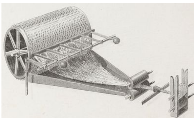
DÉTAILS DU PEIGNE BATTANT.
